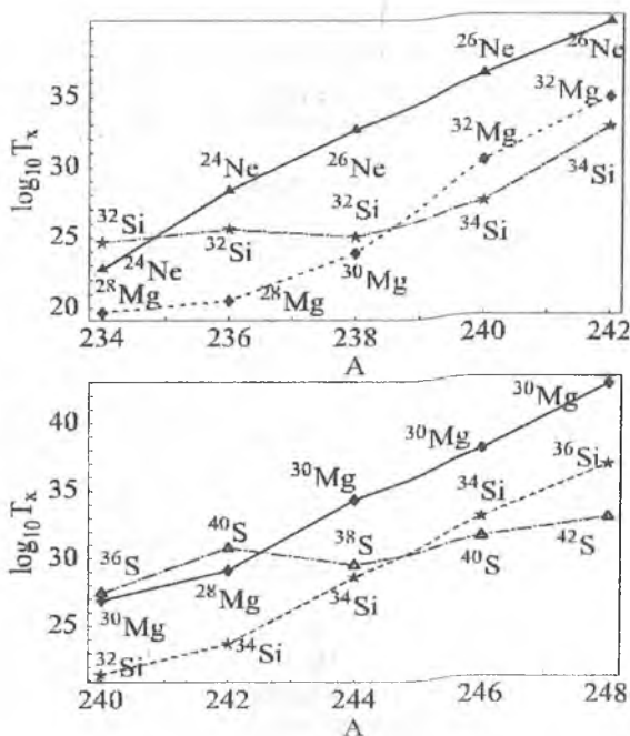
1.19-rasm. Hisoblangan yarim parchalanish davrining dastlabki(birlamchi) yadro massa soniga bog'lanishi. Bu yerda neon (qora uchburchak), magniy (qora romb) va kremniy(yulduzcha) klasterlrining plutoniydan (yuqori grafik), va magniy, kremniy va oltingugurt (yorug' uchburchaklar) klasterlarining kyuriydan (pastki grafik) chiqishi uchun. Nuqtalar yonida engil klasterlarning massa soni ko'rsatilgan.
