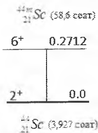
1.9-rasm. Skandiy-44 yadrosining asosiy va metastabil (izomer holatlarining) sathlarining sxemalari.
