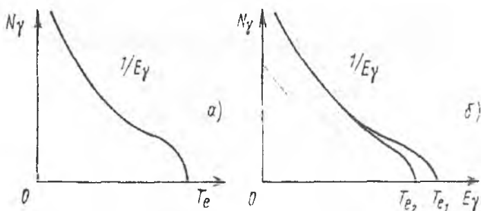
5.11-rasm. Tormozli nurlar spektri: a – energiyasi T_e bo'lgan elektronlar hosil qilgan spektr; energiyalari T_{e1} va T_{e2} bo'lgan elektronlar hosil qilgan spektrlar.
