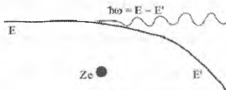
3.1-rasm. Zaryadi Ze bo'lgan yadro Kulon maydonidagi elektronning tormozlanish nurlanishi.
