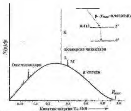
1.10 –rasm. Konversiya spektri atom qobig' energiyalari farqiga ko'ra to'g'ri keluvchi bir necha monoxromatik spektrlar.
