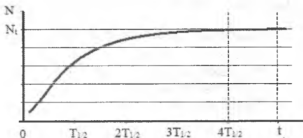
2.1-rasm. Aktivatsiya egri chiziqli
