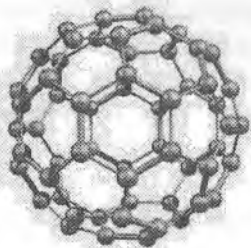
1.5-rasm. O'nlab atomlardan iborat uglerod molekulari.
