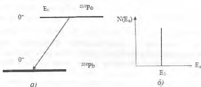
1.3-rasm. Poloniy-210 yadrosining parchalanish sxemasi (a) va \alpha -zarralar energetik spektri(b).
