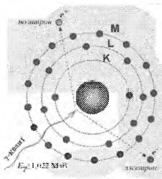
3.11-rasm. Elektron-pozitron juftining hosil bo‘lishi sxemasi.
