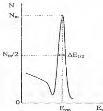
5.23-rasm. Gamma-spektr.
