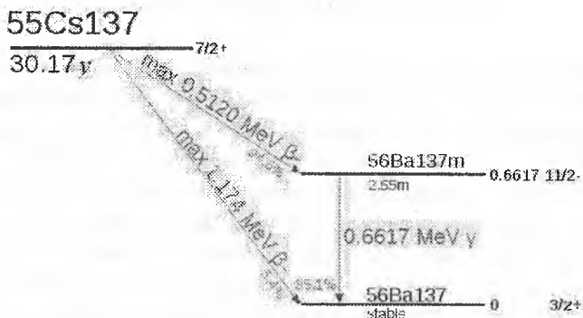
1.29 -rasm. Seziya-137 parchalanish sxemasi.
