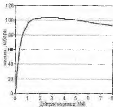
5.7-rasm. d(d,n)^3\text{He} reaksiya uchun uyg'onish funksiyasi.
