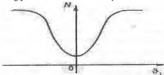
3.9-rasm. Qayd qilingan reaksiya mahsuloti bo'lgan N zarralar sonining tushayotgan zarralar dastasi yo'nalishi bilan kristallografik o'q orasidagi \theta burchakka bog'lanishi.
