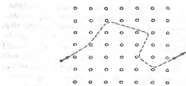
3.7-rasm. Ko'ndalang tekislikda bunday zarraning harakati umumiy holda tasodifiy "tentirash" ni ifodalaydi
