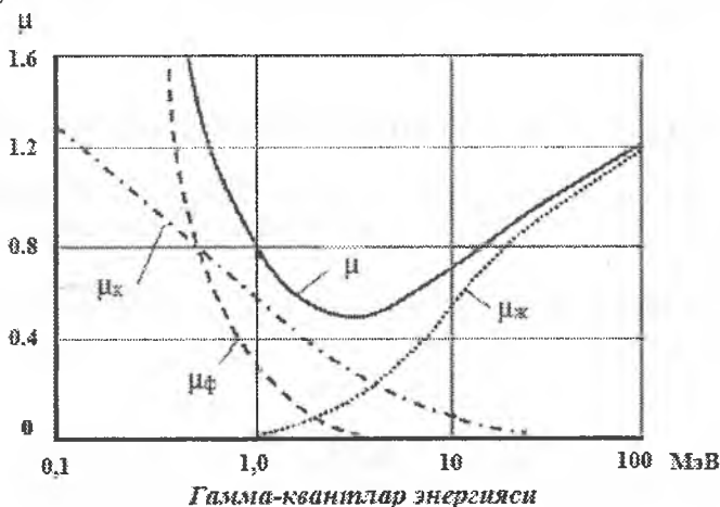
3.10-rasm. Qo'rg'oshin uchun \gamma -nurlar chiziqli yutilish koeffitsientining \gamma -kvantlar energiyasiga bog'lanishi.
