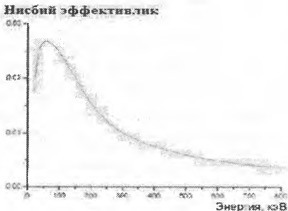
5.24-rasm. Nisbiy effektivlikning gamma-kvantlar energiyasiga bog'lanishi
