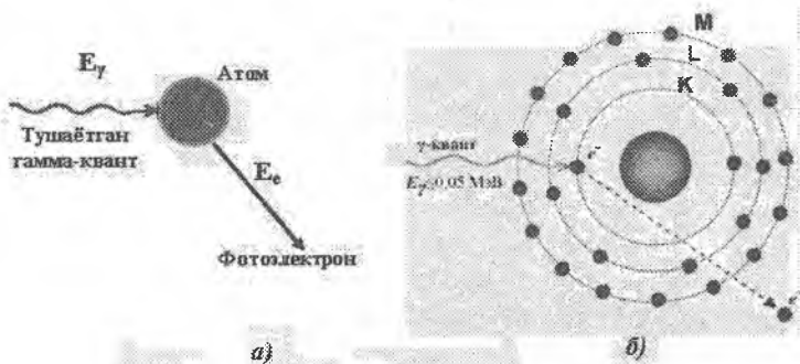
3.10-rasm. Fotoeffekt jarayonining sxemasi
