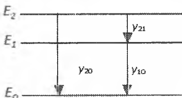
1.6-rasm. \gamma - o'tishlar sxemasi.
