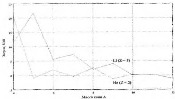
1.23-rasm. He ( Z = 2 ) va Li ( Z = 3 ) izotoplarida neytronni ajratish energiyasi.
