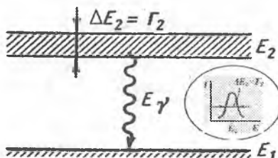
1.11-rasm. Uygʻongan holat sath va chiziqining tabiiy kengliklari.
