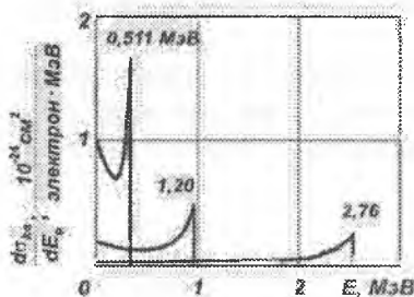
2.6-rasm. Tepki elektronlar spektri.
