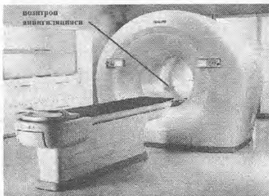
4.9-rasm. PET diagnostik (tashxislovchi) qurilmasidagi elektron-pozitron juftliklarining annigilyasiyasi.
