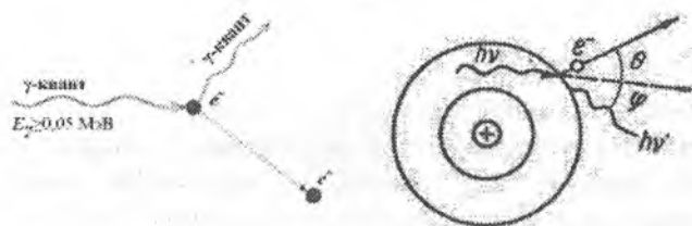
3.11-rasm. Kompton effektining yuz berish sxemasi
