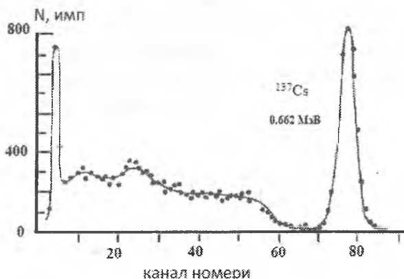
5.21-rasm. Cs-137 radionuklidning γ-spektri
