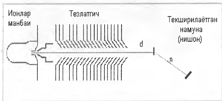
5.8-rasm. Neytron generatorning soddalashgan sxemasi
