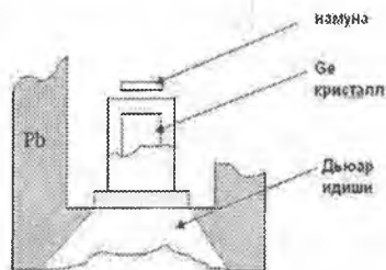
5.22-rasm. Namunaning aktivligini o'lash sxemasi
