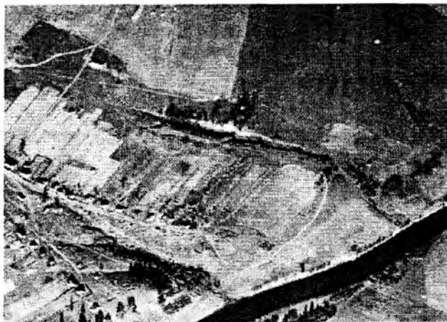
1.8-rasm. Kosmik surat.
