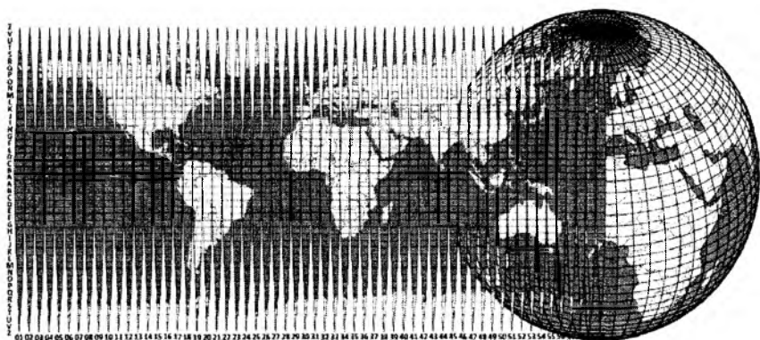
6.8-rasm. Yer sharining 60 dan 60 ta ikki burchak (ustun)larga bo'linishi.
