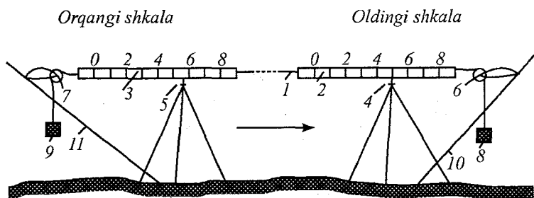
5.1-rasm. 1 — o'lchash simi; 2 va 3 — simning oldingi va orqangi shkalalari; 4 va 5 — shtativdagi seliklar; 6 va 7 — blokklar; 8 va 9 — toshlar; 10 va 11 — blokli stanoklar.
