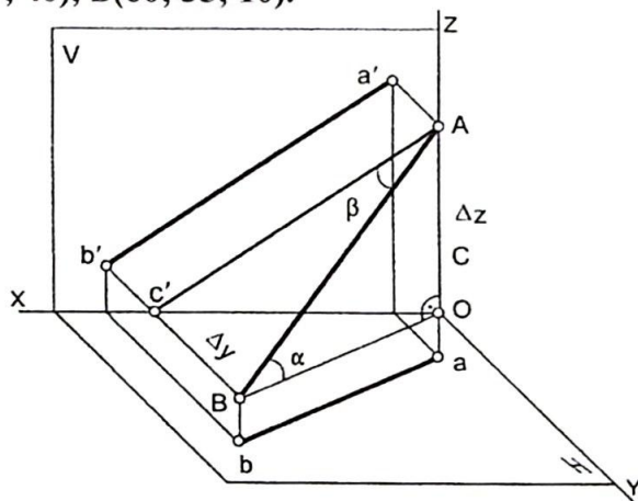
2.2 - chizma.
