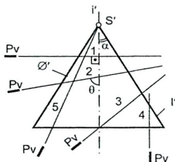
6.22 - chizma.
