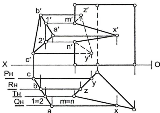
7.3- chizma.
