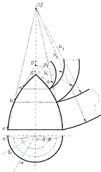
6.46 - chizma.
