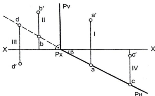
3.15 - chizma.
