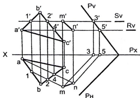
4.8 - chizma.
