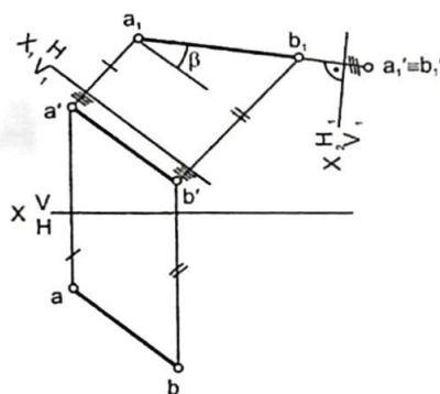
5.4 - chizma.
