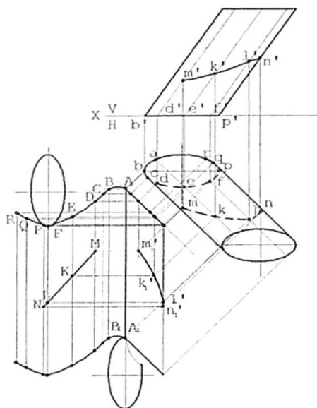
6.35 – chizma.
