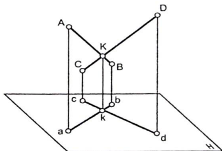
2.22 - chizma.
