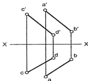
2.21 - chizma.
