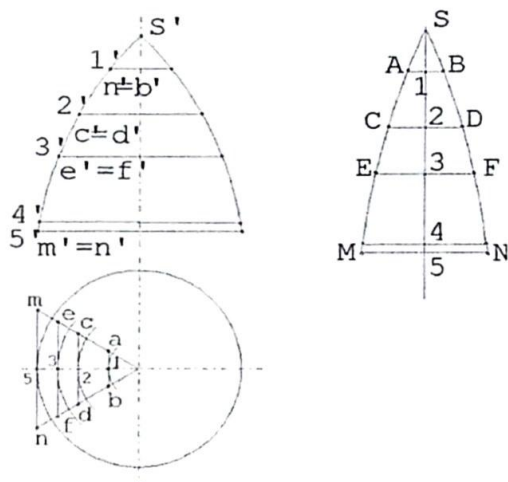
6.45 - chizma.
