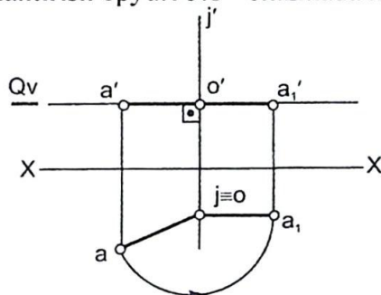
5.8 - chizma.
