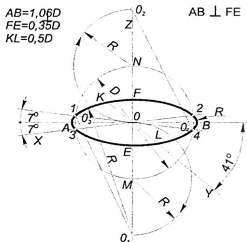
9.9 - chizma.
