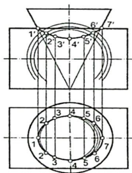
7.8 - chizma.
