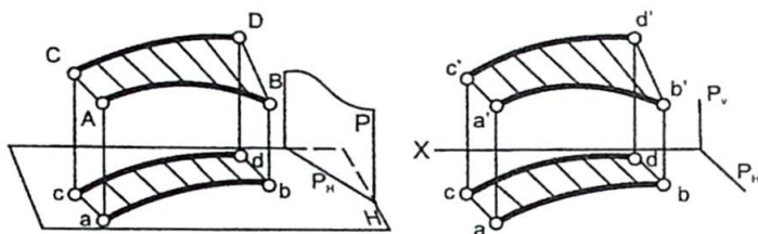
6.5 - chizma.
