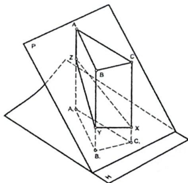
6.25 - chizma.
