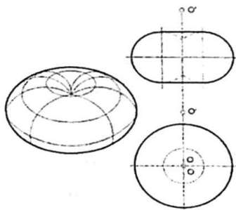
6.10 - chizma.
