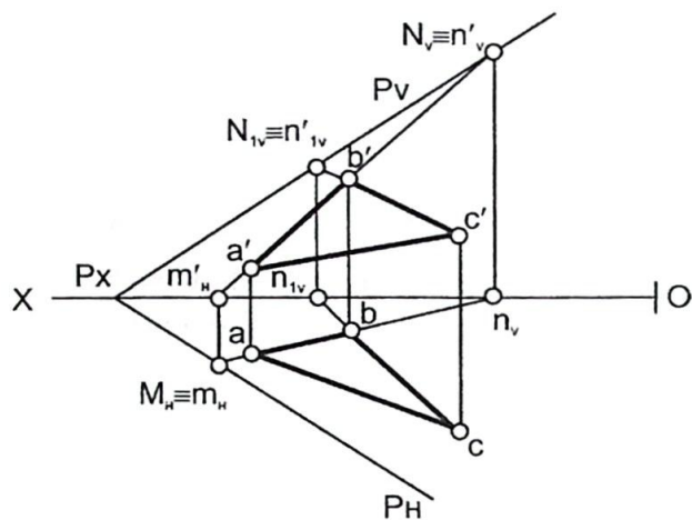
3.7 - chizma.
