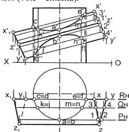
10.5 - chizma.
