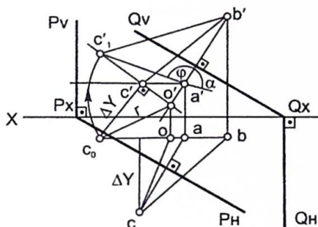
8.4 - chizma.
