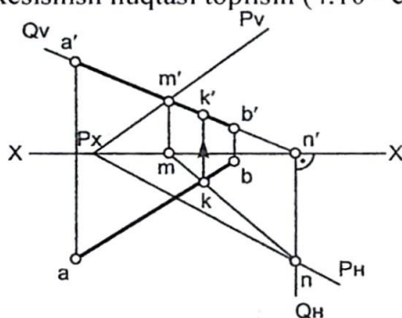
4.10 - chizma.
