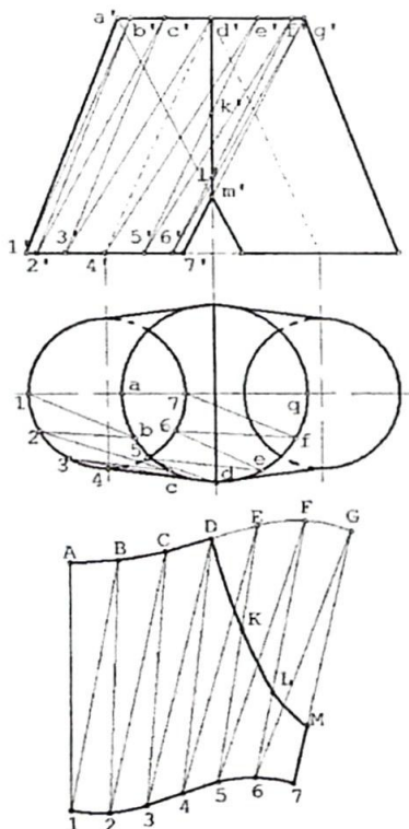
6.49 - chizma.
