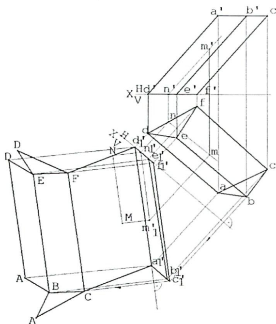
6.31 - chizma.
