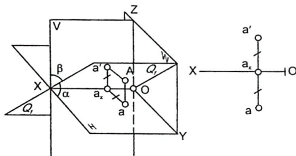
3.20 - chizma.
