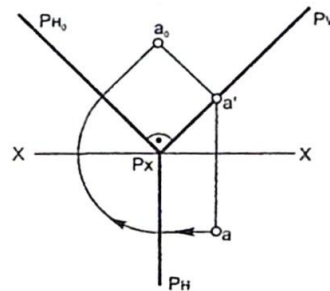
5.18 - chizma.
