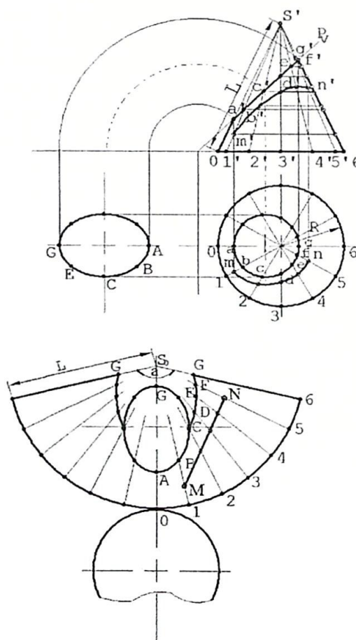
6.37-chizma.
