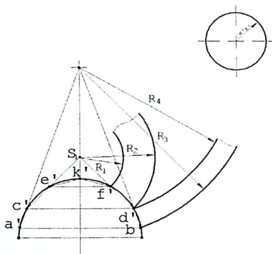
6.44 - chizma.
