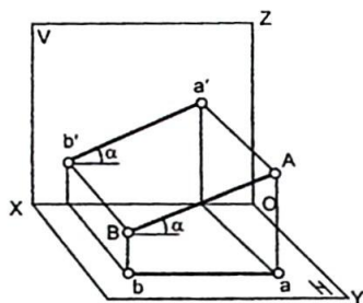
2.8 - chizma.
