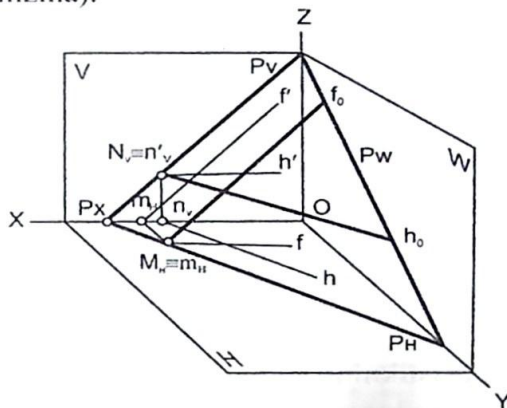
3.26 - chizma.
