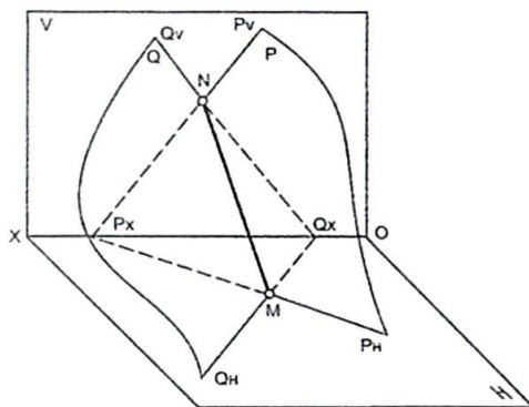
4.5 - chizma.
