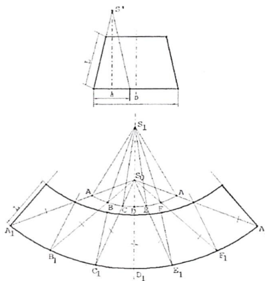
6.40 - chizma.
