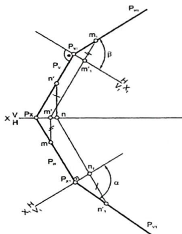
5.6 - chizma.
