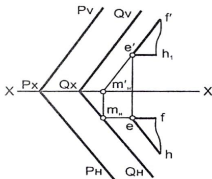
4.25 - chizma.
