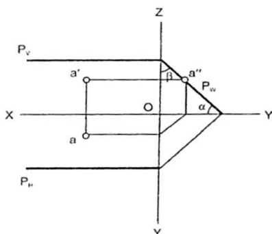
3.19 - chizma.
