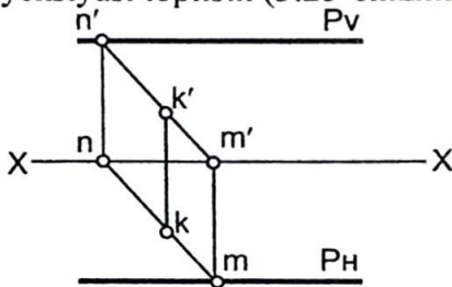
3.25 - chizma.
