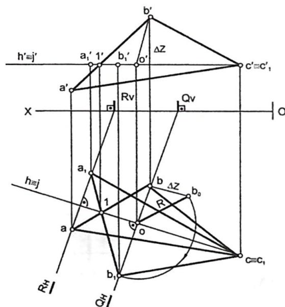
5.13 - chizma.
