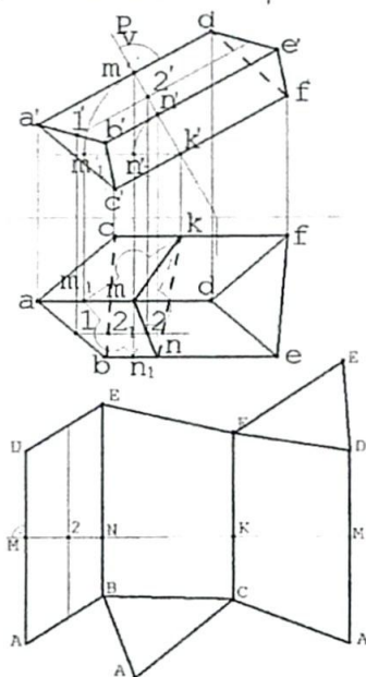
6.30 – chizma.
