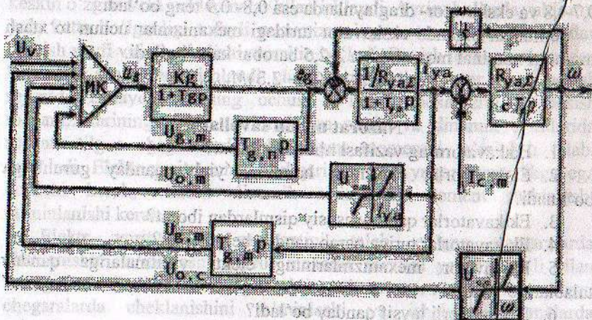
9.1-rasm. Jamlovchi kuchaytirgichli G-M tizimning strukturali sxemasi
