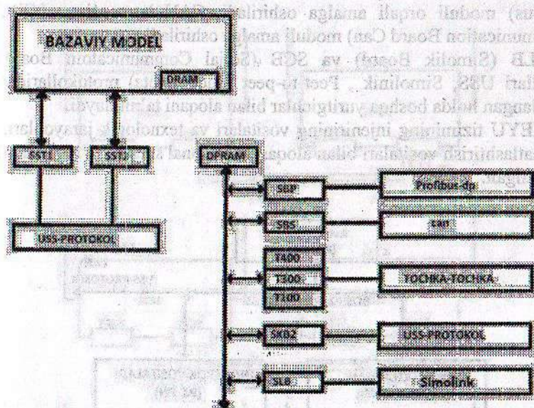
15.6-rasm. Seriyali interfeyslar to'plami
