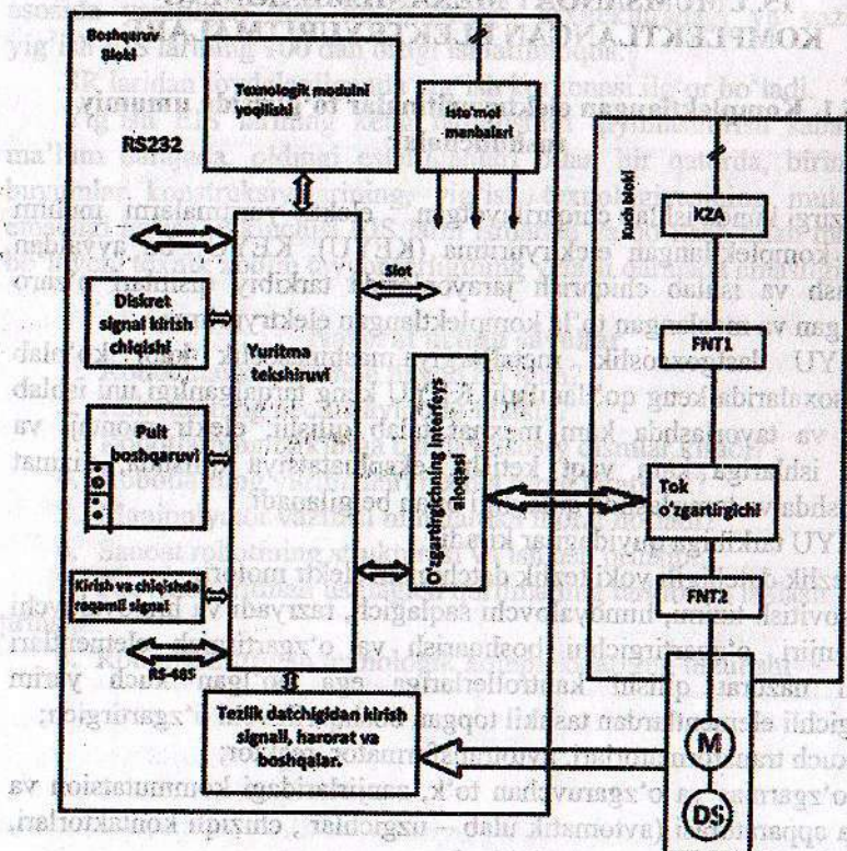
15.1-rasm. Komplektlangan elektr yuritmaning namunaviy tuzilish sxemasi
