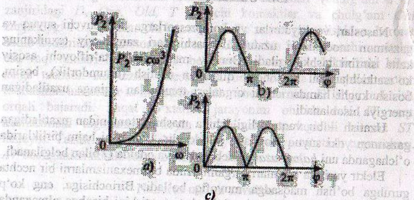
13.1-rasm. Motor validagi quvvatning tezlik va krivoship burilishining burchagiga bog'lanish grafiklari: a – markazdan qochma; b – bir harakatli porshenli; c – ikki harakatli porshenli.
