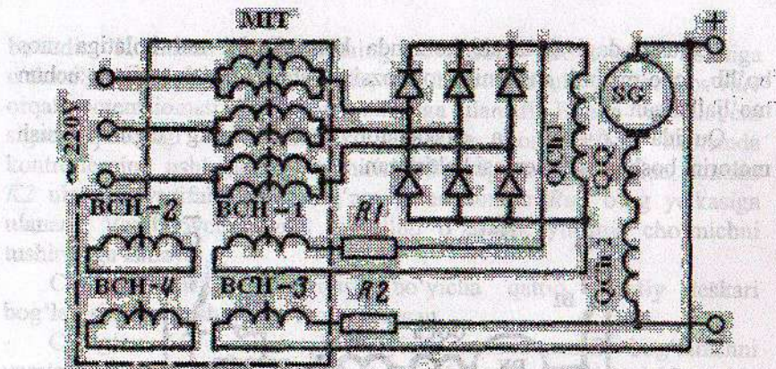
9.7-rasm. Ekskavator yuritmasi motorining qizishini bartaraf etish qismining sxemasi.
