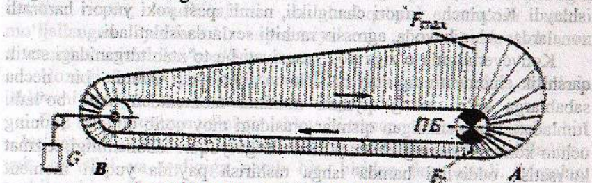
10.1-rasm. Tasmali konveyerdagi tortish kuchlarining diagrammasi.
