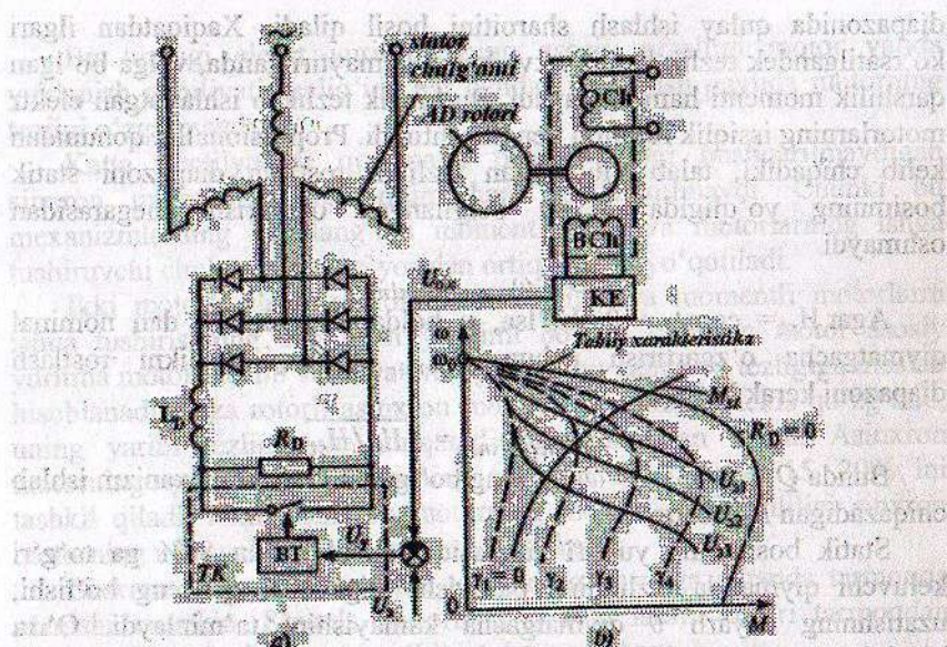
13.4-rasm. Stator zanjirining aktiv qarshiligini impulsli o'zgartiruvchi rotori qisqa tutashtirilgan asinxron motorining ulanishining sxemasi (a) va mexanik tavsiflari (b).
