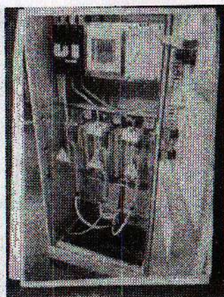
17.2-rasm . 200 kWt quvvatli elektr tejamkor qurilma kuchli bloklar va boshqarish bloklar qurilma shkafida joylashishi
