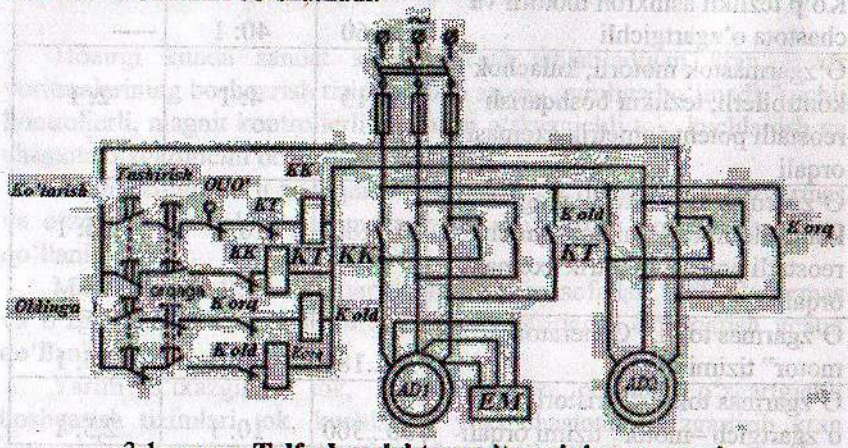
3.1- rasm . Telferlar elektr yuritmasining sxemasi.
