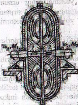
13.5-rasm. Gidromufta tuzilishi
