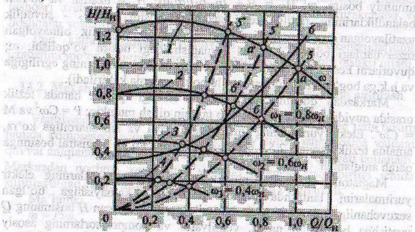
13.2-rasm. Nasos H bosimning Q uzatishga bog'liqligining tavsifi
