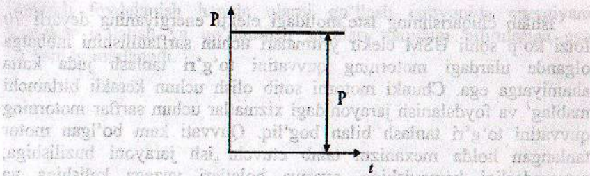
1.1-rasm. Uzoq davom etadigan ish rejimining grafigi.
