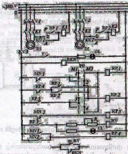
13.9-rasm. Kompresor qurilmasini avtomatik boshqarish elektr sxemasi
