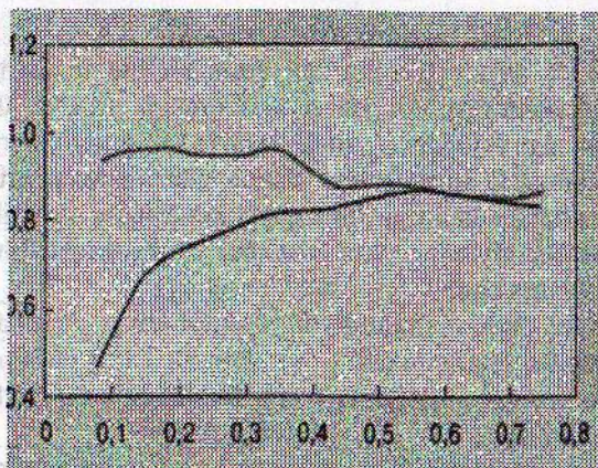
17.6-rasm. FIK (1- \eta ; 2- \eta_{\text{фопт}} ) qiymatlarini yuklanish bo'yicha o'zgarishi
