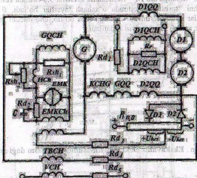
9.2-rasm. Ekskavator elektr yuritmasini mashina qo'zg'atgichli boshqarish sxemasi.
