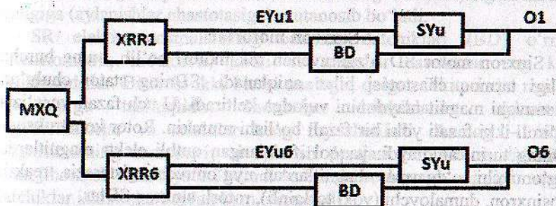
14.3-rasm. Sanoat robotlari elektr yuritmasining funksional sxemasi
