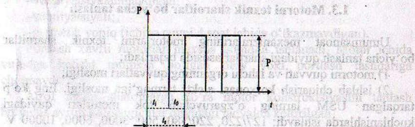
1.3-rasm . Qisqa muddatli-qaytariluvchi (siklik) ish rejimining grafigi.
