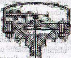
13.12-rasm. Markazdan qochma nasoslarning membranali rele tuzilishi
