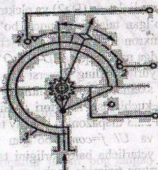
13.7-rasm . Elektr kontaktli manometr tuzilishi
