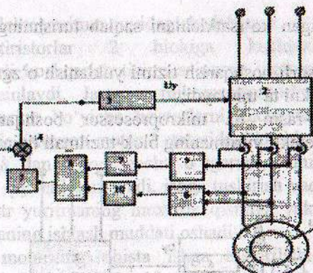
16.3- rasm . Mikroprotessor boshqaruvli energiyani tejovchi asinxron elektr yuritmaning funksional sxemasi:
