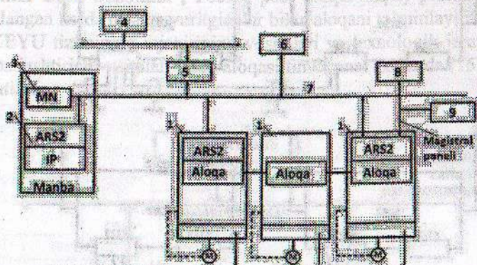
15.9-rasm. RRS-200 tizimining tarkibiy sxemasi
