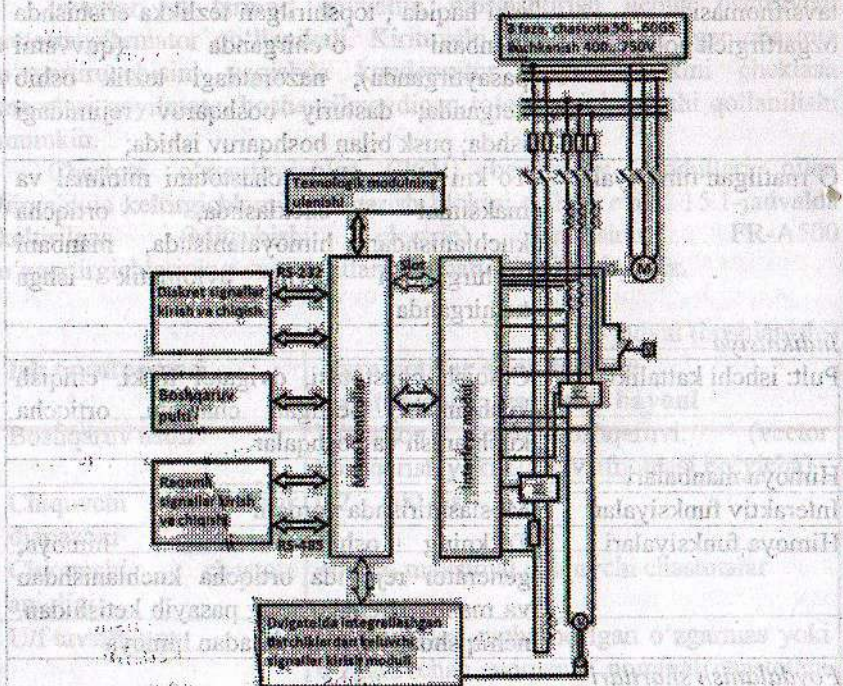
15.3-rasm. Komplekt avtomatik elektryiritmalarining standart tuzilish sxemasi
