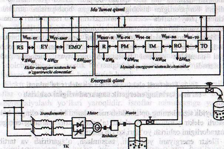
16.1-rasm. Elektr yuritmaning tuzilmasi
