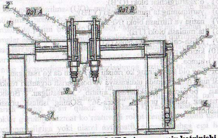
14.6-rasm. Sanoat roboti M-2IM ning umumiy ko'rinishi
