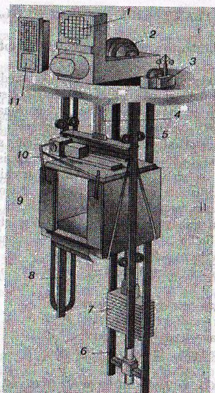
6.1- rasm . Yo'lovchi liftning umumiy ko'rinishi:
