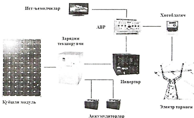
29-расм. Қуёшли фотоэлектрик батарея (аккумуляторлари билан) схемаси ва электр тармоқли коммутацияси
