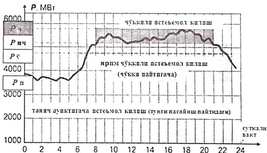
8-расм. Тигиз қисмли суткалик истеъмол графигининг мисоли
