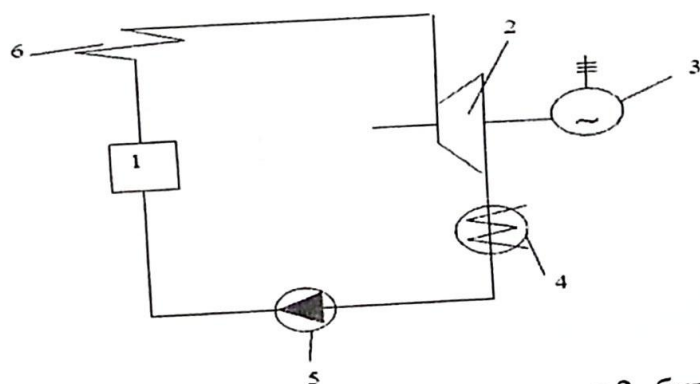
3-расм. Ренкин цикли. 1-қозон-буғ-генератори; 2- буғ-турбина; 3- электр генератори; 4- конденсатор; 5- сув насоси; 6- буғ иситгич
