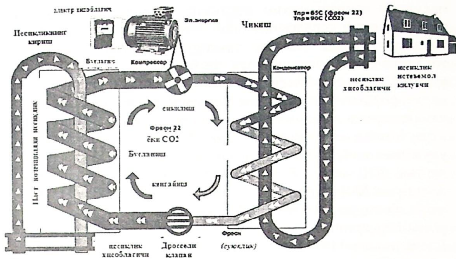
21-расм. Иссиқлик насосини ишлаш схемаси
