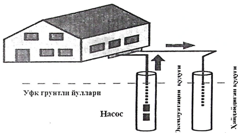
20-расм. Ерости иссиқлик энергиясидан фойдаланиш схемаси
