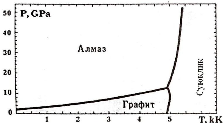
32-расм. Углероднинг тахминий фазавий диаграммаси
