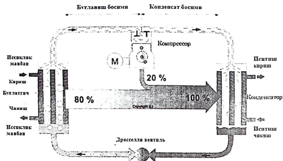
19-расм. Паст потенциалли насоснинг ишлаш принципи
