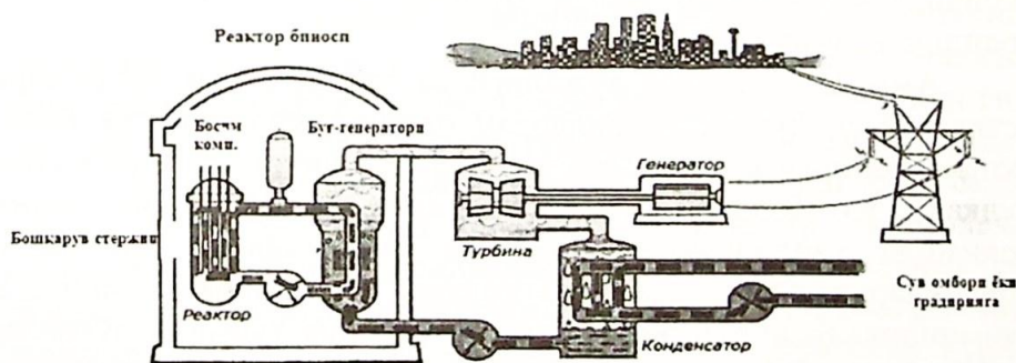
10-расм. Атом электр станциясининг ишлаш принципи
