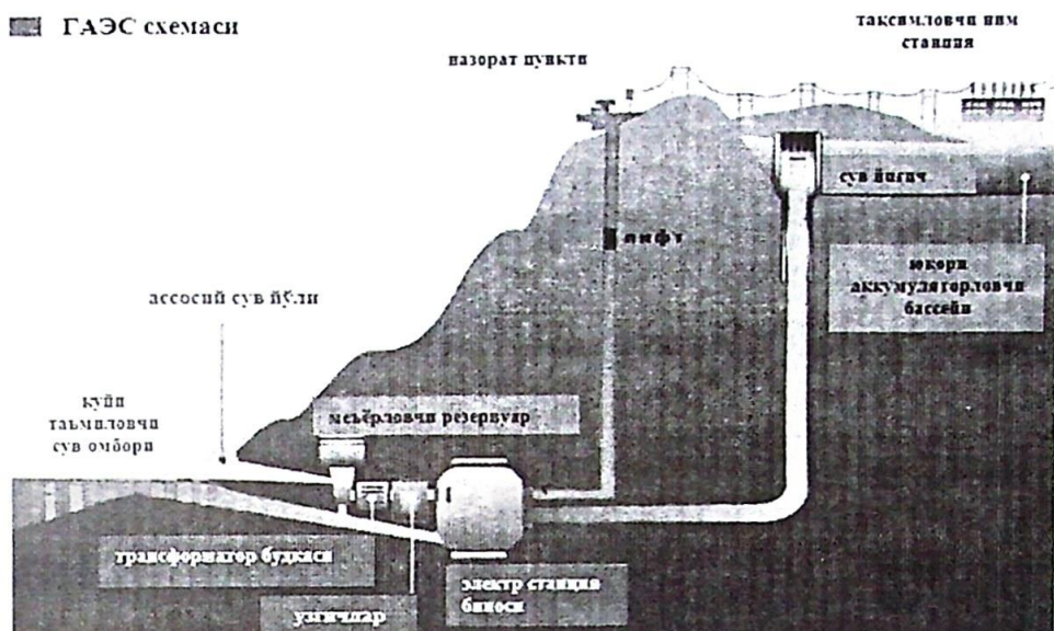
12-расм. ГАЭСнинг ишлаш схемаси
