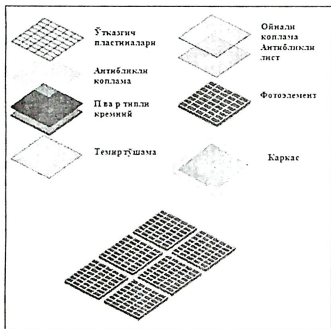
28-расм. Қуёш батареяси кетма-кет ва параллел уланган фотоэлементлардан иборат.
