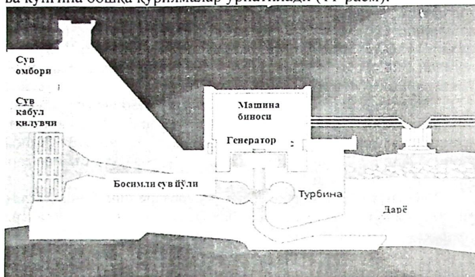
11-расм. Гидроэлектр станциясининг ишлаш принципи
