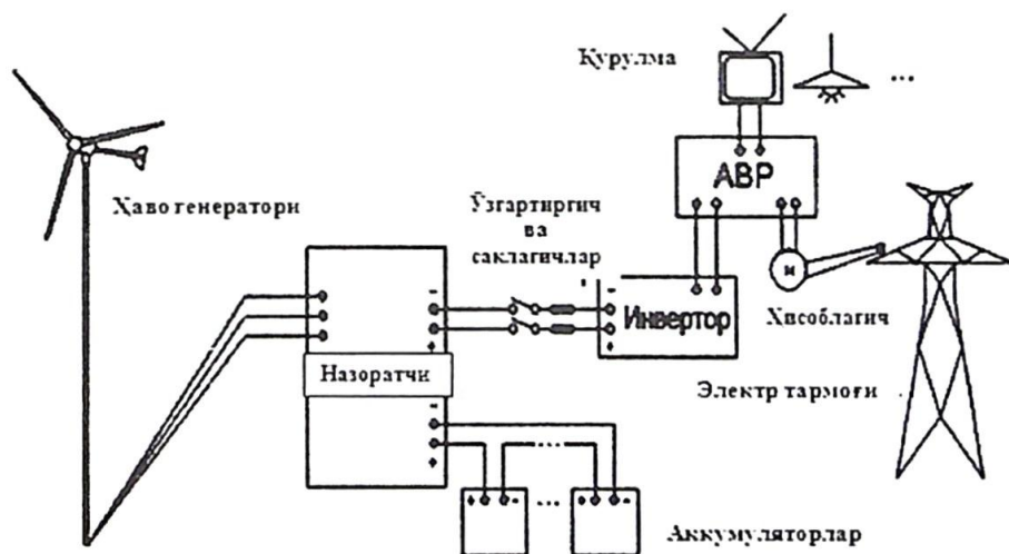
23-расм. Шамол генератори асосида электр таъминот схемаси
