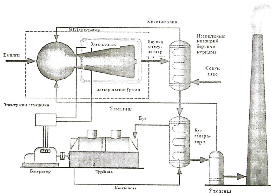
34-расм. МГД курилмасининг ишлаш схемаси
