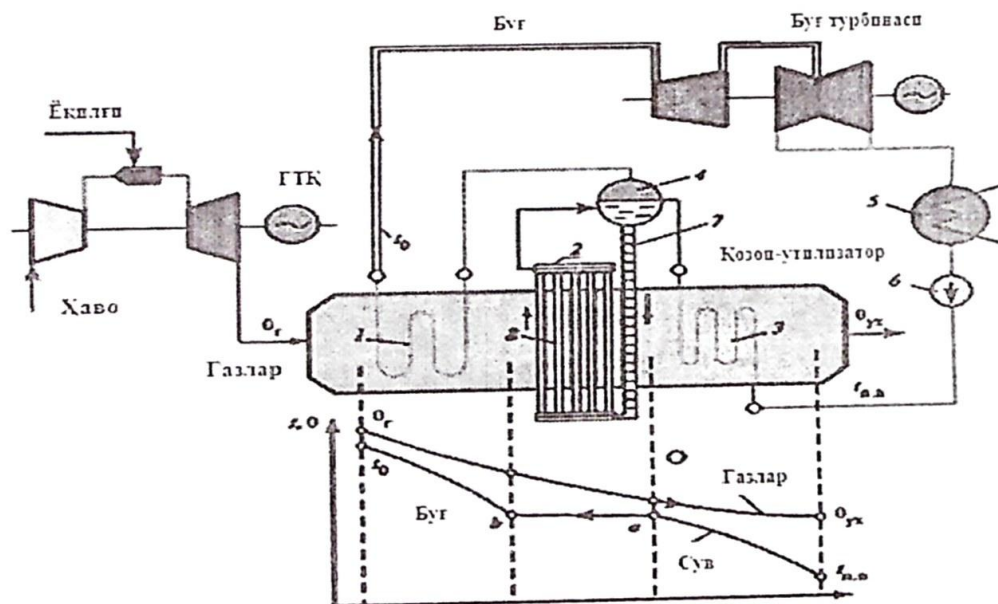
9-расм. Утилизацион русумли БГҚнинг принципиал схемаси
