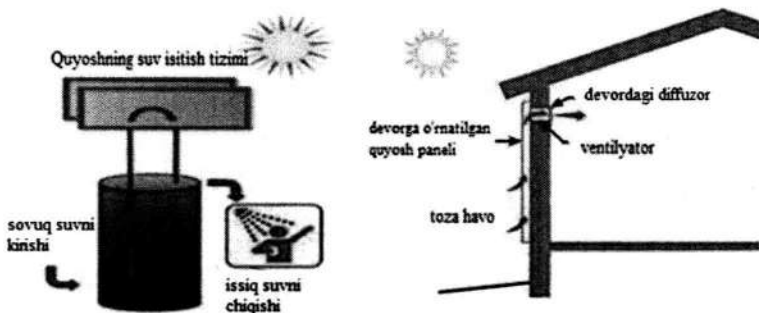
2.15 – rasm. Yassi Quyosh kollektorining ishlash tizimi.
