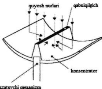
2.20-rasm. Parabolik quyosh elektr stansiyasining ko‘rinishi va ishlash tizimi.
