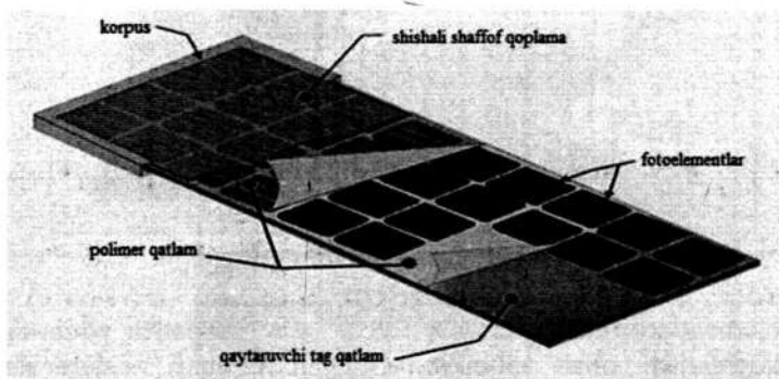
3.12-rasm. Fotovoltaiik panelning tuzilishi.
