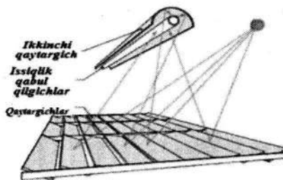
2.21-rasm. Parabolik konsentratorli quyosh elektrostansiyalarini ko‘rinishi.
