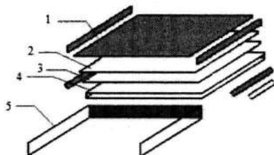
2.17 – rasm. Oynali havo kollektorining tuzilishi:
