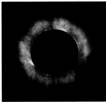
2.4-rasm. 1999-yil Quyosh tutilishidagi quyosh toji.
