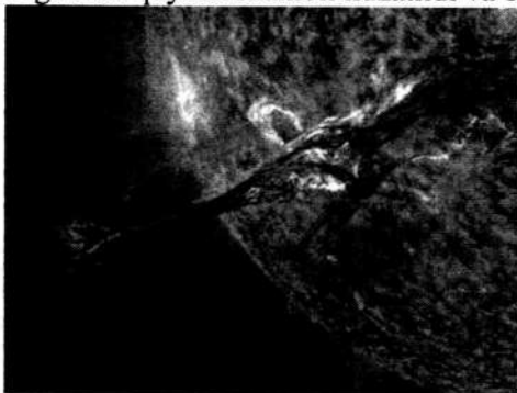
2.7-rasm. Quyosh tojni massadan ajralishi. Plazma nurlarini magnit maydon kamonlari bo'ylab cho'zilgan holati.
