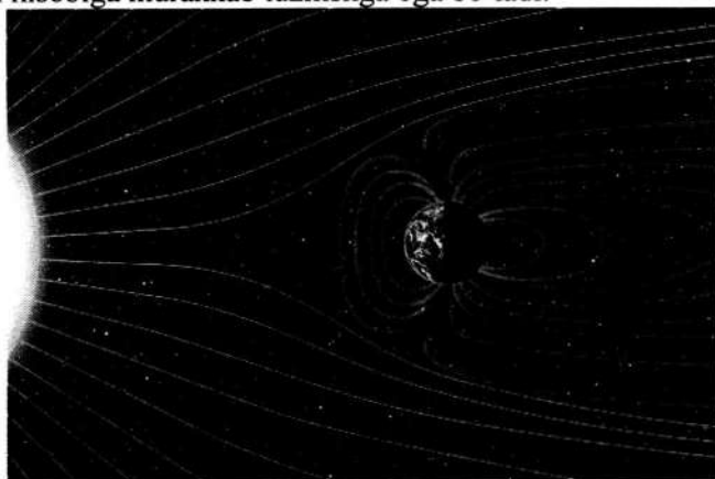
2.6-rasm. Quyosh shamoli ta'sirida Yer magnit maydonining buzilishi.
