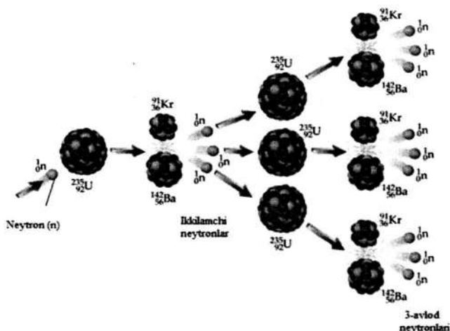
4.2-rasm. Zanjir reaksiyasi.
