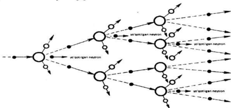
4.4-rasm. Ko'chkisimon zanjirli reaksiyada energiya tez o'sishi portlashga olib keladi.
