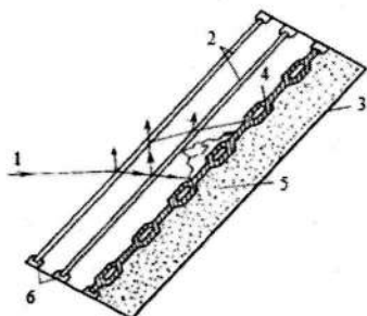
2.18-rasm. Yassi quyosh kollektori:
