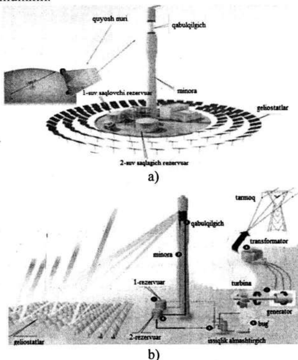
3.14-rasm. Quyosh elektr stansiyasining ishlash tamoyili.
