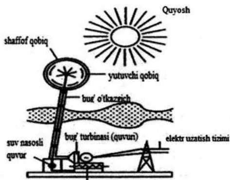
2.11-rasm. Quyosh aerostatik elektrostansiyasining tuzilishi [6].
