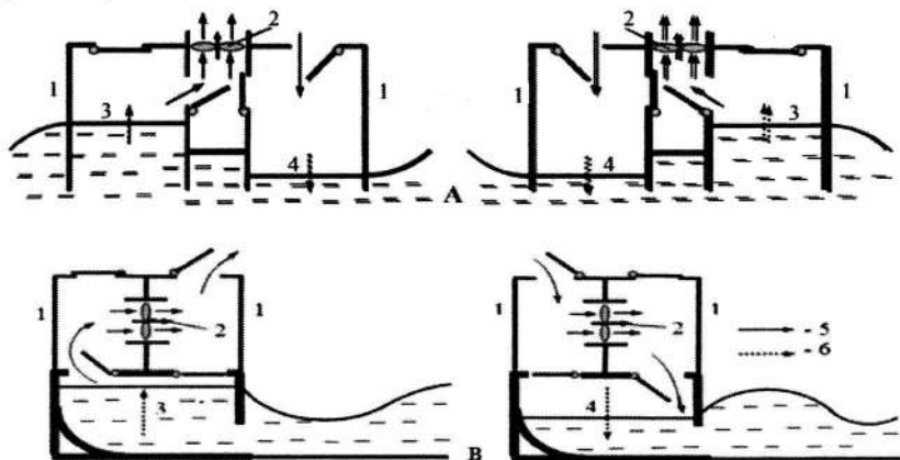
7.11-rasm. Tebranuvchi to'liqin ustunlari asosida ishlaydigan qurilmalar:
