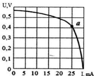
3.5-rasm. FEning volt-ampferli tavsifi.
