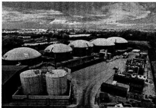
6.3-rasm. AQShning Bioenergy Devco kompaniyasi tomonidan qurilgan anaerob bioreaktorlari (AQSh, Merilend).
