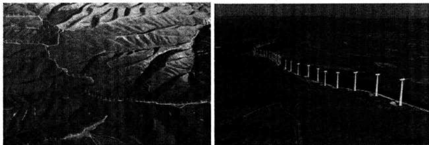
5.4-rasm. Ispaniyada yer sirtida joylashgan shamol elektrostansiyasi.
