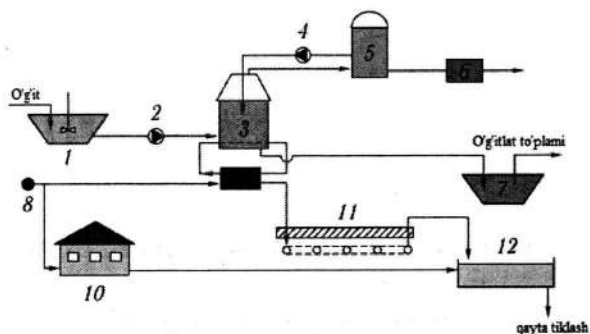
6.2-rasm. Termal suvlardan kompleks foydalanish tizimi:
