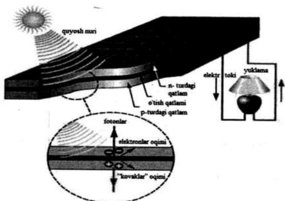
3.9-rasm. Quyosh panelining ishlash mexanizmi.
