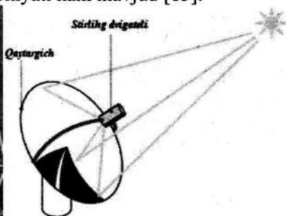
2.24-rasm. Paraboloid quyosh konsentratorlari.
