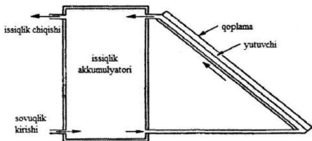
2.14– rasm. Quyosh havo kollektori.
