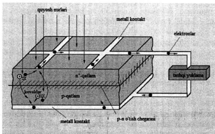
3.4-rasm. Fotoelementni ishlash mexanizmi.
