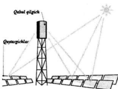
2.23-rasm. Minorali quyosh elektrostansiyalarining tuzilishi.
