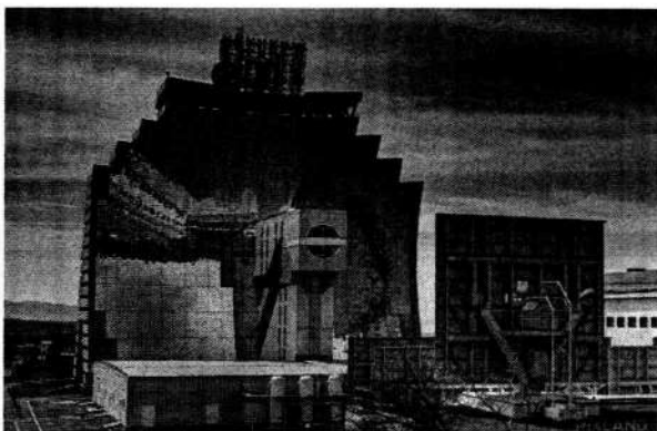
2.25- rasm. O'zbekiston Parkent tumani quyosh pechining umumiy ko'rinishi.
