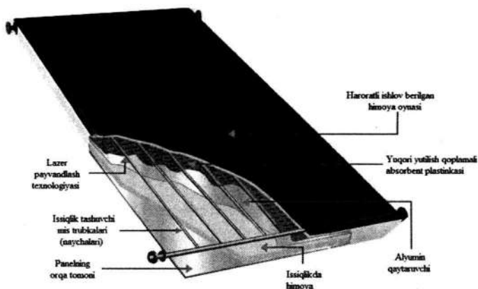
2.16 – rasm. Yassi Quyosh kollektorning umumiy ko‘rinishi va tuzilishi.
