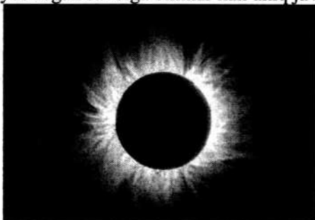
2.3-rasm. Quyosh toji
