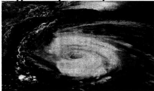
1.1-rasm. Issiqxona effektining koinotdan ko'rinishi.
