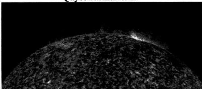
2.8-rasm. Quyoshning Hinode sun'iy yo'ldoshidagi optik teleskop (SOT) yordamida olingan Quyosh sirti va toji. 2007-yil 12-yanvarda olingan [1].
