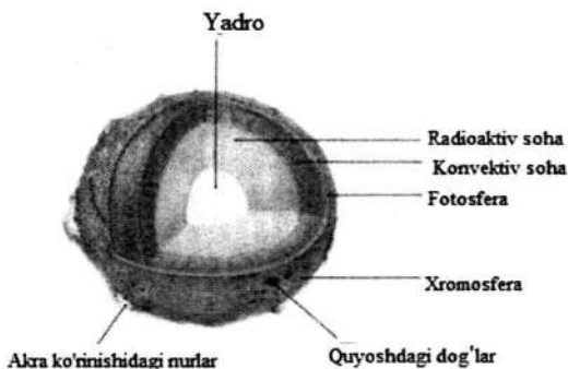
2.1-rasm. Quyoshning tuzilishi.
