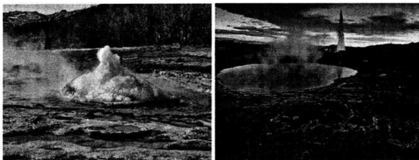
7.3-rasm. Islandiyadagi geyzerlar.
