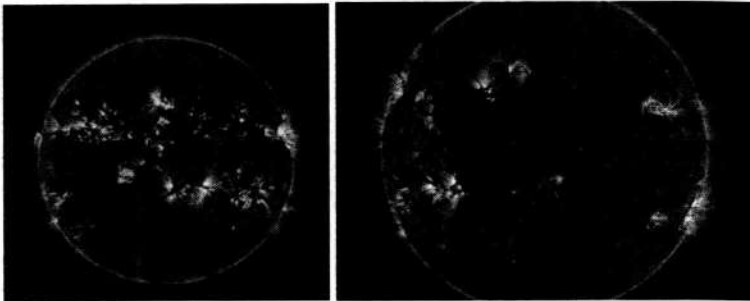
2.5-rasm. 2013-yil 9-aprel NASA / SDO tomonidan tasvirga olingan Quyoshning ko'rinishi.
