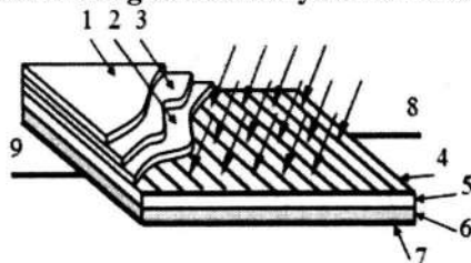
3.7-rasm. Oddiy fotoelementning konstruksiyasi:
