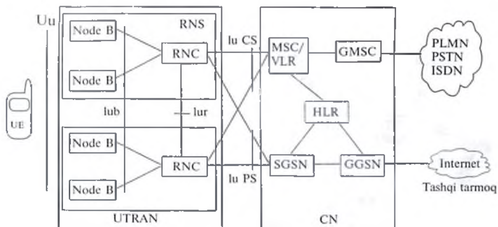
4.4-rasm. UMTS tizimlarining arxitekturası.
