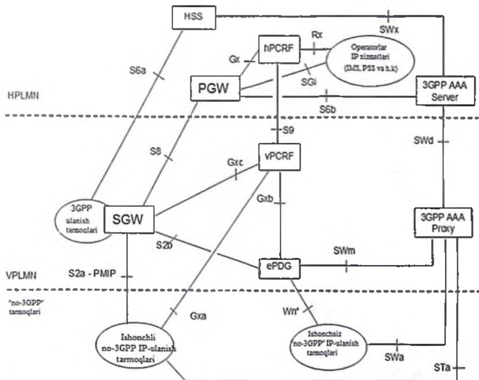
5.4-rasm. "Routing" jarayonida LTE tarmoqlarining "no-3GPP" tarmoqlari bilan PMIPv6 protokoli asosida o'zaro hamkorligi.
