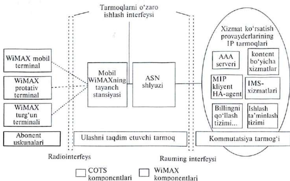
28.6-rasm. IP asosidagi WiMAXWiMAX tarmog'i arxitekturasini.
