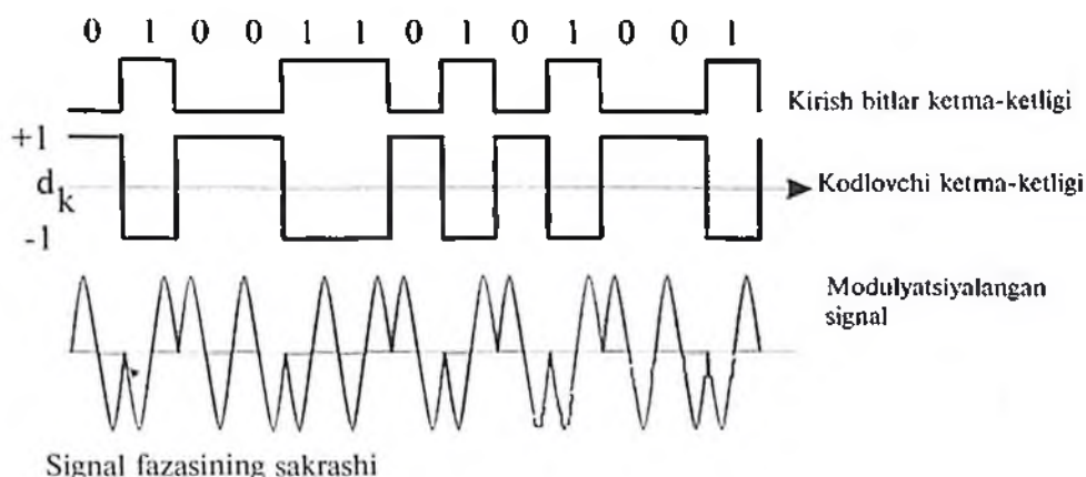
6.1-rasm. BFM (BPSK)ning ikkilik faza modulyatsiyasi.
