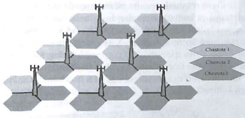
33.2-rasm. WiMAX tarmog‘ining sektorli arxitekturası.
