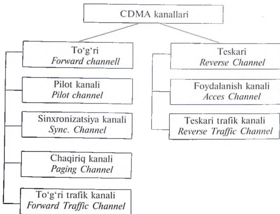
12.7-rasm. CDMA IS-95 standartidagi aloqa kanalining tuzilishi.
