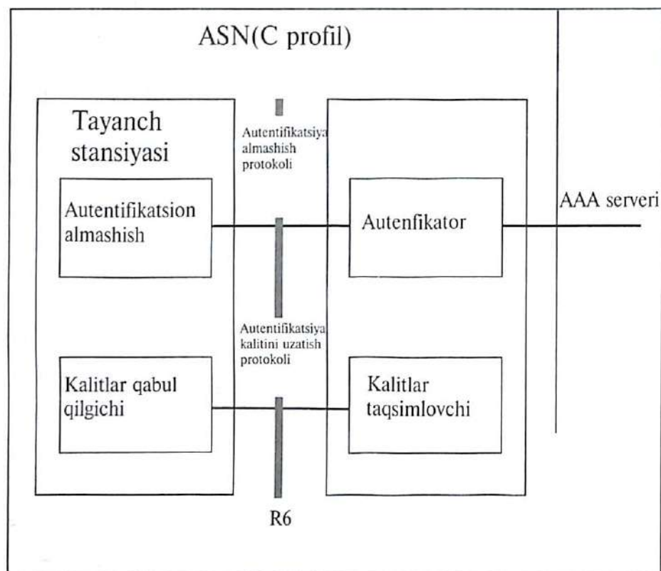
36.7-rasm. S profili uchun ASN tarmog'i xavfsizligi arxitekturasini.
