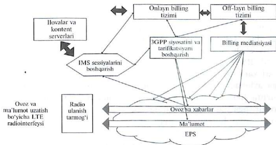
18.3-rasm. LTE tarmog'ida RSS funksiyasining 3-faza bosqichidagi ishlash sxemasi.
