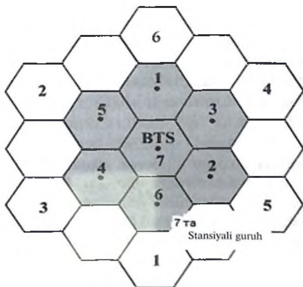
8.2-rasm. Chegaradosh qo'shni stansiyalar guruhi.
