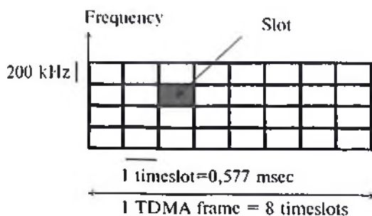
5.1-rasm. GSMga ko’p qirrali kirish (dostup).
