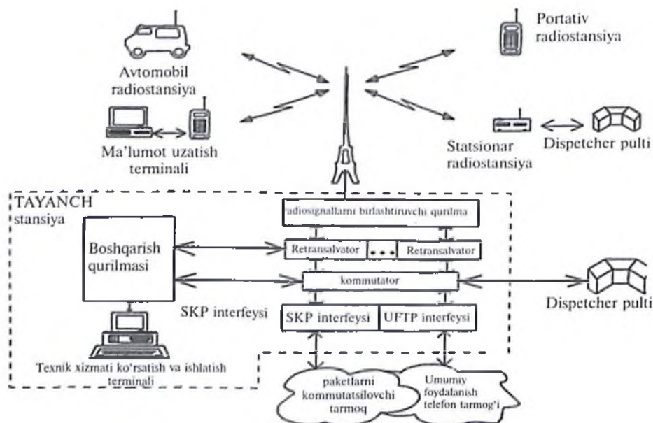
10.1-rasm. Bir zonali tranking tizimining umumlashtirilgan strukturaviy sxemasi.
