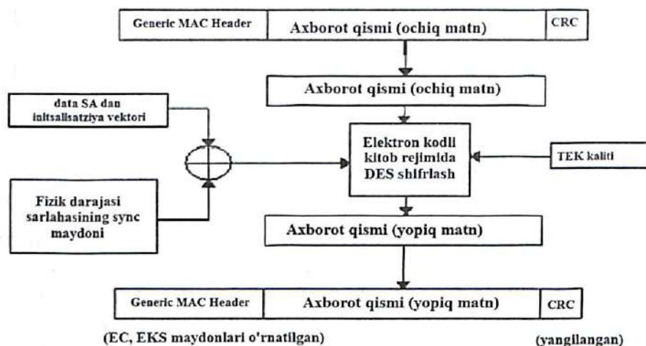
35.2-rasm. DESda ma'lumotlarni shifrlash jarayoni.
