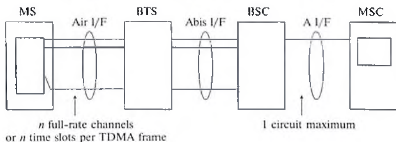
1.5-rasm. HSCSD tizimli arxetekturasi.
