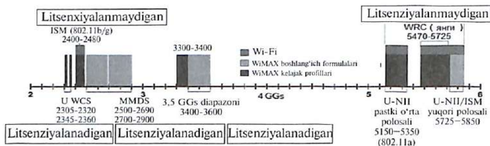
34.1-rasm. 2GGsdan 6 GGsgacha diapazonda KSU tizimlari uchun ruxsat etiladigan chastotalar polosi.
