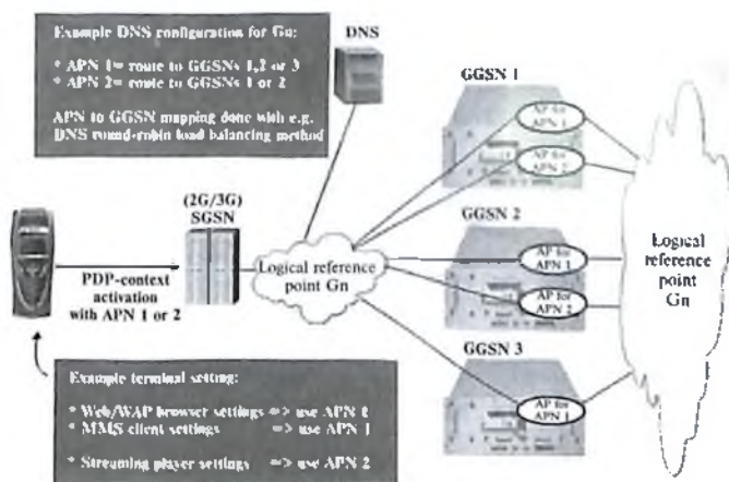
3.6- rasm. APNni DNSga bog’liqligi.
