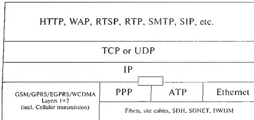
3.4-rasm. IP asosida ko'p sathli protokoli.
