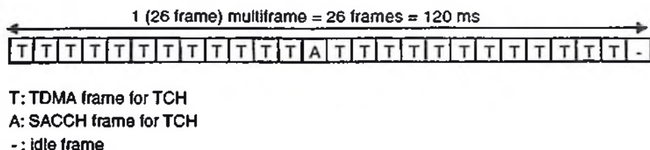
5.2-rasm. TKP boshqaruv kanalini hosil qilish.
