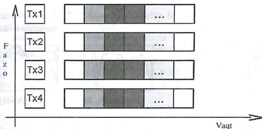
19.4-rasm. V-BLAST asosidagi fazoviy multiplekslash.
