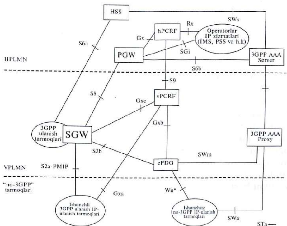
17.2-rasm. “Rouming” jarayonida LTE tarmoqlarining “no-3GPP” tarmoqlari bilan PMIPv6 protokoli asosida o‘zaro hamkorligi.
