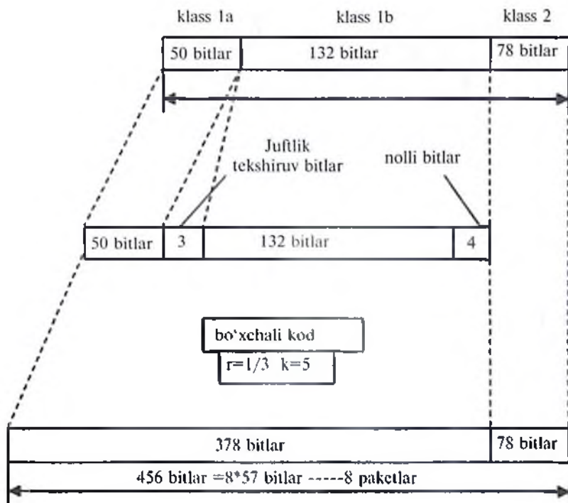
7.5-rasm. So'zlashuv kanalida kodlashtirishning umumlashtirilgan sxemasi.
