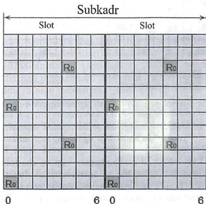
20.2-rasm. Standart SR uchun “pastga” yoʻnalishdagi signalning tuzilmasi.
