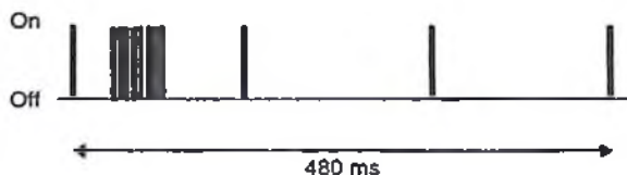
5.7-rasm. SACCH multifreymenti DTX rejimida quvvat o'zgarishi. Sinov jarayonida Samsung GT B3710 hamda Huawei E398 rusumli modemlardan foydalanildi.
