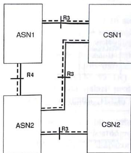
28.5-rasm. WiMAX tayanch tarmog'i tugunlarining o'zaro ta'sirlashishi.
