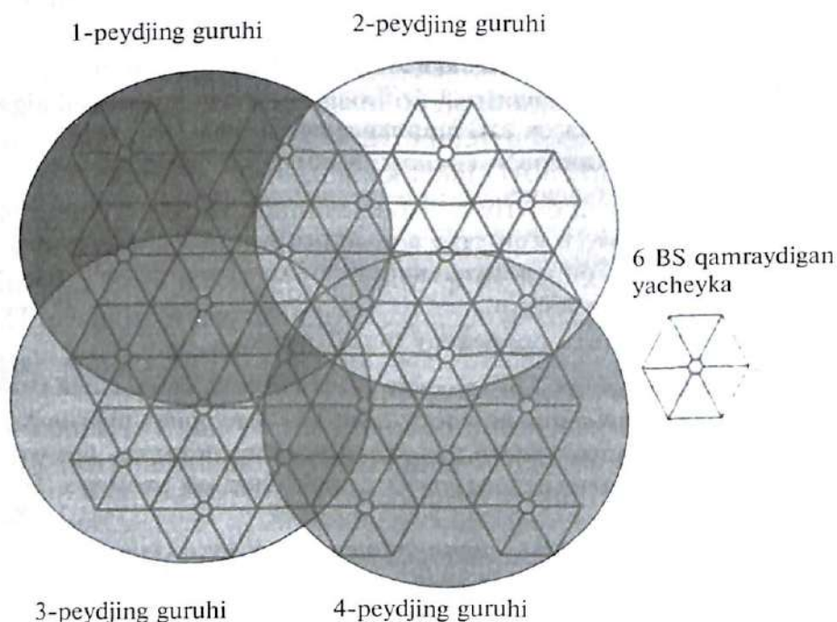
31.2-rasm. BSni peydjing guruhlariga bo'linishi.
