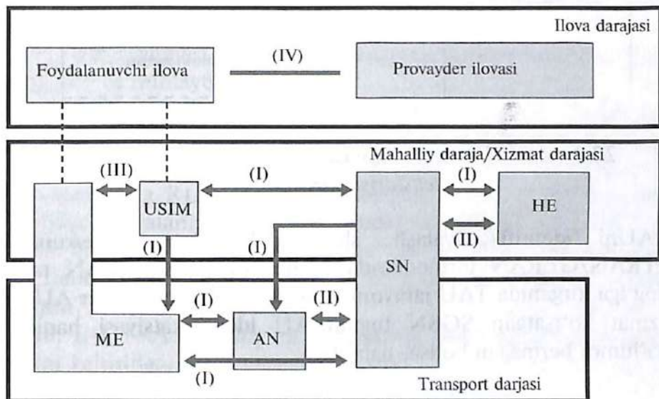
23.2-rasm. LTE/SAE tarmog'ida axborot xavfsizligining tashkil etilishi.
