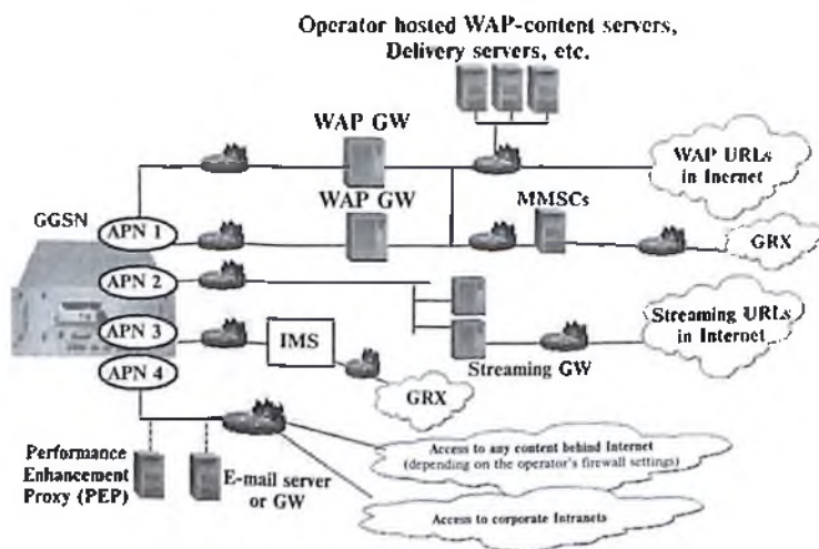
3.7-rasm. APNni proksiserverga bog'liqligi.
