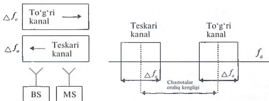
9.4-rasm. Chastotalarni dupleksli tarqoqlash prinsipida tashkillashtirish.
