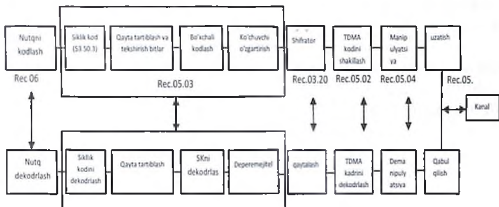
7.4-rasm. Radiotraktning tuzilish sxemasi.
