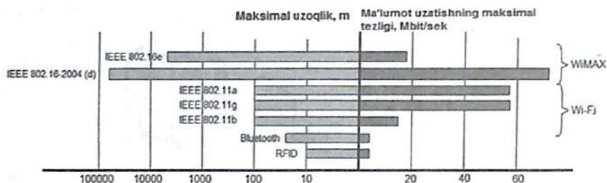
24.3-rasm. Ma'lumotlarni uzatish tezligi va aloqaning uzoqligi bo'yicha simsiz texnologiyalarning sinflarga bo'linishi.
