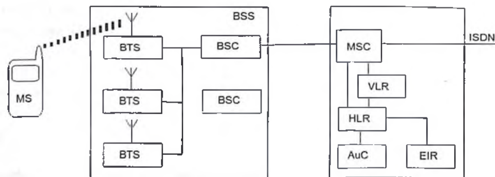
4.2-rasm. GSM tarmog'ining tuzilish sxemasi.
