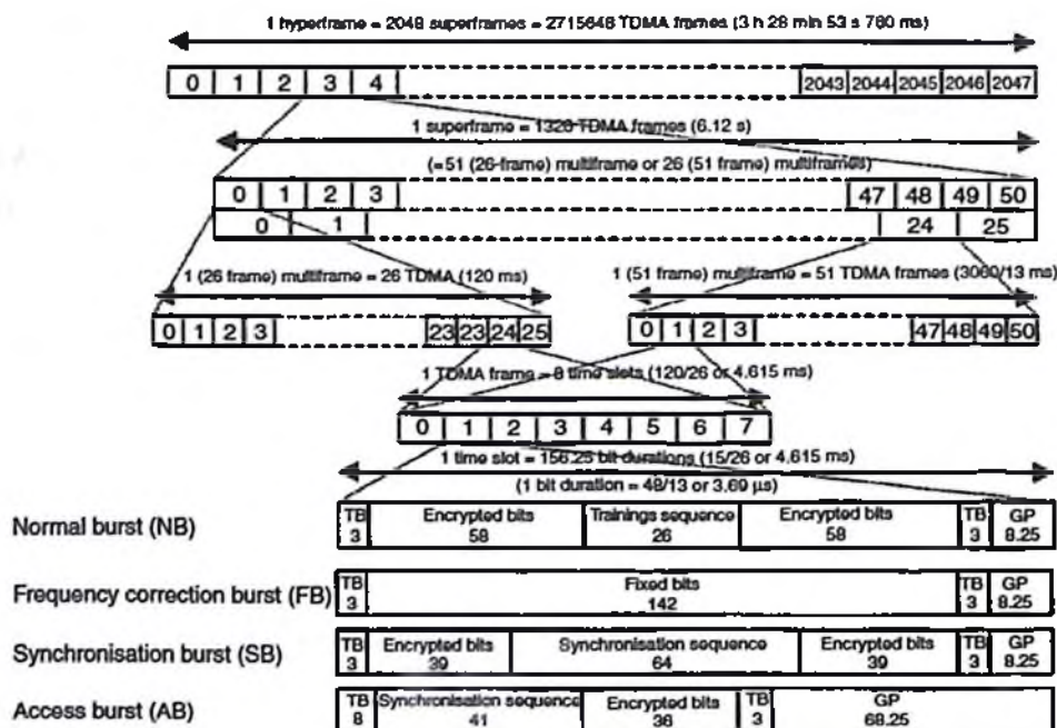
5.3-rasm. GSM vaqt intervali.
