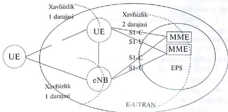
23.1-rasm. LTE tarmog'ida xavfsizlik darajalari.
