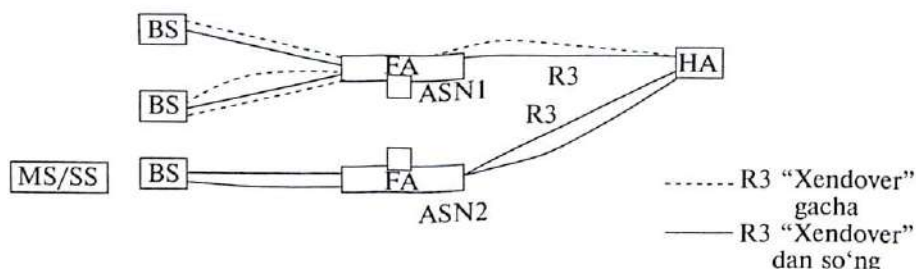
31.5-rasm. Mobillikni boshqarish turlarining aralash o'zaro ta'sirlashishi.
