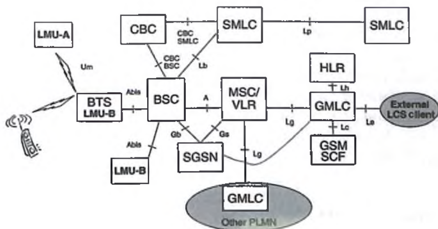
4.6-rasm. PBS arxitektura LVP.
