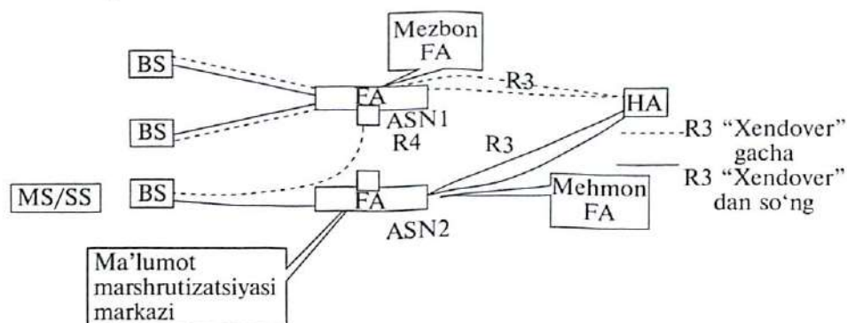
31.4-rasm. Mobillikni boshqarish turlarining ketma-ket o'zaro ta'sirlashishi.
