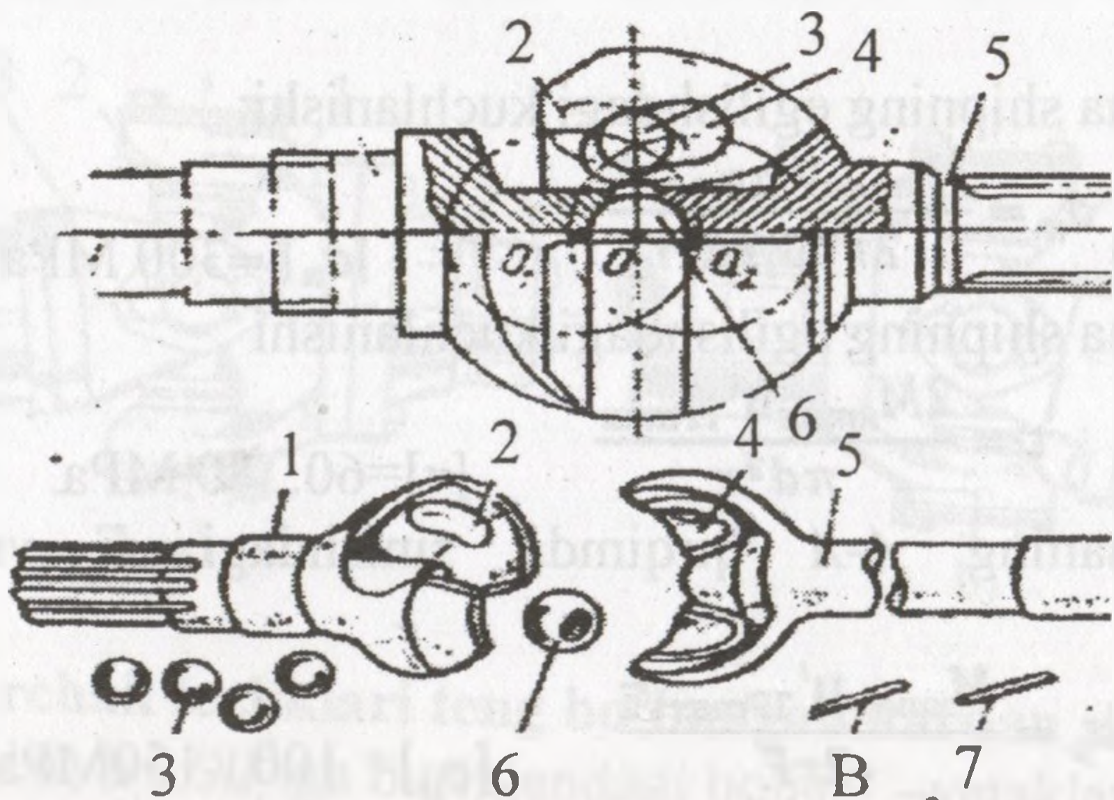
7.4-rasm. Burchak tezliklari teng bo‘lgan kardan sharniri:
