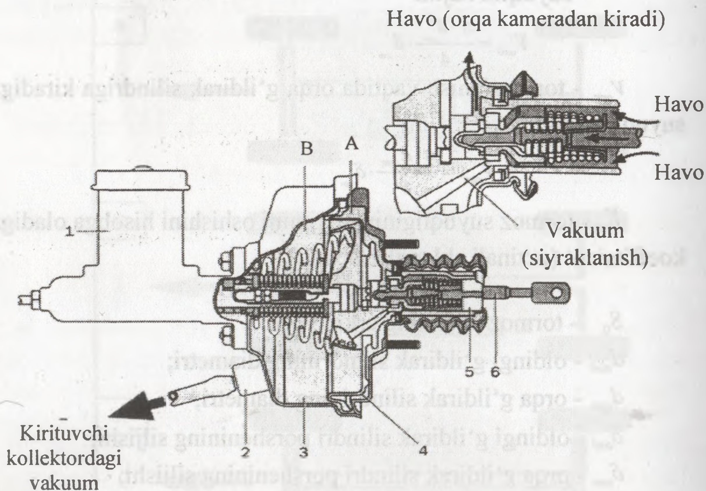
12.12-rasm. Vakuum kuchaytirgichlarning sxemasi va ishlashi: A -atmosferali hajm; B - vakuumli hajm; 1 -asosiy tormoz silindri hajmi; 2 -to'suvchi klapan; 3 -vakuum kamerasi; 4 -diafragma; 5 -havo filtri; 6 -tormoz pedalining shtoki.
