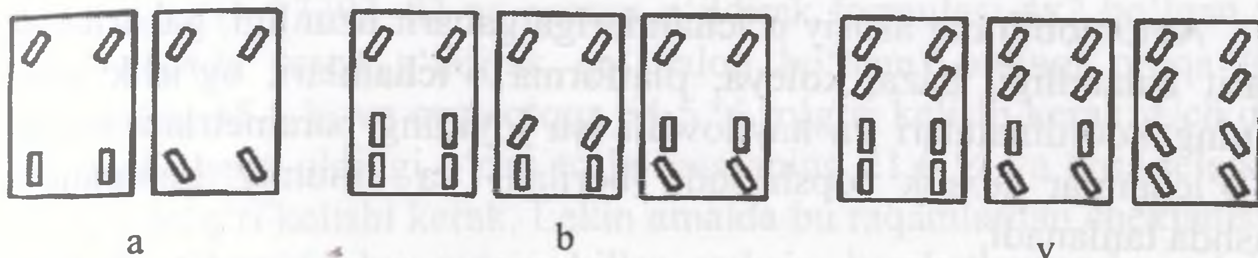
3.10 – rasm. Yuk avtomobillarda yetaklovchi va boshqariluvchi o‘qlarning joylashuvi: a – ikki o‘qli; b - uch o‘qli; v - to‘rt o‘qli;
