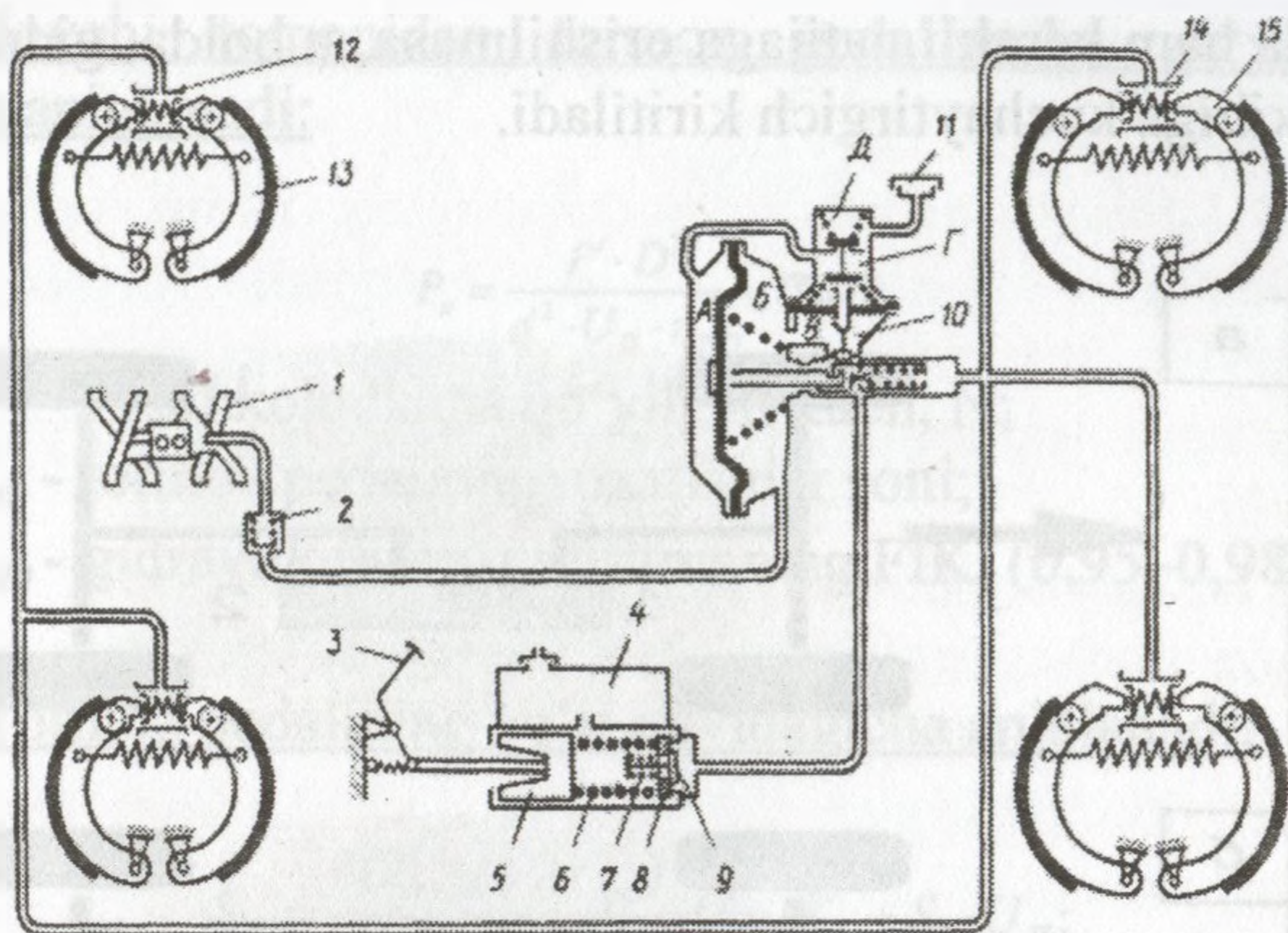
12.10-rasm. Gidravlik yuritmalı ishchi tormoz tizimi:
