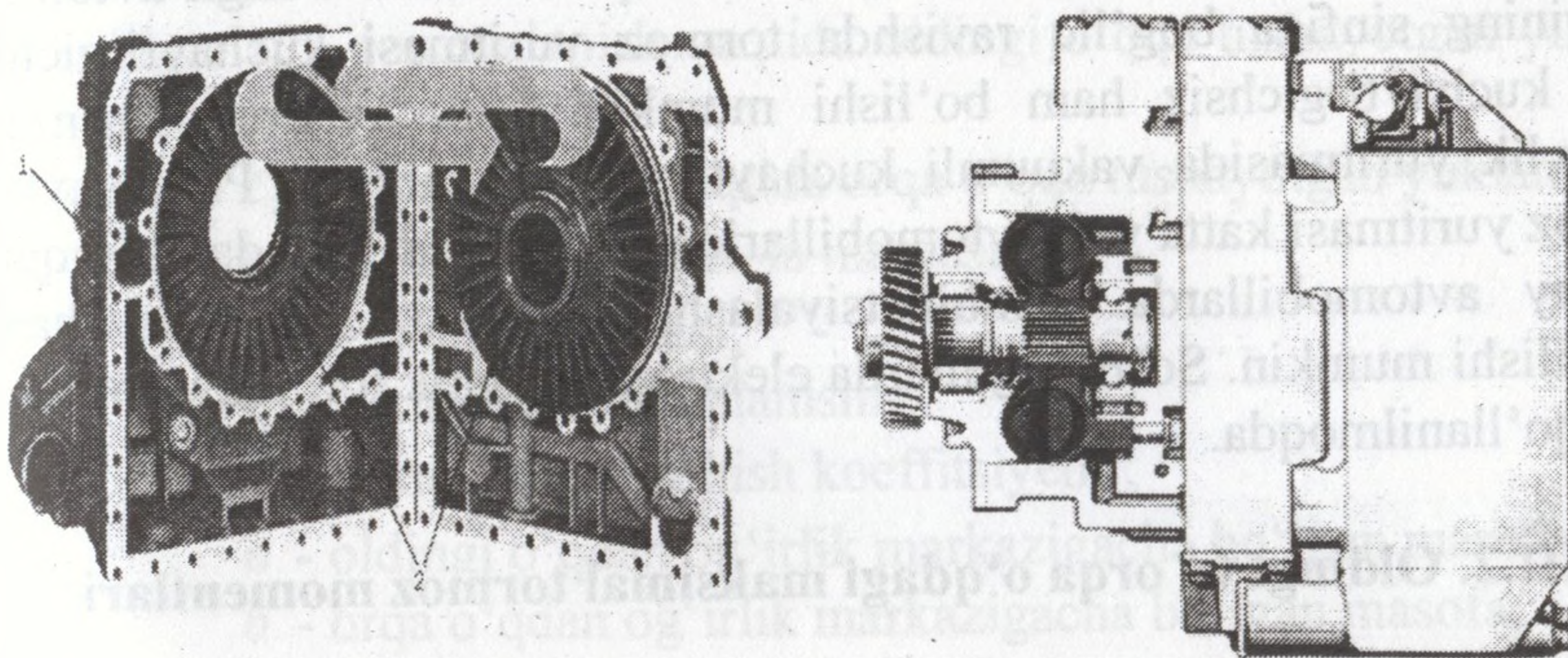
12.3-rasm. Yordamchi tormoz tizimlari (Gidravlik tormoz-sekinlatgich)
