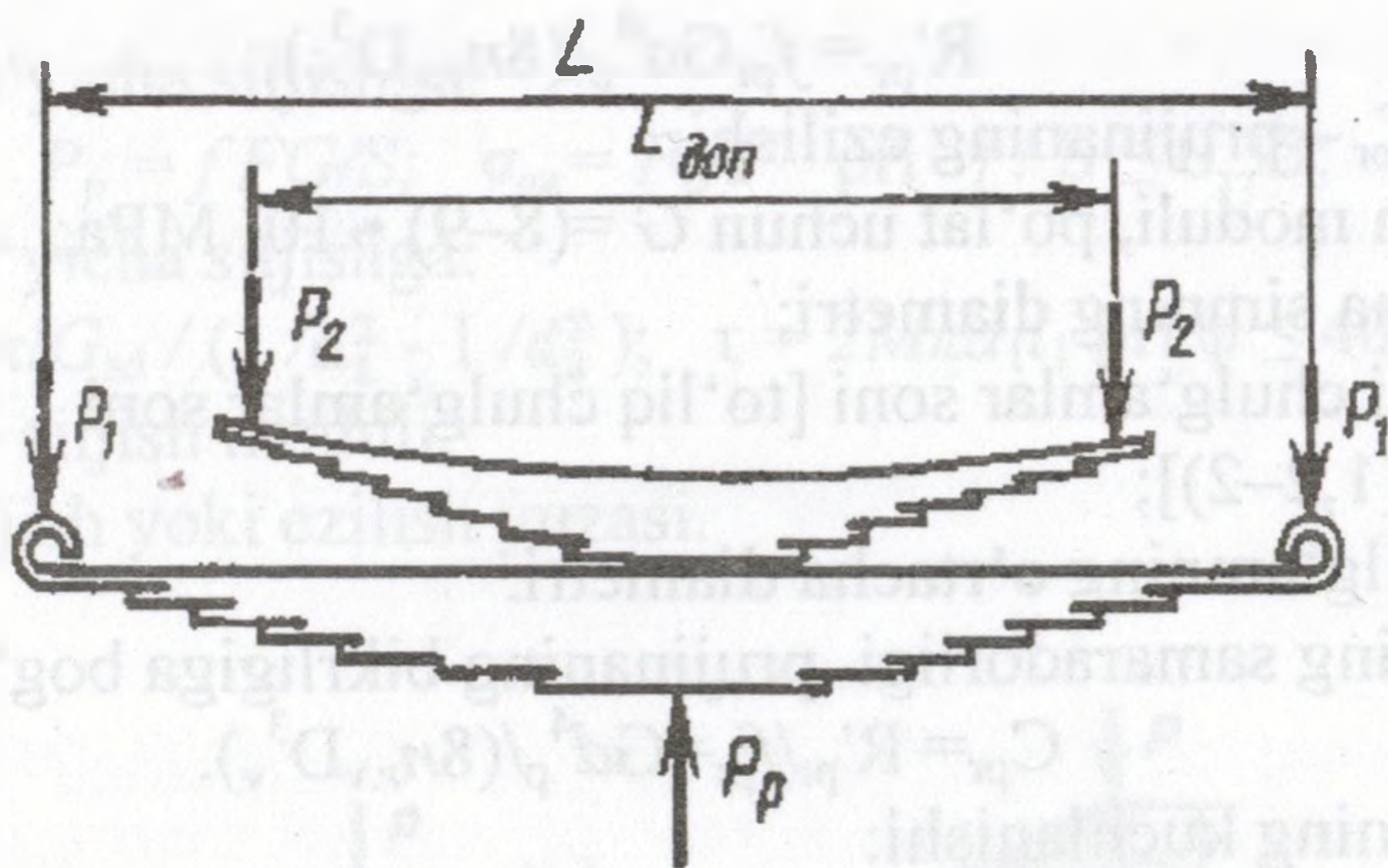
10.2- rasm. Qo'shaloq resorani hisoblash sxemasi
