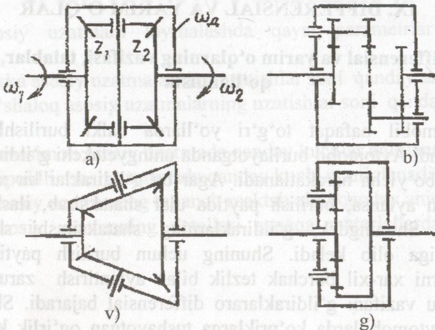
9.1-rasm. Yetaklovchi vallardagi burovchi momentlari o'zgarma nisbatli differensiallar sxemalari: a, b) – simmetrik; v, g) - nosimmetrik.
