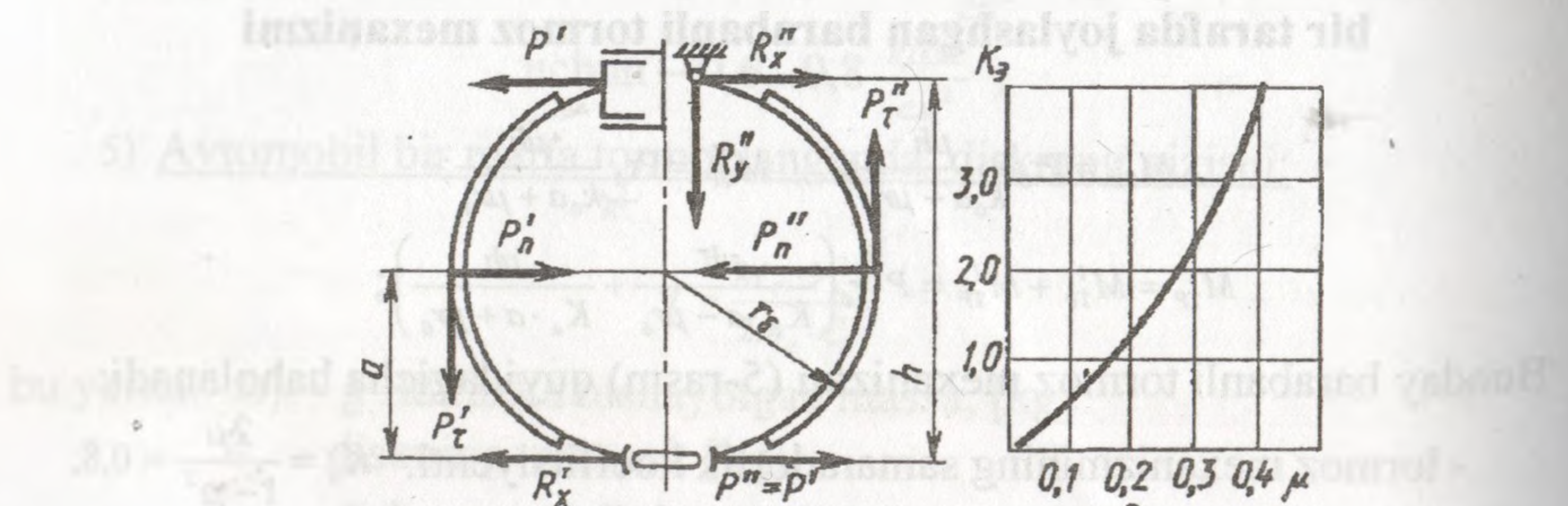
12.7-rasm. O'z-o'zidan kuchaytiruvchi tormoz mexanizmi
