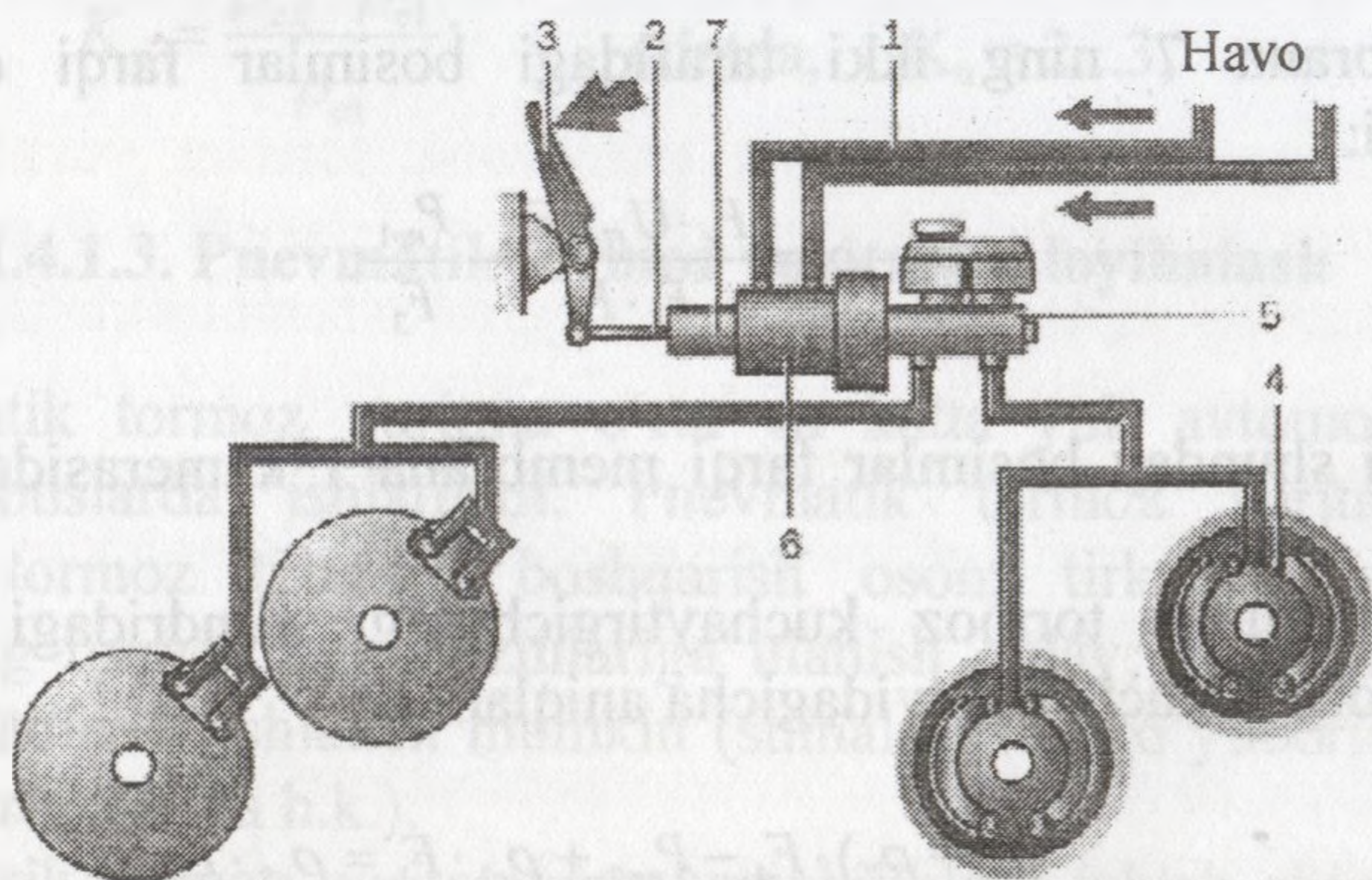
12.14-rasm. Pnevmatik kuchaytirgichli gidravlik yuritmaning sxemasi:
