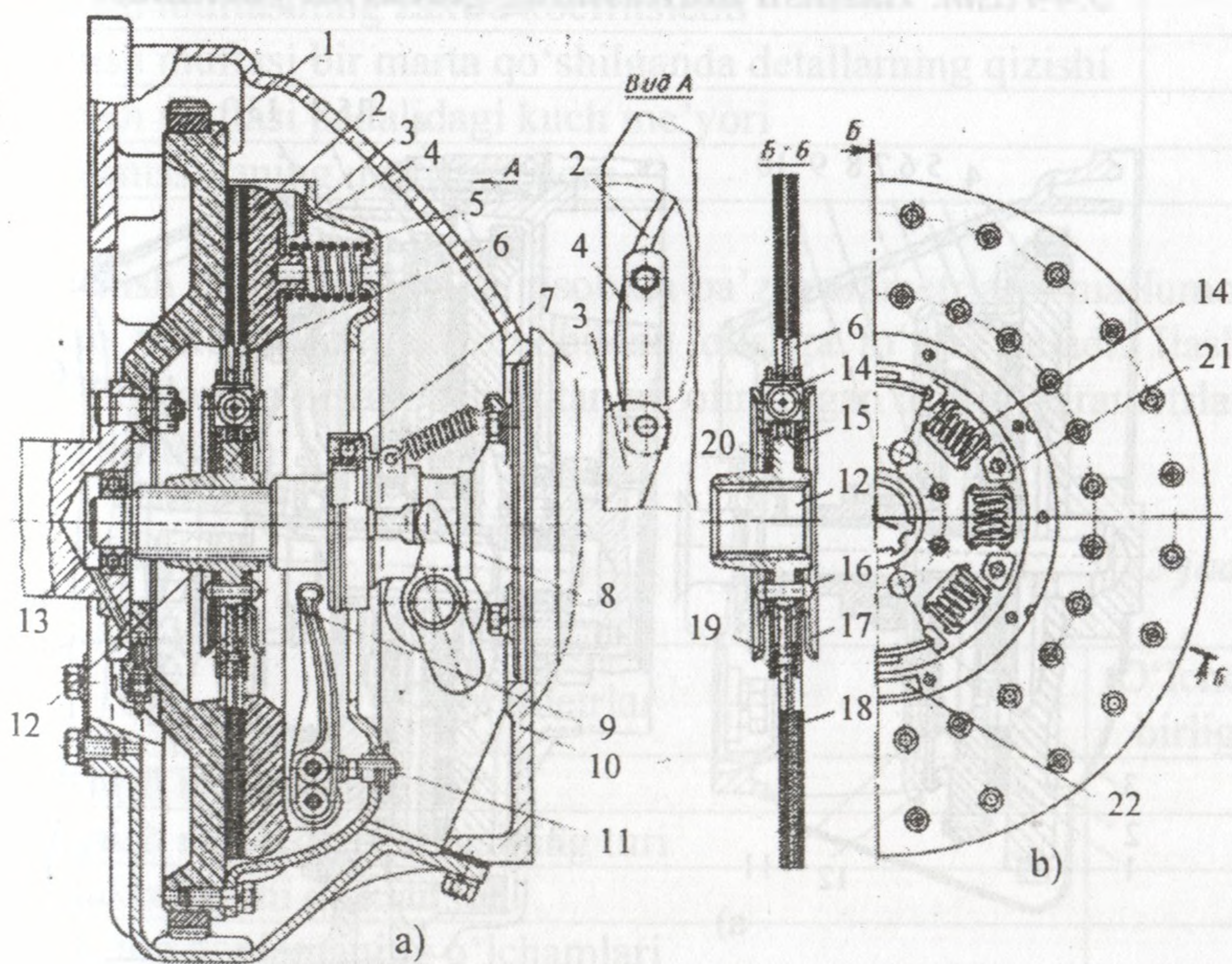
5.3-rasm. Bir diskli friksion ilashish muftasi konstruksiyasi
