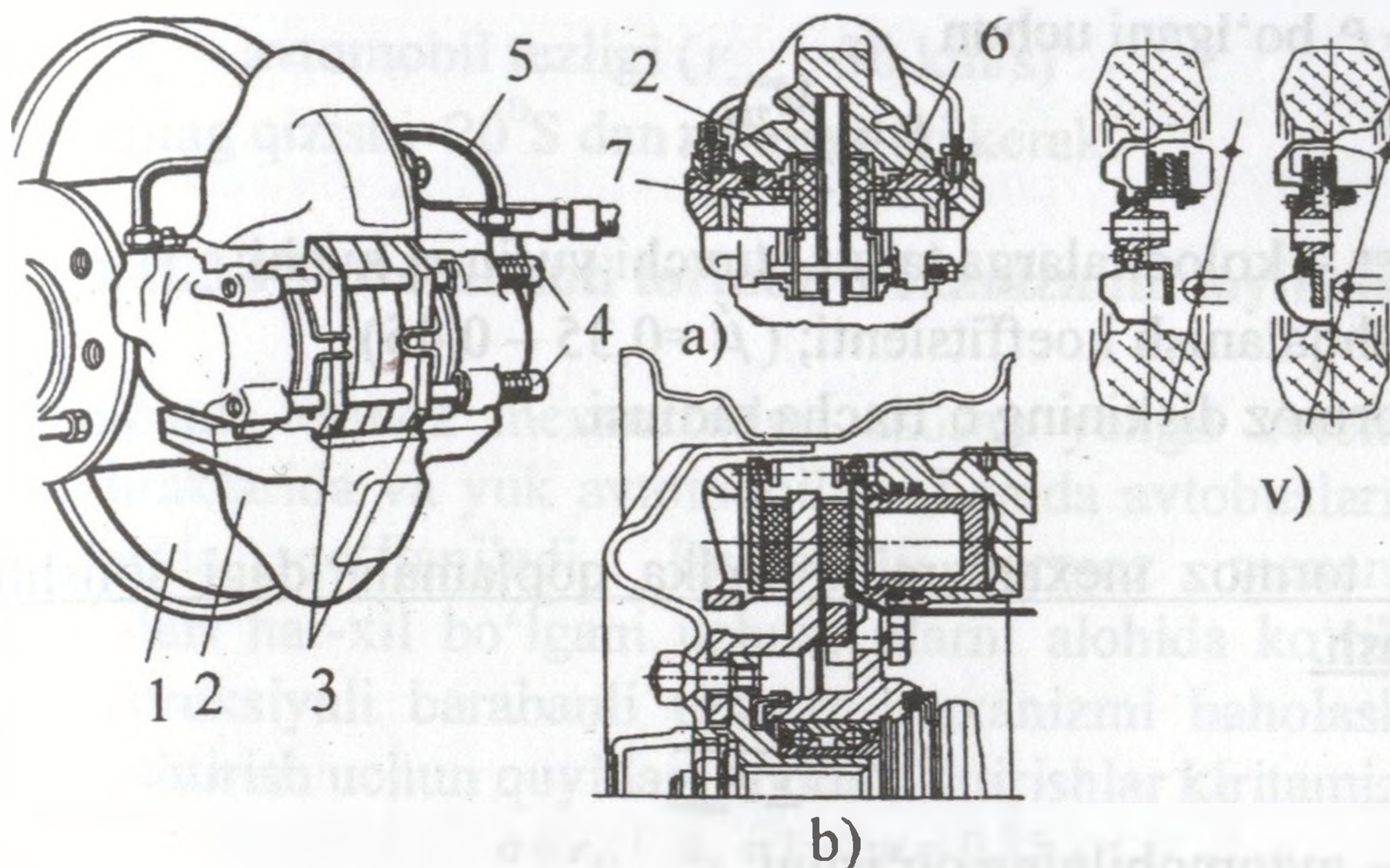
12.4-rasm. Diskli tormoz mexanizmining konstruksiyasi: a -qo'zg'almas skobali; b - qo'zg'aluvchi skobali; v – skobalarni o'rnatilish sxemalari; 1 – tormoz diski; 2 – skoba; 3 – tormoz kolodkalari; 4 – kolodka barmog'i; 5 – ulanish trubkasi; 6 – rezinali halqa; 7 – porshenlar.
