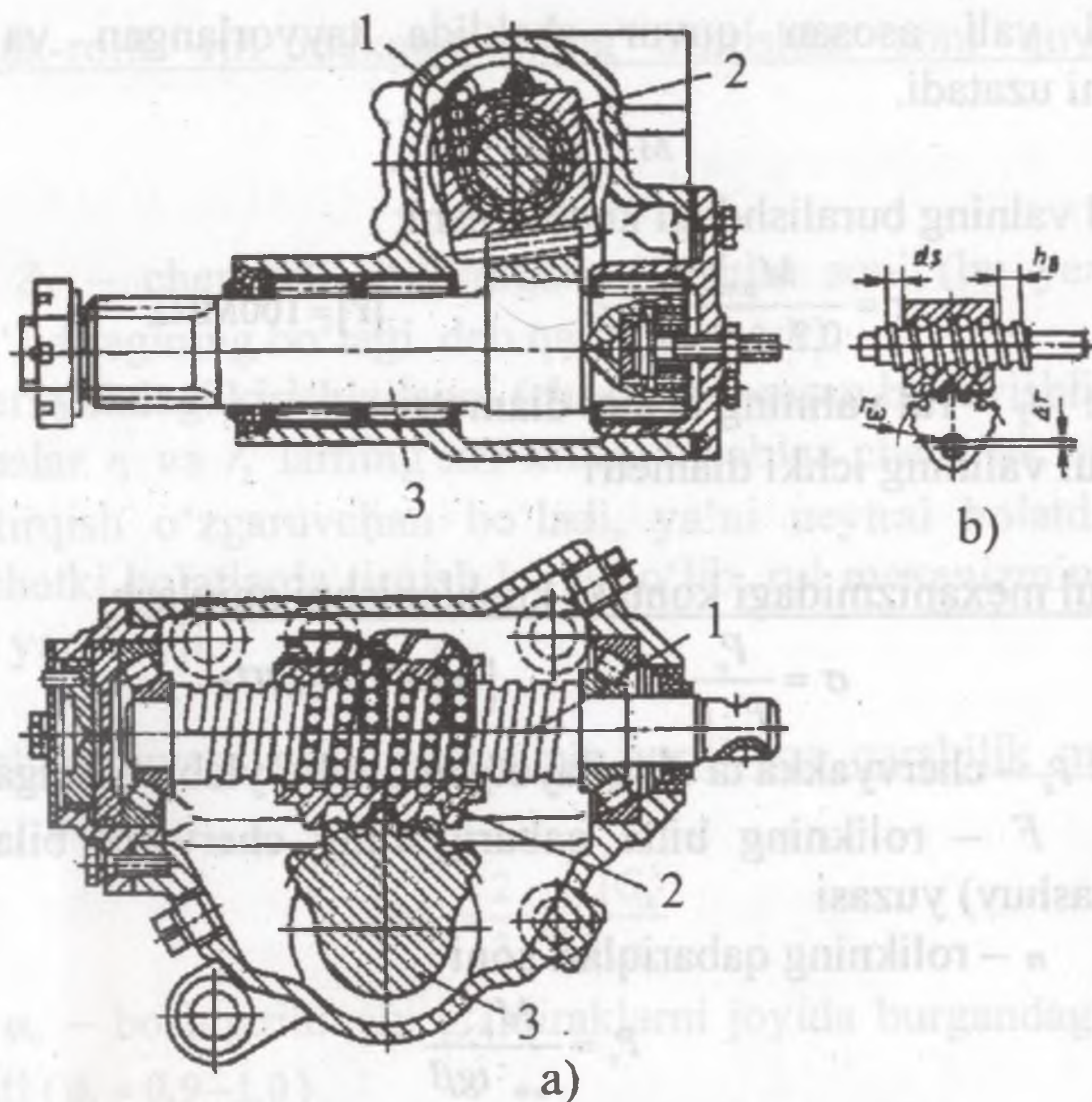
11.4-rasm. Vintli rul mexanizmi konstruksiyasi
