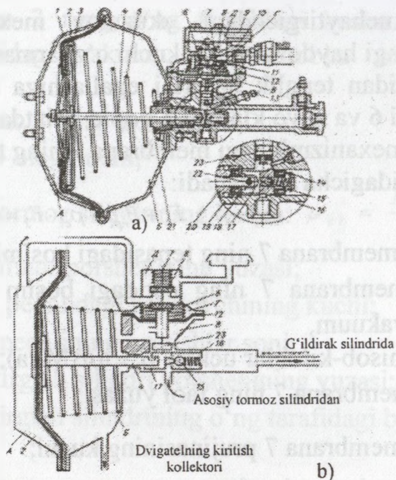
12.13-rasm. Hidrovakuum kuchaytirgichning sxemasi va ishlashi:
