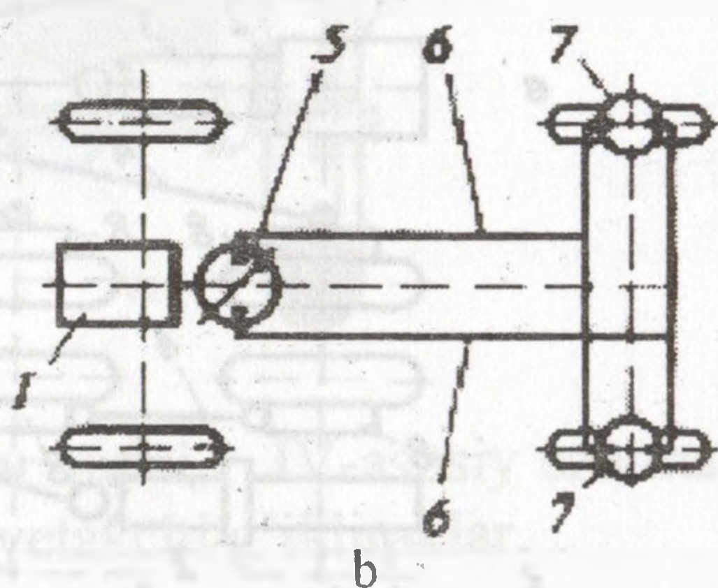
4.5-rasm. Avtomobil transmissiyalari: a – elektrik; b - gidrohajmli; 1 – dvigatel; 2 – generator; 3 – elektr simlari; 4 – elektromotor-g'ildirak; 5 - gidronasos; 6 - trubkalar; 7 – gidromotorlar.
