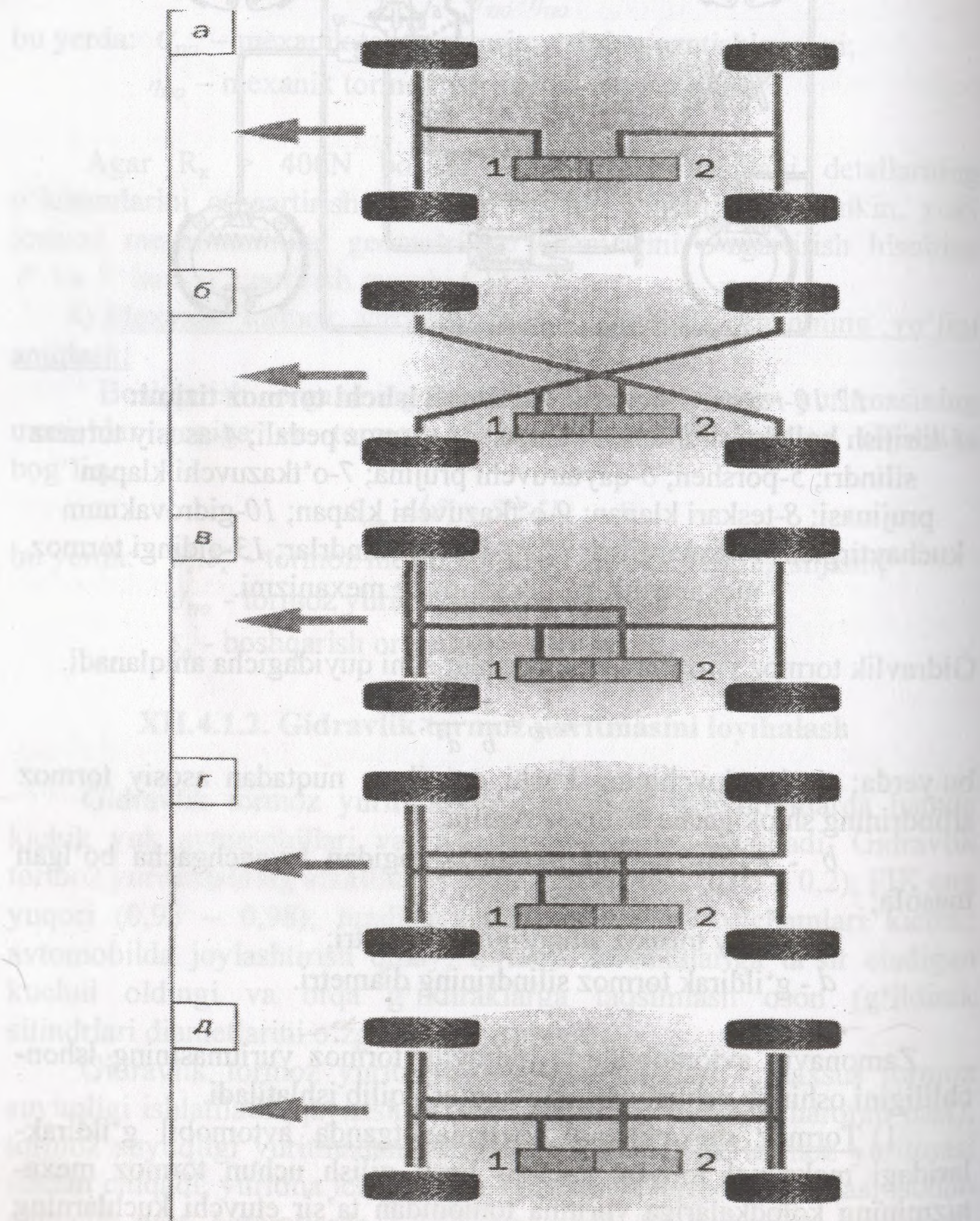
12.11-rasm. Tormoz yuritmasini ikkita mustaqil konturga ajratish usullari
