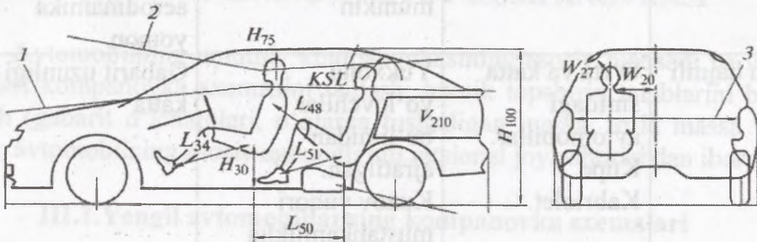
3.3-rasm. Joylashuvdagi qulaylik va haydovchi joyidan ko‘rinuvchanlikni aniqlovchi geometrik parametrlar: 1- ko‘rinuvchanlikning pastki chegarasi; 2- ko‘rinuvchanlikning yuqori chegarasi; 3- kuzovning ichki kengligi.
