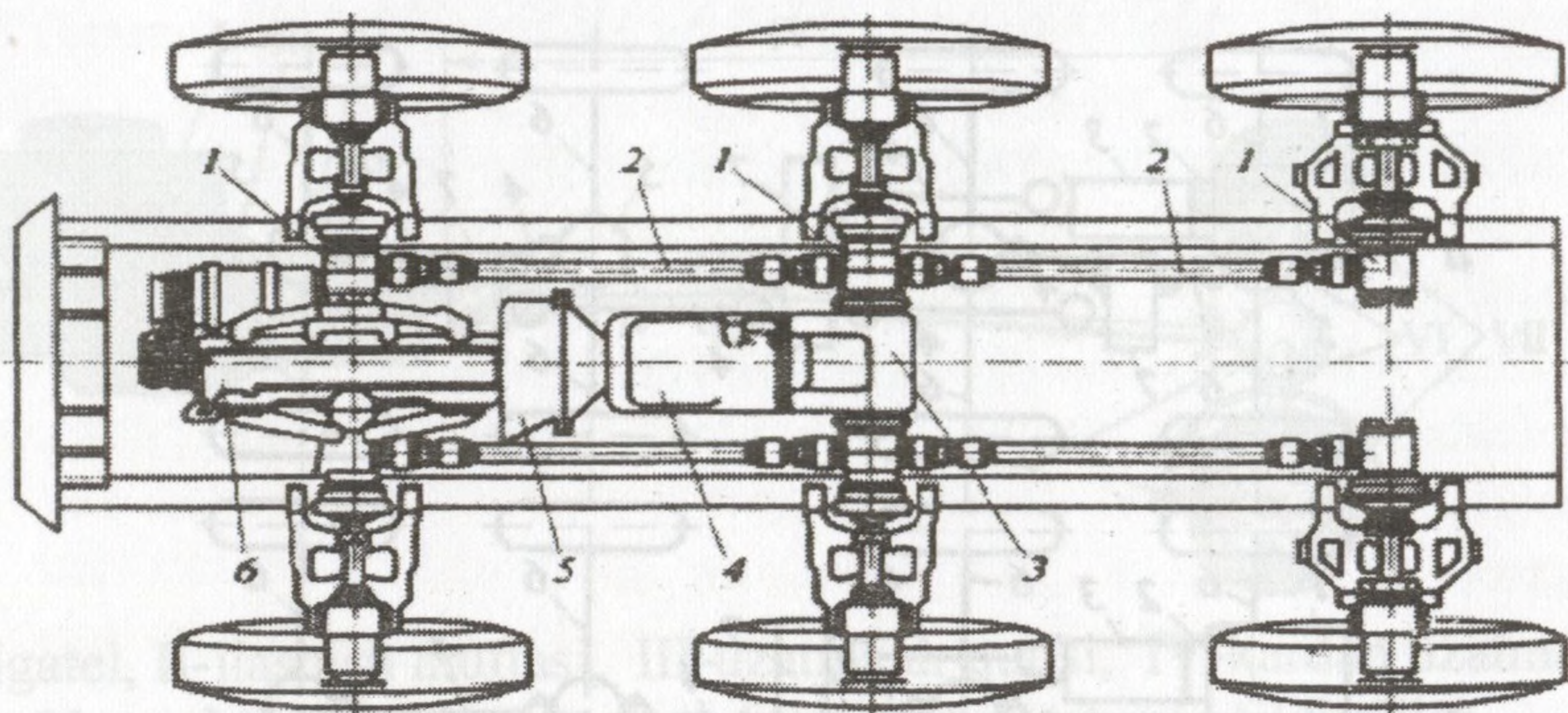
4.4-rasm. Bort uzatmali avtomobil transmissiyasining kompanovkasi:
