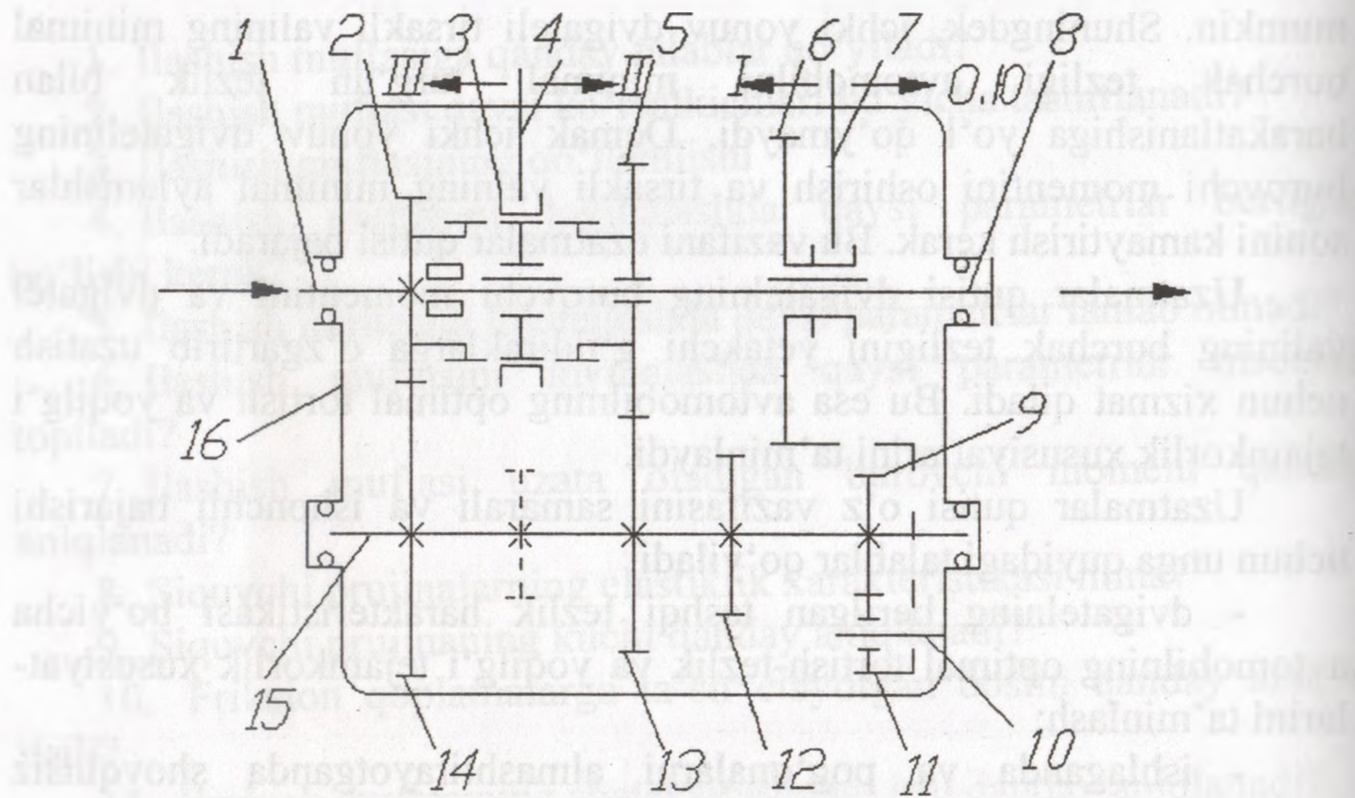
6.1-rasm. Uch pog'onali uzatmalar qutisining sxemasi:
