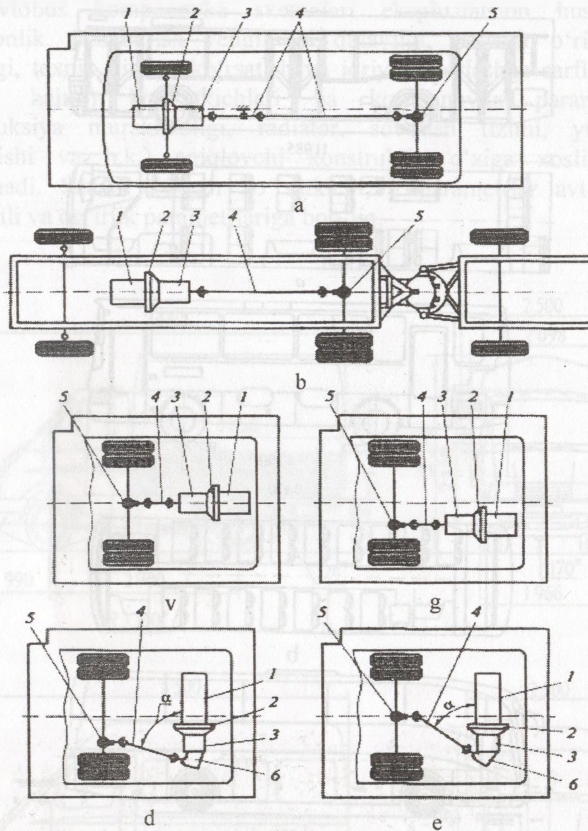
3.9-rasm. Avtobuslarda shassi agregatlarining joylashuvi sxemalari:
