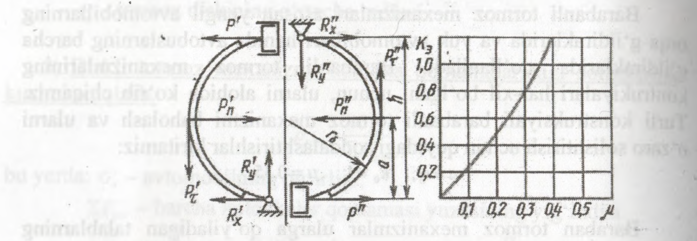
12.6-rasm. Yuritma kuchlari teng va tayanchlari qarama-qarshi bo'lgan tormoz mexanizmi
