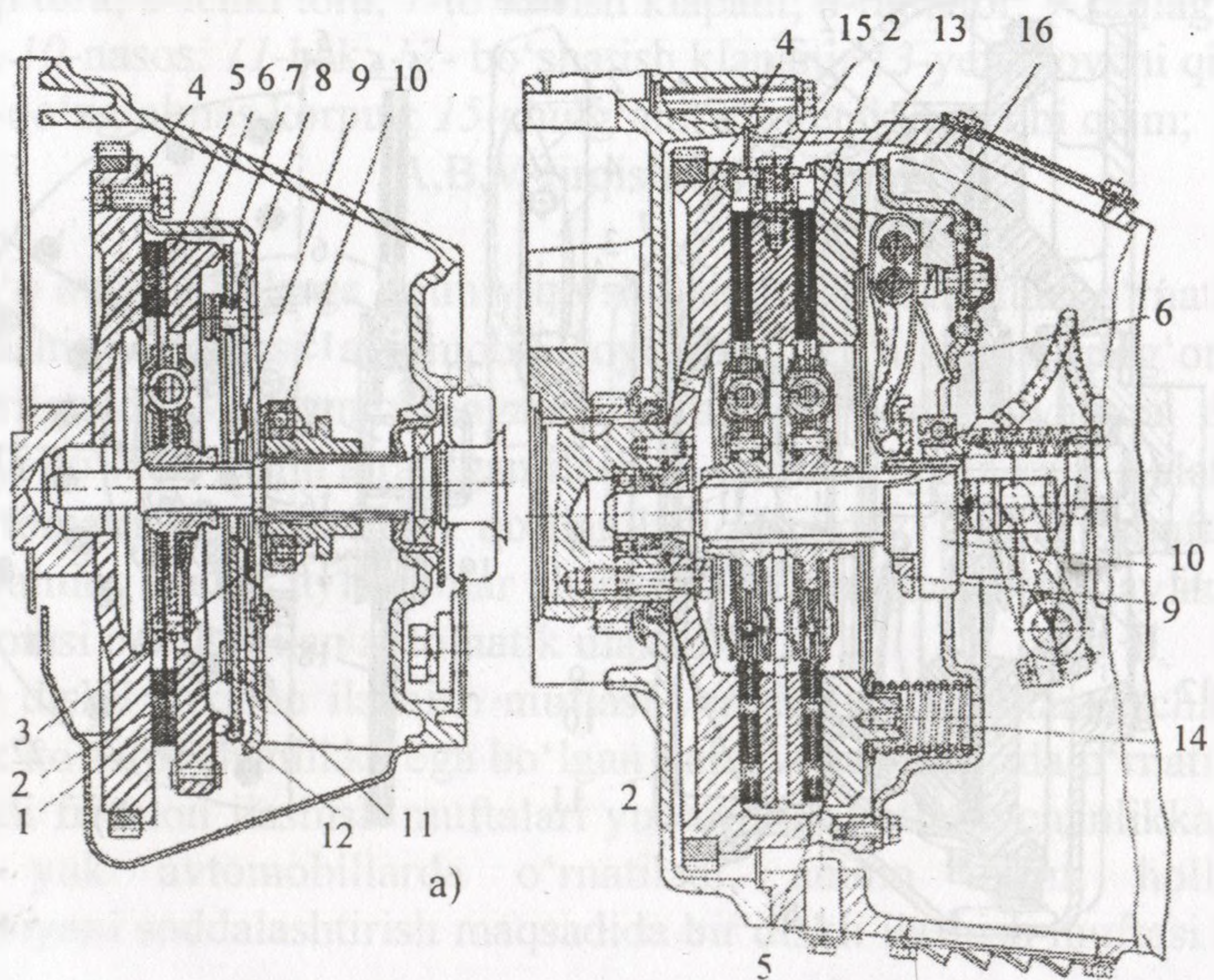
5.5-rasm. Ikki diskli friksion ilashish muftasi konstruksiyasi
