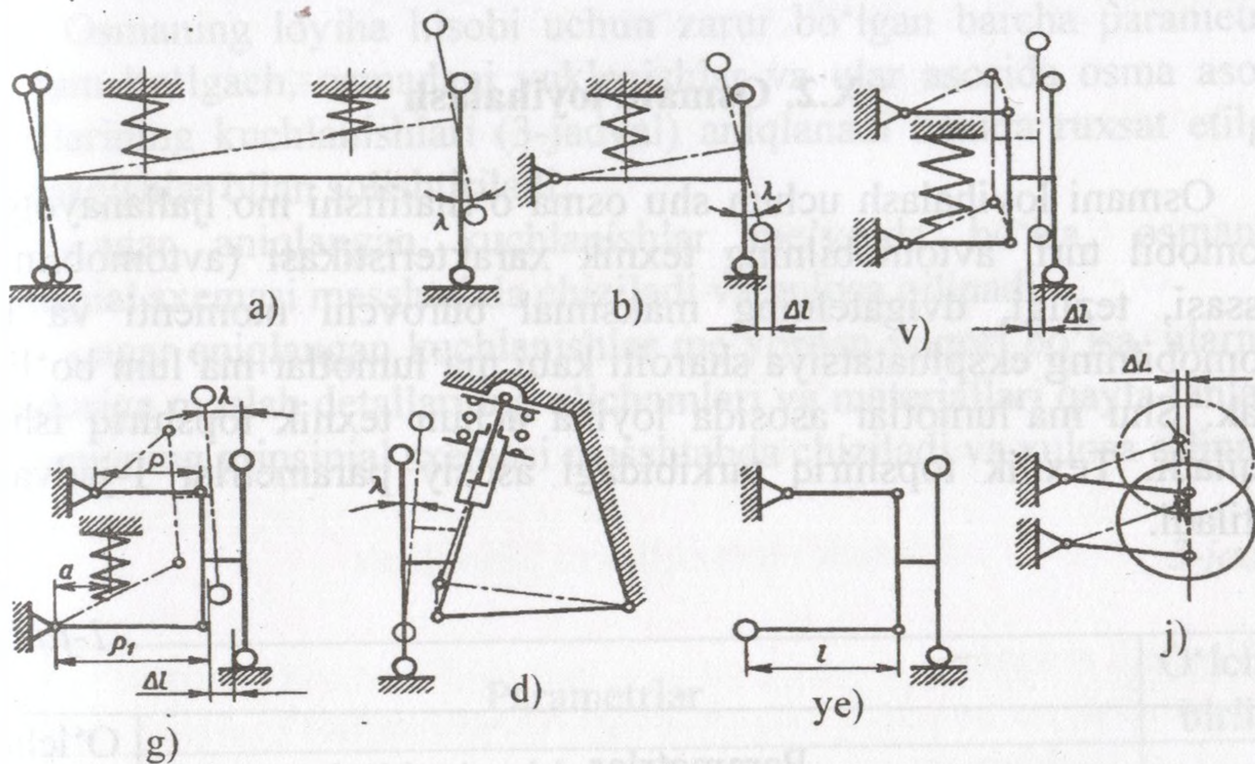
10.1-rasm. Osmaning kinematik sxemalari:
