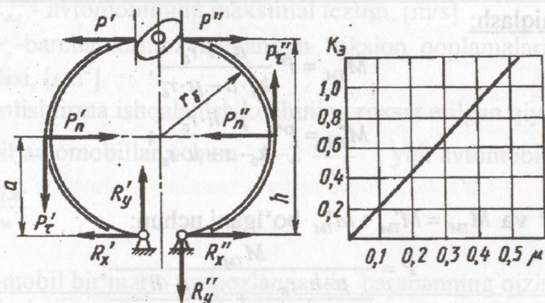
12.8-rasm. Kolodkalarining siljishlari teng bo'lgan tormoz mexanizmi
