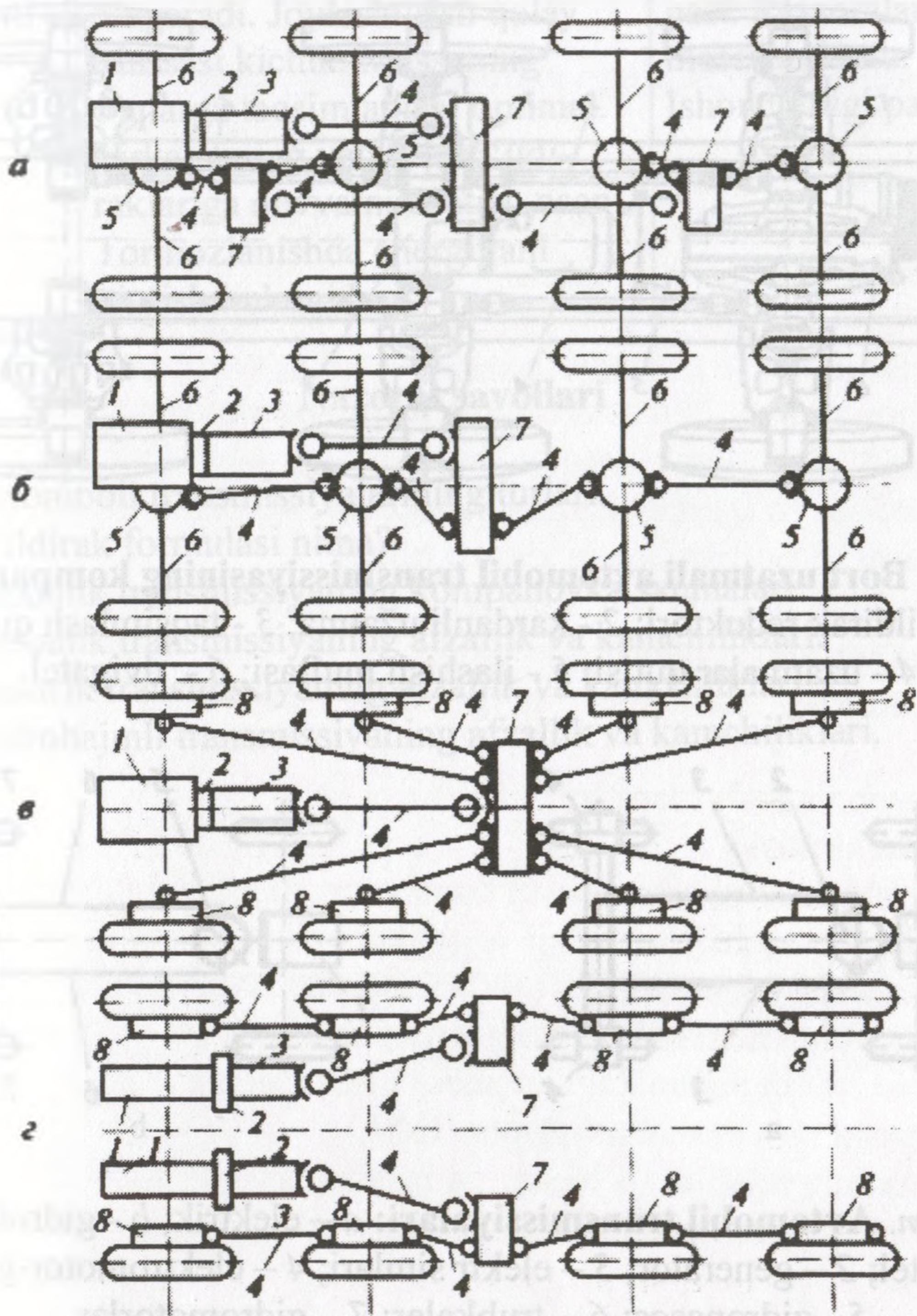
4.3-rasm. O‘tag‘on avtomobil transmissiyalarining sxemalari:
