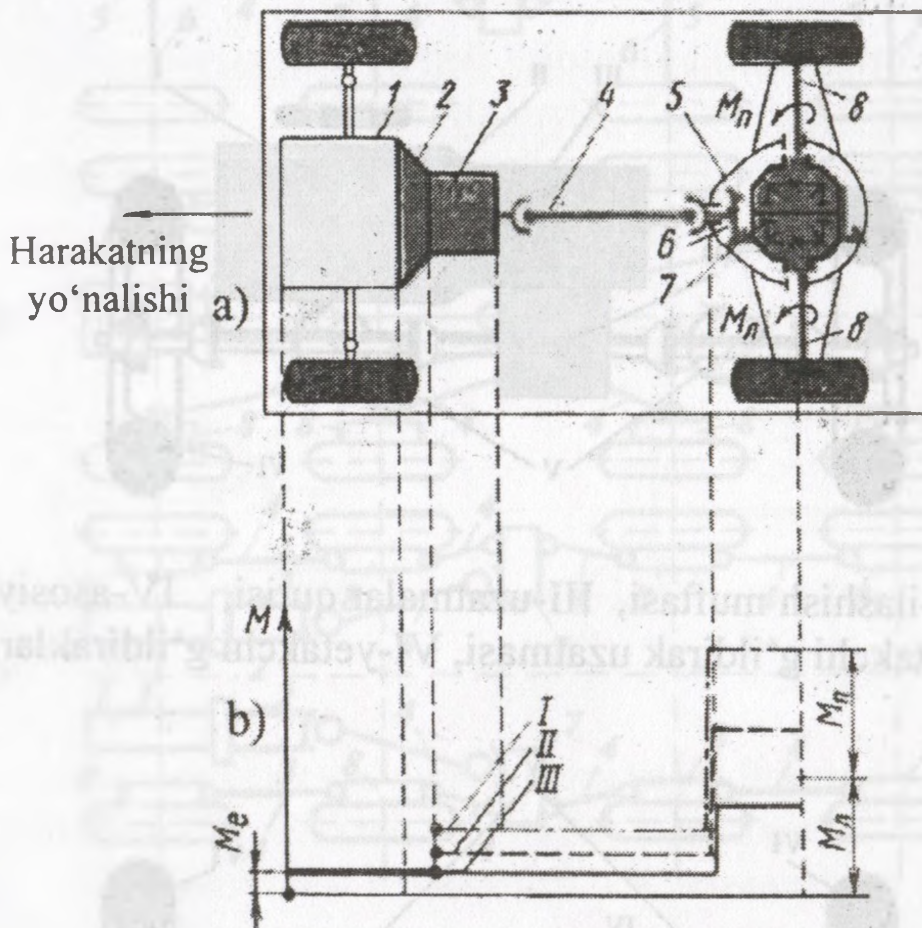
4.1-rasm. Mexanik transmissiyada burovchi momentning uzatilishi:
