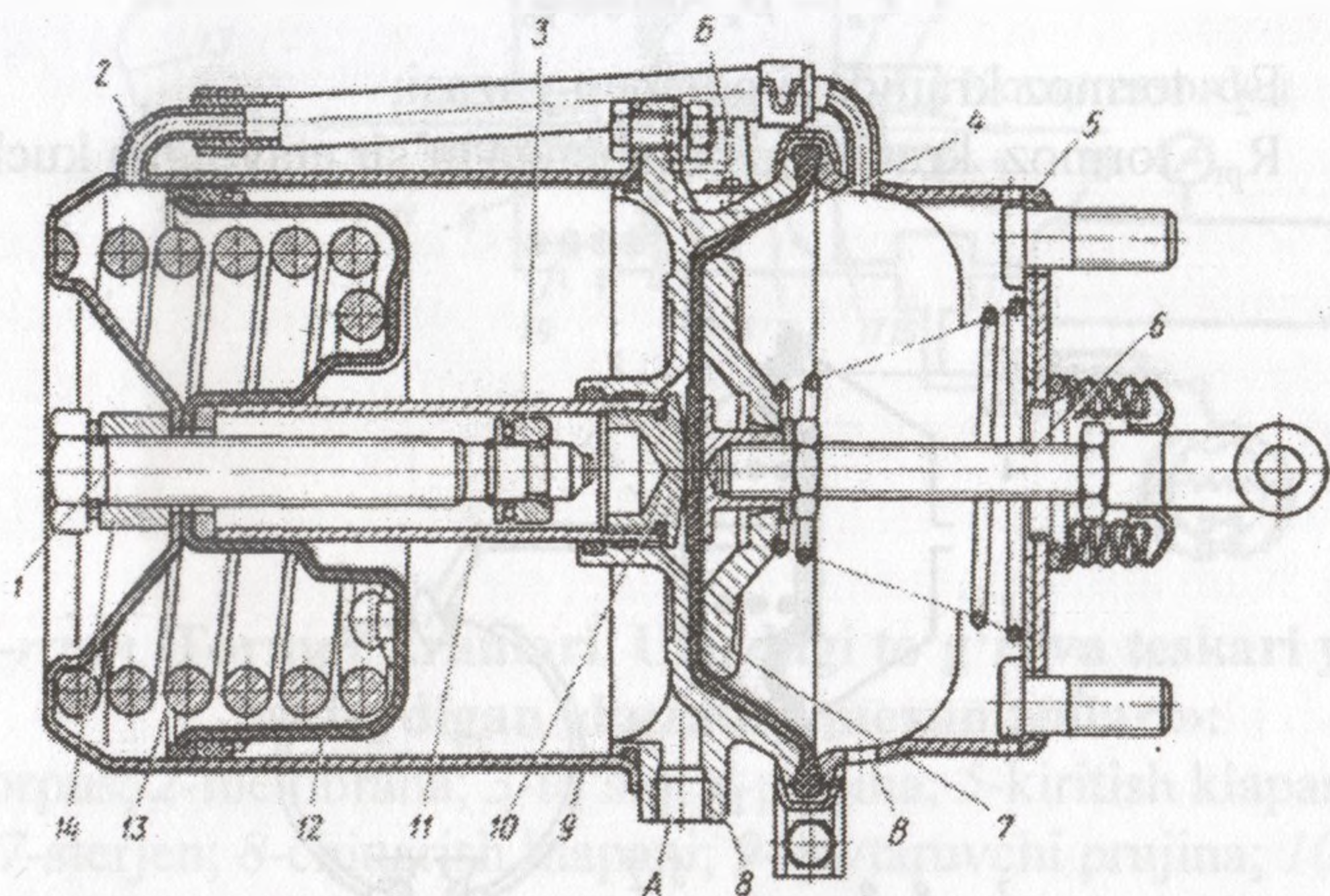
12.19-rasm. Prujina energiya akkumulyatorli tormoz kamerasi:
