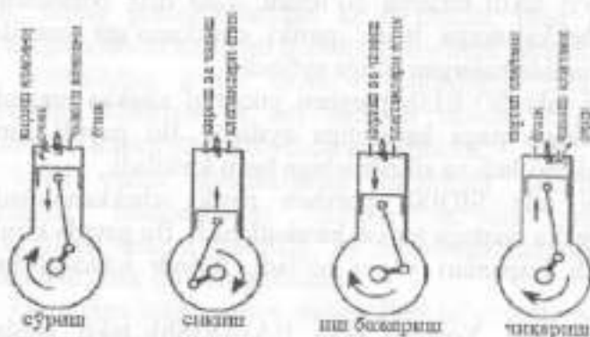
3.12-рasm. To'rt taktli dvigatellarda taktlarni bajarilishi
