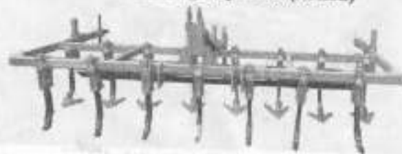
3.36-rasm. ChPK-3 rusumli kombinatsiyalashgan tuproqqa ishlov beruvchi chizel
