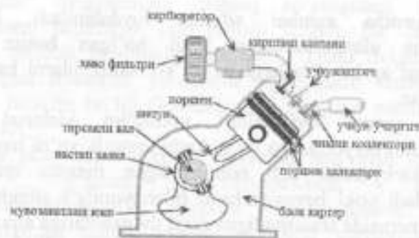
Карбюраторная двигательная установка
