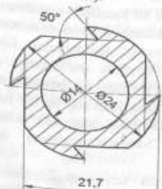
2.5-rasm. Paxta terish shpindelining ko'ndalang kesimi sxemasi
