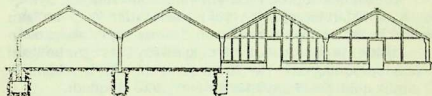
22- rasm. Arkli issiqxonaning ko'ndalang kesimi.
