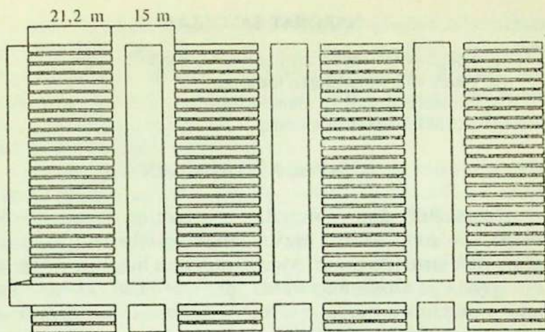
23- rasm. Parniklarning joylashtirilishi.
