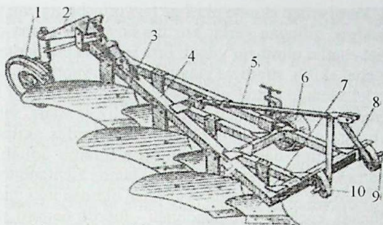
6-rasm Ikki yarusli plug PD-4-35:
