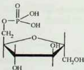
\beta -D-Fruktoza-6-fosfat
