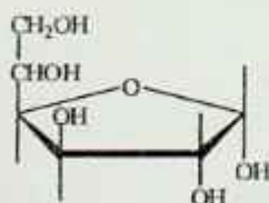
Glukofuranoza
