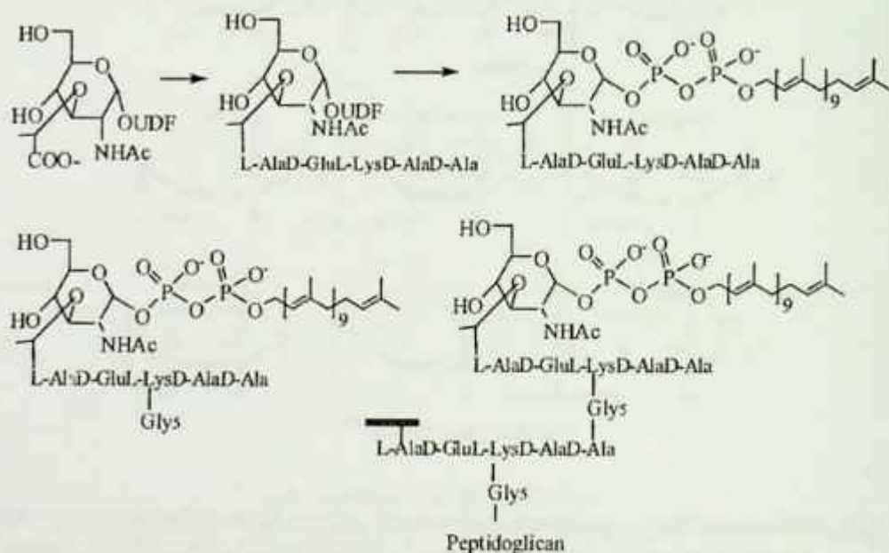
Bakteriyalar hujayra devorlari biosintezi sxemasi.
