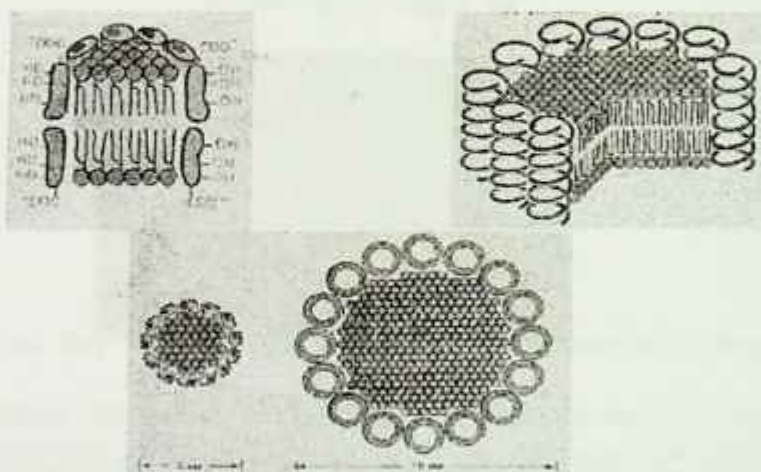
23-rasm. Disksimon mitsellyar agregatlar
