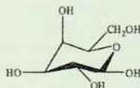
Galaktoza
