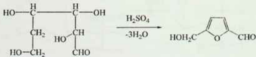
α-Oksimetilfurfurol
