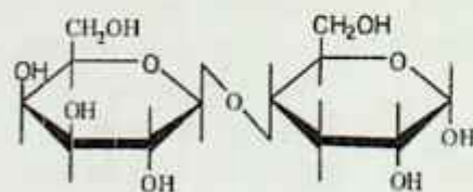
Laktoza
