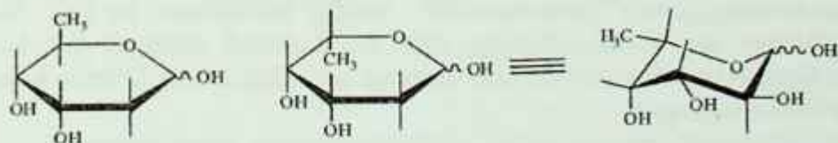
D-Digitoksoza
