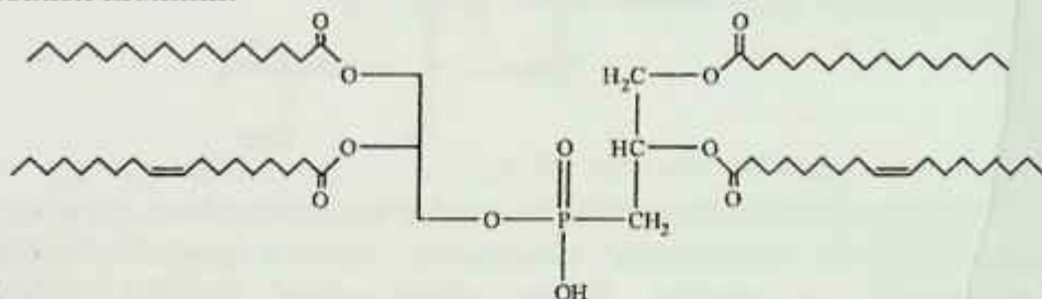
Fosfatidilglukozaminilglitserin
