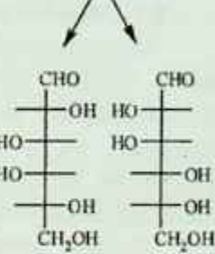
D-galaktoza D-taloza
