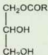
1(3)-monoglitsерид [1(3)-monoalkilglitsерин]
