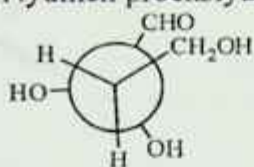
To'silgan konformatsiya
