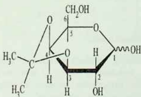
D-Galaktoza -3,4-ketal
