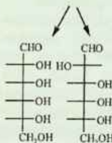
D-alloza D-altroza
