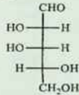
D-liksoza
