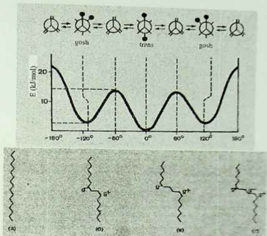
32-rasm. Uglevodorod zanjirida tutashgan gosh-trans-izomerlanish natijasida siniqlarning (kinklar) shakllanishi:
