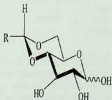
D-Glukoza-4,6-asetal
