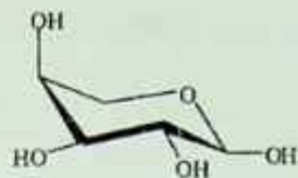
L-Arabinosa
