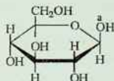
\beta -D-glukopiranoza
