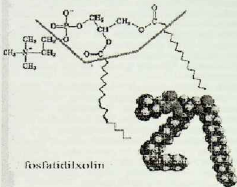
17-rasm. Fosfatidilxolinning tuzilishi.
