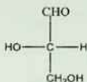
L-glitserin aldegid
