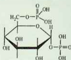
\alpha -D-Glukoza-1,6-difosfat
