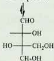
D- apioza
