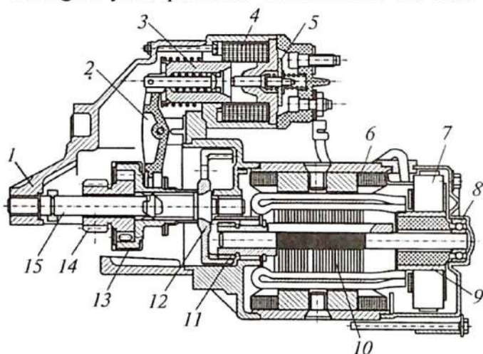
2.13-rasm. Ichki ilashgan reduktorli starter:
