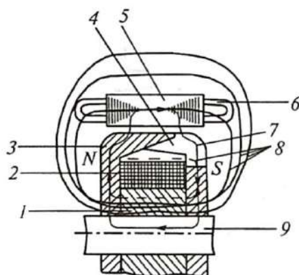
1.17-rasm. Generatorning magnit tizimi.
