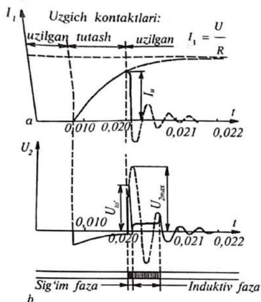
3.3-rasm. Uzgich kontaktlari ulanganda va uzilganda birlamchi tok ( i_1 ) va ikkilamchi kuchlanish ( U_2 ) ni o'zgarishi (kontakt uzilgan daqiqadan boshlab vaqt masshtabi 10 marta oshirilgan).
