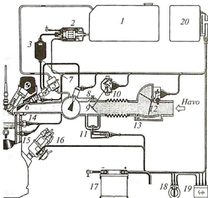
6.3-rasm. «L-Jetronic» yonilg'i purkash tizimining tarkibiy chizmasi:
