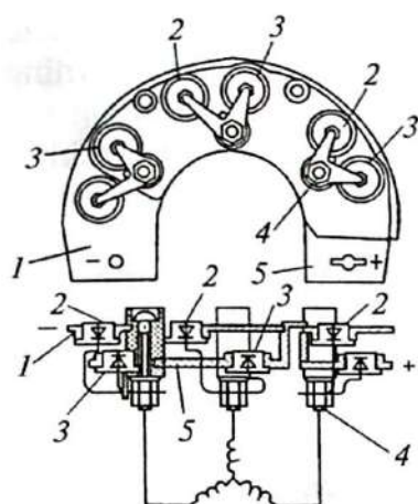
1.24-rasm. БПВ turidagi to'g'rilagich bloki.
