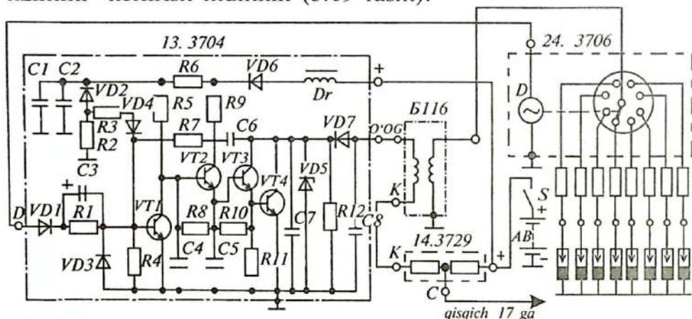
3.19-rasm. Magnitoelektr datchikli kontaktsiz o't oldirish tizimining umumiy chizmasi.
