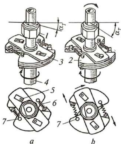
3.5-rasm. Markazdan qochma rostlagichni ishlashi:
