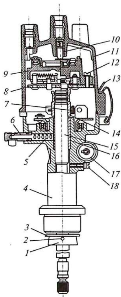
3.11-rasm. 30.3706 belgili uzgich-taqsimlagich:
