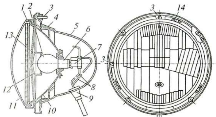
5.4-rasm. \Phi\Gamma 140 belgili avtomobil farasi.
