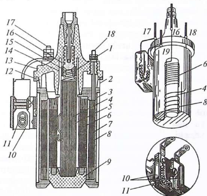
3.9-rasm. O't oldirish g'altagi.
