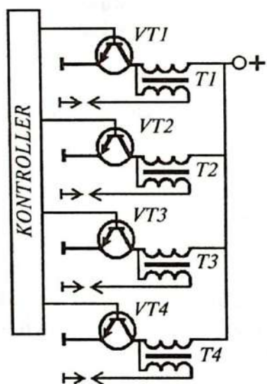
3.24-rasm. Har bir silindrga alohida o'rnatilgan g'altaklarning ulanish chizmasi.
