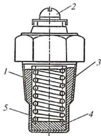
4.1-rasm. Termorezistorli harorat datchigi.
