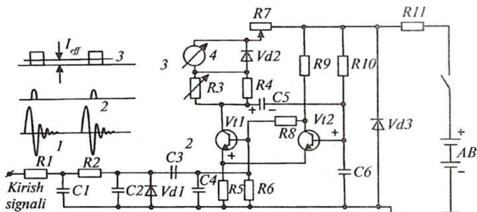
4.15-rasm. Elektron taxometr chizmasi.
