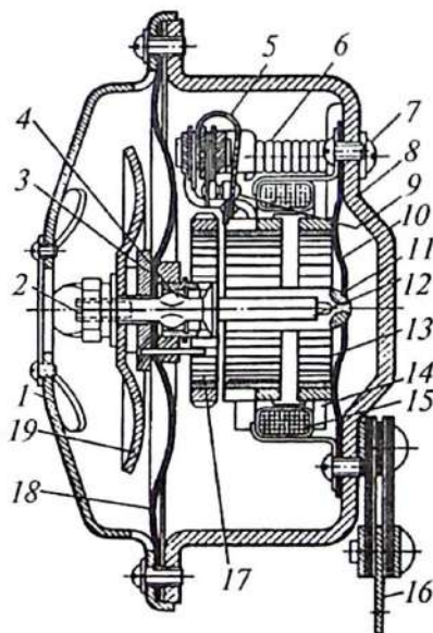
7.7-rasm. Shovqinli (karnaysiz) tovush signali:
