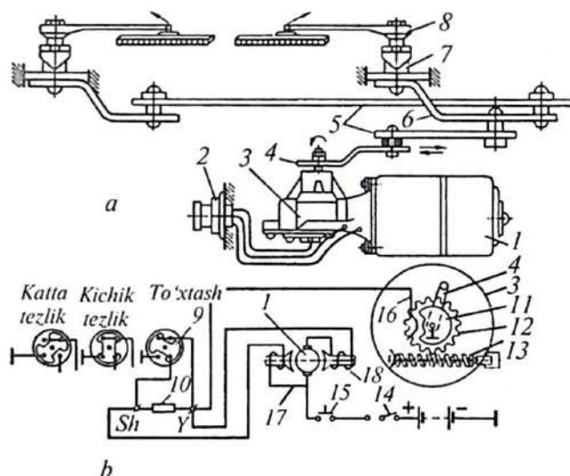
7.3-rasm. Oynatozalagich:
