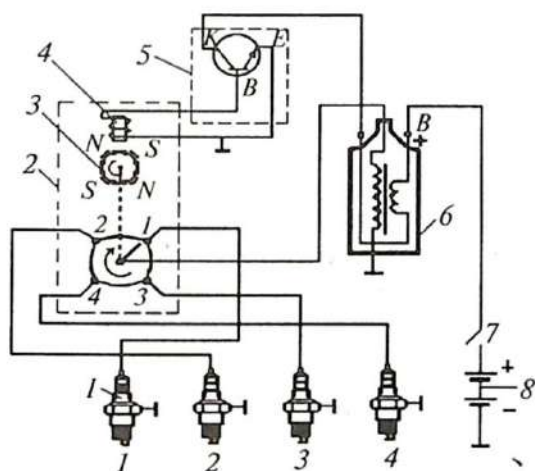
3.14-rasm. Magnitoelektr datchikli kontaktsiz-tranzistorli o't oldirish tizimi.
