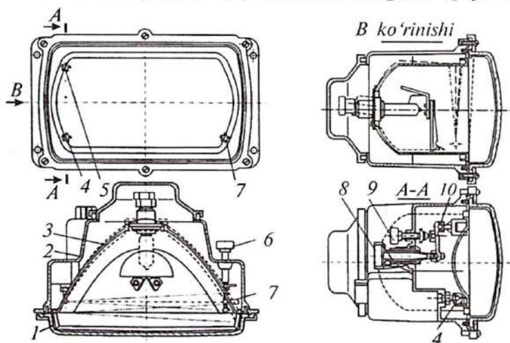
5.5-rasm. To'g'ri burchakli faralarning tuzilishi.
