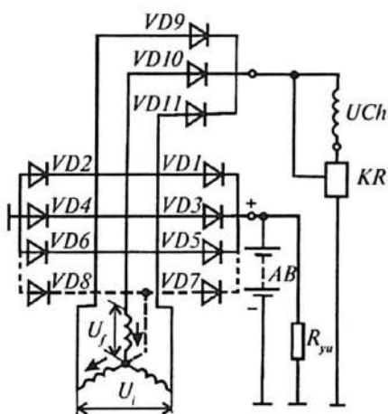
1.20-rasm. Oʻz-oʻzini uygʻotuvchi oʻzgaruvchan tok generatorining chizmasi.
