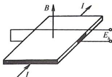
3.17-rasm. Yarimo'tkazgichli datchikning ishlash prinsipi.
