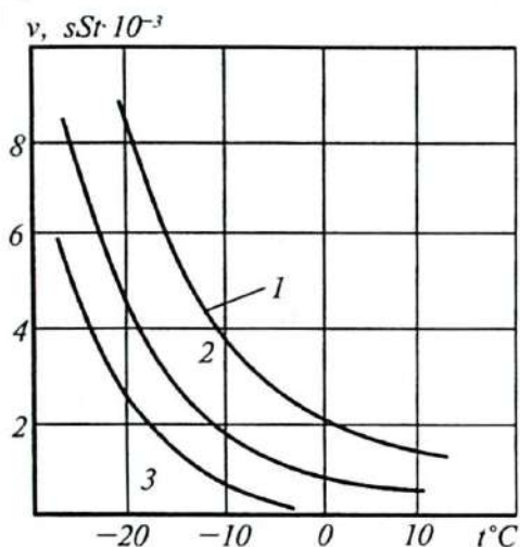
2.2-rasm. Motor moylari qovushqoqligining haroratga bog'liqligi:
