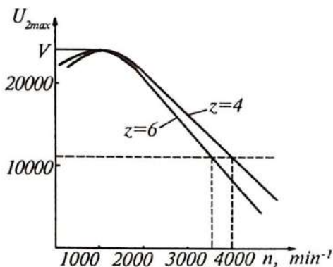
3.4-rasm. Kontaktli o't oldirish tizimining ishchi tavsifnomasi.
