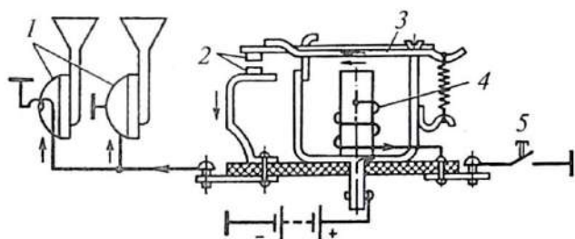
7.6-rasm. Signallar relesining ulanish chizmasi.
