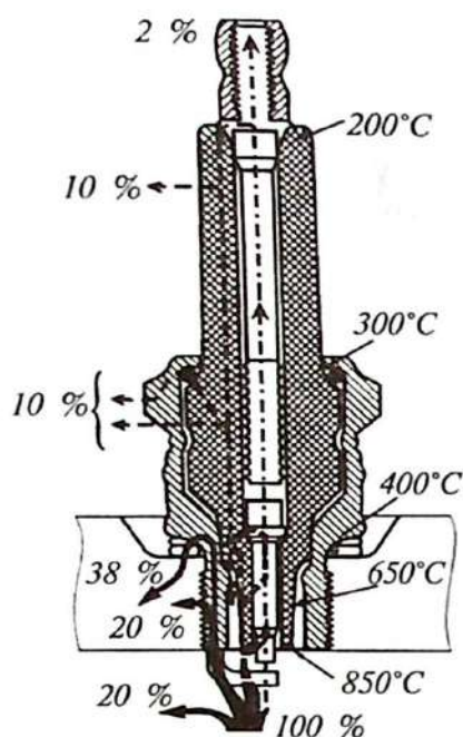
3.27-rasm. O't oldirish shamidan issiqlikni chiqish muhiti.
