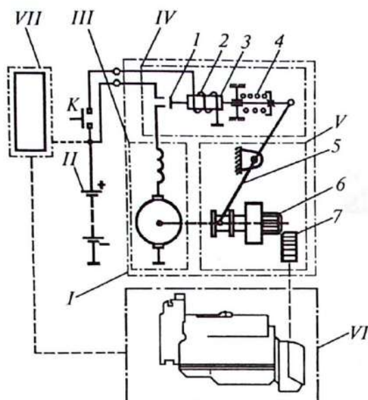
2.1-rasm. Dvigatelni ishga tushirish tizimining umumiy chizmasi:
