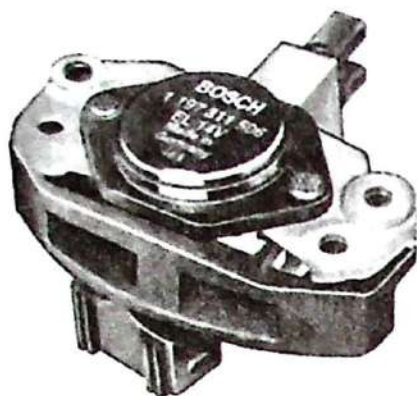
1.34-rasm. «BOSCH» (Germaniya) firmasining kuchlanish rostlagichi—choʻtkatutqich tuguni.
