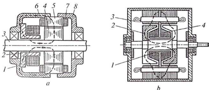
1.28- pacm. Induktorli ( a ) va qisqartirilgan qutbli ( b ) kontaktsez (choʻtkasiz) generatorlar.
