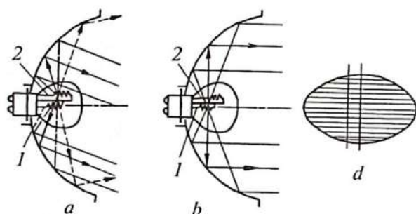
5.3-rasm. Amerika yorug'lik taqsimlash tizimidagi optik sistemalarda nur tarqalish chizmasi:
