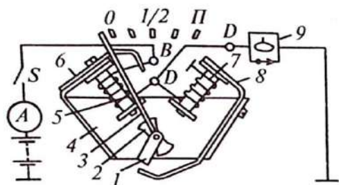
4.9-rasm. Elektromagnitli yonilg'i sathi ko'rsatkichi.
