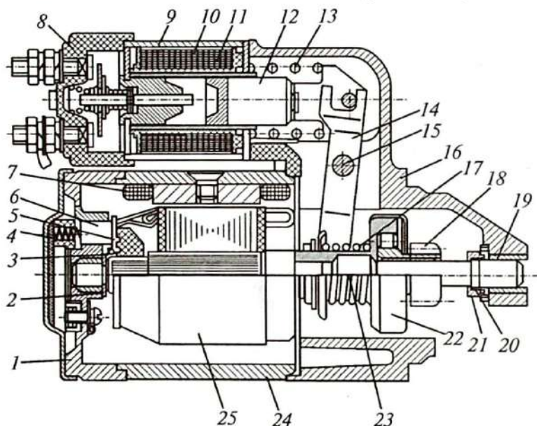
2.8-rasm. Ko'ndalang kollektorli 26.3708 belgili starter:
