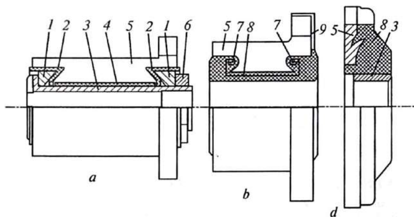
2.7-rasm. Starterlarning kollektorlari:
