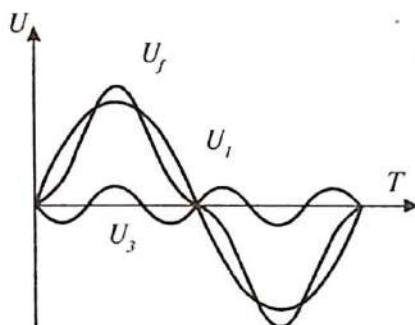
1.21-rasm. Faza kuchlanishi U_f ni birinchi U_1 va uchinchi U_3 garmonika sinusoidalarning yig'indisi shaklidagi ko'rinishi.
