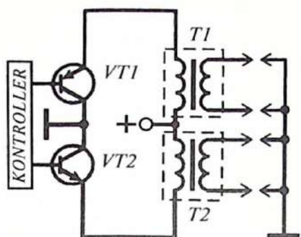
3.22-rasm. Ikki chiqish joyiga ega bo'lgan o't oldirish g'altagini ulash chizmasi.
