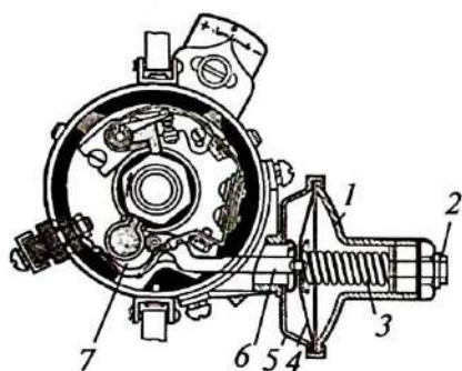
3.6-rasm. Vakuum-rostlagich.
