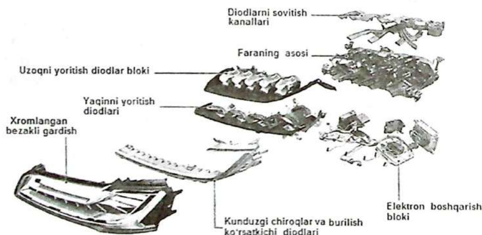
5.9-rasm. Yorug'lik diodlari asosidagi Matrix LED farasi.
