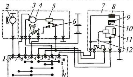
7.4-rasm. CJL-136 belgili oynatozalagich elektr yuritmasining umumiy chizmasi.
