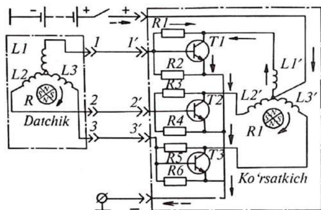
4.14-rasm. Elektr yuritmalı spidometr chizması.
