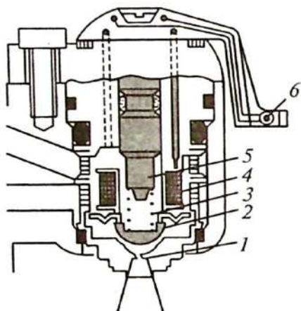
6.5-rasm. Markaziy purkash forsunkasi:
