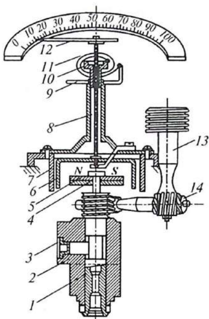
4.12-rasm. Spidometrning tezlik o'lchash mexanizmi.
