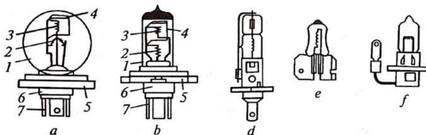
5.15-rasm. Avtomobil faralarida ishlatiladigan lampalar:
