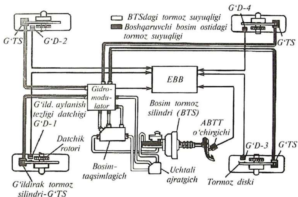
6.10-rasm. ABTTli to'rt tarmoqli gidravlik tormoz tizimi.
