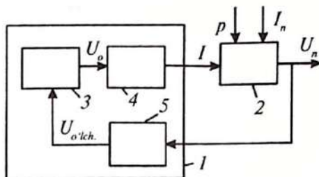
1.29-rasm. Generator kuchlanishini rostlashning tarkibiy chizmasi.
