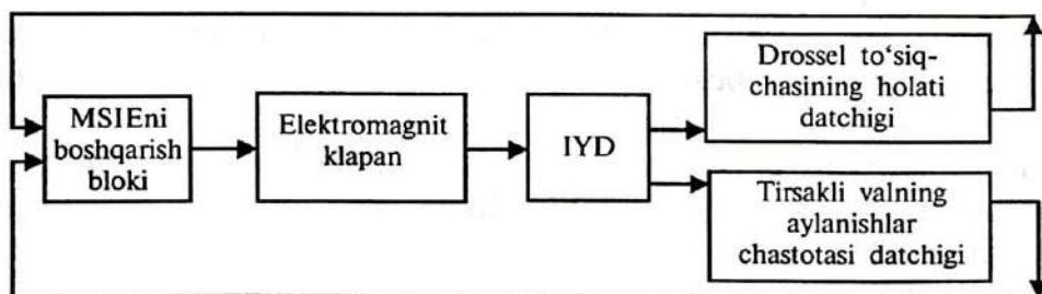
6.1-rasm. MSIEEBTning tarkibiy chizmasi.
