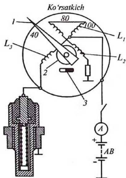
4.3-rasm. Logometrik termometrning umumiy chizmasi.
