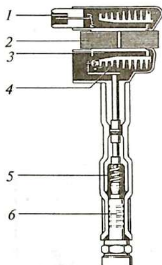
3.25-rasm. O't oldirish transformatori:
