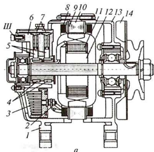
1.23-rasm. 32.3701 belgili o'zgaruvchan tok generatori: a—ko'ndalang kesimi; b—asosiy qismlari.
