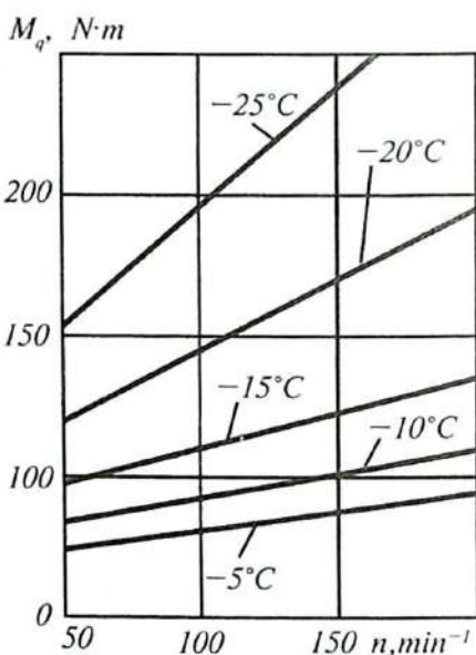
2.3-rasm. Qarshilik momentini dvigatelning aylanishlar chastotasi va moy haroratiga bog'liqligi.
