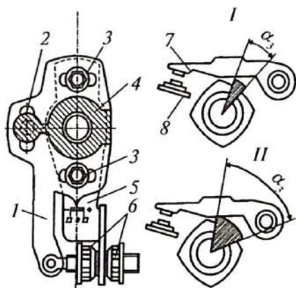
3.7-rasm. Oktan-korrektor:
