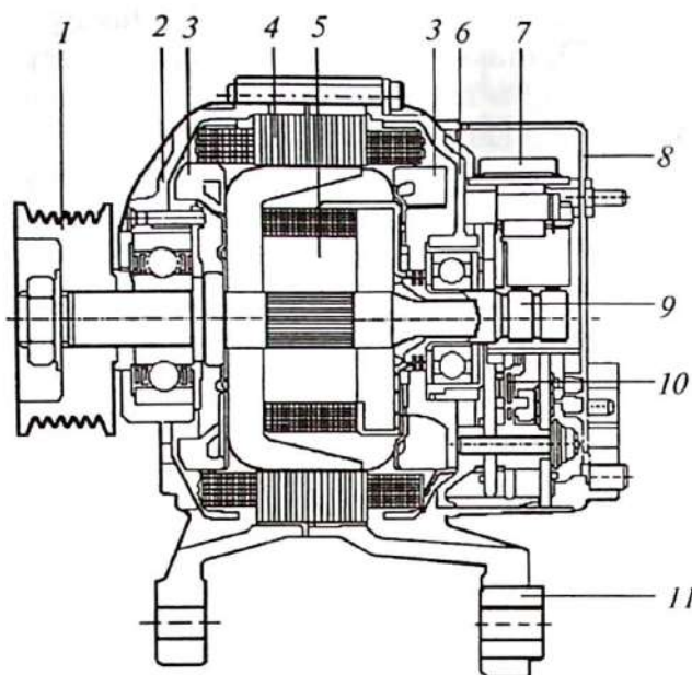
1.27-rasm. «BOSCH» firmasining kompakt (ixcham) generatori:
