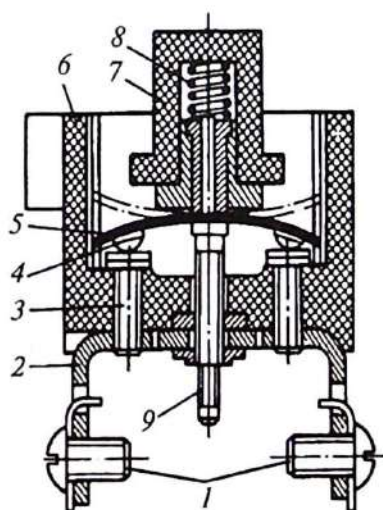
8.5-rasm. Bir marta ishlaydigan termobimetall saqlagichlar.
