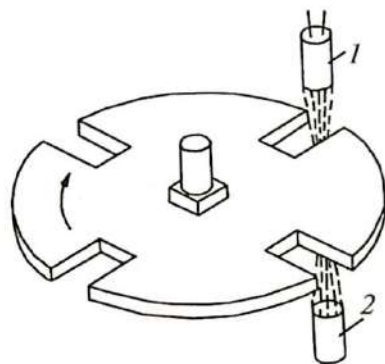
3.16-rasm. Fotoelektr datchikning umumiy chizmasi.
