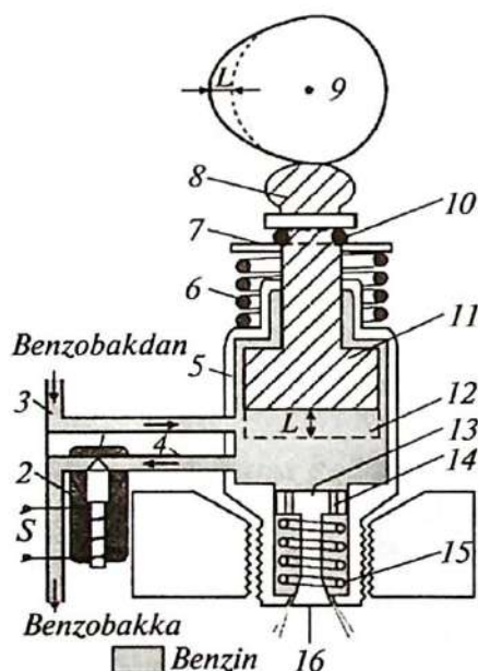
6.9-rasm. Bevosita silindrlarga purkash tizimining nasos-forsunkasi:
