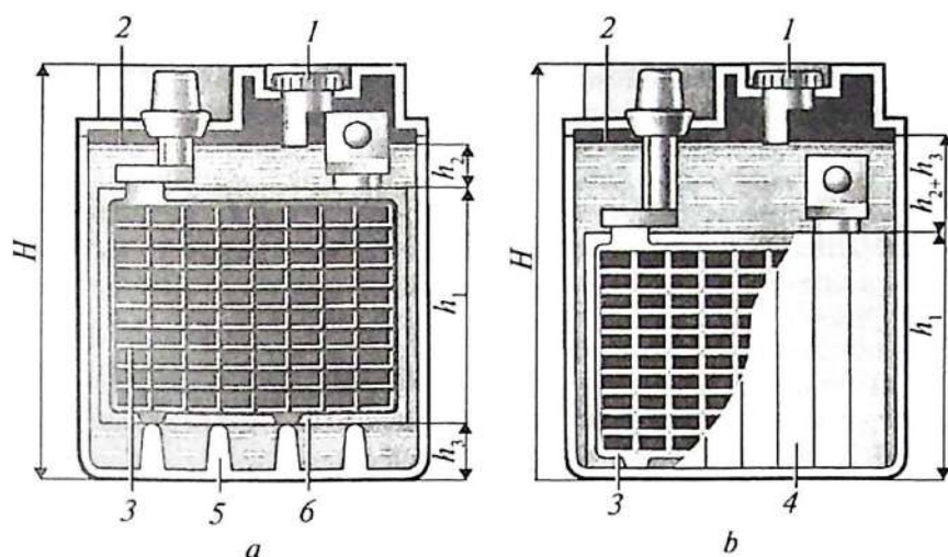
1.6-rasm. Separator-konvert ishlatilganda akkumulatorga quyiladigan elektrolit miqdorining ortishi:
