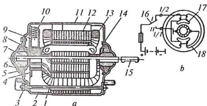
7.1-rasm. Elektromagnitli uyg'otish tizimidagi elektrodvigatel:
