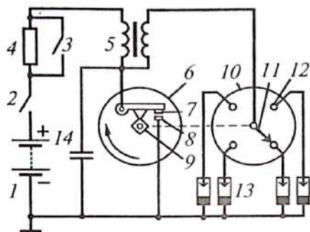
3.2-rasm. Kontaktli o't oldirish tizimining umumiy chizmasi.
