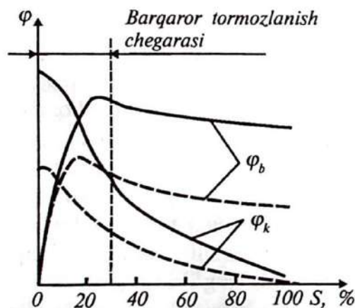
6.11-rasm. Avtomobil g'ildiraklarini yo'l bilan bo'ylama \varphi_b va ko'ndalang \varphi_k yo'nalishdagi tishlashish ko'effitsiyentlarini sirpanish S ga bog'liqligi: sidirg'a chiziq—quruq yo'l; punktir chiziq—ho'l yoki muzlagan yo'l.
