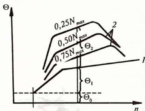
3.8-rasm. Markazdan qochma va vakuum-rostlagich birgalikda ishlaganda o't oldirishning ilgarilatish burchagining o'zgarishi:
