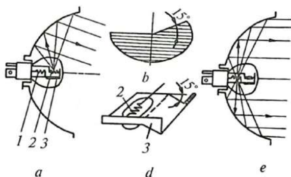
5.2-rasm. Yevropa yorug'lik taqsimlash tizimidagi optik sistemalarda nur tarqalish chizmasi:
