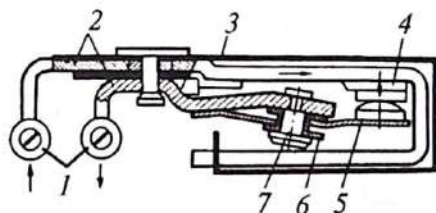
8.4-rasm. Uzluksiz ishlaydigan termobimetall saqlagichlar.
