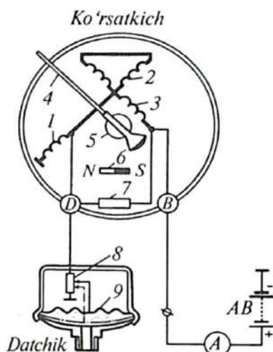
4.6-rasm. Magnitoelektr (logometrik) manometrning umumiy chizmasi:
