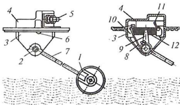
4.8-rasm. Yonilg'i sathini o'lchash asbobining reostatli datchigi.
