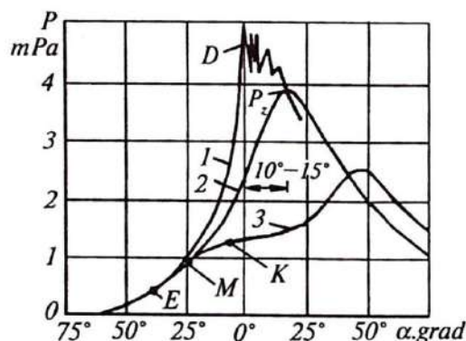
3.1-rasm. Dvigatel silindrlaridagi bosimning o't oldirish daqiqasiga bog'liqligi: I —ertaroq o't oldirilganda ( D —detonatsiya); 2—me'yorida o't oldirilganda; 3—kechroq o't oldirilganda. O't oldirish daqiqalari: E —erta; M —me'yorida; K —kech.
