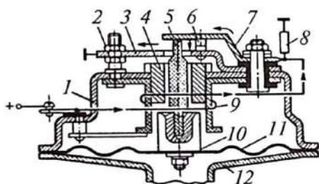
7.5-rasm. Elektr tovush signali.
