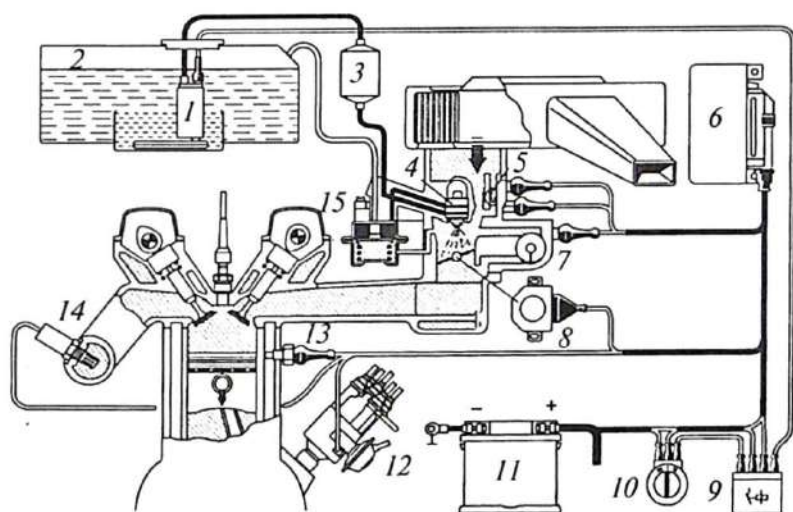
6.4-rasm. Bir nuqtali «Mono-Jetronic» yonilg'i purkash tizimi:
