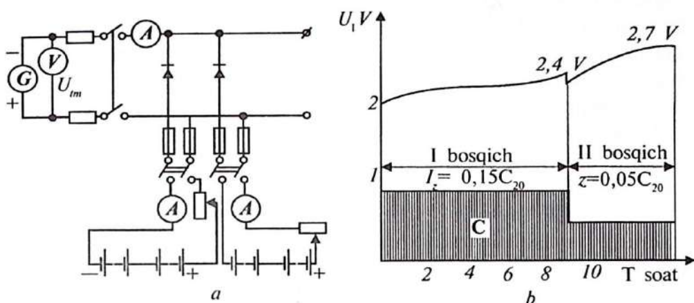
1.10-rasm. Akkumulatorlar batareyasini tok qiymati o'zgarmas bo'lganda zaryad qilish:
