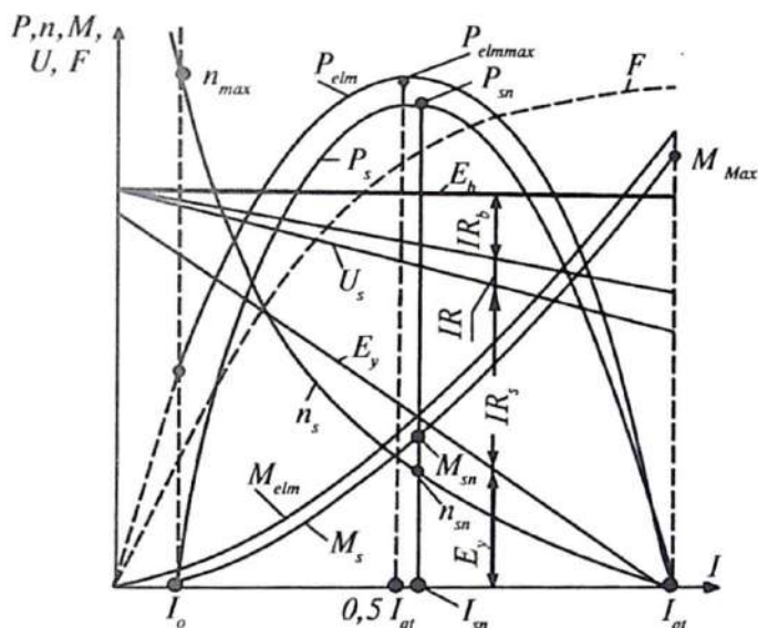
2.4-rasm. Starterning elektromexanik tavsifnomasi.
