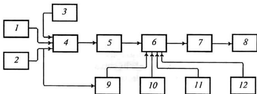
6.2-rasm. Benzinli dvigatellarda yonilg'i purkalishini elektron boshqarish tizimining tarkibiy chizmasi.
