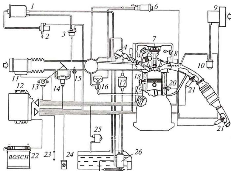
6.8-rasm. «Motronic 3.1» yonilg'i purkash tizimining tarkibiy chizmasi:
