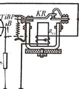
1.31-rasm. Kontakt-tranzistorli kuchlanish rostlagichining umumiy chizmasi.
