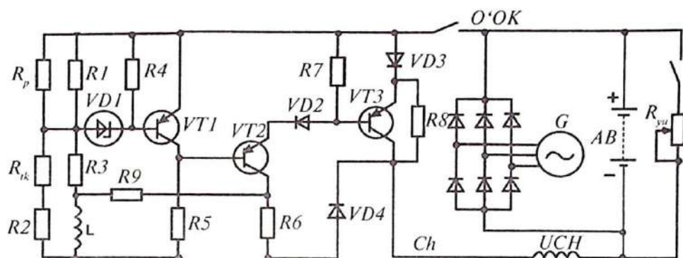
1.32-rasm. PP-350 belgili kuchlanish rostlagichining chizmasi.
