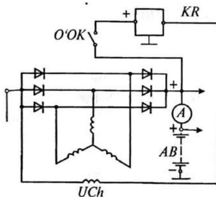
1.19-rasm. Tashqaridan uyg'otiladigan o'zgaruvchan tok generatorining chizmasi.
