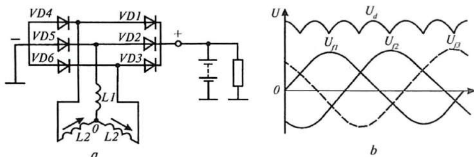
1.18-rasm. Uch fazali ikki yarimdavrlı to'g'rilagich chizmasi.
