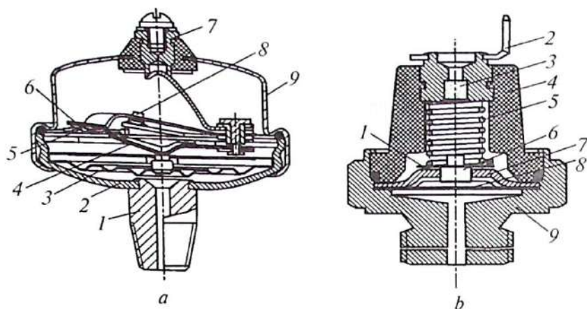
4.7-rasm. Avariya bosim xabarchilarining datchiklari: a—MM10 (membranali); b—MM120 (prujinali).
