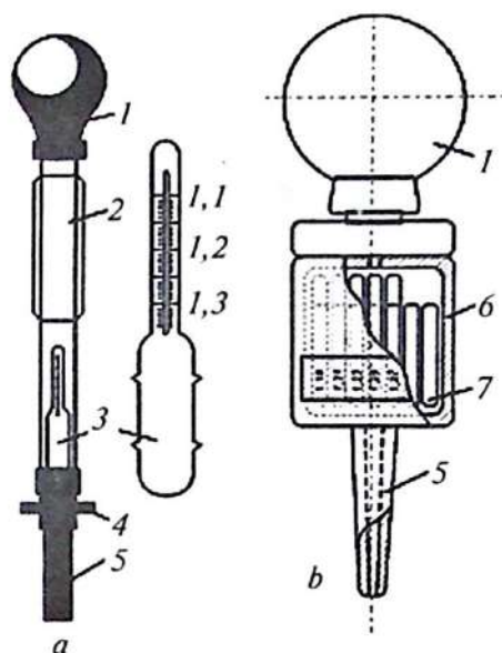
1.13-rasm. Elektrolit zichligini o'lchash asboblari:
