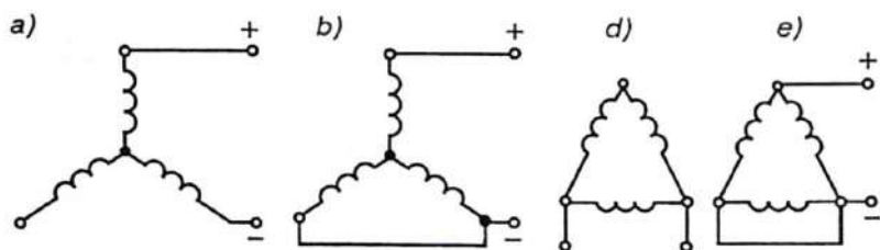
4.12- rasm. Dinamik tormozlashda asinxron dvigatel stator chulg'amlarini o'zgarmas (to'g'rilangan) tok manbayiga ulash sxemasi.
