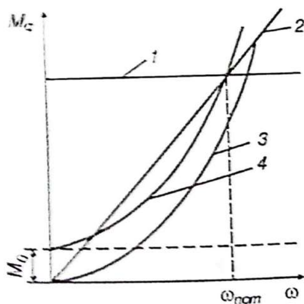
1.3- rasm. Statik momentning tezlikka bog'liqligi: 1 — tezlikka bog'liq bo'lmagan (o'zgarmas) moment; 2 — tezlikka chiziqli bog'liq bo'lgan moment; 3 — burchak tezlik kvadratiga proporsional bo'lgan moment; 4 — burchak tezlikka proporsional va o'zgarmas tashkil etuvchisi bo'lgan moment.
