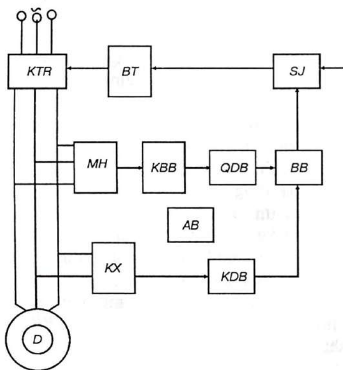
9.1- rasm. Energiyani tejaydigan asinxron elektr yuritma.
