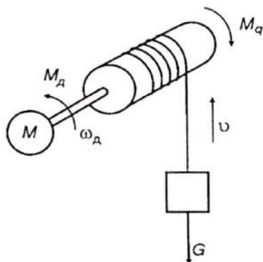
1.6- rasm. Yuk ko'taruvchi qurilmaning soddalashtirilgan kinematik sxemasi.
