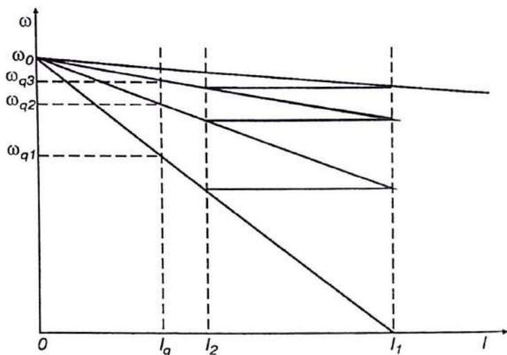
6.4- rasm. Dvigatelni reostat yordamida ishga tushirilgan holatidagi mexanik tavsiflar.
