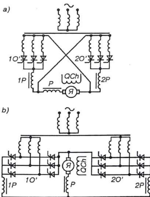
3.10- rasm. BO'-D reversiv tizimining ikkita komplekt ventildan foydalanilgan kuchli zanjir sxemasi: a — almashilgan nol chiqishli; b — ko'priksimon o'zgartgichli.
