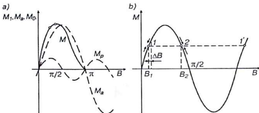
4.17- rasm. Burchak statik tavsiflari: a — ochiq ko'rsatilgan qutbli; b — reaktiv dvigatel.
