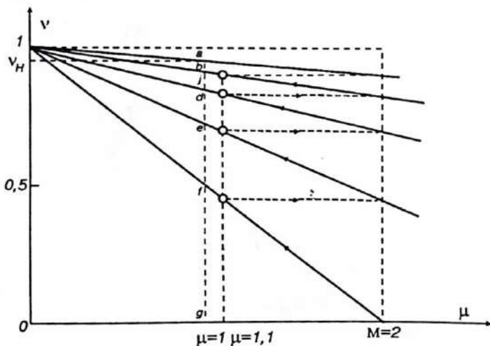
2.3- rasm. Mustaqil qo'zg'atishli o'zgarmas tok dvigatelinini ishga tushirish reostatlari qiymatini hisoblash.
