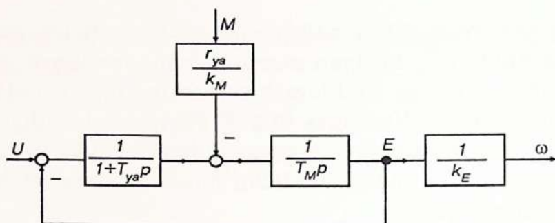
5.1- rasm. Mustaqil qo'zg'atishli o'zgarmas tok dvigatelining tezlikni mo'tadillash tizimidagi tuzilish sxemasi.
