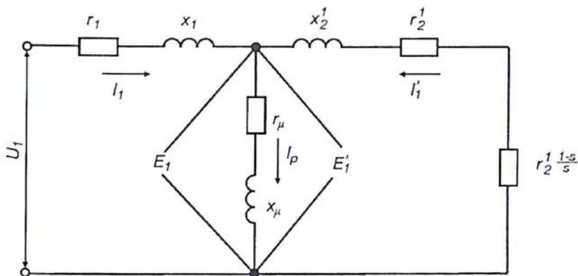
4.1-rasm. Asinxron mashina parametrlarini ikkilamchi zanjirdan (rotordan) birlamchi zanjirga (statorga) keltirilgan holatdagi bitta fazaning ekvivalent sxemasi.
