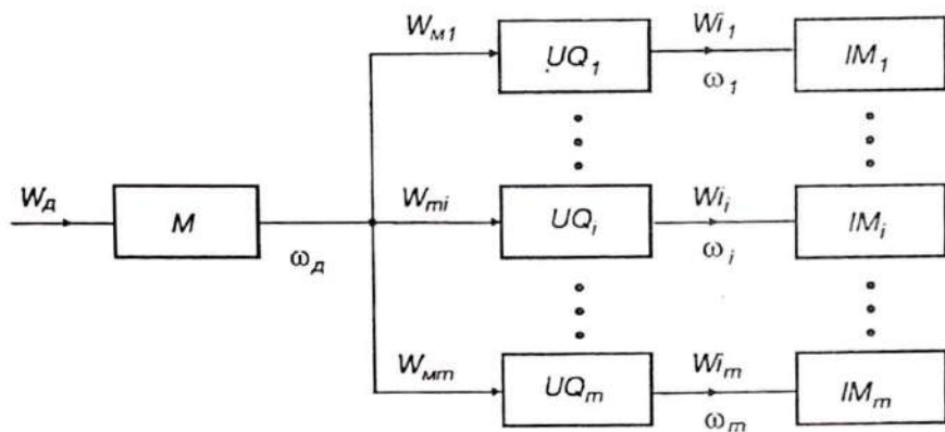
2-rasm. Guruhli elektr yuritmaning funksional sxemasi.
