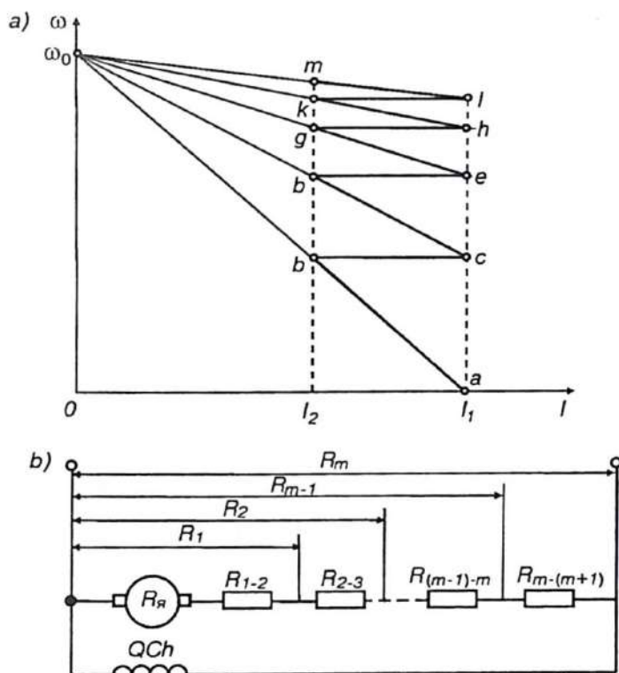
2.13- rasm. Mustaqil qo'zg'atishli dvigatelni ishga tushirish diagrammasi (a) va rezistor seksiyalarining ulanish sxemasi (b).
