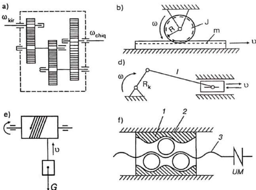
1.2- rasm. Uzatish qurilma turlari: a — reduktor; b — tishli-reykali uzatma; d — krivoship-shatunli mexanizm; e — yuk ko'tarish barabani; f — vint-tebranma gayka uzatmasi.
