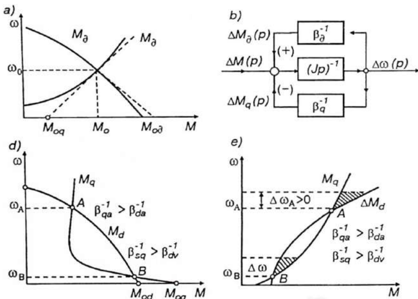
1.7-rasm. Elektr yuritmaning statik ustuvorligini aniqlash:
