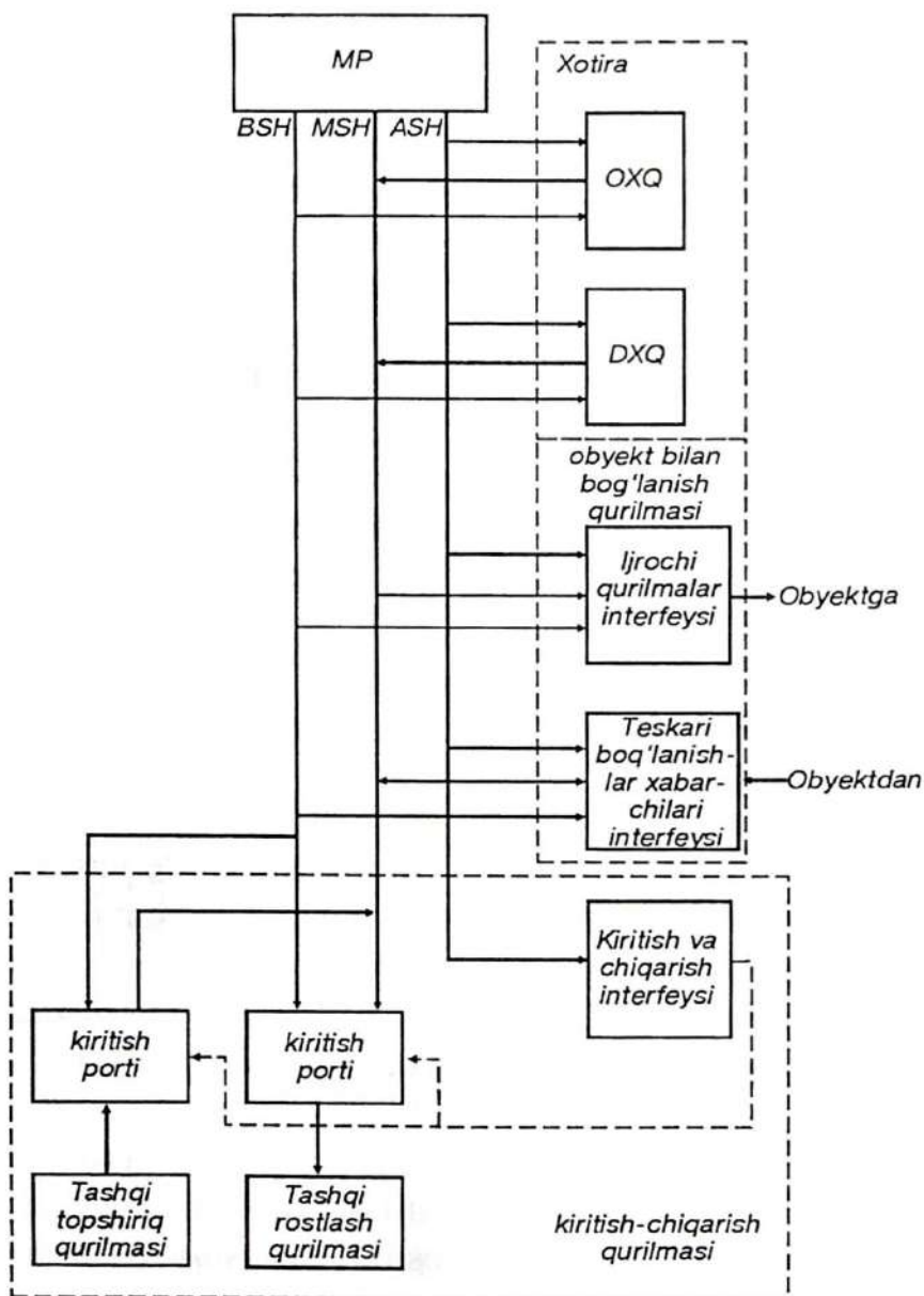
8.2- rasm. MP tizimining tuzilish sxemasi.
