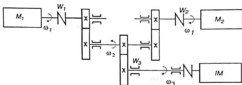
4- rasm. Ko'p dvigatelli elektr yuritmaning funksional sxemasi.
