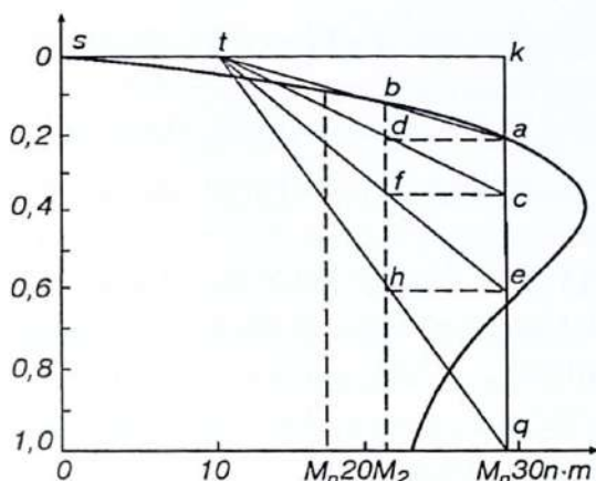
4.9- rasm. Asinxron dvigatelning ishga tushirish reostatini hisoblash grafigi.
