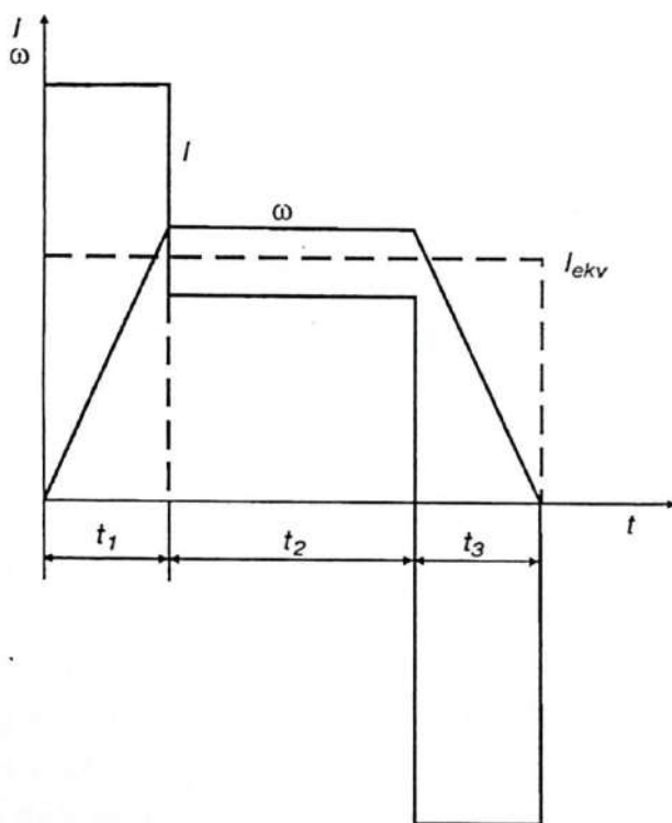
7.5- rasm. Dvigatelning qisqa ish grafigi.
