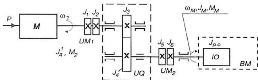
1.1- rasm. Elektr yuritma mexanik qismining funksional sxemasi: M — dvigatel, UM_1 va UM_2 — ulanish muftalari; UQ — uzatish qurilmasi (reduktor); IO — ijrochi mexanizmning ish organi.
