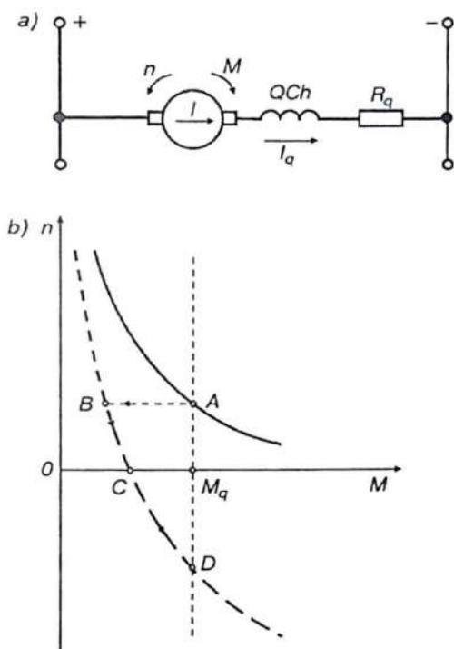
2.26- rasm. Dvigatelning aktiv statik moment ostida teskari ulash va reverslash rejimidagi mexanik tavsiflari.
