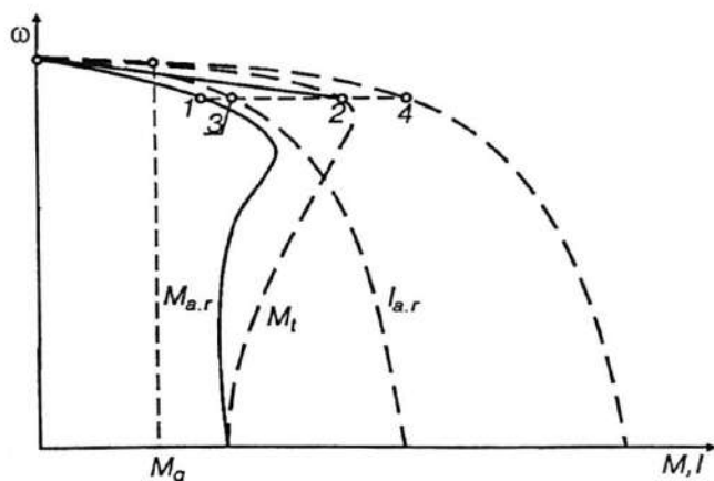
4.8- rasm. Dvigatel statoridagi tok va elektromagnit momentlarning tabiiy tavsifda ( M_t , I_t ) va sun'iy tavsiflarda aktiv-reaktiv qarshiliklarni ulab ishga tushirishdagi ( M_{a,r} , I_{a,r} ) bog'lanishlar.
