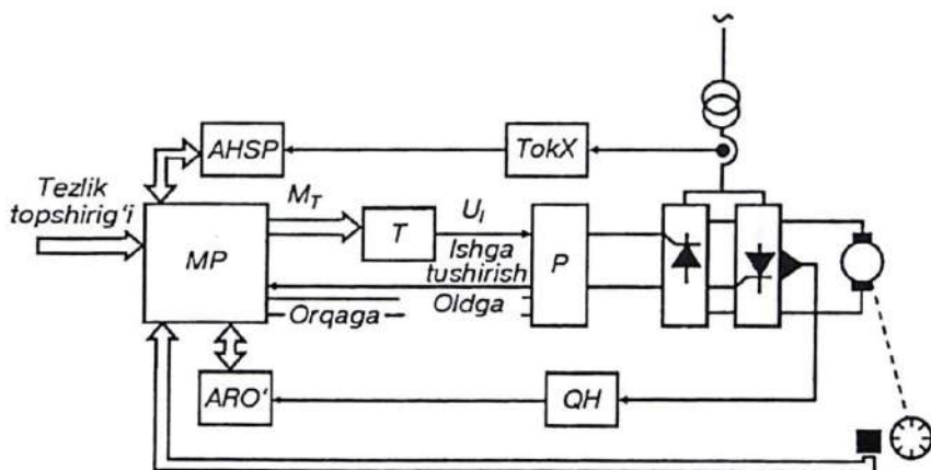
8.4- rasm. Elektr yuritmaning mikroprotessorli tizimi.
