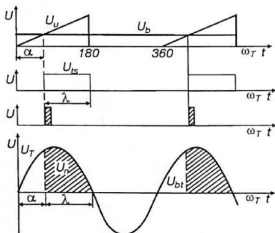
3.6- rasm. Boshqariluvchi to'g'rilagich tizimida signallar diagrammasi.
