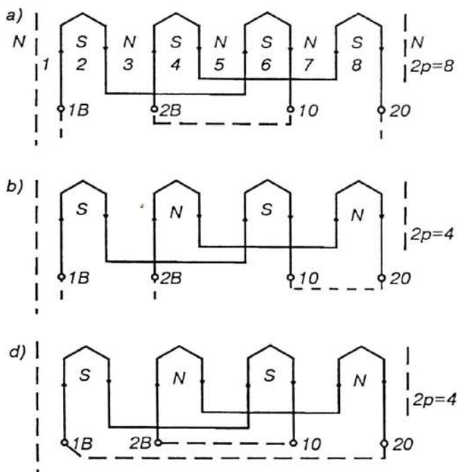
4.14- rasm. Koʻp fazali asinxron dvigatelning stator fazalari seksiyalarining ulanish sxemalari: juft qutblar sonini 2p = 8 (a) va 2p = 4 ni seksiyalarni ketma-ket (b) va parallel (d) ulagan holatdagi sxemalari.
