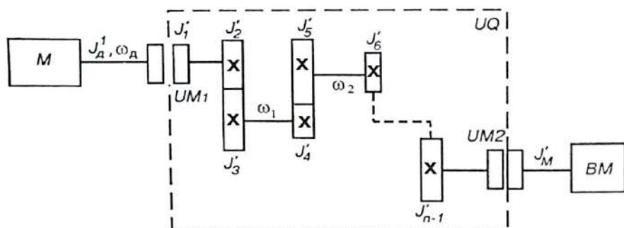
1.5- rasm. Elektr yuritmaning kinematik sxemasi.
