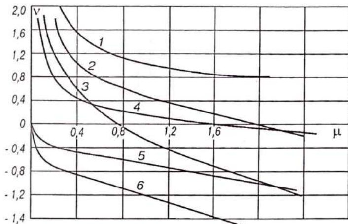
2.18- rasm. Dvigatelning 2.17- rasm, a dagi sxema bo'yicha qo'shimcha rezistor ulangan holatidagi mexanik tavsiflari.
