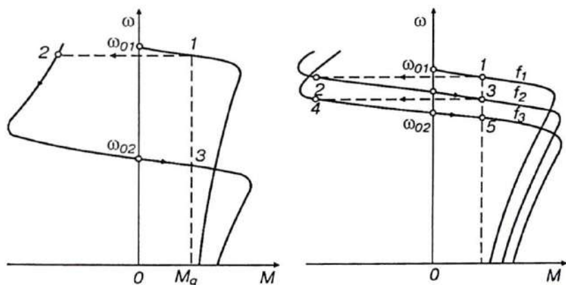
4.10- rasm. Asinxron dvigatelning reaktiv statik moment qo'yilganda generator tormozlash rejimidagi mexanik tavsiflari:
