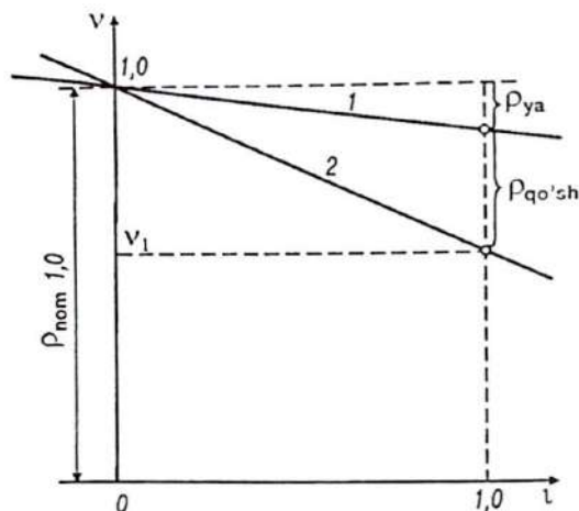
2.12- rasm. Mustaqil qo'zg'atishli dvigatelning mexanik tavsifini qurish.
