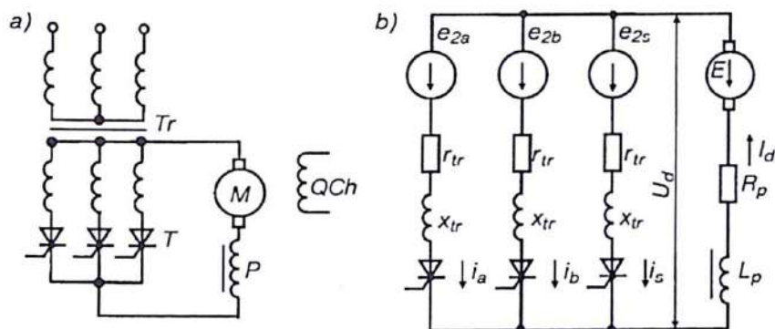
3.7- rasm. Uch fazali nul sxemali o'zgartgich BO'-D tizimi: a — tizim kuchli zanjirining soddalashtirilgan prinsiplal sxemasi; b — ekvivalent sxemasi.
