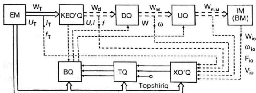
I- rasm. Avtomatlashtirilgan elektr yuritmaning funksional sxemasi.
