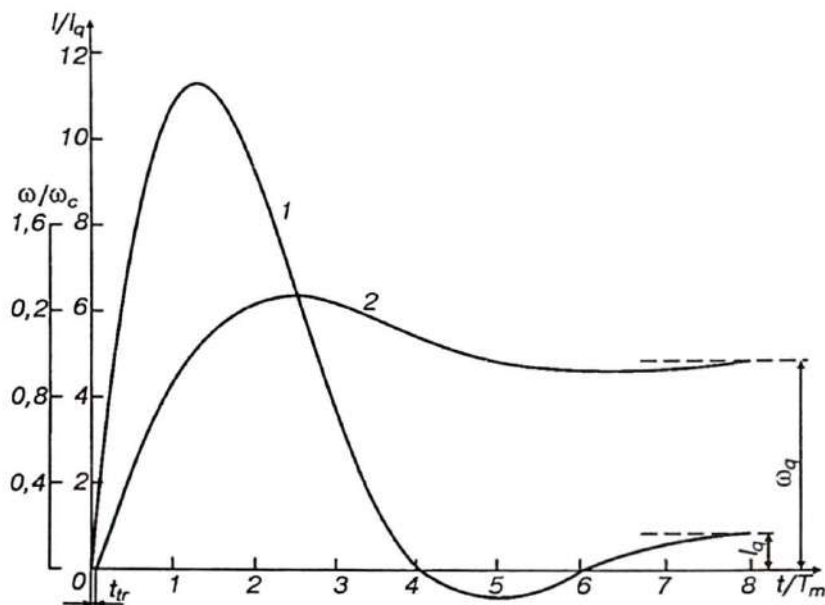
6.7- rasm. Mustaqil qo'zg'atishli dvigatelni reostatsiz ishga tushirganda tok va tezlikning o'tkinchi tavsifi. 1 — nisbiy birliklarda tok egri chizig'i; 2 — tezlik.
