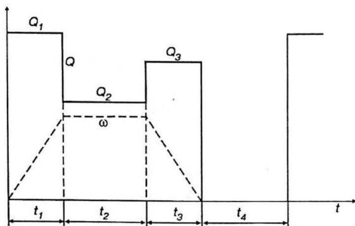
7.4- rasm. Tezlikning trapetsioidal diagrammasi va dvigateldagi isroflar grafigi.
