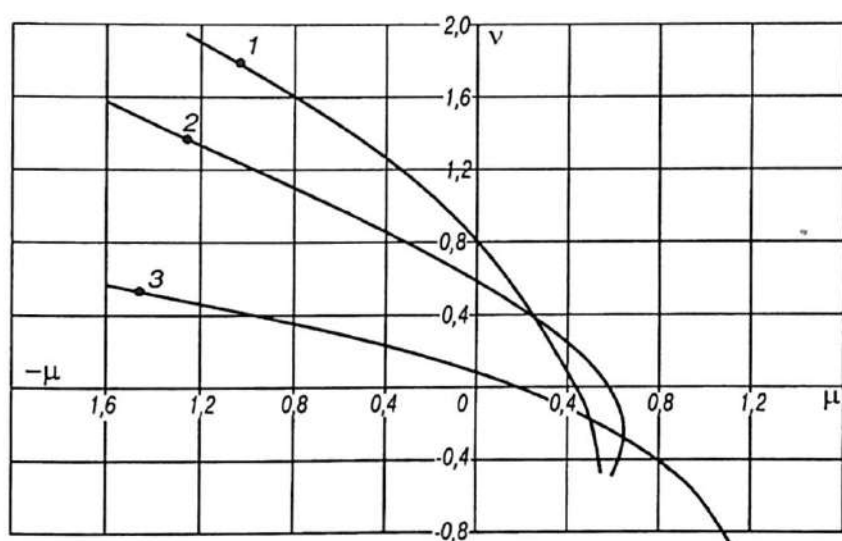
2.21- rasm. Dvigatelning 2.17- rasm, e dagi sxema bo'yicha qo'shimcha rezistorlar ulangan holatdagi mexanik tavsiflari.
