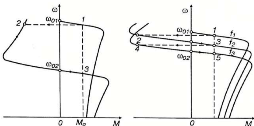
4.11- rasm. Asinxron dvigatelning ulanish sxemasi va mexanik tavsiflari: a — reaktiv statik momentda teskari ulanish rejimida; b — shuning o'zi, aktiv statik momentda.
