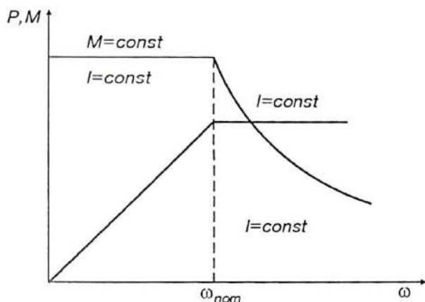
3.3- rasm. Generator-dvigatel tizimida o'zgarmas moment va quvvatda tezlikni rostdlash rejimlari.
