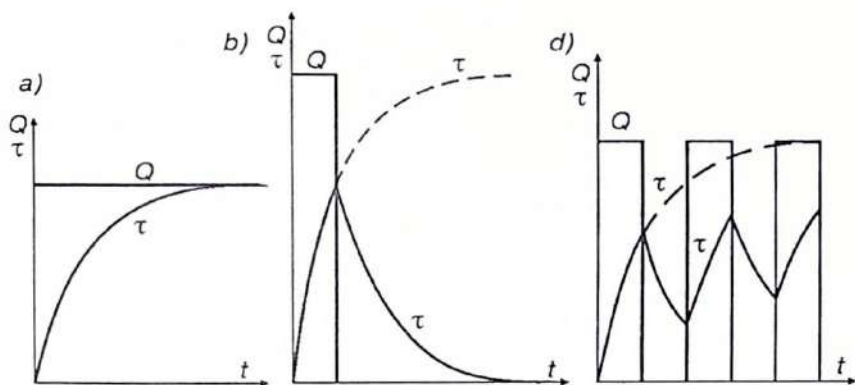
7.2- rasm. Elektr yuritmaning yuklama diagrammalari va dvigatel harorati o'zgarishining egri chiziqlari: a — davomli; b — qisqa; d — qaytar-qisqa ishlash rejimlarida.
