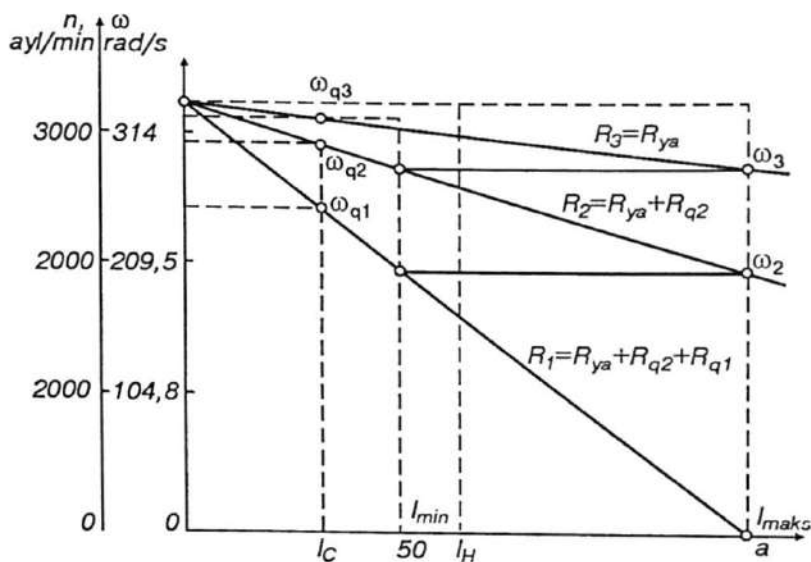
6.8- rasm. Ishga tushirish reostatlarini hisoblashga doir grafik.
