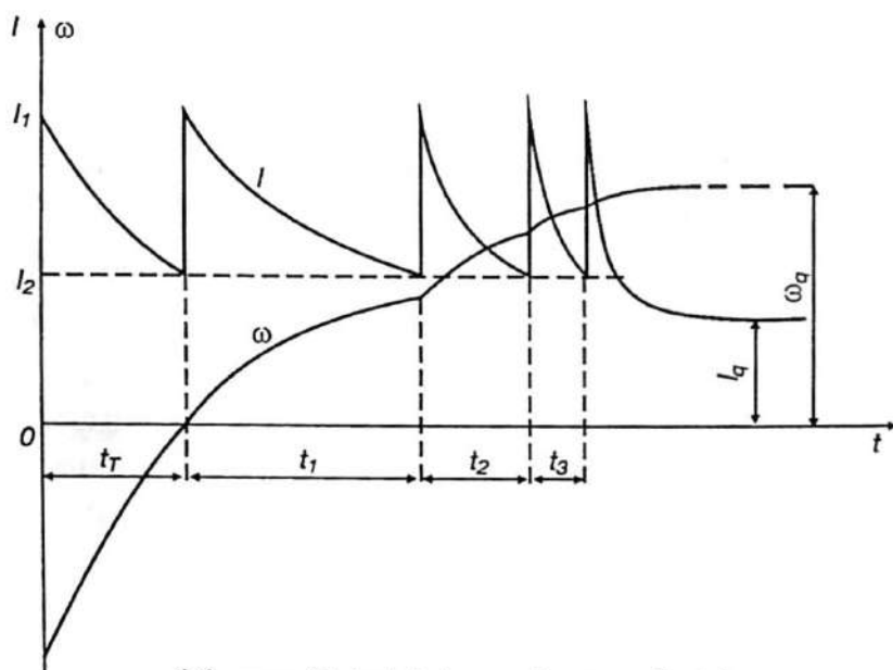
6.6- rasm. Dvigatelni reverslayotganda tok va tezlikning o'zgarish grafiqi.
