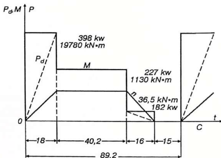
7.7- rasm. Shaxta ko'targichining yuklama diagrammasi.
