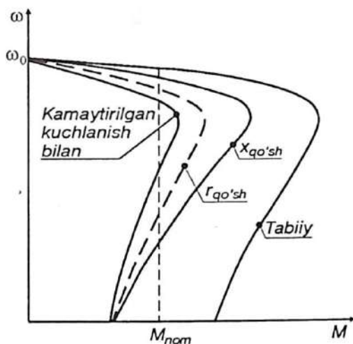
4.3- rasm. Asinxron dvigatelning nominal yoki pasaytirilgan kuchlanishdagi yoki statorga aktiv ( r_{qo'sh} ) va reaktiv ( X_{qo'sh} ) qo'shimcha qarshiliklar ulangan holatidagi mexanik tavsiflari.
