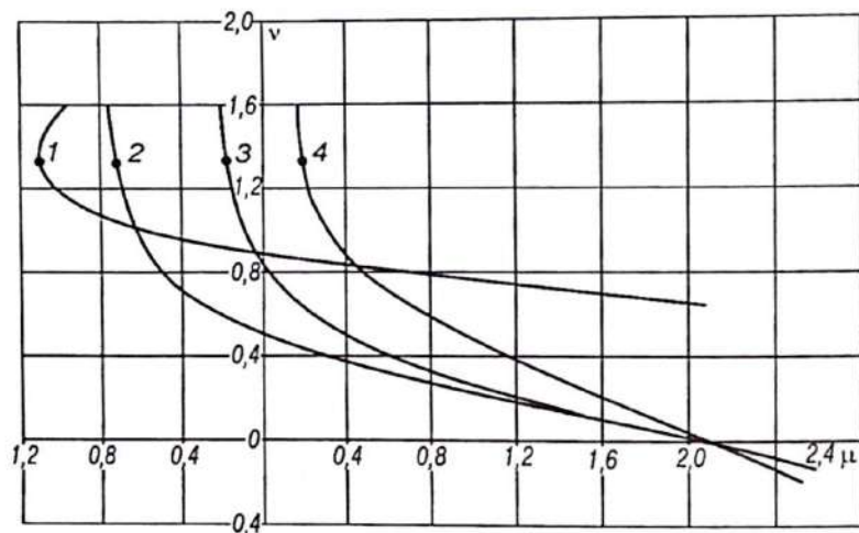
2.19- rasm. Dvigatelning 2.17- rasm, b dagi sxema bo'yicha qo'shimcha rezistorlar ulangan holatdagi mexanik tavsiflari.
