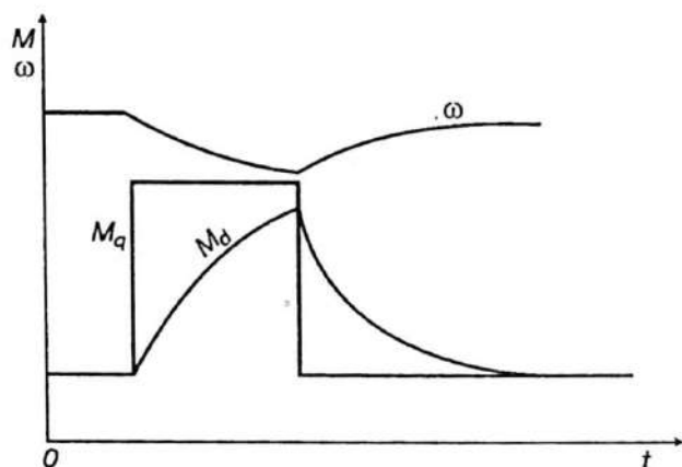
6.2- rasm. Yuklama berilganda moment va tezlikning o'zgarish grafiklari.
