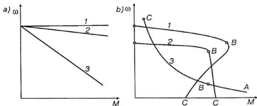
2.1- rasm. Dvigatelning mexanik tavsiflari: a — o'zgarmas; b — o'zgaruvchan qattqlikdagi. 1 — absolut qattiq; 2 — qattiq; 3 — yumshoq.
