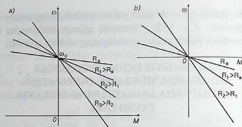
2.2-rasm. Mustaqil qo'zg'atishli o'zgaras tok dvigatelining kuchlanish o'zgaras bo'lgandagi va yakor zanjiridagi qarshiliklar o'zgargandagi (a), kuchlanish nol bo'lgandagi (b) mexanik tavsiflari.
