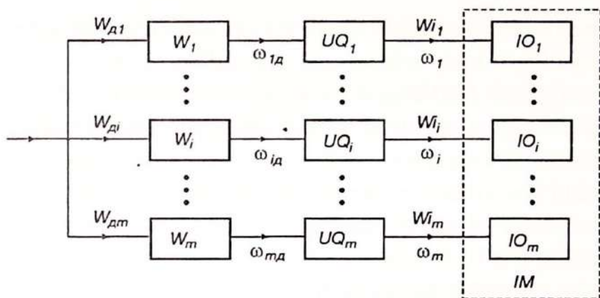
3- rasm. Individual elektr yuritmaning funksional sxemasi.
