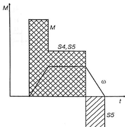
7.3- rasm. Nominal rejimlar S_4 va S_5 uchun yuklama diagrammalari.
