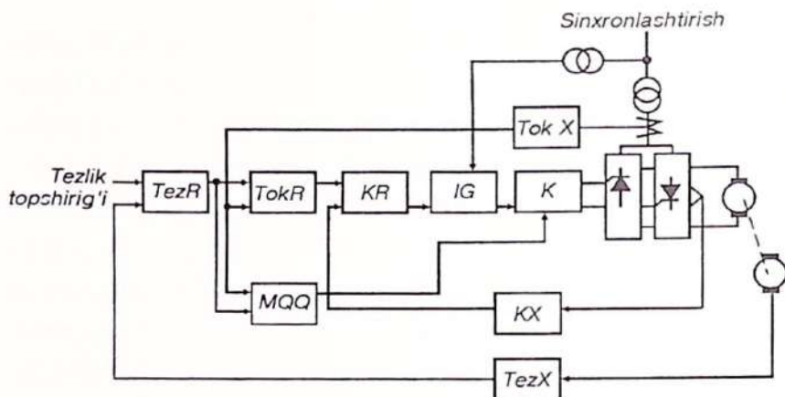
8.3- rasm. Elektr yuritmaning analog tizimi.
