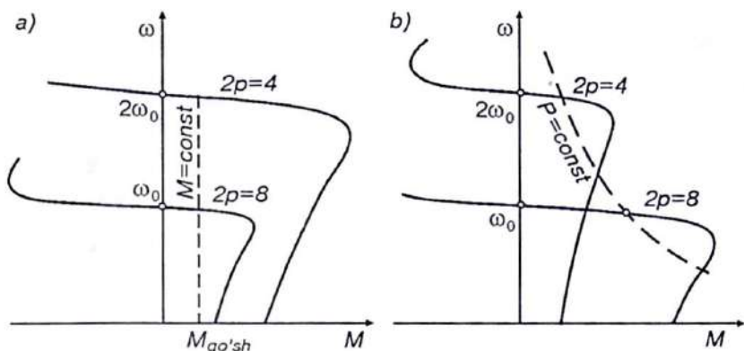
4.15- rasm. Ikki tezlikli dvigatelning mexanik tavsiflari: a — o'zgarmas moment rejimida; b — o'zgarmas quvvat rejimida.
