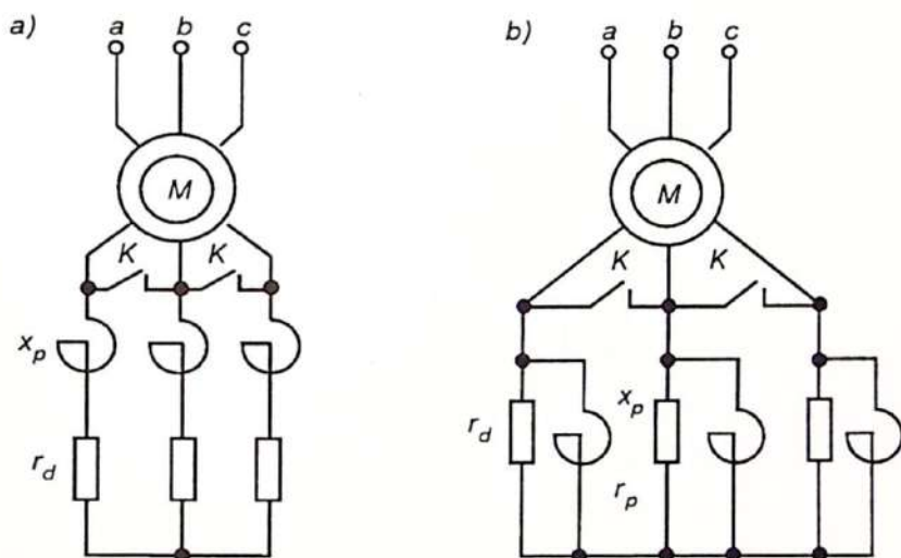
4.7- rasm. Rotor zanjiriga induktiv va aktiv qarshiliklarini ketma-ket ( a ) va parallel ( b ) ulanish sxemalari.
