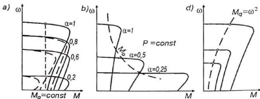
4.16- rasm. CHO-AD yuritma mexanik tavsiflari: a — o'zgarmas momentda; b — o'zgarmas quvvatda; d — ventilyatorli yuklamada.
