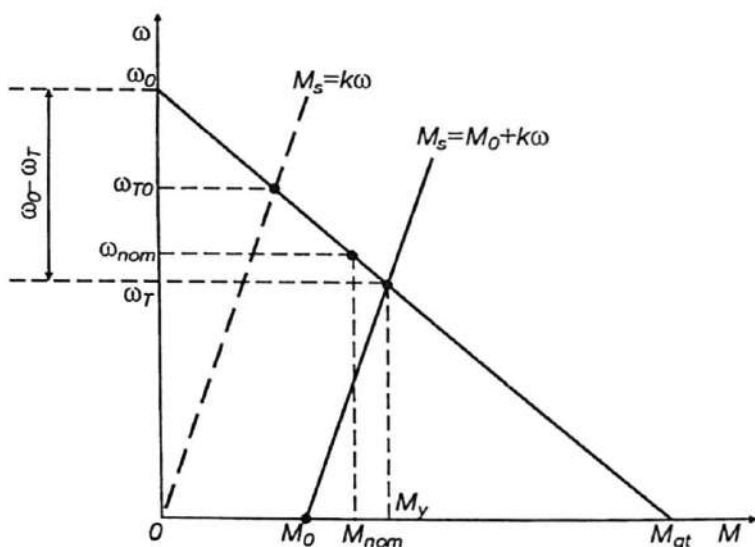
6.3- rasm. Statik momentlar turlicha bo'lgan holat uchun mexanik trassidagi ish nuqtalari.
