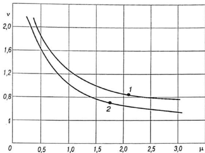
2.20- rasm. Dvigatelning 2.17- rasm, b dagi sxema bo'yicha qo'shimcha rezistorlar ulangan holatdagi mexanik tavsiflari.
