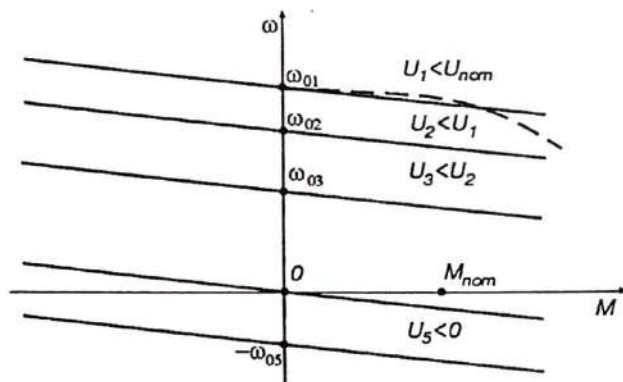
2.4- rasm. Dvigatel yakoriga berilayotgan kuchlanish o'zgartirilgandagi mexanik tavsiflar.
