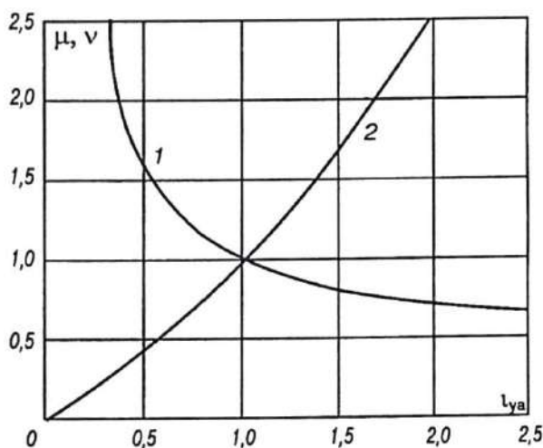
2.16- rasm. ДП rusumidagi ketma-ket qo'zg'atishli dvigatellarning universal tavsiflari: 1 — \nu = f(i_{ya}) 2 — \mu = f(i_{ya}) .
