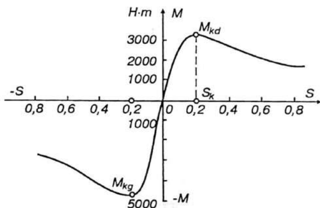
4.4- rasm. Faza rotorli asinxron dvigatelning dvigatel va generator rejimidagi tabiiy tavsiflari (6- misol).
