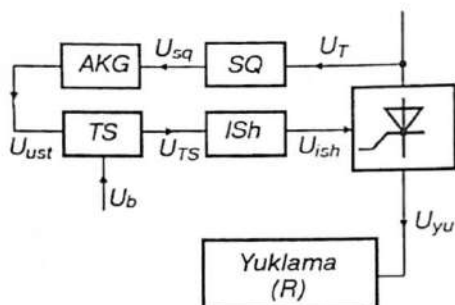
3.5- rasm. Boshqariluvchi to'g'rilagich sxemasi.
