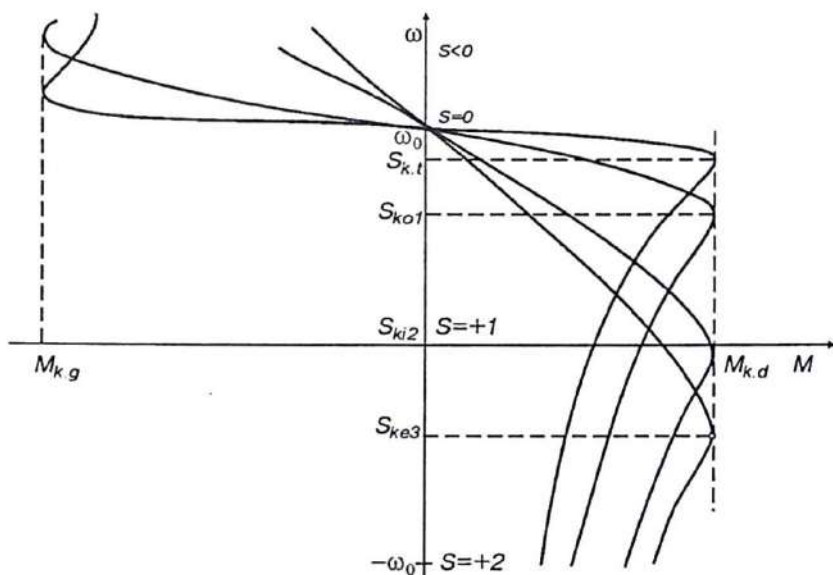
4.5- rasm. Faza rotorli asinxron dvigatelning mexanik tavsiflari.
