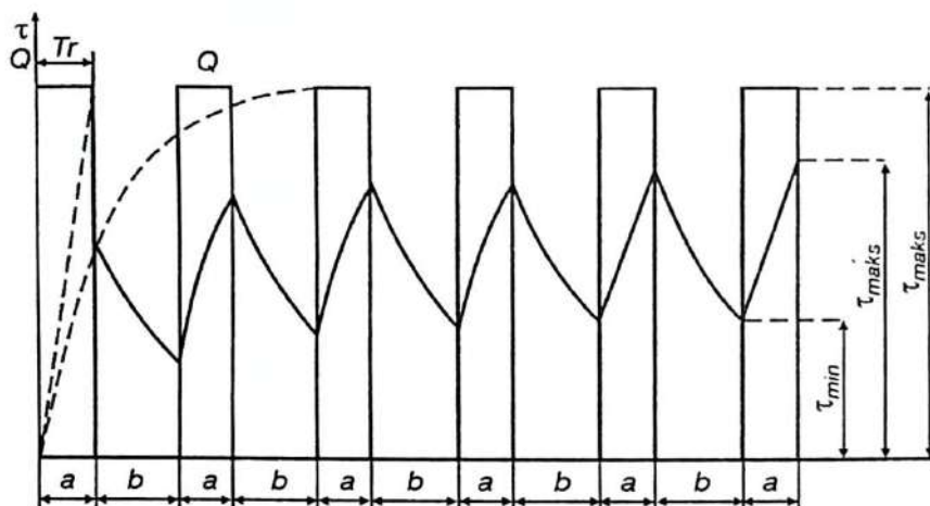
7.6- rasm. Dvigatelning qaytar-qisqa ish rejimining ideallashtirilgan grafigi.
