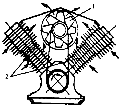
2.38-rasm. Havo bilan sovitish tizimining sxemasi: 1— parrak ; 2— silindr qobirg'alari
