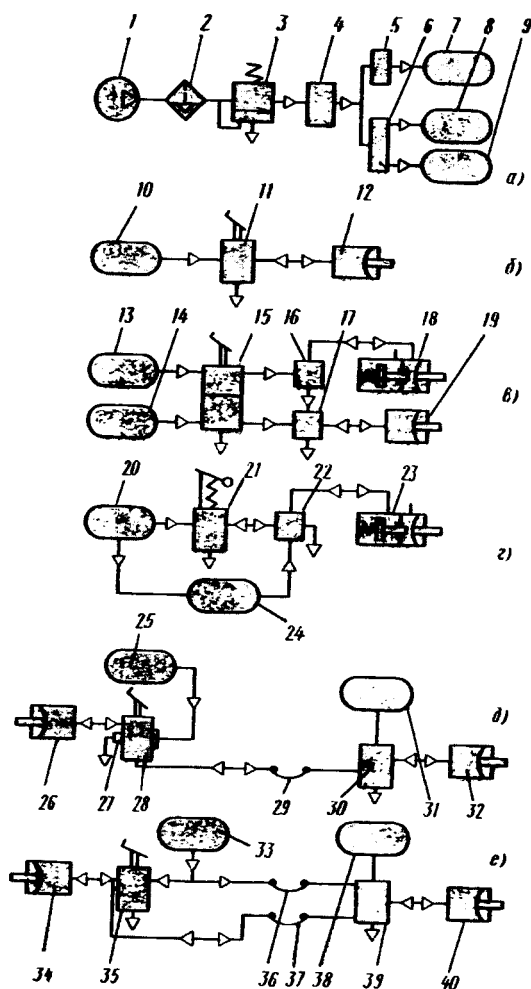
7.16-rasm. Pnevmatik tormoz yuritmalarining sxemalari:
