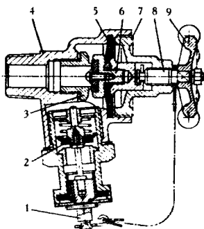
2.105-rasm. To'ldirish ventili:
