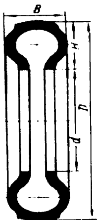
4.6-rasm. Shinaning o'lchamlari: d-to'g'ining diametri; V-shinaning eni; N-profilining balandligi; D-shinaning tashqi diametri
