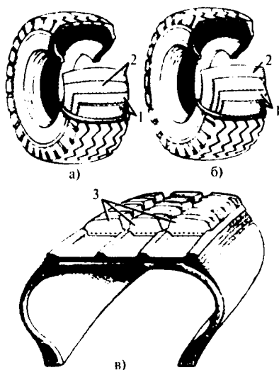
4.7-rasm. Shinaning turlari: a) diagonal kordli; b) R shinasi; d) RS shinasi. 1 - yostiqlik qatlami; 2 - karkas; 3 - protektorning olinuvchi xalqalari
