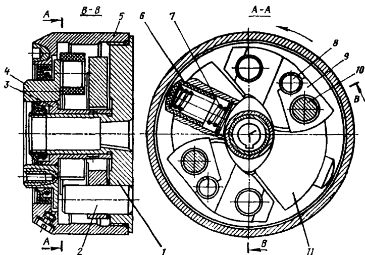
2.87-rasm. Yonilg'i purkashini ilgarilatish avtomatik muftasi: 1-yetaklanuvchi yarim mufta; 2-yuk o'qi; 3-yetakchi yarim mufta vtulkasi; 4-yetakchi yarim mufta; 5-mufta korpusi; 6-prujina stakani; 7-prujina; 8-yuk barmog'i; 9-yetakchi yarim mufta prostavkasi; 10-prostavka o'qi; 11- yuk 155
