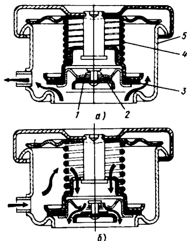
2.33-rasm. Radiator qopqog'i:
