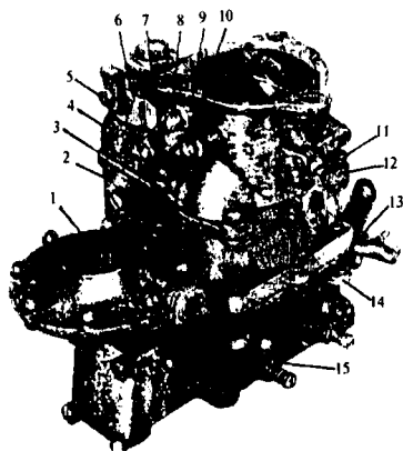
2.56-rasm. K-88A karburatori:
