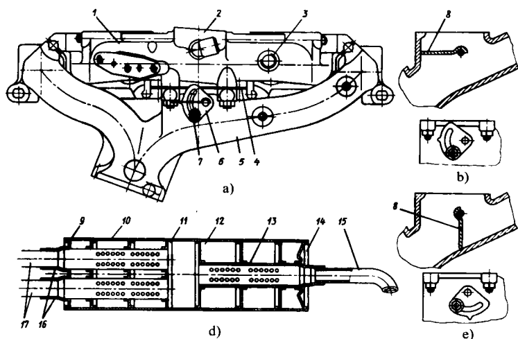
2.71-rasm. Kiritish va chiqarish tizimi hamda yonuvchi aralashmani isitish elementlari:
