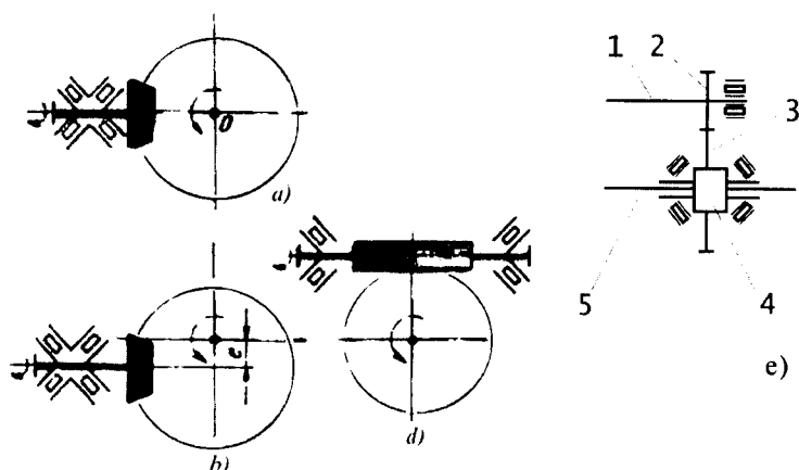
3.42-rasm. Yakka asosiy uzatmalar sxemasi:
