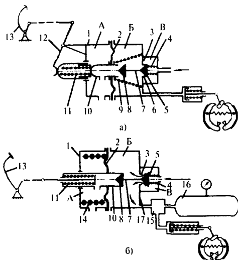
7.14-rasm. «Kuzatish mexanizmlari»ning sxemalari:
