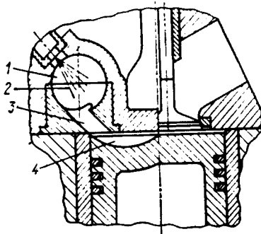
2.74-rasm. Uyurma turli ajratilgan yonish kamerasi:
