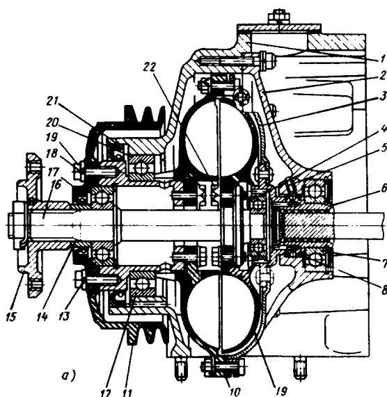
2.36-rasm. Hidravlik yuritmal ventilatorning gidromuftasi: a-konstruksiyasi; b-gidromuftaning termodatchikli uzgichi; 1-old qopqoq; 2-korpus; 3-kojux; 4, 7, 12, 13 va 20-sharchali podshipniklar; 5-moy keladigan nay; 6-yetakchi val; 8-zichlovchi xalqa; 9-yetaklanuvchi g'ildirak; 10-yetakchi g'ildirak; 11-shkiv; 14-tirak vtulka; 15-parrak gupchagi; 16-yetaklanuvchi val; 17 va 21 siquvchi salniklar; 18-qistirma; 19 va 22 - boltlar; 23-uzgich korpusi; 24-kran richagi; 25-termodatchik
