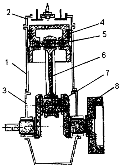
2.9-rasm. Bir silindrli porshenli ichki yonuv dvigateli: krivoship-shatunli mexanizm;
