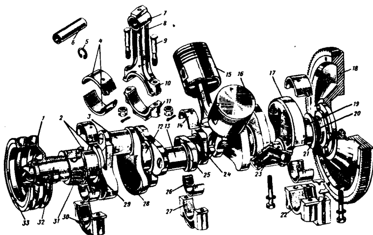
1-xropovik; 2-tirak xalqalar; 3 va 13 shatun bo'yinlar; 4, 14 va 26- vkladishlar; 5-prujinali xalqa; 6-porshen harmog'i; 7-shatunning yuqori kallagi; 8-shatun o'zagi; 9-boltlar; 10-shatunning pastki kallagi; 11-shatun qopqog'i; 12, 19, 24 va 29-o'zak bo'yinlar; 15 va 16 - porshenlar; 17 va 28- posongilar; 18-maxovik; 20-tirsakli valning orqa uchi; 21-moy qaytargich burti; 22, 27 va 30-o'zak podshipniklarning qopqog'i; 23-kir tutgich; 25 - jag'lar; 31-tishli g'ildirak; 32-tirsakli valning old uchi; 33-shkiv
