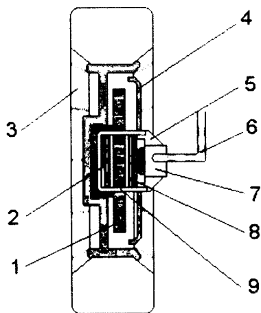
7.7-rasm. «Neksiya» avtomobilining diskli tormoz mexanizmi:
