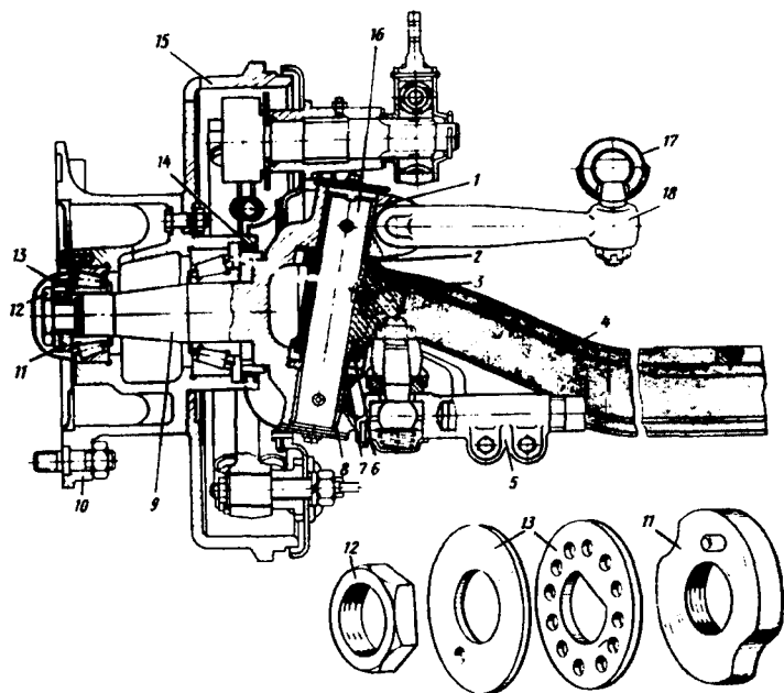
4.11 - rasm. ZIL-130 yuk avtomobilining boshqariluvchi ko'prigi: 1,8-bronza vtulkalar; 2-rostagich tiqinlar; 3-ponasimon bolt; 4-ko'prik to'sini; 5-rulning ko'ndalang tortqisi; 6,7-tayanch podshipnik shaybalari; 9-burish sapfasi; 10-g'ildirak gupchagi; 11-rostlovchi gayka; 12-kontrgayka; 13-qulf shayba; 14-moy tutgich; 15-tormoz barabani; 16-shkvoren; 17-rulning bo'ylama tortqisi; 18-buruvchi richag
