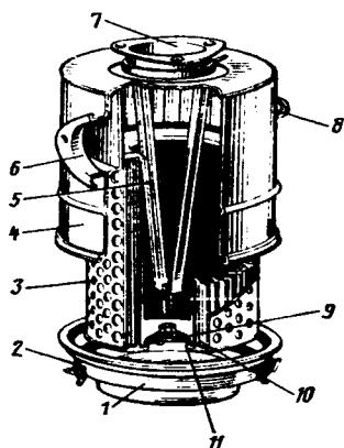
2.90-rasm. Havo filtri: 1-filtrlovchi element tutqichi; 2-qotirish ilgagi; 3,11-inersion panjara ning tashqi va ichki kojuxlari; 4-korpus; 5-markaziy kronshteyn; 6,7-kiritish va chiqarish patrubkalari; 8-ejeksion chang chiqarish patrubkasi; 9-filtrlovchi elementni qotirish gaykasi; 10-filtrlovchi karton
