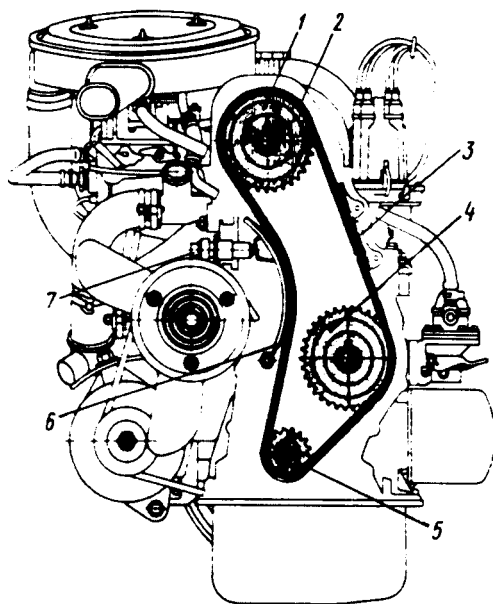
2.21-rasm. VAZ-21011 avtomobil dvigateli taqsimlash valining zanjirli yuritmasi: 1-etaklanuvchi yulduzcha; 2-ikki qatorli zanjir; 3-zanjirni tinchlantirish tuzilmasi; 4-moy flsasining yulduzchasi; 5-etakchi yulduzcha; 6-bashmak; 7-taranglash tuzilmasi
