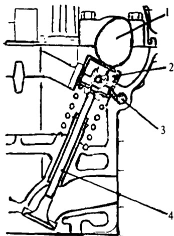
2.23-rasm. Neksiya avtomobili S2 rusumli dvigatelining gaz taqsimlash mexanizmda gidrokompensatorning joylashtirish sxemasi: 1-taqsimlash valining mushtchasi; 2-gidrokompensator; 3-moy kanali; 4-klapan
