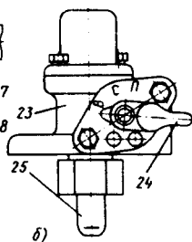
2.36-rasm. Hidravlik yuritmal ventilatorning gidromuftasi: a-konstruksiyasi; b-gidromuftaning termodatchikli uzgichi; 1-old qopqoq; 2-korpus; 3-kojux; 4, 7, 12, 13 va 20-sharchali podshipniklar; 5-moy keladigan nay; 6-yetakchi val; 8-zichlovchi xalqa; 9-yetaklanuvchi g'ildirak; 10-yetakchi g'ildirak; 11-shkiv; 14-tirak vtulka; 15-parrak gupchagi; 16-yetaklanuvchi val; 17 va 21 siquvchi salniklar; 18-qistirma; 19 va 22 - boltlar; 23-uzgich korpusi; 24-kran richagi; 25-termodatchik
