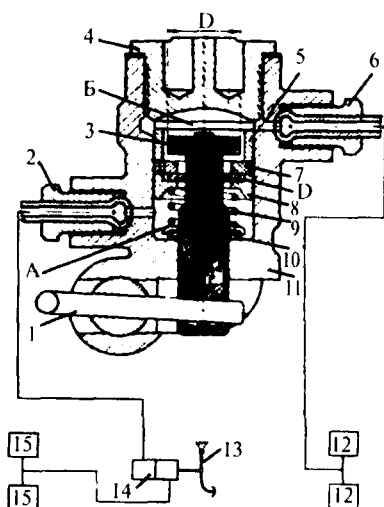
7.12-rasm. Tormoz kuchlarini rostlagichi sxemasi:
