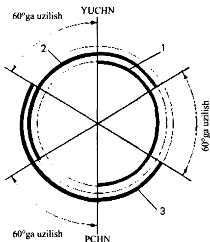
2.5-rasm. To'rt taktli uch silindrli ish tartibi 1-3-2 bo'lgan dvigatelda ish yo'li taktlarini o'tishida o'zaro uzilishni tasvirlovchi diagramma:
