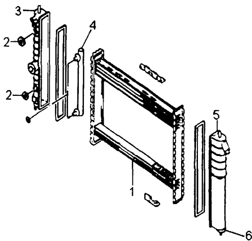
2.32-rasm. Neksiya avtomobili radiatorining detallari:
