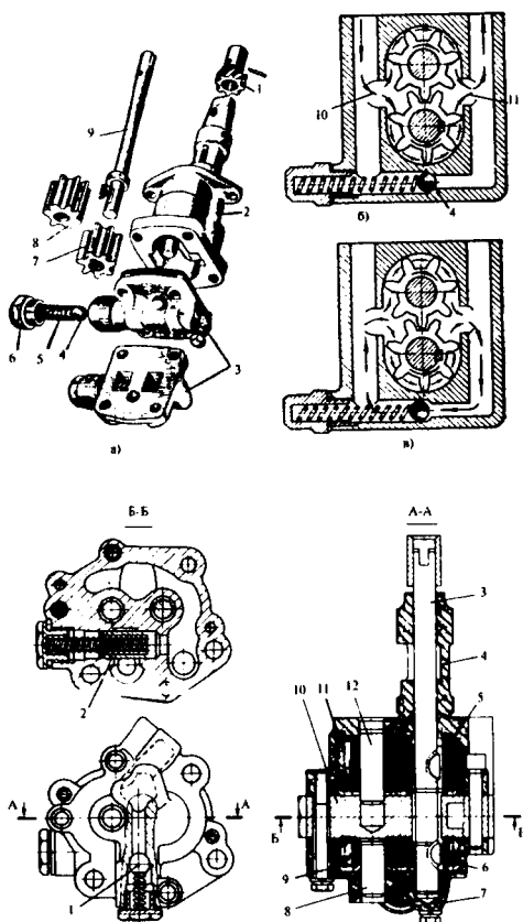
2.41-rasm. Ikki seksiyali shesternalari tashqi ilashgan moy nasosining sxemasi:
