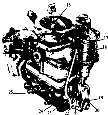
2.56-rasm. K-88A karburatori:
