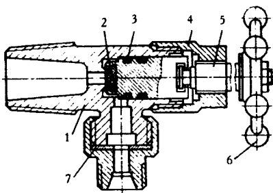
2.106-rasm Sarflash ventili:
