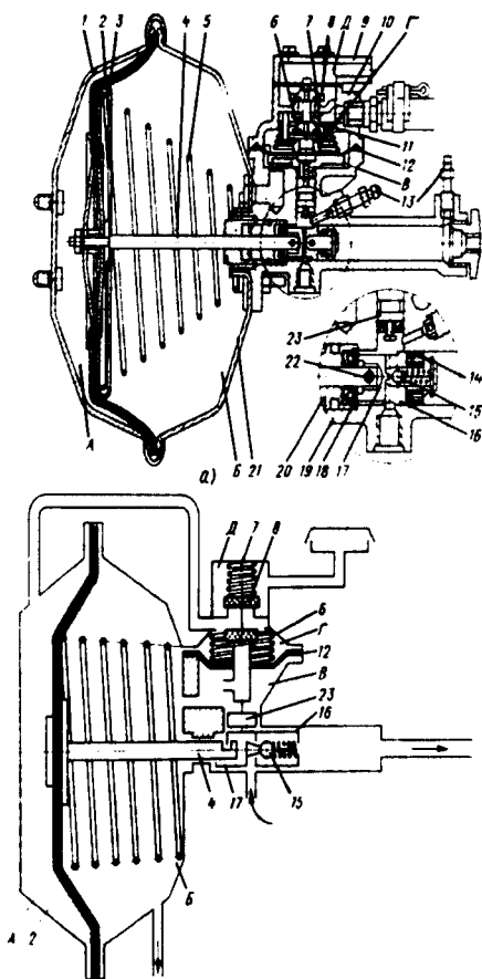
7.11-rasm. Hidrovakuum kuchaytirgichi sxemasi: a-bo'ylama qirg'iq; b-sxema; 1-vakuum kamerasi; 2-membrana; 3-tarelka; 4-turtkich; 5va 11-membrana prujinalari; 6-vakuum klapani; 7-klapanlar prujinasi; 8-atmosfera klapani; 9-qopqoq; 10-«kuzatuv» mexanizmining korpusi; 12-«kuzatuv» mexanizmining membranasi; 13-o'tkazish klapanlari; 14-manjeta; 15-sharikli klapan; 16-porshen; 17-klapan turtkichi; 18-tayanch shaybasi; 19-silindr; 20-zichlovchi korpus; 21-gayka; 22-shtift; 23-plunjer; A-D-hajmlar
