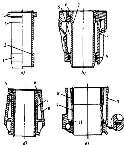
2.11-rasm. Silindrlar gilzasi:
