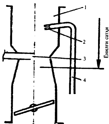
2.53-rasm. Oddiy ekonostat
