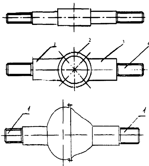
4.10-rasm. Bo'laklarga ajraladigan to'sin: 1 - to'sin bo'laklarining chuloklari
