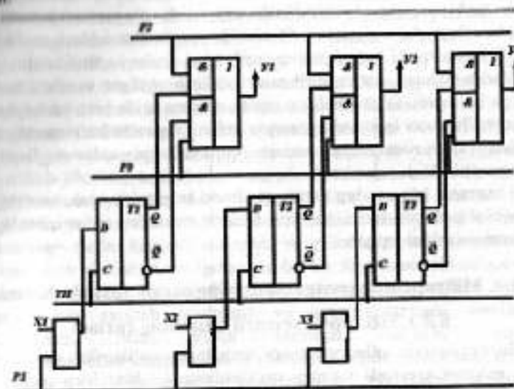
8.3-rasm. Sonning to'g'ri kodni teskarisiga aylantiruvchi va ma'lumotni saqlovchi registr sxemasi.
