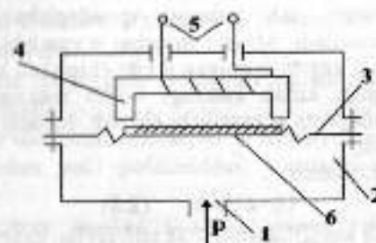
2.7-rasm. Induktiv manometruing sxemasi.
