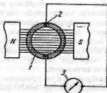
2.35-rasm. Induksion sarf o'lchagich sxemasi.
