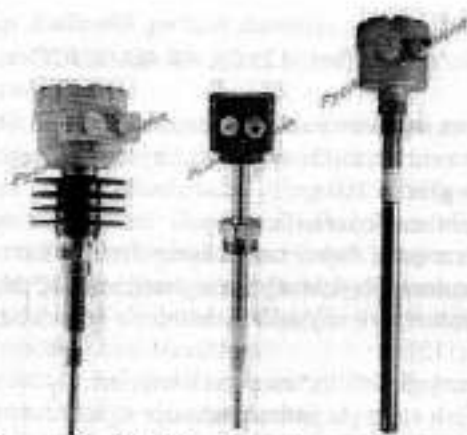
2.26-rasm. Sath sig'im signalizatorlar ko'rinishi.
