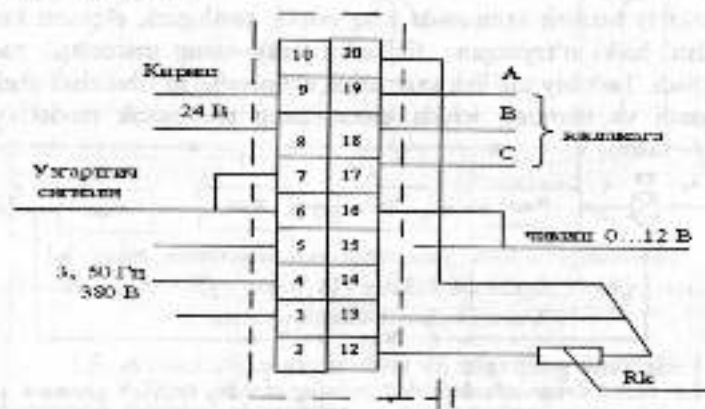
1.8-rasm. Avtomatikaning montaj sxemasi.
