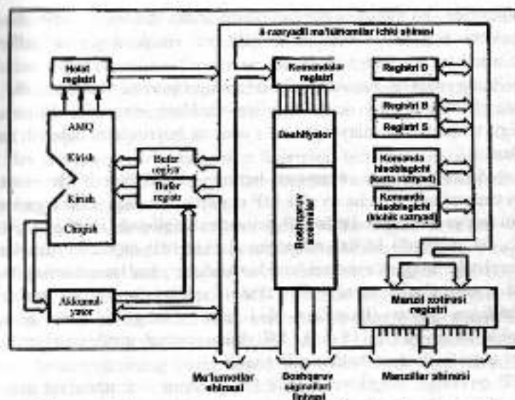
8.5 - rasn. 8-razryadli mikroprotsessorning struktura sxemasi.
