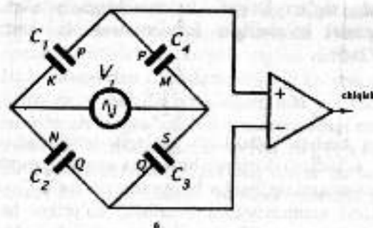
2.33-rasm. Sig'im ko'prikl ko'rinishidagi datchiklarning ekvivalent sxemasi.
