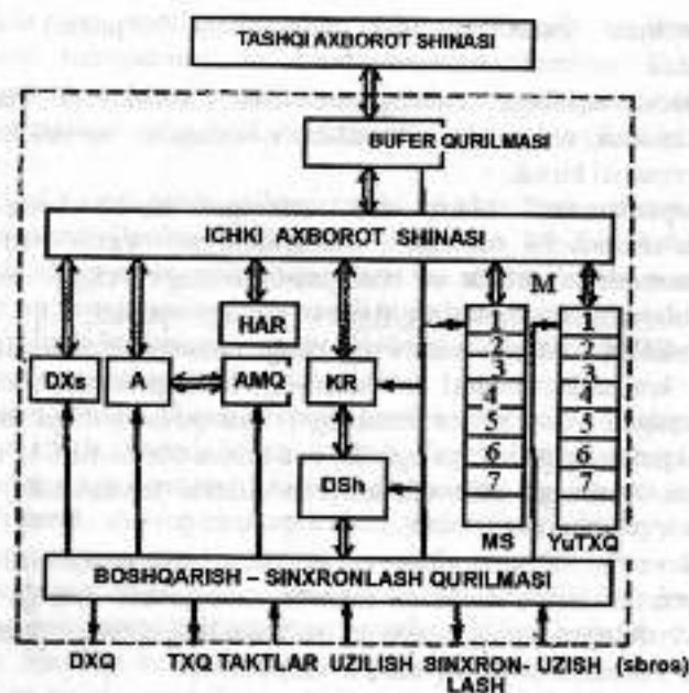
8.4-rasm. Mikroprotessorning soddalashtirilgan struktura sxemasi.
