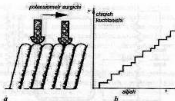
2.3-rasm. Simli potensiometrlarning kamchiliklari: a) potensiometrni polzunogi bir vaqtini o'zida ikkita o'ramasini ulashi mumkin; b) kuchlanishni notekisligi.
