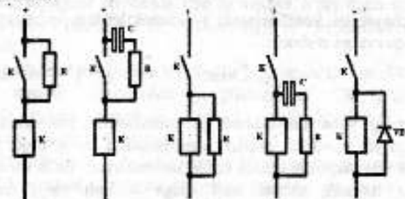
3.1-rasm. Rele kontaktlarini (a, b) va cho'lg'amlarini (v, g, d) uchqundan saqlash uchun shuntlash.
