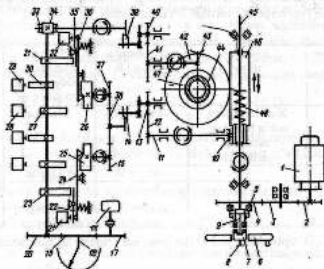
5.2- rasm. Unifikatsiyalangan elektr yuritmalar surgichlarining kinematik sxemasi.
