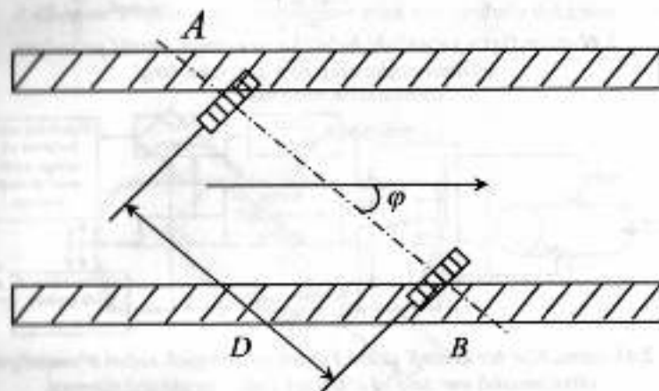
2.39-rasm. Suv quvurining ikki tomoniga qarama-qarshi joylashtirilgan ultratovush generatori.
