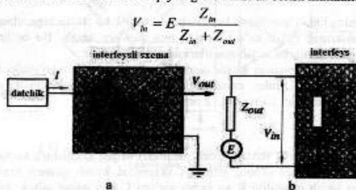
2.30-rasm, a – interfeys sxemasini kompleks kirish parametri; b – kuchlanish ko'rinishidagi chiqish signalga ega bo'lgan datchikni ekvivalent sxemasi.
