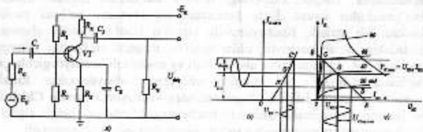
4.1-rasm. Umumiy emmitterli ( UE ) kuchaytirish kaskadining sxemasi hamda kirish va chiqish xarakteristikalarini.
