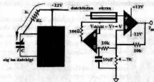
2.32-rasm. a) platada paydo bo'ladigan oqim toki u interfeysni kirish zanjirlarida, tavsifnomalarni o'zgarishiga olib keladi; b) kirish zanjirlarini aktiv ekranlash.
