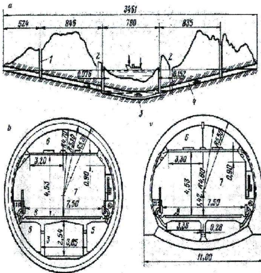
9.10 -rasm. Suvosti tunnelli:
