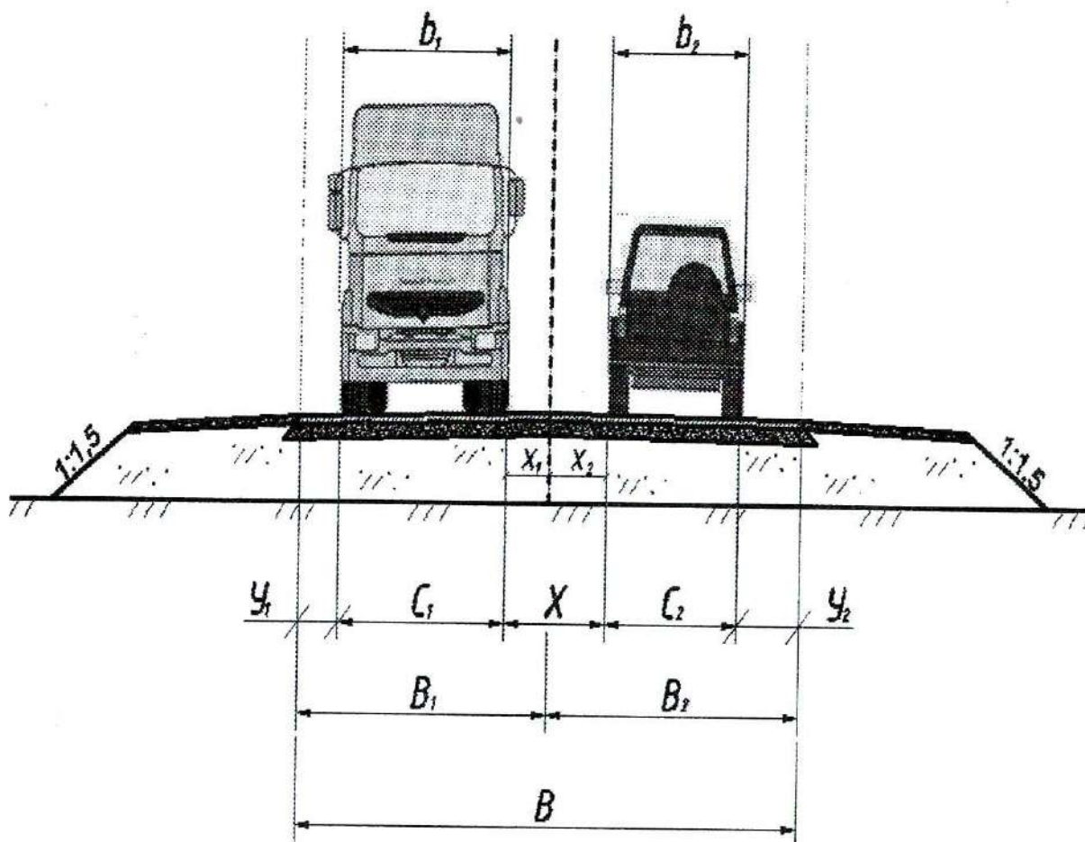
8.10-rasm. Yo'l qatnov qismini aniqlash chizmasi
