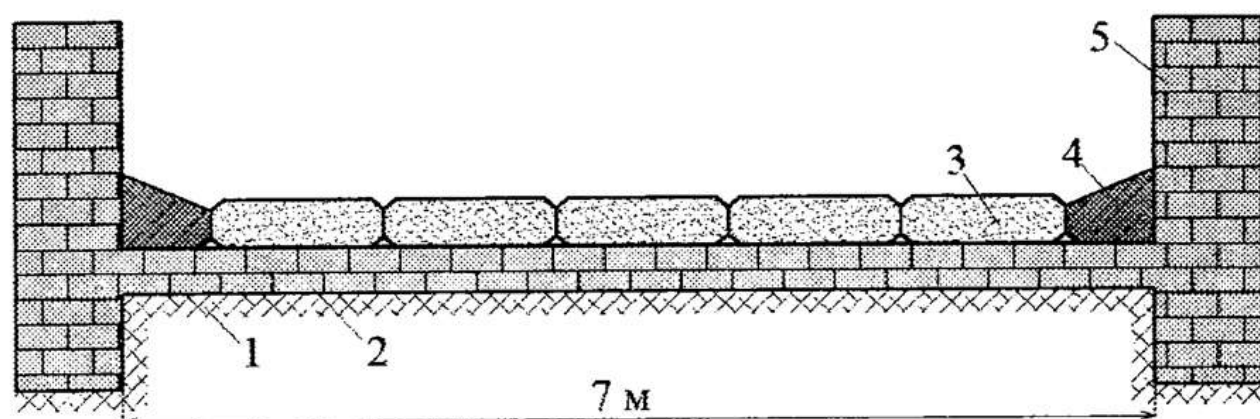
1.1-rasm. Vavilondagi Marduk xudosi qasriga boradigan yo'lning ko'ndalang kesimi:
