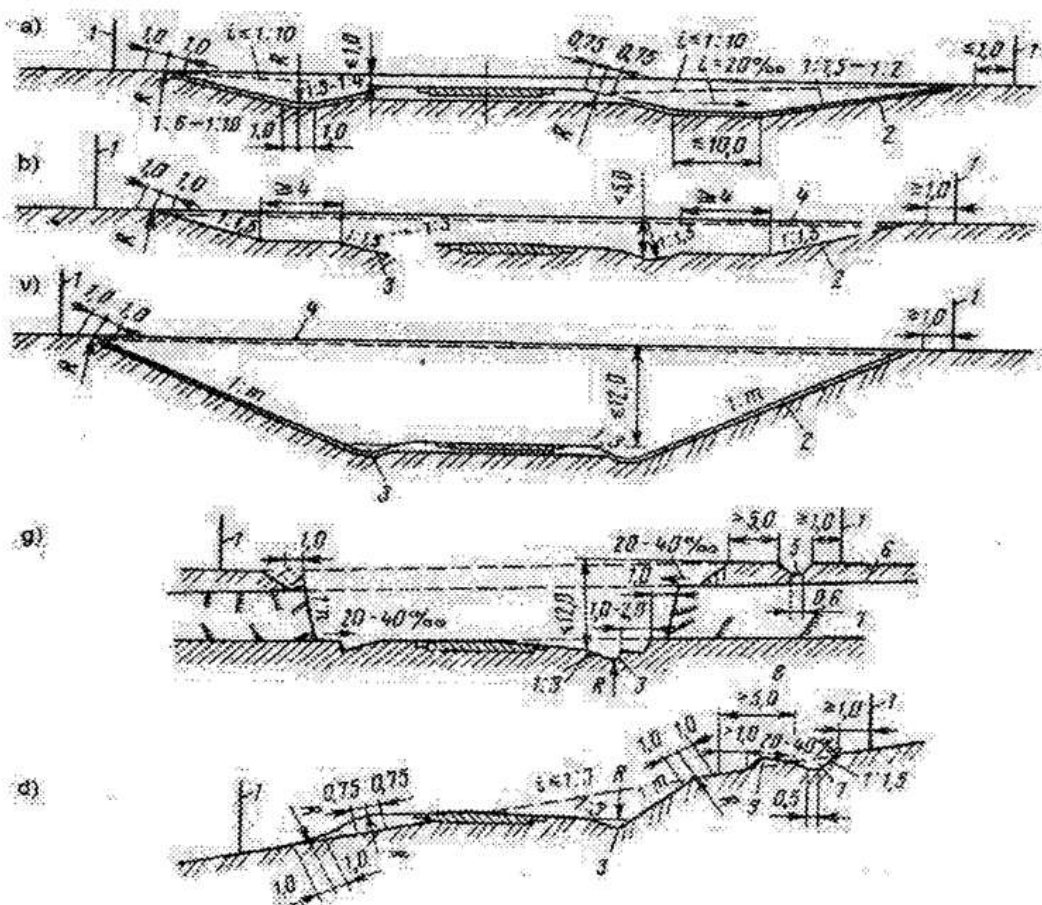
8.12-rasm. O'ymalardagi yo'l poyining ko'ndalang kesimi:
