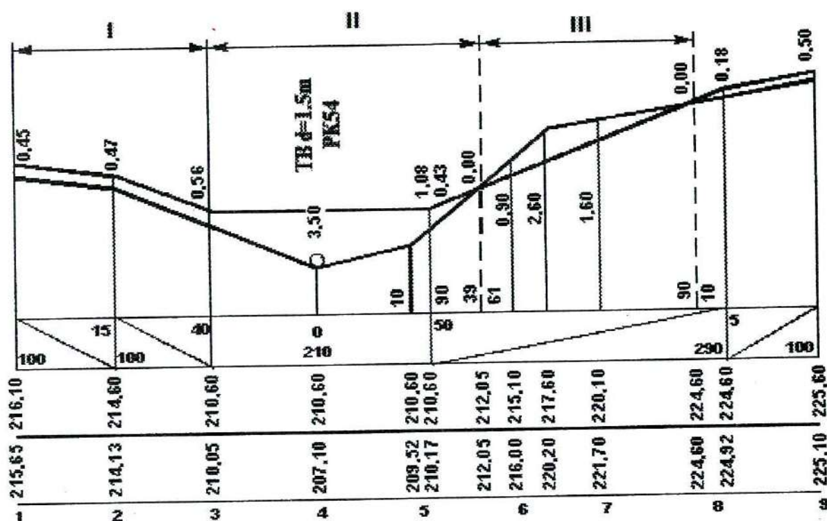
8.2-rasm. Bo'ylama kesimda yo'lning joylashishi:
