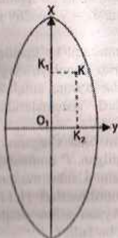
1.10-rasm. Gauss-Kryuger proyeksiyasida atohida zonaning tekislikda tasvirlanishi
