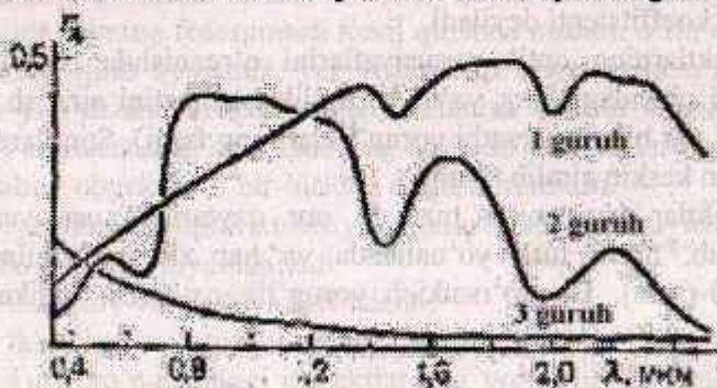
4.4-rasm. Tabiiy obyektlarning spektr yorug'lik koeffitsienti
