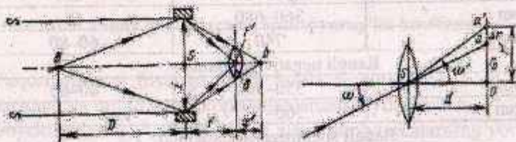
4.5-rasm. Ko'rish maydoni va distorsiya vujudga kelishi
