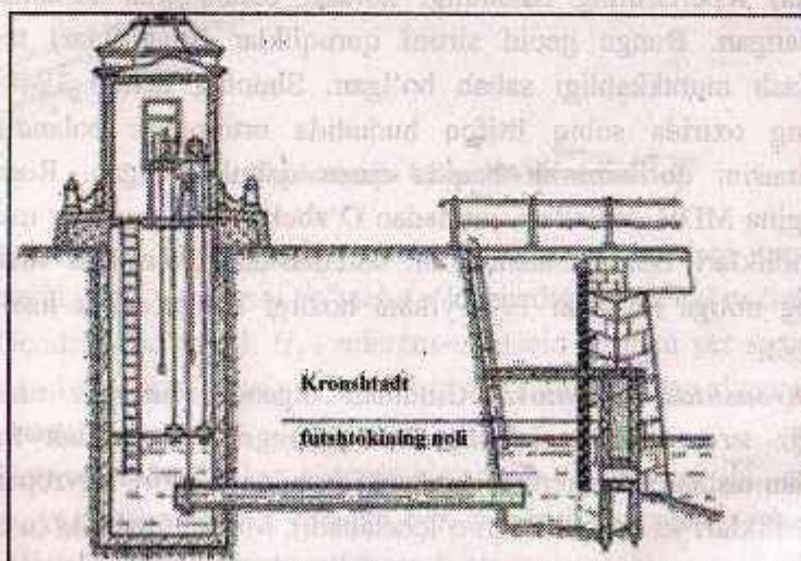
1.14-rasm. Kronshtadt futshtokining konstruktiv tuzilishi
