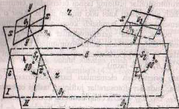
4.21-rasm. Bosh bazis tekisliklari
