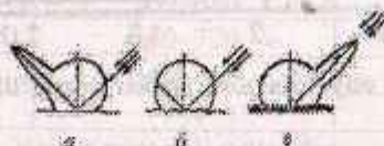
4.3-rasm. Turli yuzalardan qaytgan nurlanishning indikatrasi: a- silliq yuzadan; b- barcha yo'nalishlarda nurlanishning yorug'ligi bir xil bo'lgan tekisliklar; v- o'yib ishlangan yuzalar
