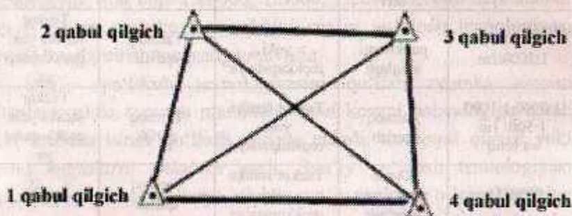
2.2-rasm. 4ta punktda bajariladigan seanslardan 1-2, 2-3, 3-4 chiziqlarni erkin aniqlash sxemasi:
