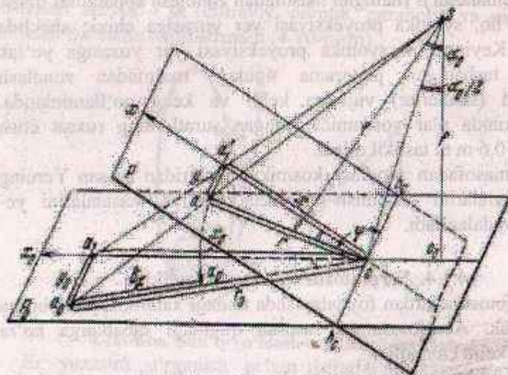
4.11-rasm. Gorizontaal va og'ish burchagi bo'lgan aerofotosurat orqali chiziqli xatoliklarni aniqlash
