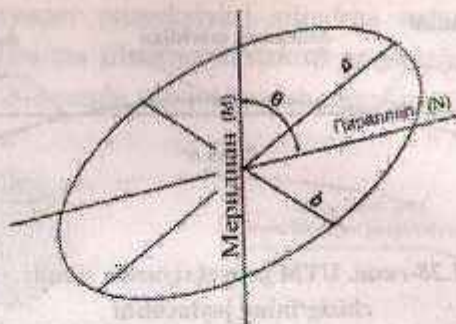
1.29-rasm. Xatoliklar ellipst va uning elementlari
