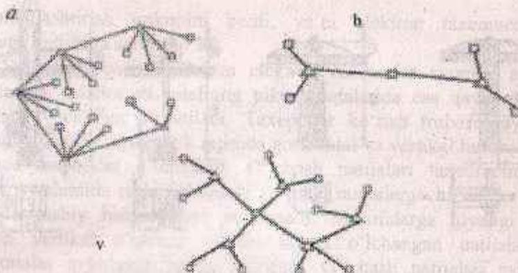
2.3-rasm. Osmat nuqtalar usulida syomka asosini rivojlantirish sxemalari:
