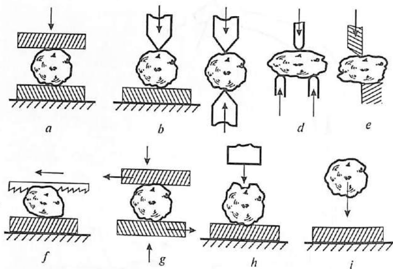
66-rasm. Maydalash usullari sxemalari:
