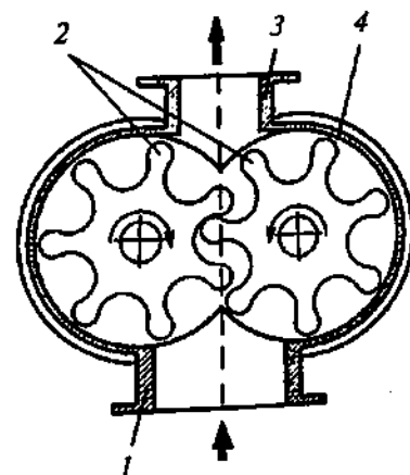
60- rasm. Shesternali nasos sxemasi:
