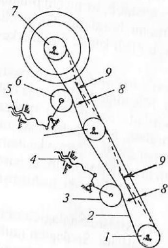
26-rasm. Ventilatorga harakat uzatuvchi tasmani taranglovchi moslama;
