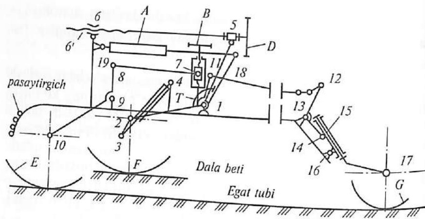
3-rasm. Tirkalma plug mexanizmlarining sxemasi.
