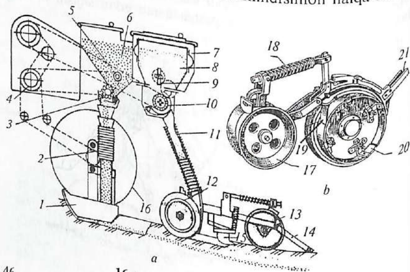
16-rasm. Sabzavot seyalkasi.
