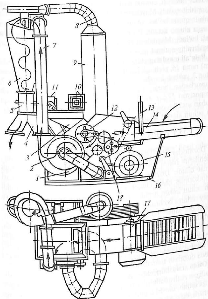
67-rasm. КДУ-2,0 markali universal maydalagich: 1—maydalash apparati; 2—ventilator; 3—yuklash kovshi; 4—bo'shatish shlangi; 5—shluzli zatvor; 6—siklon; 7—oziqa quvuri; 8—havo quvuri; 9—filtrlash shlangi; 10—ampermetr-indikator; 11—chervakli reduktor; 12—pichoqli baraban; 13—ishga tushirish richagi; 14—ta'minlash tarnsportyori; 15—elektr dvigatel; 16—rama; 17—presslash transportyori; 18—reduktor.
