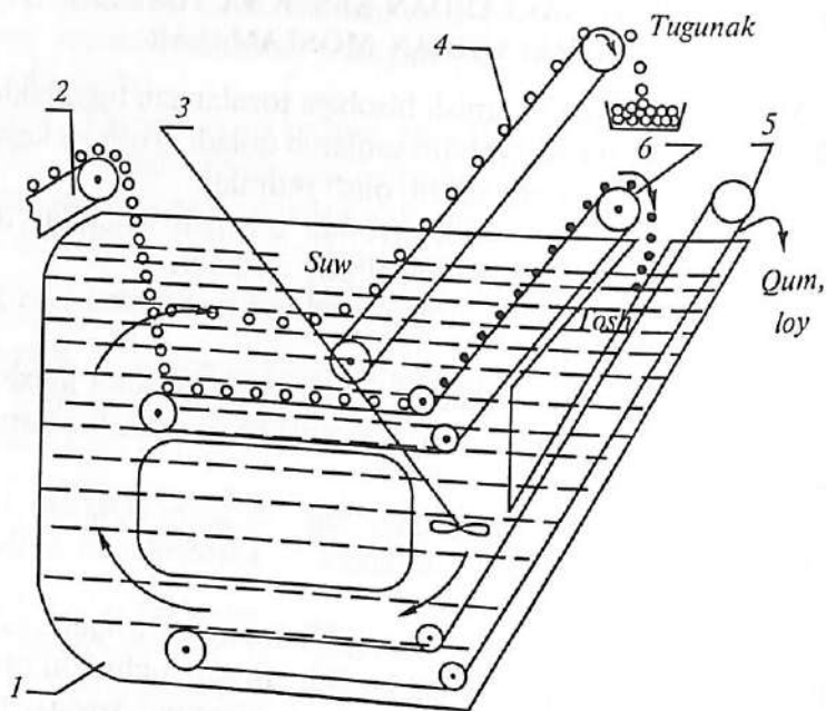
51-rasm. Kartoshka tugunaklarini zichligi bo'yicha suspenziyada tosh-kesaklarni ajratish sxemasi.
