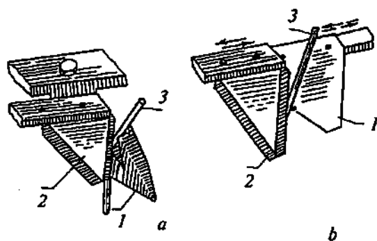
32- rasm. Tirakli o'rish apparati.
