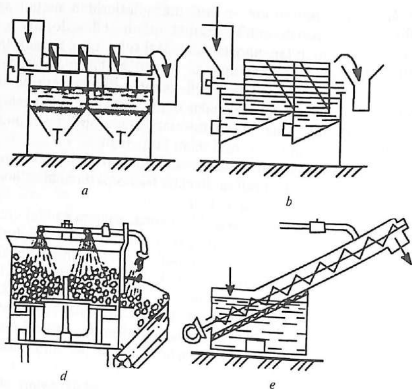
64-rasm. Ildizmeva yuvgichlar sxemasi:
