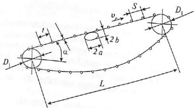
50-rasm. Chiviqli elevator o'lchamlari.
