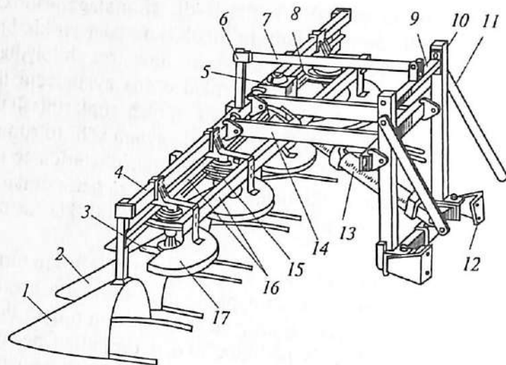
18- rasm. QXT- 4B g'oz uchlarini chilpish moslamasi.
