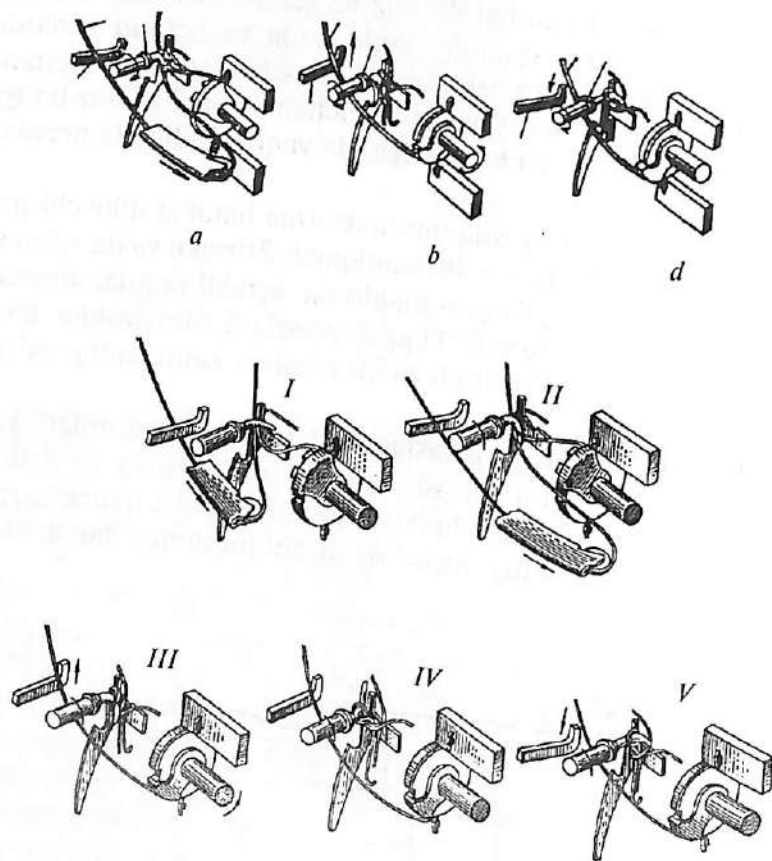
41-rasm. Sim bilan bog'lashda tuguncha hosil qilish.
