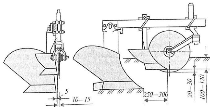
4-rasm. Plug ishchi qismining tuzilishi.
