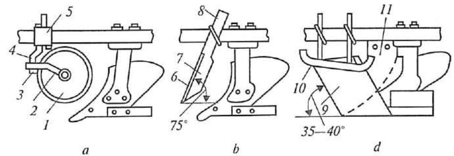
8-rasm. Plug pichoqlari.
