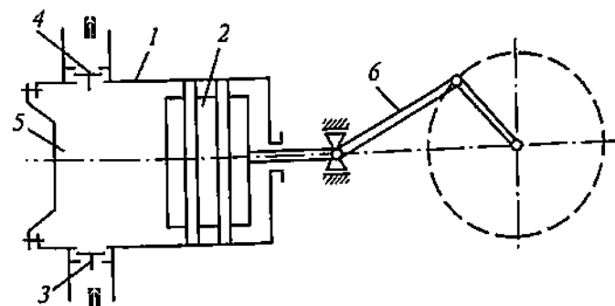
59- rasm. Porshenli nasos sxemasi:
