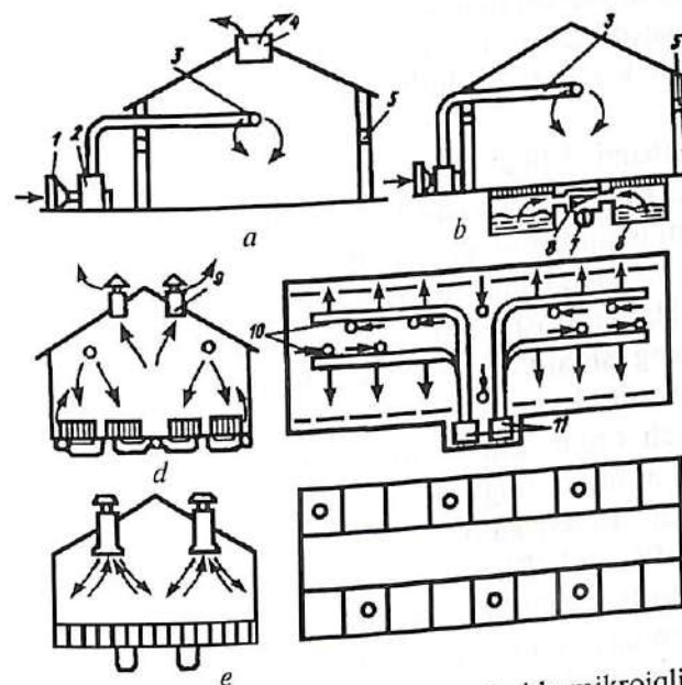
56-rasm. Turli chorvachilik inshootlarida mikroiqlimni tashkil etish tizimlari:
