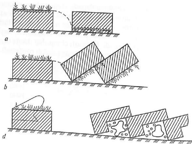
6- rasm. Tuproqqa asosiy ishlov berish sxemasi.
