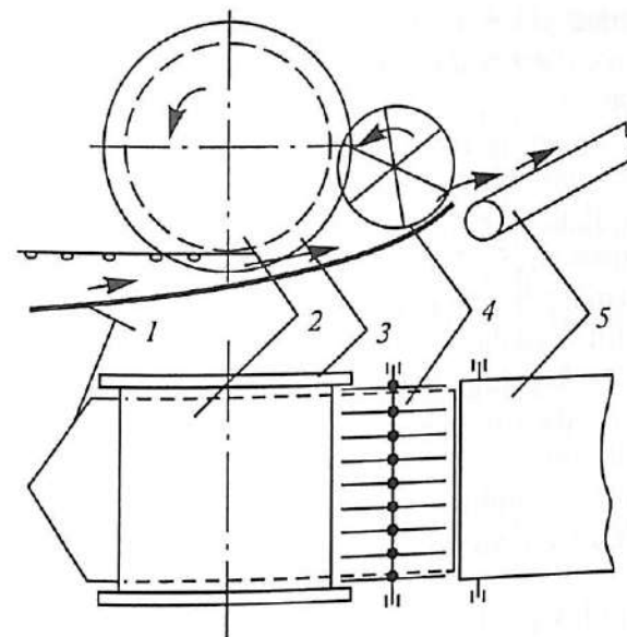
48-rasm. 1—passiv lemex; 2—erkin aylantiruvchi baraban; 3—disklar; 4—uzatuvchi biter; 5—transportyor.
