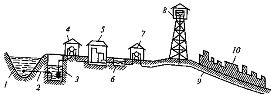
57-rasm. Yer yuzidagi (ochiq) suv manbayidan suv bilan ta'minlash sxemasi:
