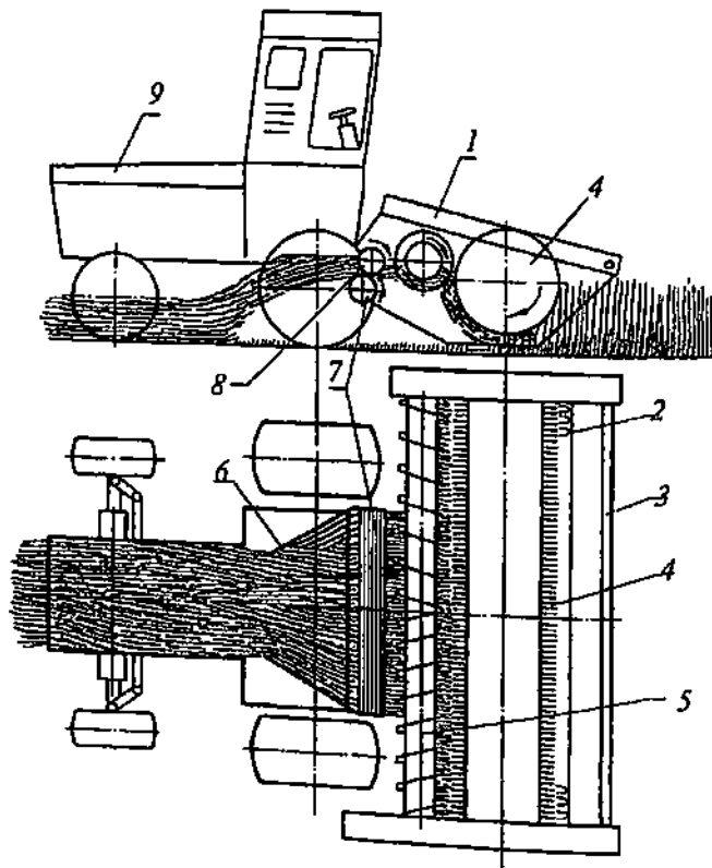
39-rasm. Pichano'rgich-ezgi ning texnologik jarayoni sxemasi.
