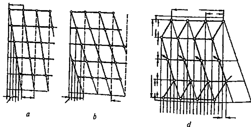
11-rasm. Borona tishlarini joylashtirish.
