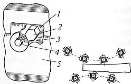
23- rasm. 1—disk; 2—rostlovchi vint; 3—shayba; 4—bolt; 5—oldingi qopqoq
