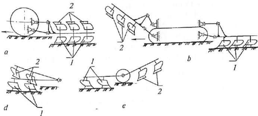
1- rasm. Tekis haydash pluglarining sxemasi.
