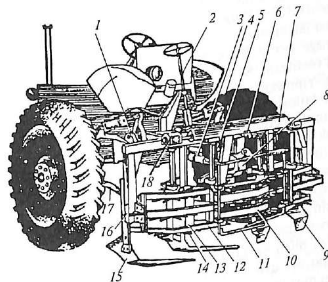
30-rasm. KB-3,6 markali g'o'zapoyani yulib bir qatarga uzluksiz tashlab ketadigan mashina:
