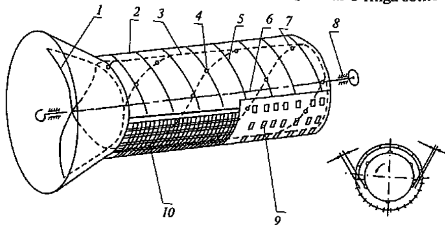
35- rasm. Aksial-rotorli yanchish apparatining sxemasi.
