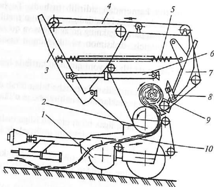
42- rasm. Rulonlab presslagich sxemasi.
