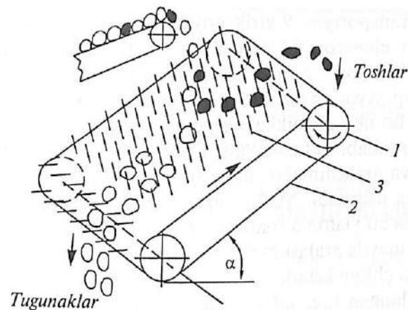
52-rasm. Qoziqchali transportyor yordamida toshlardan kartoshkani ajratish sxemasi:
