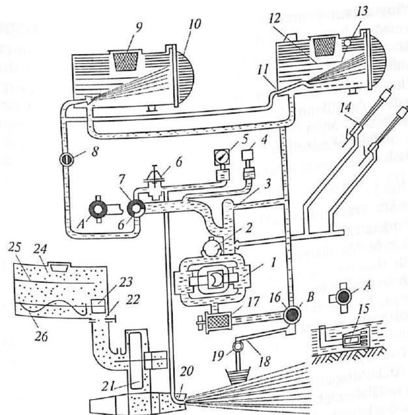
20-rasm. Paxtachilikka moslashtirilgan purkagichning texnologik sxemasi.
