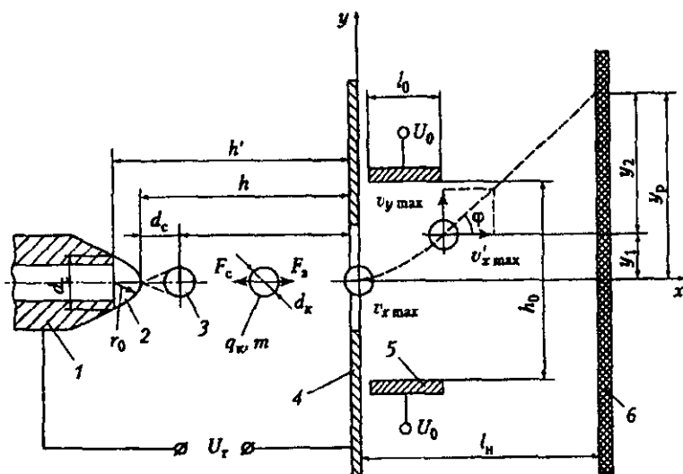
8.26-rasm. Uzlusiz oqimli bosmada zaryadlangan tomchining siljishini hisoblash sxemasi:
