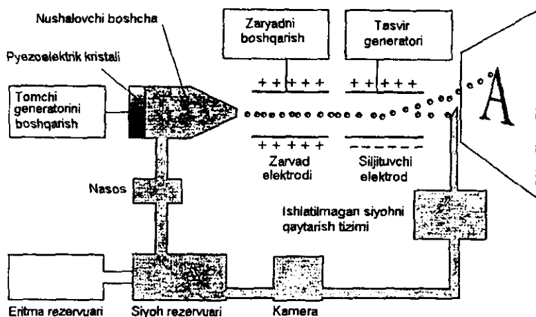
8.24-rasm. Uzlaksiz oqimli bosma printerining sxemasi.
