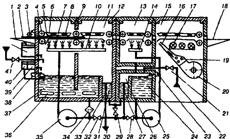
6.12-rasm. Aralash tashish qurilmasi boʻlgan FBQga ishlov berish oqim tizimi.
