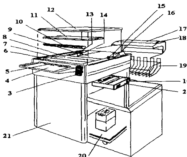
4.3-rasm. Multiline protsessorining asosiy qismlari.
