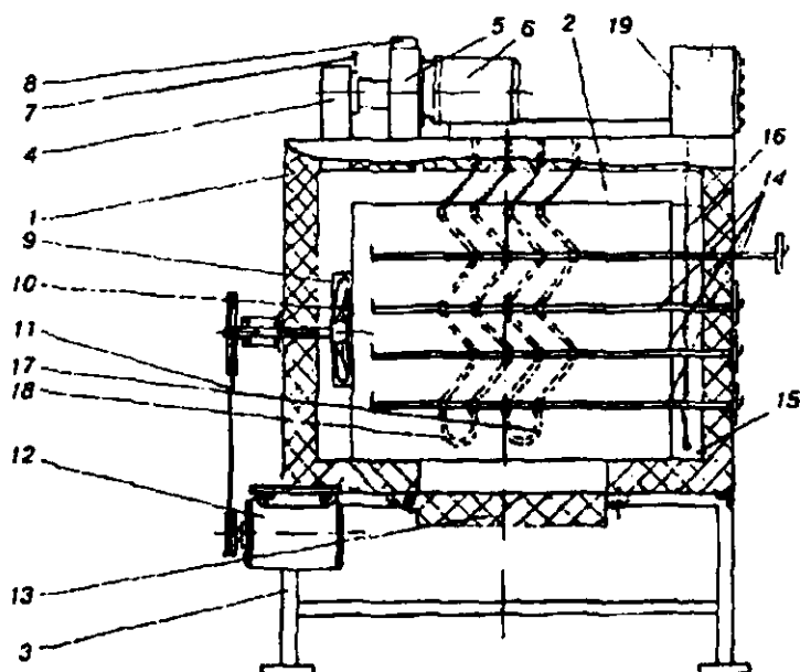
6.21-rasm. Fotopolimer qoliplarni quritish uskunasi- ning prinsipial sxemasi.
