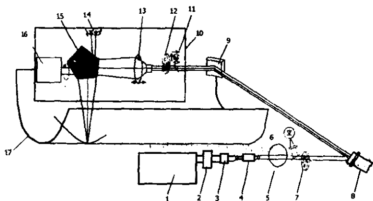
7.3-rasm. Guenberg rekorderning optik sxemasi.
