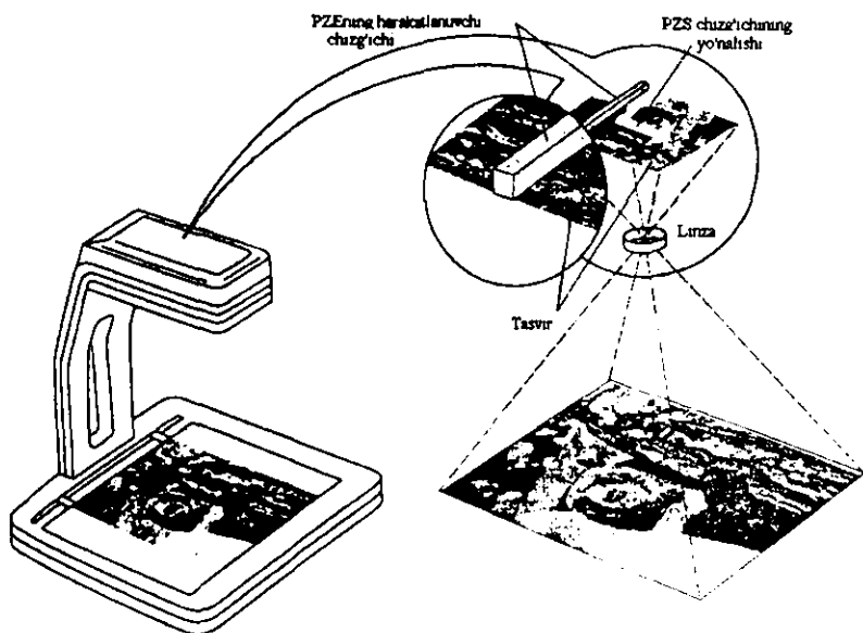
1.7-rasm. Proyeksion skanerning ishlash sxemasi.
