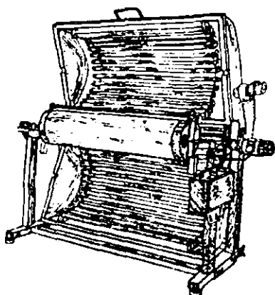
5.12-rasm. Ochiladigan nurlantiruvchi moslamali eksponirlovchi qurilma.
