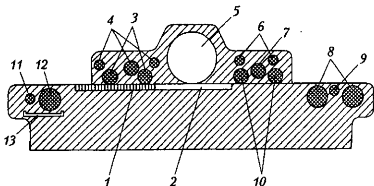
8.40-rasm. Ofset sinov nusxasini olish qurilmasining sxemasi.
