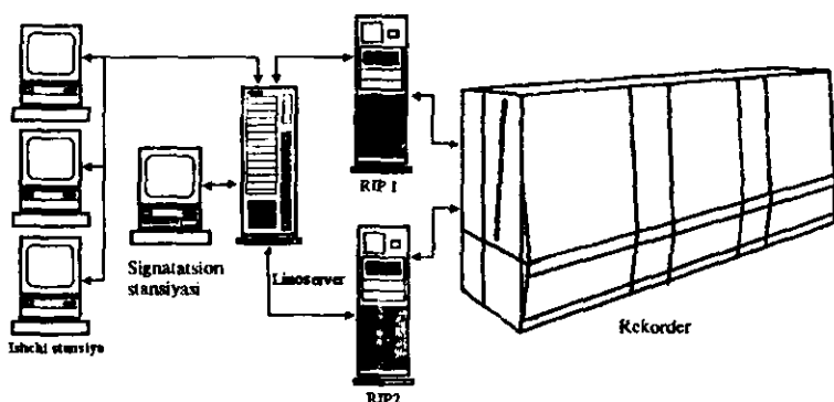
7.2-rasm. Gutenberg «Computer-to-Plate» sistemasining tuzilishi.
