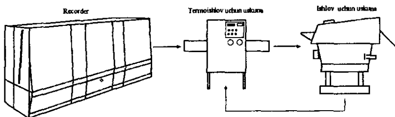
7.5-rasm. Bosma qolip tayyorlash uchun uskunalar majmui.
