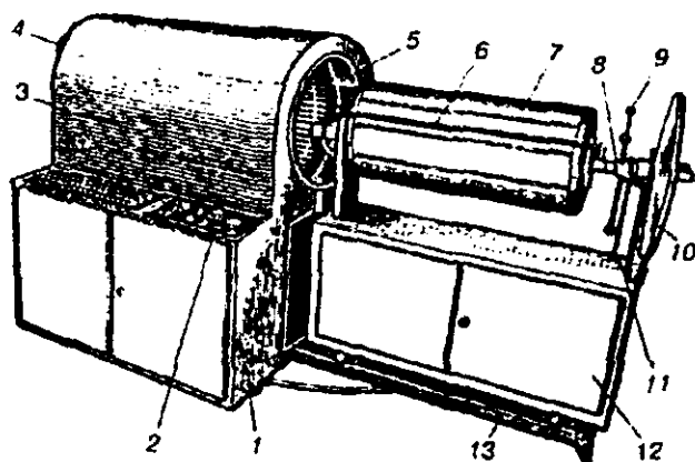
5.11-rasm. Silindr turidagi eksponirlovchi qurilma.
