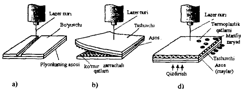
3.6-rasm. Quruq plyonkalarga ekspozitsiya jarayoni sxemalari.
