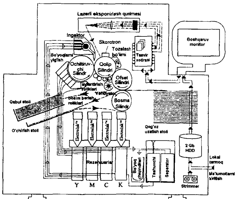
8.21-rasm. Raqamli bosish mashinasi:
