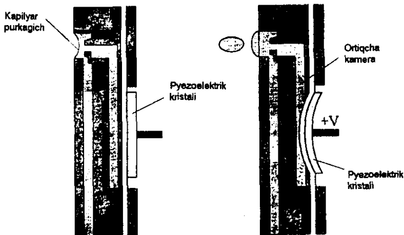
8.28-rasm. Pyezoelektrik boshcha sxemasi.
