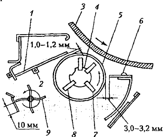
8.4-rasm. «Magnitli kist» turidagi ochiltirish qurilmasining sxemasi.
