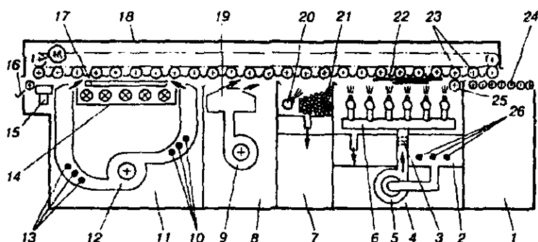
6.11-rasm. Aylanuvchi magnit roliklari asosida tashuvchi qurilmaning FBQga ishlov beruvchi oqim tizimi.
