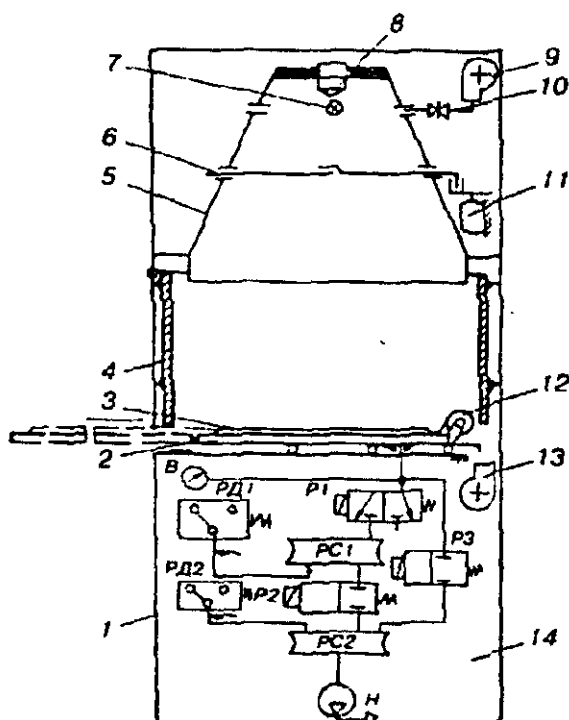
5.6-rasm. Metallogagenli yorug'lik manbali eksponirlovchi qurilmalarning sxemasi.
