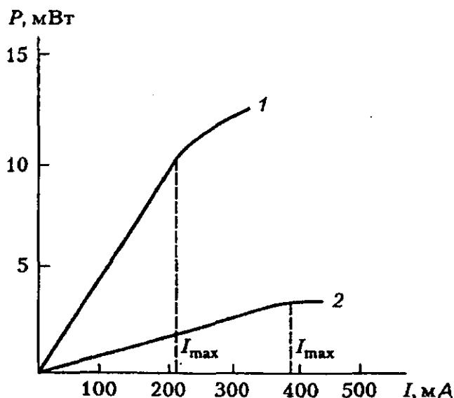
8.14-rasm. Turli yuza YOND ning vatt-ampere tavsifnomalari: 1-GaAlAs; 2-Jn GaAsP/JnP.
