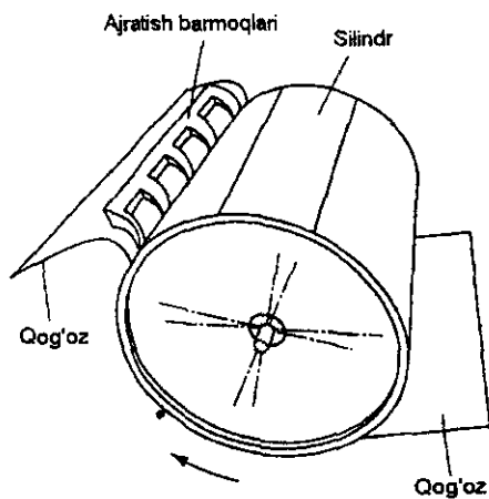
8.18-rasm. Ajratish barmoqlari.
