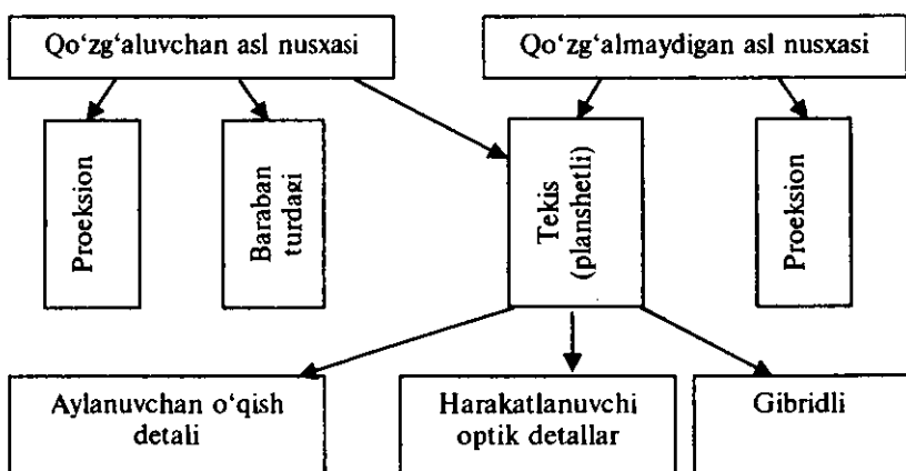
1.3-rasm. Skanerlash mexanizmlari klassifikatsiyasi.
