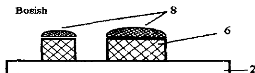
7.4-rasm. Termoplastinalarga tasvir yozish: 1 – emulsiya qatlami (termopolimer), 2 – alyumin asosi, 3 – lazer nuri, 4 – eksponirlangan polimer, 5 – qizdirish elementi, 6 – bosiluvchi elementlar, 7 – ochiltirgich, 8 – bosma bo'yog'i.
