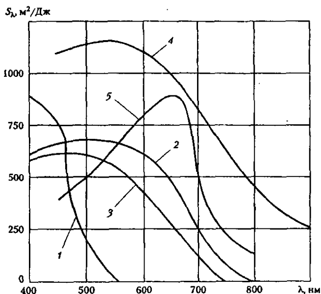
8.2-rasm. Ko'p marta qo'llanadigan EFQning spektral sezgirtligi: S_{\lambda} – fotosezgirtlik; \lambda – to'liqin uzunligi; 1 – Se, 2 – Se-Te; 3 – \text{As}_2\text{Se}_3 ; 4 – ko'p komponentli tuzimlar; 5 – amorf kremniy.
