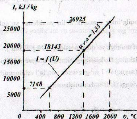
3.2. - rasm. Yoqilg'ini yonish issiqligi 600 ... 2000 °C oralig'ida yonish mahsulotlari uchun I -diagrammasi
