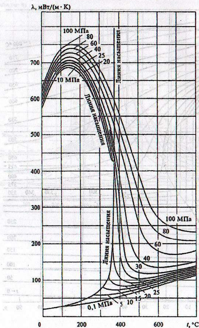
4-rasm. Suv va suv bug' issiqlik va bosimning issiqlik o'tkazuvchanligiga bog'liqligi
