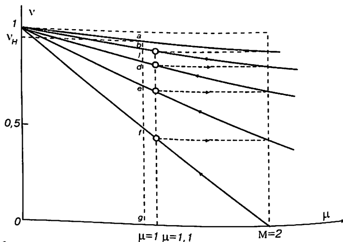
2.3- rasm. Mustaqil qo'zg'atishli o'zgaras tok dvigateli ishga tushirish reostatlar qiymatini hisoblash.
