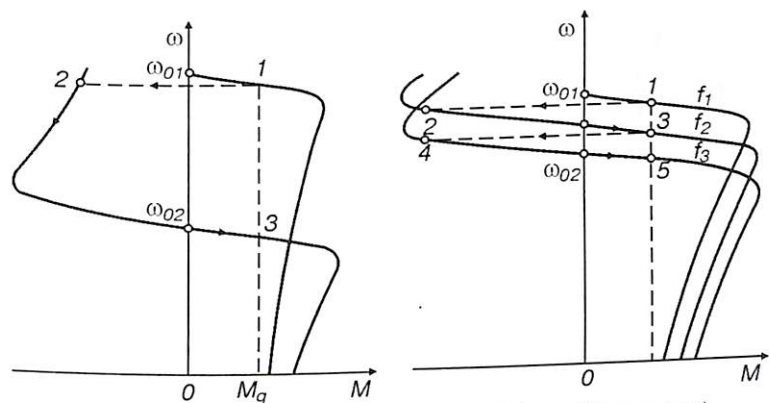
4.10- rasm. Asinxron dvigatelning reaktiv statik moment qo'yilganda generator tormozlash rejimidagi mexanik tavsiflari: a — juft qutblar sonini o'zgartirilgan holatidagi; b — tezlikni chastotali rostlangan holatidagi.
