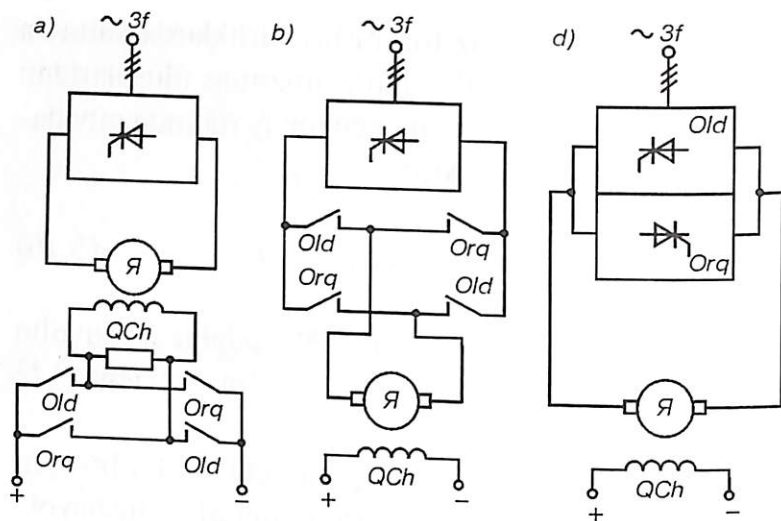
3.9- rasm. BO'-D tizimida reverslashning prinsipial sxemasi: a — dvigatel qo'zg'atish chulg'amini teskari ulash bilan; b — dvigatel yakorini teskari ulash bilan; d — ikkita komplekt o'zgartgichdan foydalanish bilan.
