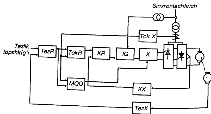
8.3- rasm. Elektr yuritmaning analog tizimi.
