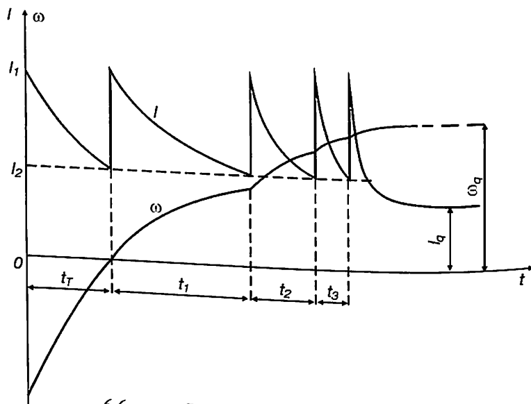
6.6- rasm. Dvigatelni reverslayotganda tok va tezlikning o'zgarish grafiği.
