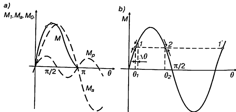
4.17- rasm. Burchak statik tavsiflari: a — ochiq ko'rsatilgan qutbli; b — reaktiv dvigatel.
