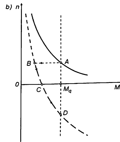
2.26- rasm. Dvigatelning aktiv statik moment ostida teskari ulash va reverslash rejimidagi mexanik tavsiflari.
