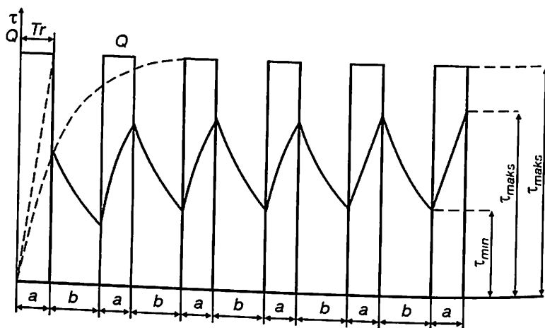
7.6- rasm. Dvigatelning qaytar-qisqa ish rejimining ideallashtirilgan grafigi.
