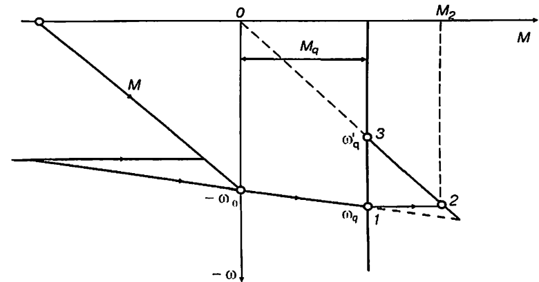
2.7- rasm. Ko'tarish mexanizmi yuritmasining rekuperativ tormozlash rejimidagi mexanik tavsiflari.
