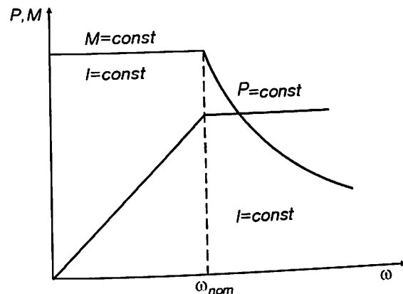
3.3- rasm. Generator-dvigatel tizimida o'zgaras moment va quvvatda tezlikni rostdlash rejimlari.
