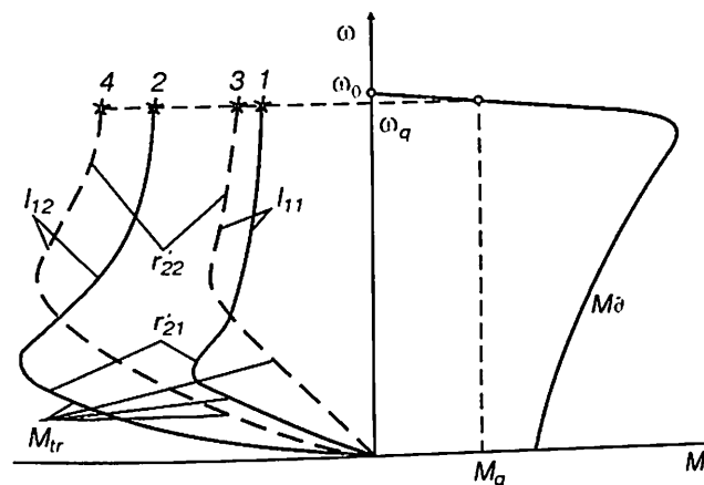
4.13- rasm. Asinxron dvigatelni qo'zg'atish tokining turli qiymatlarida o'zgartirib yoki rotor zanjirida turli qo'shimcha qarshilik kiritib olingan dinamik tormozlashdagi mexanik tavsiflari.
