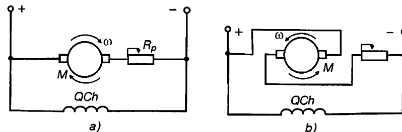
2.5- rasm. Mustaqil qo'zg'atishli dvigatel yakorini to'g'ri (a) va teskari (b) yo'nalishda aylantiruvchi ulanish sxemalari.
