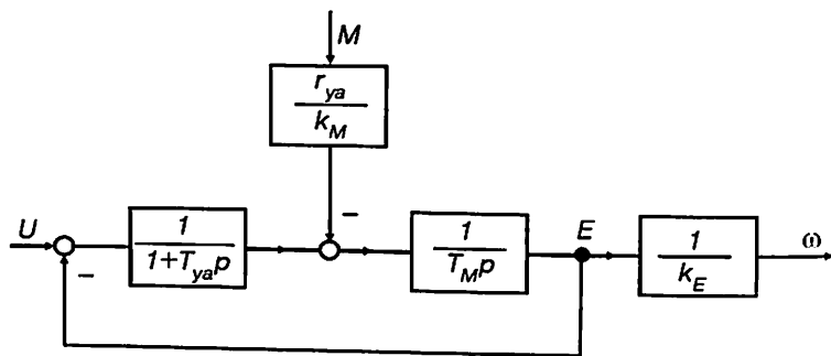
5.1- rasm. Mustaqil qo'zg'atishli o'zgarmas tok dvigatelining tezlikni mo'tadillash tizimidagi tuzilish sxemasi.
