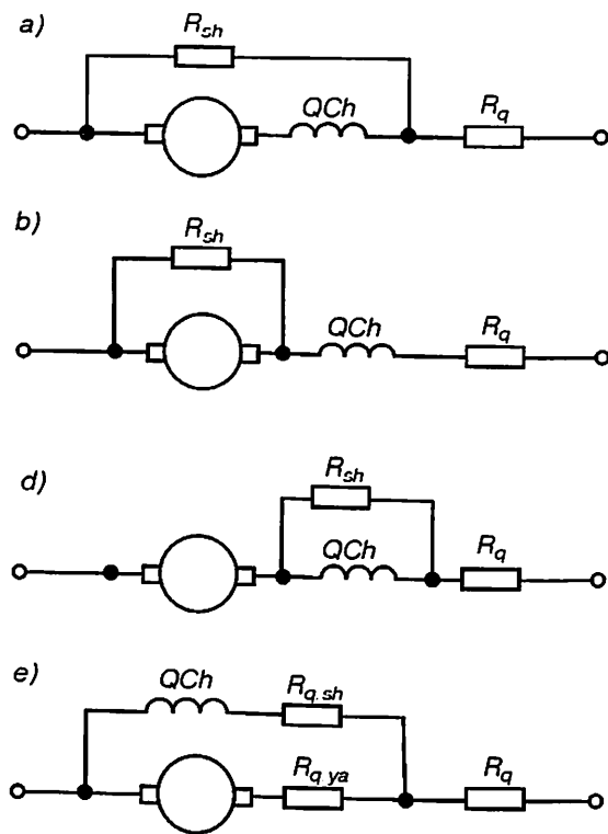
2.17- rasm. Ketma-ket qo'zg'atishli dvigatelda ketma-ket ulangan va shuntlovchi rezistorlarning ulanish sxemasi.
