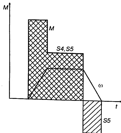
7.3- rasm. Nominal rejimlar S_4 va S_5 uchun yuklama diagrammalari.
