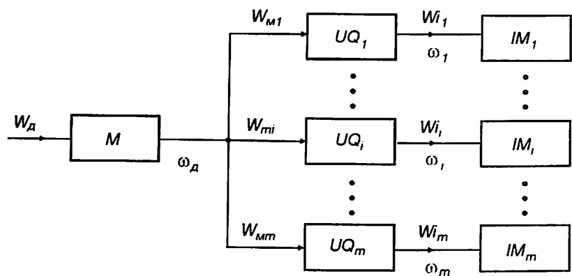
2- rasm. Guruhli elektr yuritmaning funksional sxemasi.
