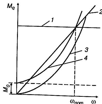
1.3- rasm. Statik momentning tezlikka bog'liqligi:
