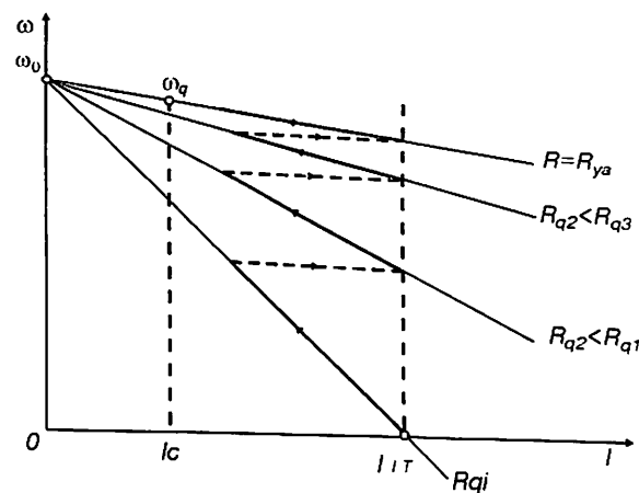
2.6- rasm. Dvigatelni ishga tushirish diagrammasi.
