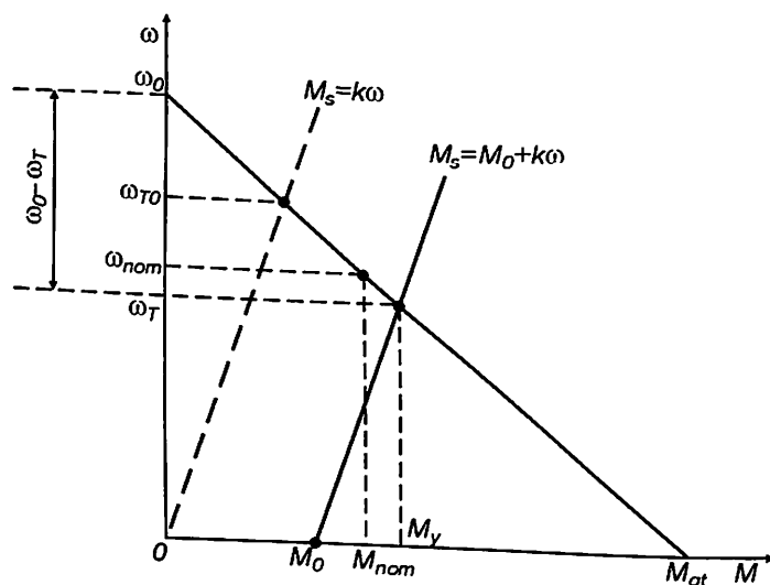
6.3- rasm. Statik momentlar turlicha bo'lgan holat uchun mexanik tavsifdagi ish nuqtalari.
