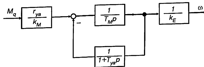
5.2- rasm. Mustaqil qo'zg'atishli o'zgarmas tok dvigatelining tashqi ta'sir uchun tuzilish sxemasi.
