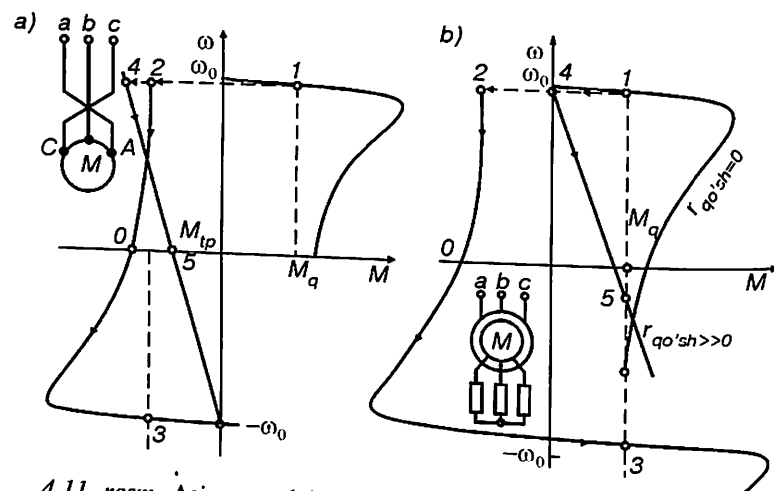
4.11- rasm. Asinxron dvigatelning ulanish sxemasi va mexanik tavsiflari: a — reaktiv statik momentda teskari ulanish rejimida; b — shuning o'zi, aktiv statik momentda.
