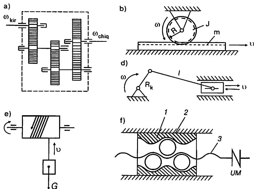
1.2- rasm. Uzatish qurilma turlari:
