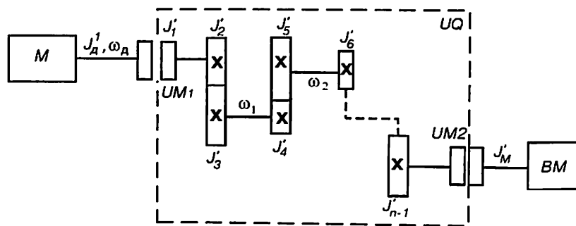
1.5- rasm. Elektr yuritmaning kinematik sxemasi.
