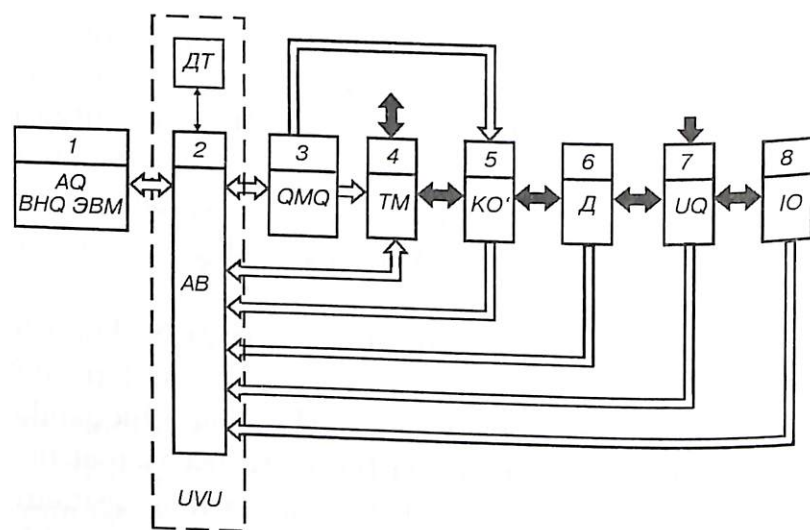
8.1- rasm. MP boshqarishli elektr yuritmaning tipik tizimi.
