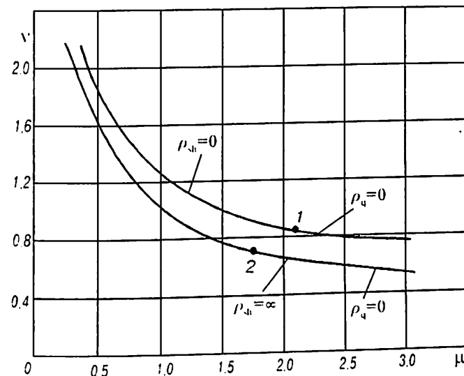
2.20- rasm. Dvigatelning 2.17- rasm, b dagi sxema bo'yicha qo'shimcha rezistorlar ulangan holatdagi mexanik tavsiflari.
