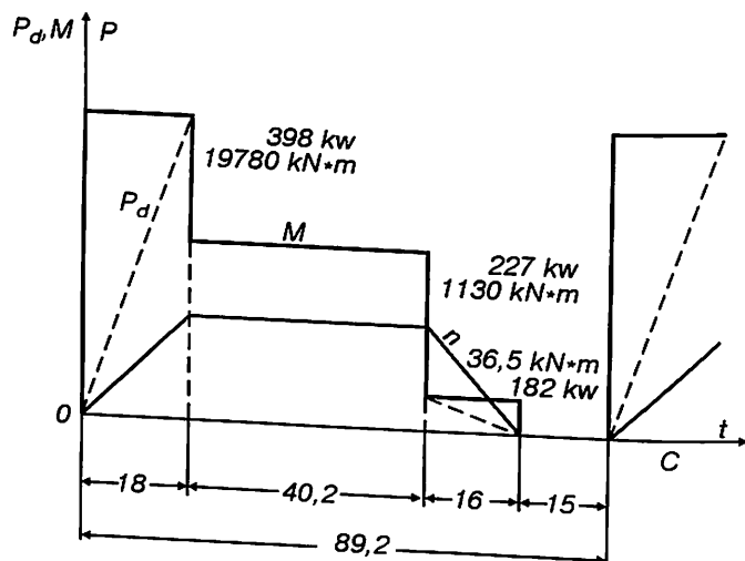
7.7- rasm. Shaxta ko'targichining yuklama diagrammasi.
