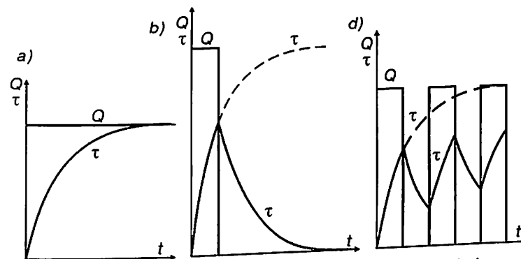
7.2- rasm. Elektr yuritmaning yuklama diagrammalari va dvigatel harorati o'zgarishining egri chiziqlari: a — davomli; b — qisqa; d — qaytar-qisqa ishlash rejimlarida.
