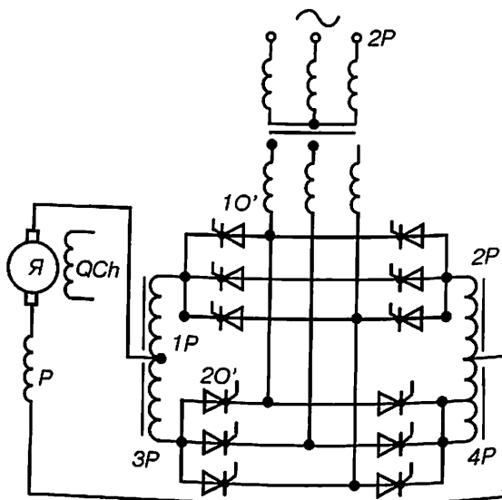
3.11- rasm. BO'-D tizimida o'zgartgichlarni qarama-qarshi parallel ulanish sxemasi: a — nol chiqishli; b — ko'priksimon.
