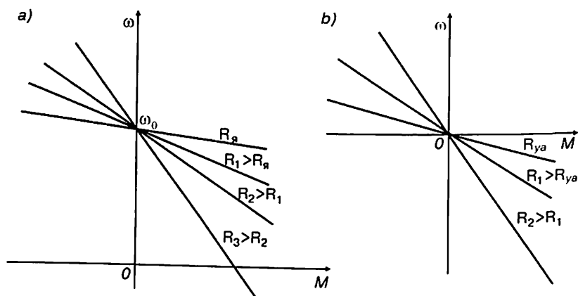
2.2- rasm. Mustaqil qo'zg'atishli o'zgarmas tok dvigatelining kuchlanish o'zgarmas bo'lgandagi va yakor zanjiridagi qarshiliklar o'zgargandagi (a), kuchlanish nol bo'lgandagi (b) mexanik tavsiflari.
