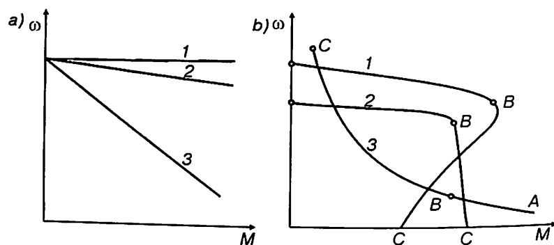
2.1- rasm. Dvigatelning mexanik tavsiflari: a — o'zgaras; b — o'zgaruvchan qattqlikdagi. 1 — absolut qattiq; 2 — qattiq; 3 — yumshoq.
