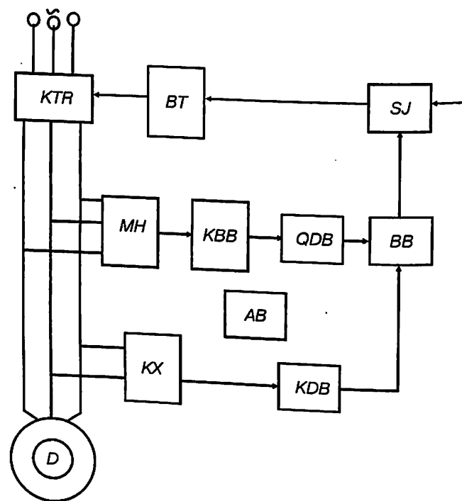
9.1- rasm. Energiyani tejaydigan asinxron elektr yuritma.
