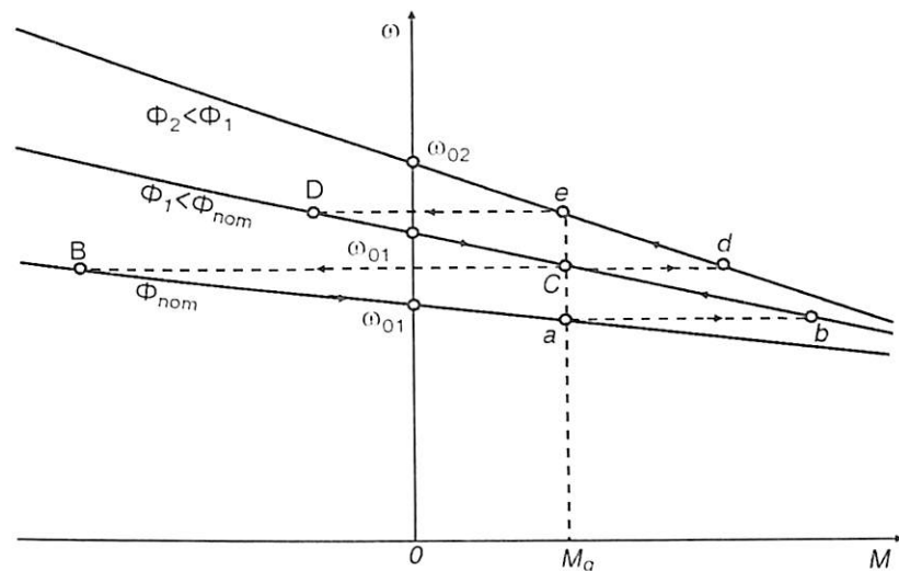
2.15- rasm. Mustaqil qo'zg'atishli dvigatelning magnet oqimi pasaytirilgandagi mexanik tavsiflari.
