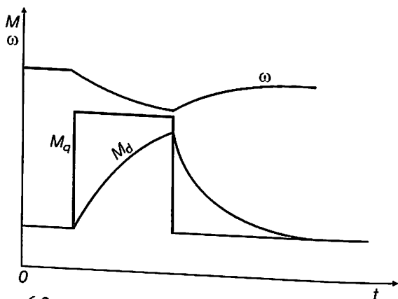
6.2- rasm. Yuklama berilganda moment va tezlikning o'zgarish grafiklari.
