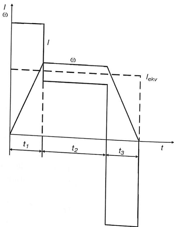
7.5- rasm. Dvigatelning qisqa ish grafigi.
