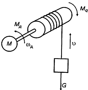
1.6- rasm. Yuk ko'taruvchi qurilmaning soddalashtirilgan kinematik sxemasi.
