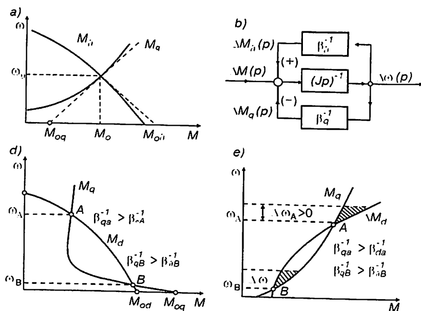
1.7-rasm. Elektr yuritmaning statik ustuvorligini aniqlash: a — statik yuklama va dvigatel tavsiflarini chiziqlashtirish; b — yuritmaning chiziqlashtirilgan modeli tuzilish sxemasi; d — yuklamani kichik tezliklarda noustivor va e — ustuvor ishlash variantlari.
