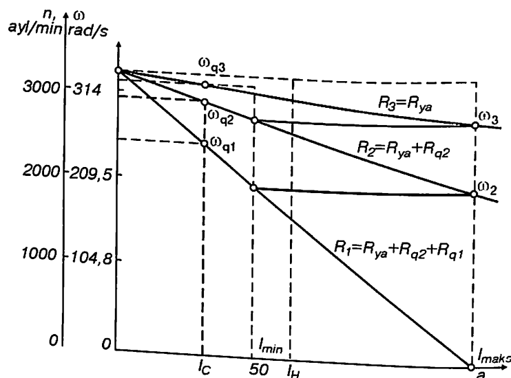
6.8- rasm. Ishga tushirish reostatlarini hisoblashga doir grafik.
