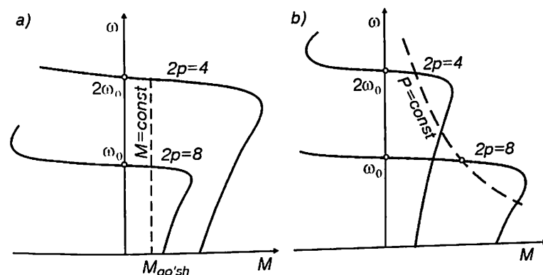
4.15- rasm. Ikki tezlikli dvigatelning mexanik tavsiflari: a — o'zgarmas moment rejimida; b — o'zgarmas quvvat rejimida.
