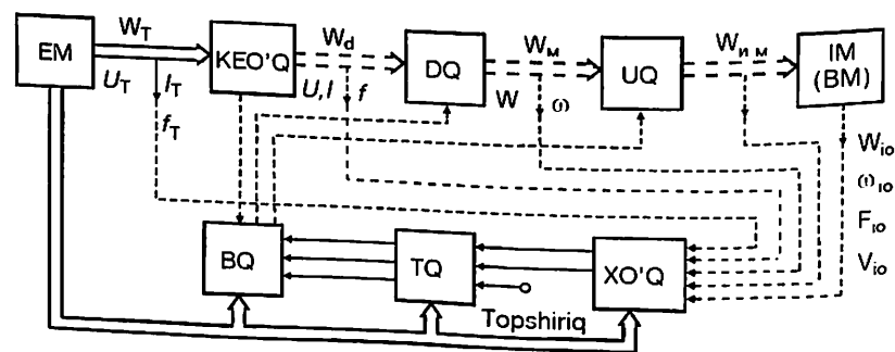
1-rasm. Avtomatlashtirilgan elektr yuritmaning funksional sxemasi.
