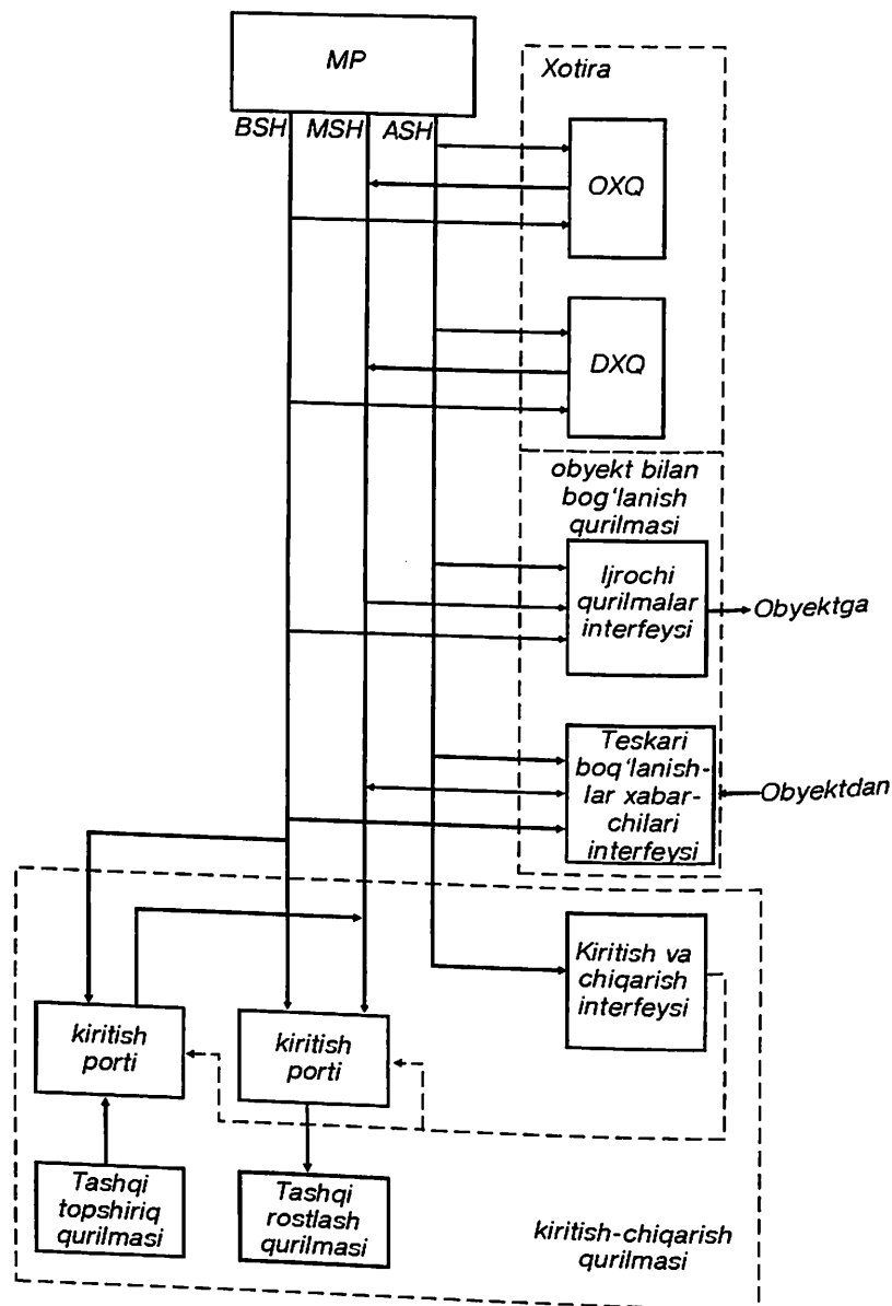
8.2- rasm. MP tizimining tuzilish sxemasi.
