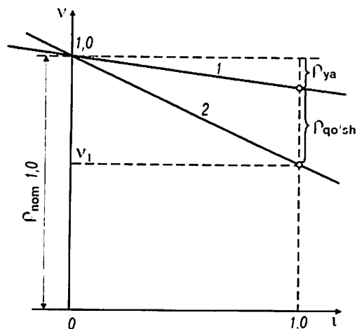
2.12- rasm. Mustaqil qo'zg'atishli dvigatelning mexanik tavsifini qurish.
