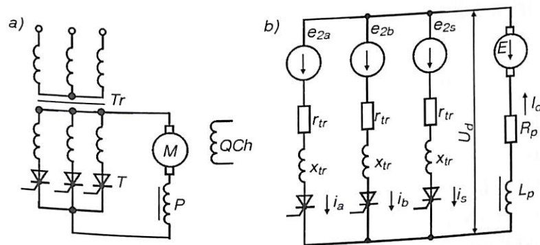
3.7- rasm. Uch fazali nul sxemali o'zgartgich BO'-D tizimi: a - tizim kuchli zanjirining soddalashtirilgan prinsipial sxemasi; b - ekvivalent sxemasi.
