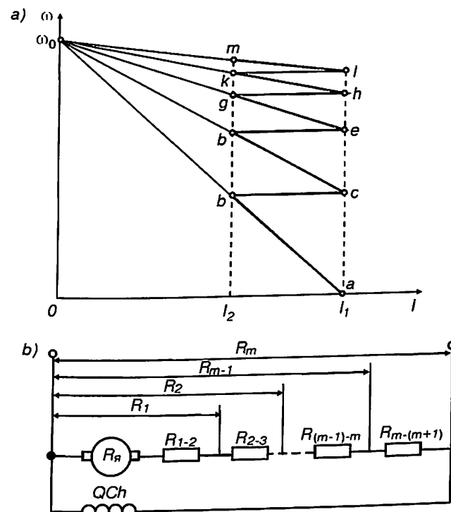
2.13- rasm. Mustaqil qo'zg'atishli dvigatelni ishga tushirish diagrammasi (a) va rezistor sekiyalarinih ulanish sxemasi (b).
