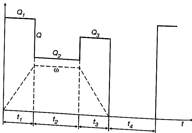
7.4-rasm. Tezlikning trapetsioidal diagrammasi va dvigateldagi isroflar grafigi.
