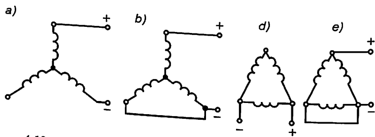
4.12- rasm. Dinamik tormozlashda asinxron dvigatel stator chulg'amlarini o'zgarmas (to'g'rilangan) tok manbayiga ulash sxemasi.
