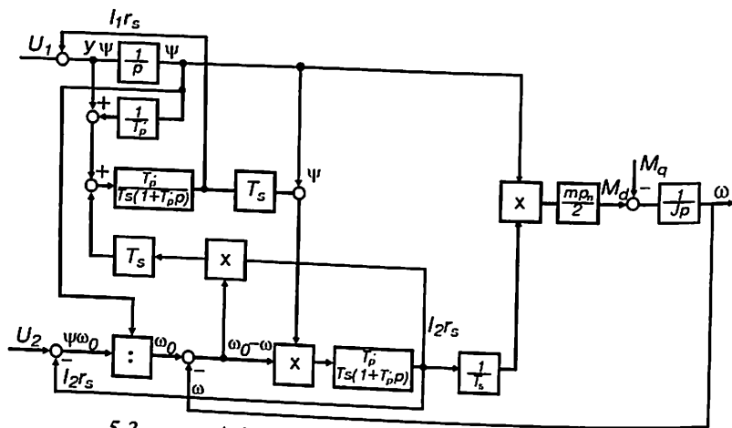
5.3- rasm. Asinxron dvigatelning tuzilish sxemasi.
