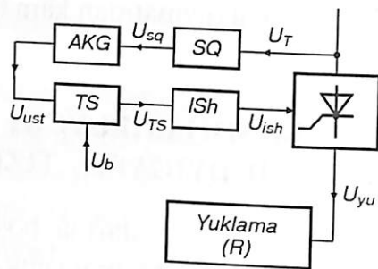
3.5- rasm. Boshqariluvchi to'g'rilagich sxemasi.
