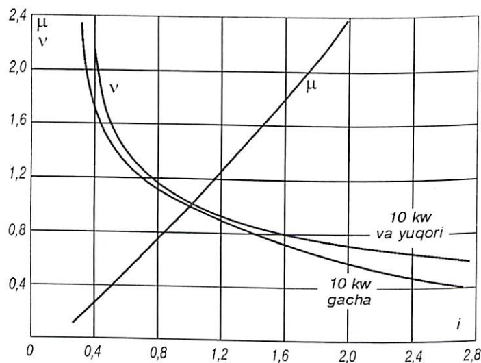
2.22- rasm. Ketma-ket qo'zg'atishli dvigatel momentinining va tezligining yakor tokiga bog'liqligi (nisbiy birliklarda).
