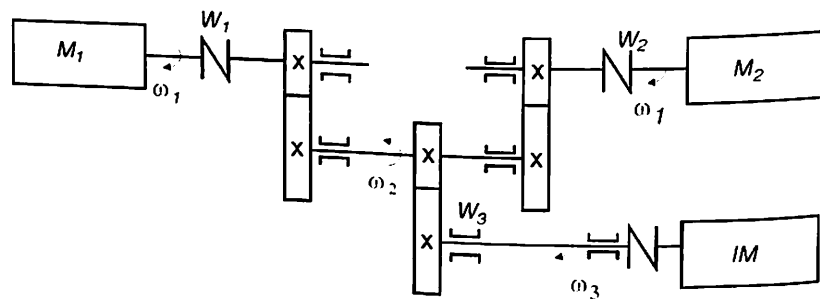
4- rasm. Ko'p dvigatelli elektr yuritmaning funksional sxemasi.
