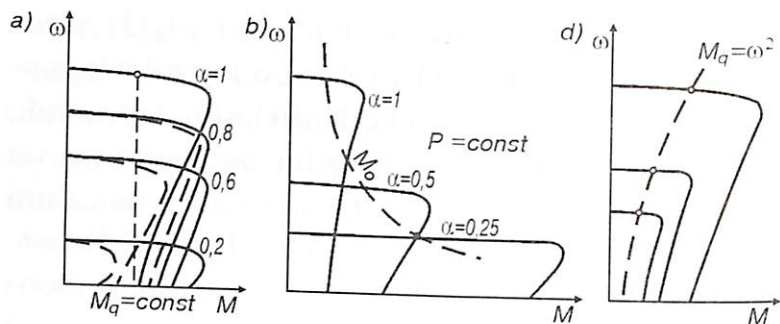
4.16- rasm. CHO-AD yuritma mexanik tavsiflari: a — o'zgaras momentda; b — o'zgaras quvvatda; d — ventilyatorli yuklamada.
