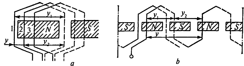
11.4- rasm. Sirtmoqsimon (a) va to'liqsimon (b) chulg'amlarning seksiyalari.
