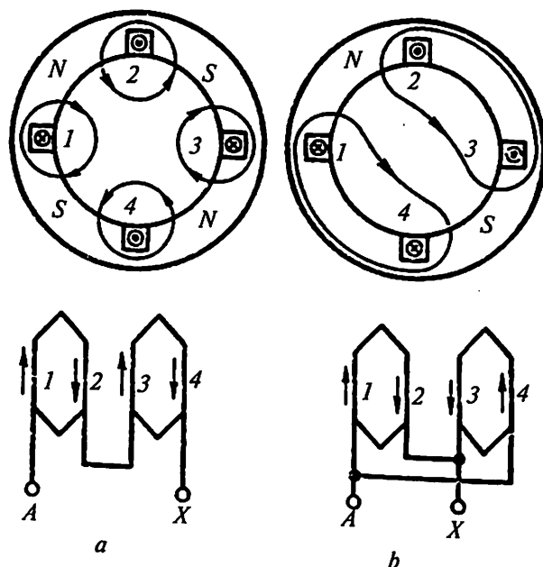
14.6- rasm. Stator faza chulg'ami qutblar sonini o'zgartirishning eng oddiy sxemalari.
