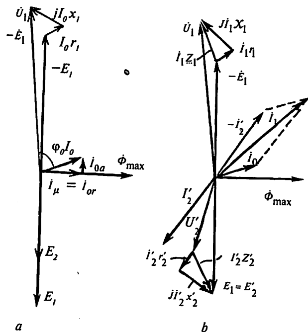
12.2- rasm. Rotori tormozlangan asinxron mashinaning salt ishlash (a) va yuklama ulangan (b) rejimlari uchun vektor diagrammalar.
