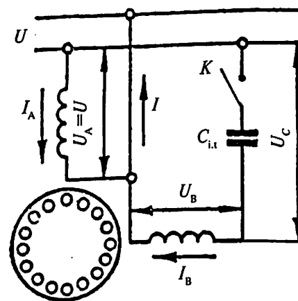
15.3- rasm. Kondensatorli asinxron motor sxemasi:
