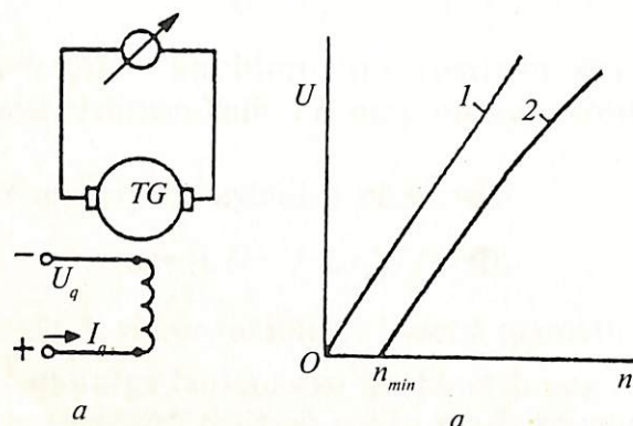
5.1- rasm. O'zgaras tok taxogeneratori (a) ning to'g'ri chiziqli (1) va egri chiziqli (2) chiqish xarakteristikalar (b)
