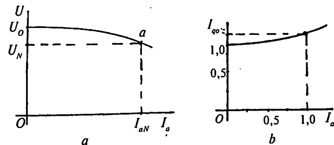
3.2- rasm. Mustaqil qo'zg'atishli o'zgarmas tok generatorining tashqi (a) va rostlash (b) xarakteristikalari.
