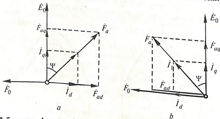
17.5- rasm. Ayon qutbli sinxron generatorning yakor toki va MYK ning bo'ylama va ko'ndalang tashkil etuvchilari.
