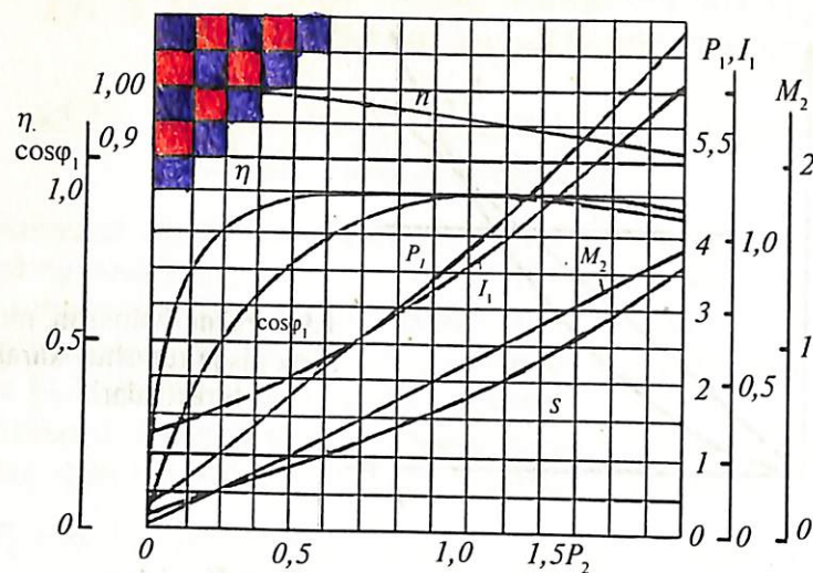
13.3- rasm. Asinxron motorning ish xarakteristiklari.
