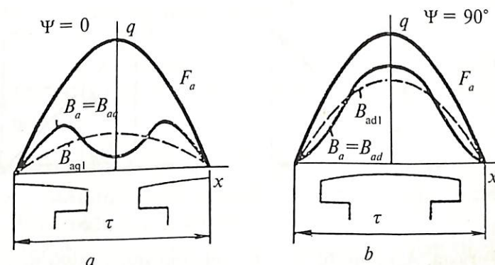
17.4- rasm. Mashina magnit induksiyasining tarqalish egri chizig'i.
