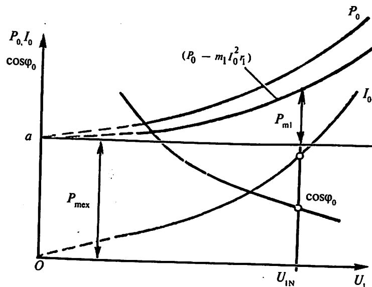
13.1- rasm. Asinxron motorning salt ishlash xarakteristikallari.
