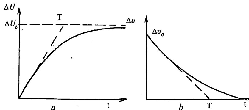
21.2- rasm. Mashina qizishi (a) va sovishi (b) ning vaqt bo'yicha o'zgarishi.
