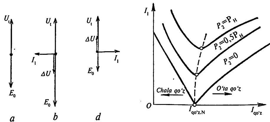
18.3- rasm. P_{em} P_2 = 0 bo'lganda, tarmoqqa parallel ulangan noayon qutbli sinxron generatorning sodda vektor diagrammalari va U- simon xarakteristikalari.
