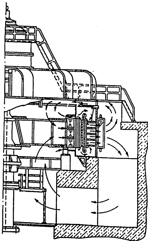
21.9- rasm. Hidrogeneratorning ventilatsiya sxemasi.
