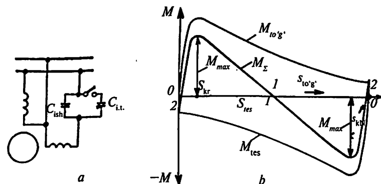
15.1- rasm. Bir fazali motor: a — ulanish sxemasi; b — mexanik xarakteristikalari: C_{ish} — ish kondensatori; C_{ish.t} — ishga tushirish kondensatori.
