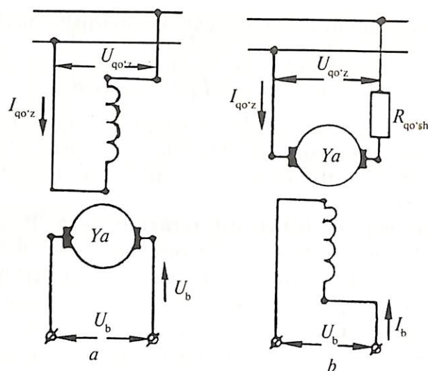
5.2- rasm. Ijrochi o'zgaras tok motorlari: (a)— yakordan boshqariladigan, (b) — qutbdan boshqariladigan.
