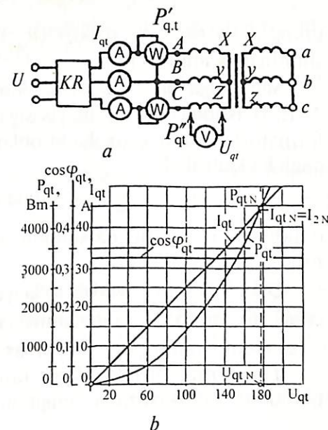
7.4- rasm. Ikki chulg'amli uch fazali transformatorni qisqa tutashirib tajriba o'tkazish sxemasi (a); qisqa tutashuv xarakteristikallari (b); KR — kuchlanishni rostlagich.
