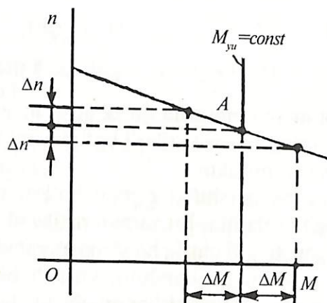
4.4- rasm. Elektr motor va ish mexanizmining turg'un ishlash shartlarini tushuntirishga oid mexanik xarakteristikalar.
