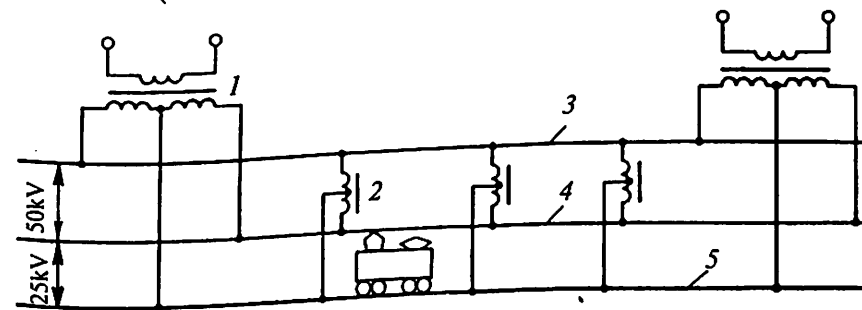
9.5- rasm. Elektrlashtirilgan temiryo'lning 2x25 kV li elektr ta'minoti sistemasining tortish podstansiyasidagi ikkilamchi chulg'ami bo'lingan bir fazali maxsus maqsadli kuch transformatori:
