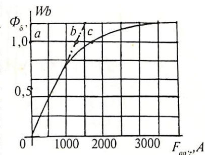
2.2- rasm. O'zgaras tok mashinasining magnit xarakteristikasi.
