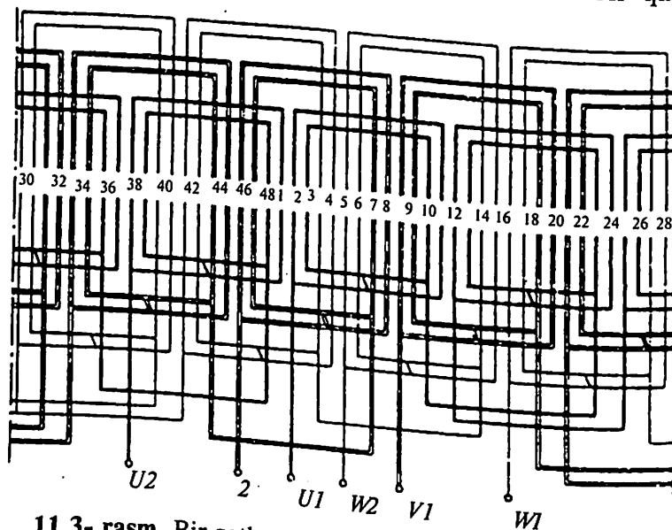
11.3- rasm. Bir qatlamli konsentrik chulg'am sxemasi: Z=48, 2p=4, q=4, a=1 .
