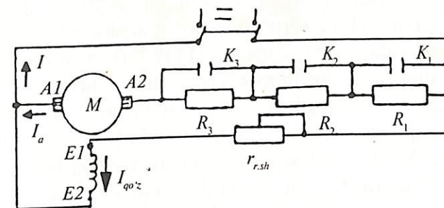
4.7- rasm. Avtomatlashtirilgan elektr yuritmada parallel qo'zg'atishli o'zgarmas tok motorini ishga tushirish.
