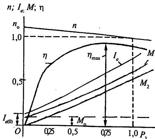
4.1- rasm. Parallel qo'zg'atishli motorning ish xarakteristikalarini.
