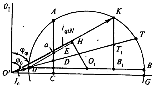
13.5- rasm. Asinxron mashinaning soddalashtirilgan doiraviy diagrammasi.
