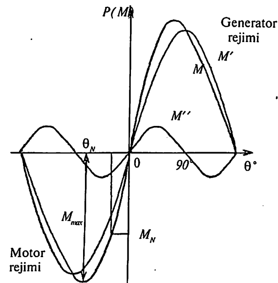
19.3- rasm. Ayon qutbli sinxron mashinaning burchak xarakteristikasi:
