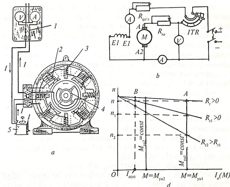
4.9- rasm. Parallel qo'zg'atishli motorda tajriba o'tkazish qurilmasi (a); tajriba o'tkazish sxemasi (b); motorning tezlik xarakteristikallari (d): 1 — ulab-uzgich; 2 — qo'zg'atish chulg'ami; 3 — qo'shimcha qutb chulg'ami; 4 — kollektor; 5 — ishga tushirish reostati.
