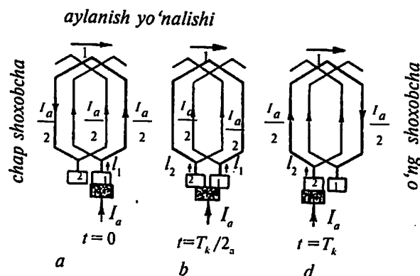
2.5- rasm. Kommutatsiyalanuvchi seksiyada tok yo'nalishining o'zgarishi.
