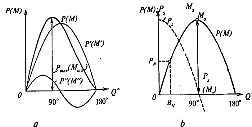
18.2- rasm. SG larning burchak xarakteristikalar:
