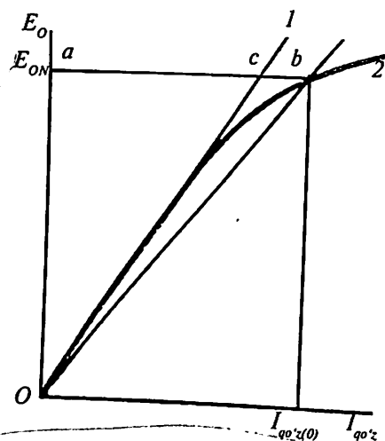
17.2-rasm. Sinxron generatorning salt ishlash xarakteristikasi:
