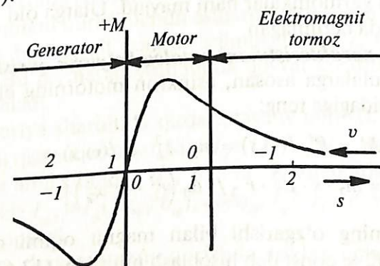
13.4- rasm. Asinxron motorning mexanik xarakteristikasi.
