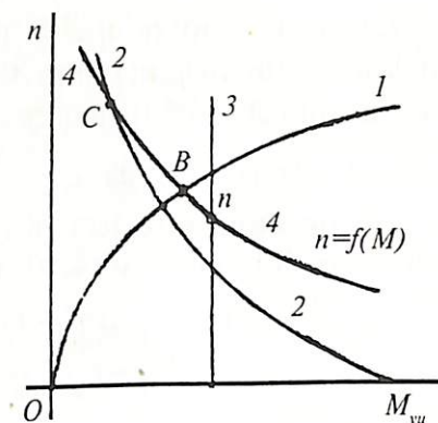
4.5- rasm. Har xil ish mexanizmlariga xos bo'lgan n = f(M_{yu}) bog'lanish (1, 2 va 3); 4 — ketma-ket qo'zg'atishli motorning tabiiy mexanik xarakteristikasi n = f(M_{yu})
