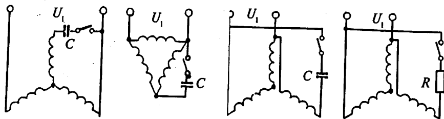
15.2-rasm. Uch fazali qisqa tutashgan rotorli asinxron motorni bir fazali elektr tarmog'idan ishlatish.
