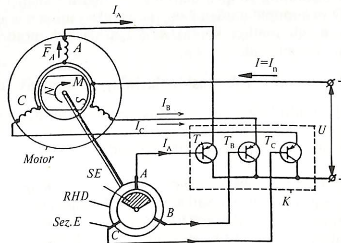
5.3- rasm. Kontaktsiz o'zgaras tok motorining prinsipial sxemasi.
