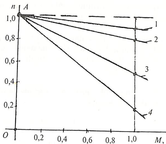
4.3- rasm. Parallel qo'zg'atishli motorning mexanik xarakteristikalar.
