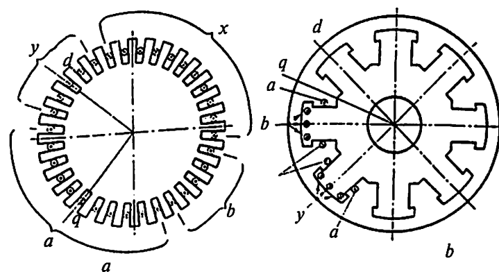
20.1- rasm. Qo'zg'atish chulg'amlari ax va by har xil bo'lgan noayon qutbli rotor (a) va dempfer chulg'ami o'rniga ko'ndalang qo'zg'atish chulg'ami o'rnatilgan ayon qutbli rotor (b).
