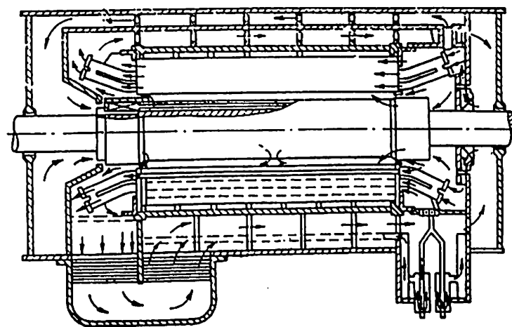
21.7- rasm. Ventilatsiyasi aksial sistemali, quvvati 300 MW bo'lgan turbogeneratorning konstruktiv sxemasi.
