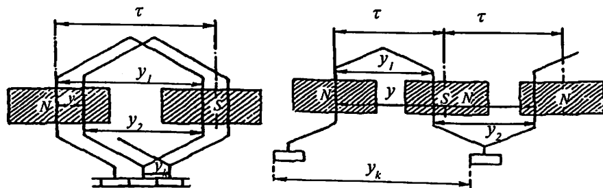
1.4- rasm. O'zgarmas tok mashinasi sirtmoqsimon va to'liqsimon yakor chulg'amlarining elementlari va qadamlari.
