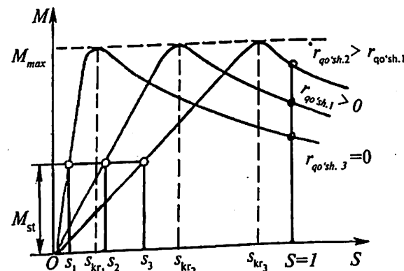
13.7- rasm. Faza rotorli asinxron motorning mexanik xarakteristikalari: M_{st} — statik moment; M_{\text{max}} — maksimal moment; s_{kr1} , s_{kr2} , s_{kr3} — tegishlixa kritik sirpanishlar; r_{qo'sh1} , r_{qo'sh2} , r_{qo'sh3} — tegishlixa qo'shimcha qarshiliklar.
