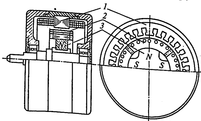
20.4- rasm. O'zgaras magniti rotorda radial joylashtirilgan sinxron motor:
