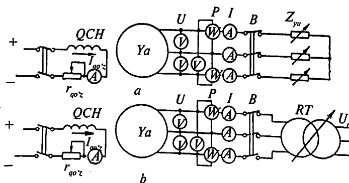
17.7-rasm. Sinxron generator xarakteristikalarini tajriba o'tkazib qurish.
