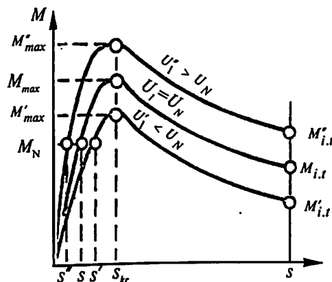
13.6- rasm. Kuchlanish nominaldan farqli bo'lgandagi mexanik xarakteristikalar.
