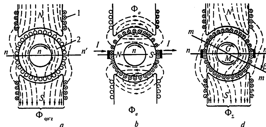
2.4- rasm. O'zgarmas tok mashinasining magnit maydoni:
