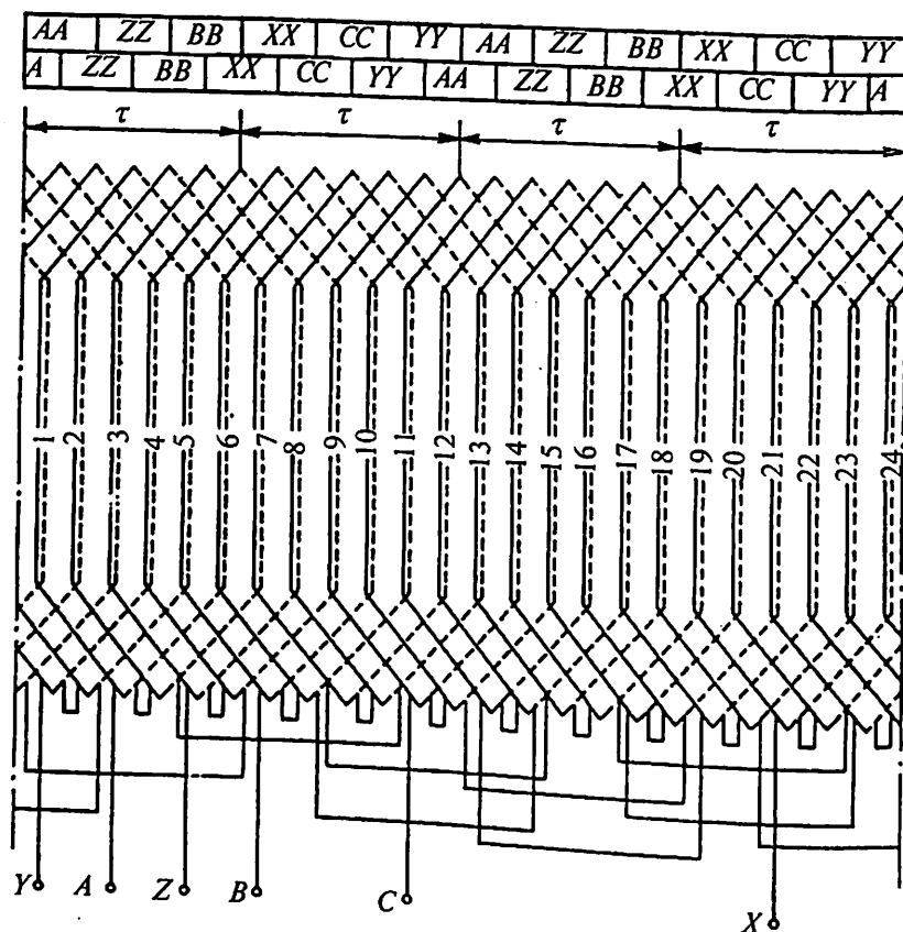
11.5- rasm. Uch fazali ikki qatlamli sirtmoqsimon chulg'am sxemasi: Z = 24 , m = 3 , 2p = 4 , y = 5 .
