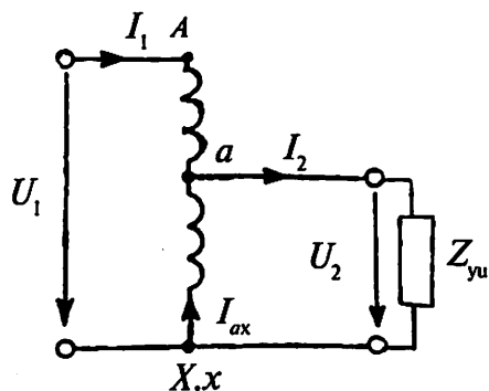
9.2- rasm. Chulg'amining bir qismi ikkilamchi chulg'am vazifasini bajaradigan bir fazali pasaytiruvchi avtotransformator- ning prinsipial sxemasi.
