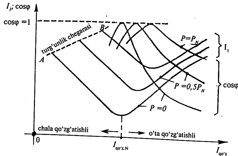
19.4- rasm. Sinxron motorning U - simon xarakteristikalari.
