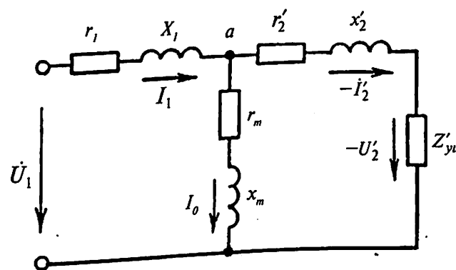
12.3- rasm. Rotori tormozlangan asinxron mashinaning almashtirish sxemasi.
