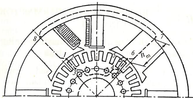
2.1- rasm. Kompensatsiyalovchi chulg'ami bo'lmagan o'zgaras tok mashinasining magnit zanjiri.
