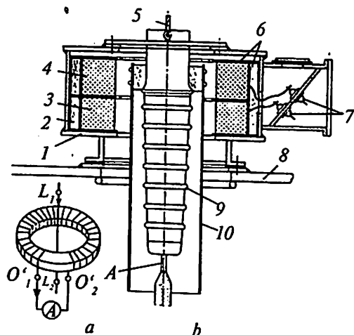
9.7- rasm. Kuchlanishi 110 kV bo'lgan kuch transformatori baki-ning ichiga o'rnatilgan tok transformatorining ulanish sxemasi (a): L_1 va L_2 — birlamchi chulg'am uchlari; O_1 va O_2 — ikkilamchi chulg'am uchlari; tok transformatorining konstruksiyasi (b):
