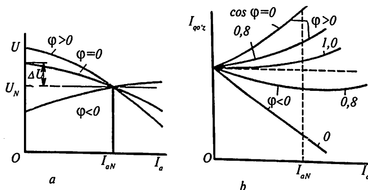
17.9- rasm. Sinxron generatorning tashqi (a) va rostlash (b) xarakteristikalari.
