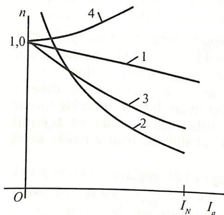
4.10- rasm. Har xil qo'zg'atishli motorlarning n=f(I_a) — tezlik xarakteristikalar:
