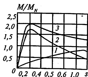
14.4- rasm. Qo'sh katakli motorning mexanik xarakteristikalari.
