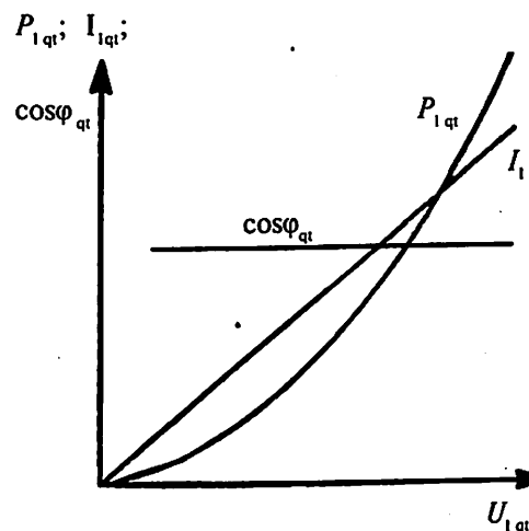
13.2- rasm. Asinxron motorning qisqa tutashuv xarakteristikallari.
