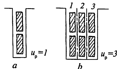
1.3- rasm. O'zgarmas tok mashinalarida elementar paz sxemasi.
