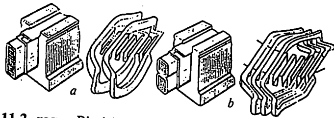
11.2- rasm. Bir (a) va ikki (b) qatlamli chulg'amlarning g'altaklarda joylashishi.
