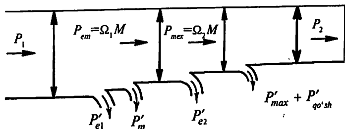
12.5- rasm. Asinxron motorning energetik diagrammasi.
