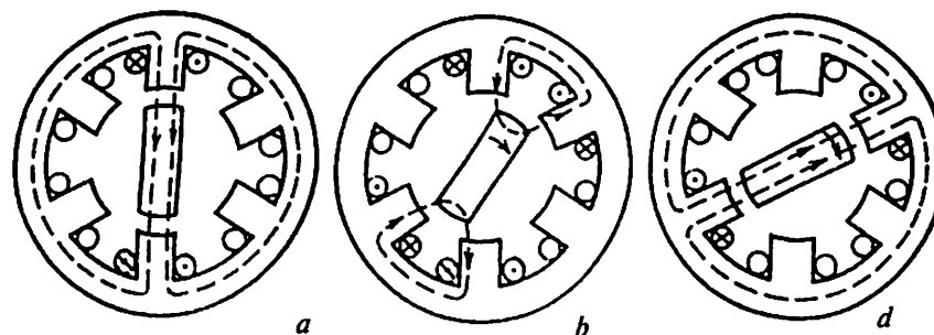
20.5- rasm. Ikki qutbli — qadamli reaktiv motorning ishlash prinsipi.
