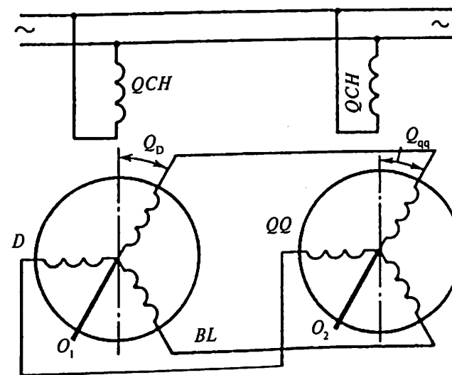
16.3- rasm. Selsinning indikator rejimi: D — datchik; QQ — qabul qilgich (priyomnik); BL — bog'lovchi liniya (sim)lar; QCH — qo'zg'atish chulg'ami.
