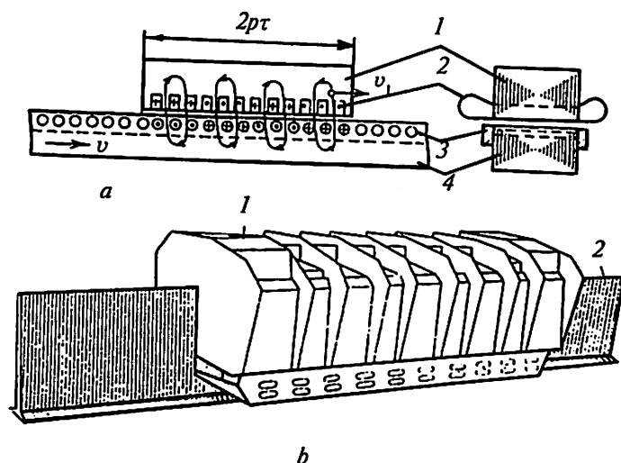
16.4- rasm. Chiziqli asinxron motor: a — elektromagnit sxemasi; b — umumiy ko‘rinishi: 1 — stator po‘lat o‘zagi; 2 — stator chulg‘ami; 3 — rotor chulg‘ami; 4 — rotor po‘lat o‘zagi.
