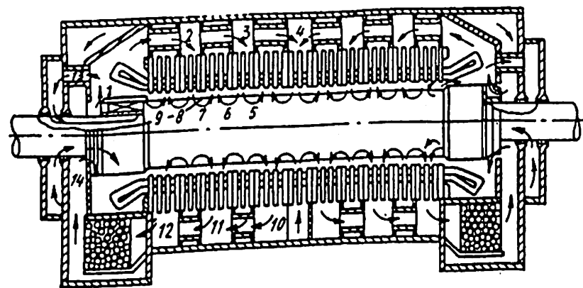
21.8- rasm. Ventilatsiyasi radial sistemali, quvvati 200 MW bo'lgan turbogeneratorning konstruktiv sxemasi.
