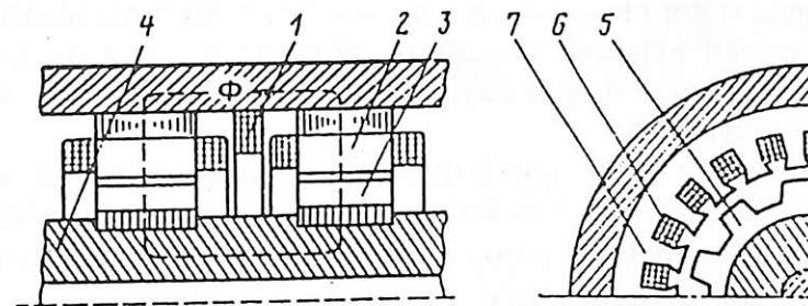
20.2- rasm. Qutblari bir xil ishorali induktorli generator:
