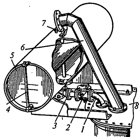
10.1-rasm. Kengaytirgich (5), saqllovchi truba (6), gaz relesi (2) va naychali moy ko'rsatkich (4) larning transformator bakida joylashtirilishi:
