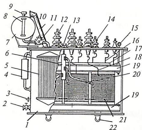
6.1- rasm. Kuchlanishi 35 kV, quvvati 1000 ÷ 6300 kV·A bo'lgan pasaytiruvchi kuch transformatori:
