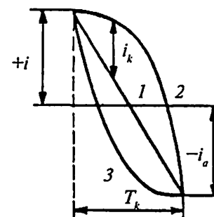
2.6- rasm. O'zgaras tok mashinasida tok kommutatsiyasi:
