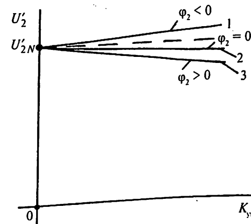
7.5- rasm. Transformatorning tashqi xarakteristikalarini uchun. 1 — aktiv sig'im; 2 — aktiv; 3 — aktiv-induktiv yuklamalar
