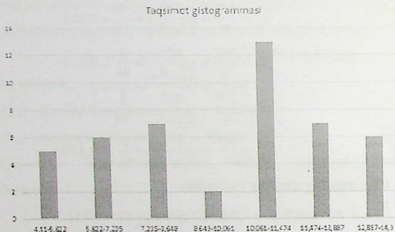
2.2.6-rasm. Tuproq namligi o'lchamlarining taqsimot gistogrammasi
