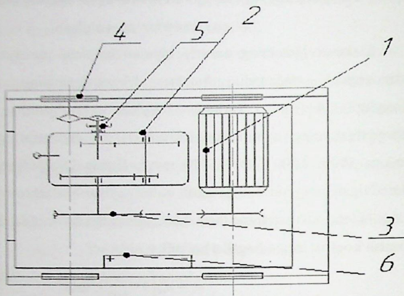
3.2.1-rasm. 1-elektrodvigatel, 2-reduktor, 3- shkv, 4- g'ildirak, 5- mufti, 6-elekt manbai
