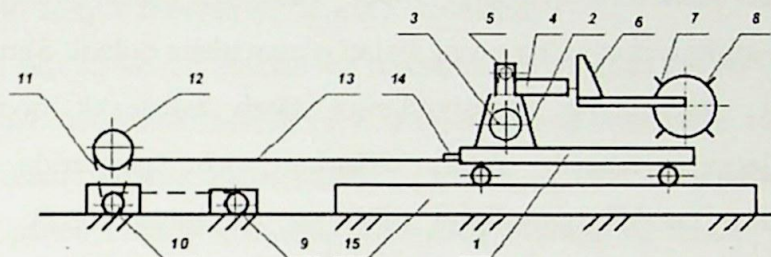
1.3.4-Rasm. Eksperimental o'rnatish sxemasi:
