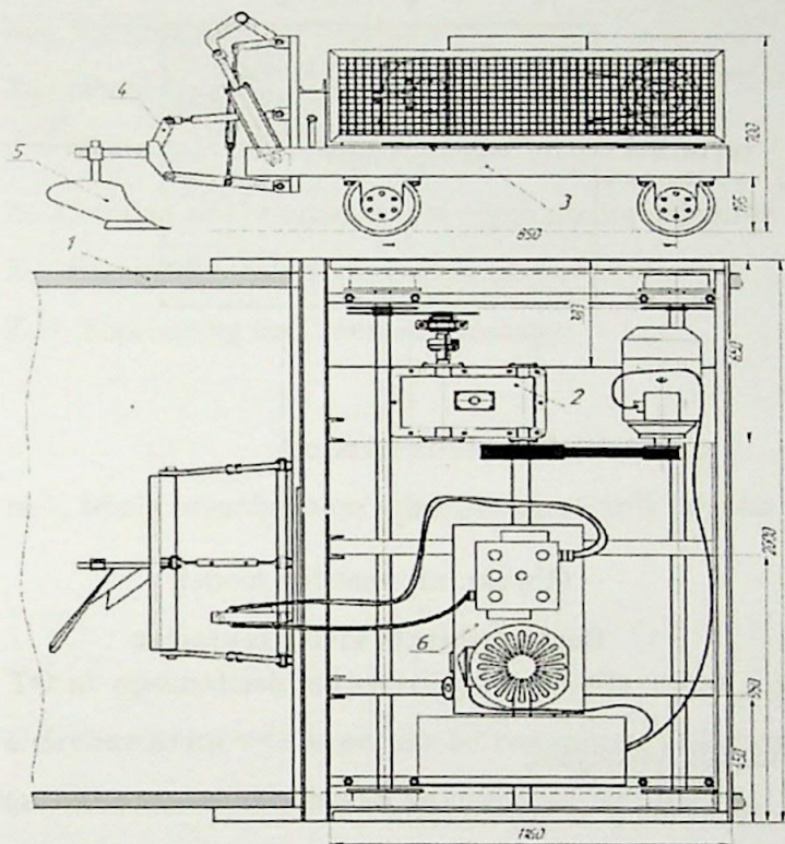
2.2.1-rasm Yangi ko'rinishdagi Kichik tuproq kanalli aravacha konstruktiv ko'rinishi:
