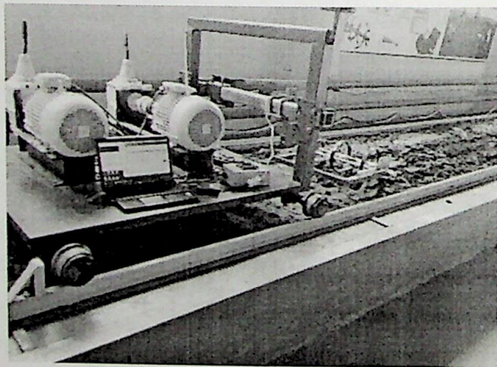
1.3.5-Rasm kombinatsiyalashgan ishchi organlarni sinash stendi
