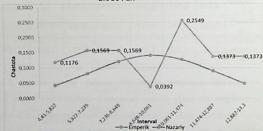
2.2.9-rasm tuproq namligi bo‘yicha nazariy va empirik taqsimotni approksimatsiyalash grafigi
