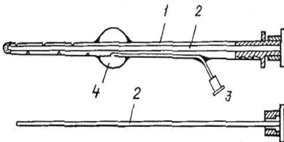
5-rasm. Embrionlarni yuvib olishda ishlatishda kateter
