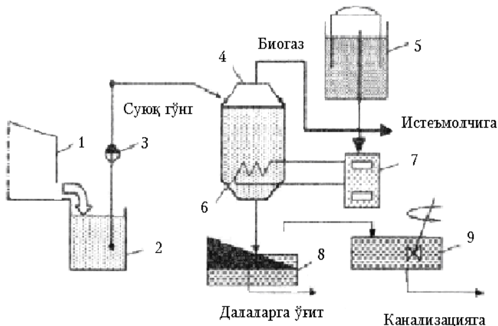
18-rasm. Go'ng sharbatini biogaz usqurmasida qayta ishlashni texnologik chizmasi
