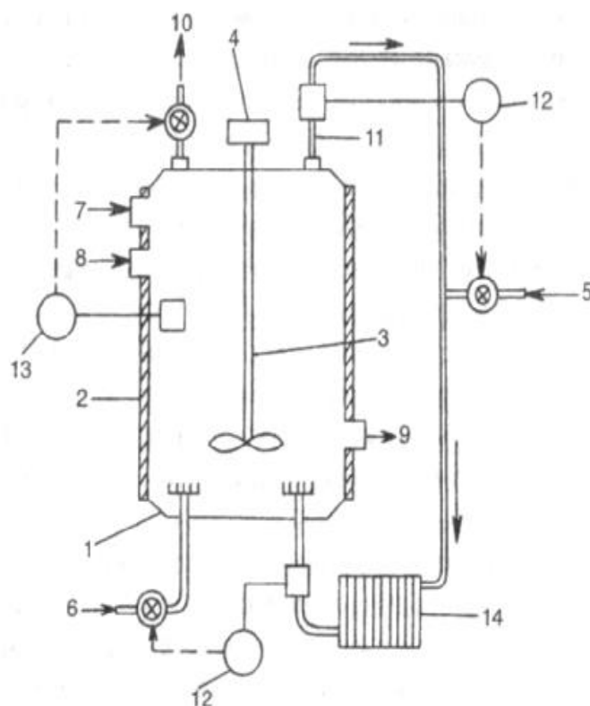
6.2-расм. Газсимон углеводородларда микроорганизмлар ўстириш учун ферментёр
