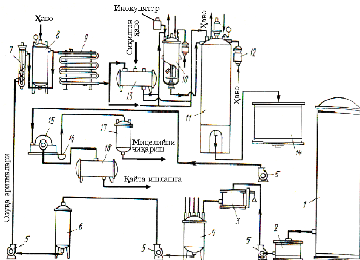
5.4-расм. Суюқликда ўстириш усулида лимон кислота олишнинг технологик чизмаси (Карклиньш ва Пробок, 1972):
