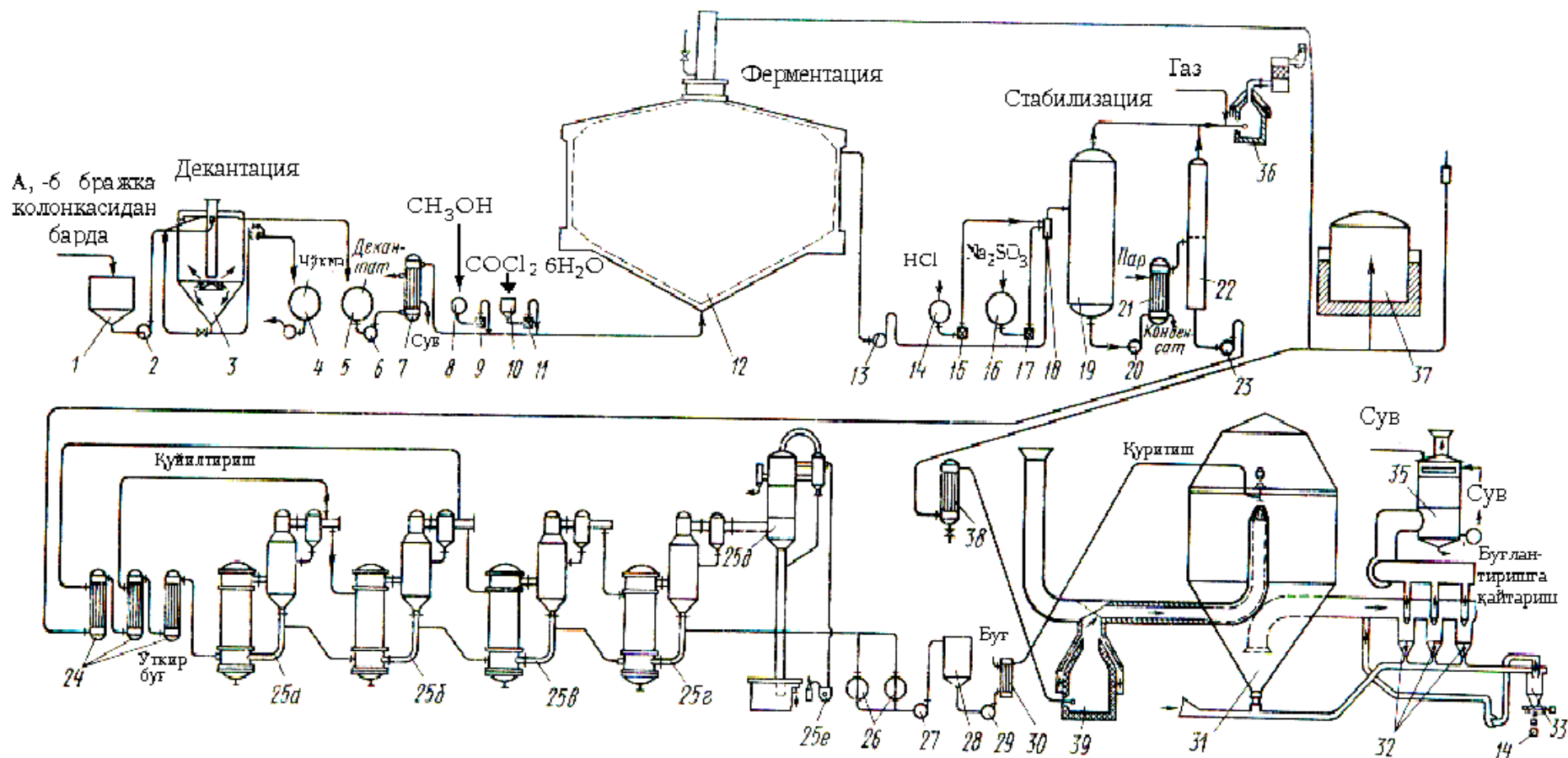
7.2-чизма. B 12 -витамины концентратини метан ҳосил қилувчи аралаш культуралар ёрдамида олишнинг технологик чизмаси:
