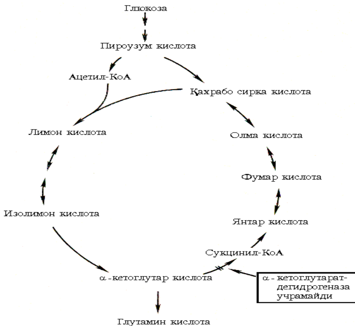
4.2-расм. Corynebacterium gluhamicum бактериясининг глутамин кислота биосинтези чизмаси
