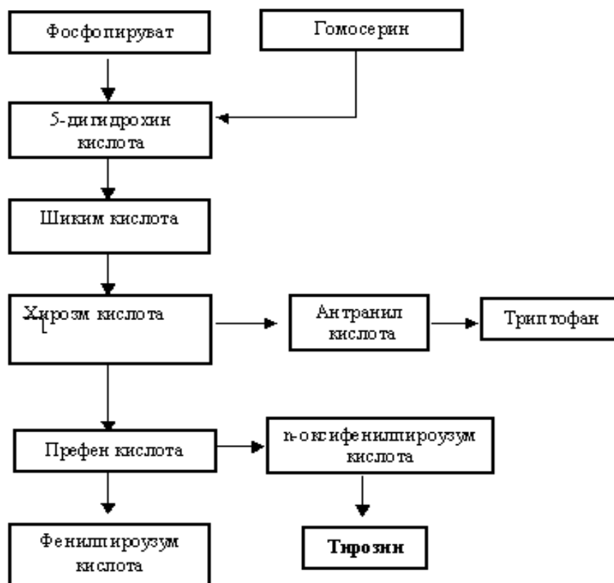
6.5-чизма. Триптофан, фенилаланин ва тирозин синтези
