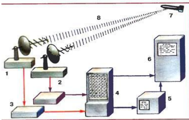
3.6-rasm. Radiolokatorning ishlash sxemasi.
