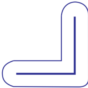
buferlangan chiziqlar
