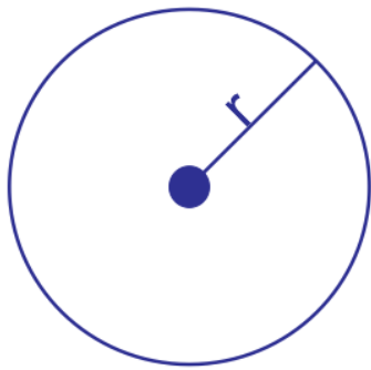
buferlangan nuqtalar
