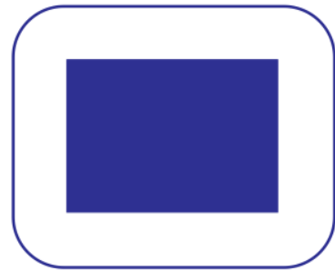
buferlangan maydonlar
