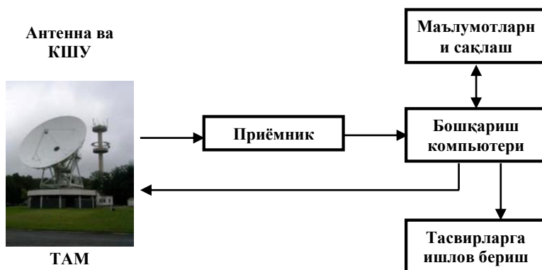
3.7-rasm. Yo'ldoshdan axborot qabul qilish stanstiyasining sxemasi.
