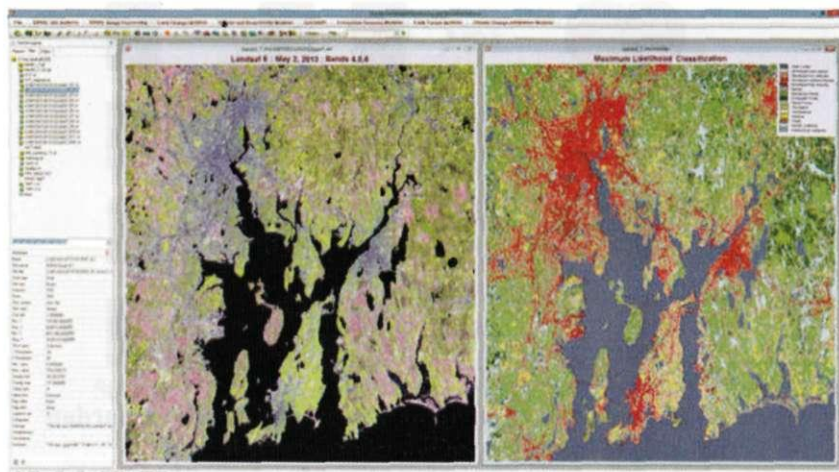
40-rasm. Landsat-8 olingan tasvir (a) va qaytadan kodlash orqali yerdan foydalanish turi ko'rsatkichi (b) uyalarga belgilandi
