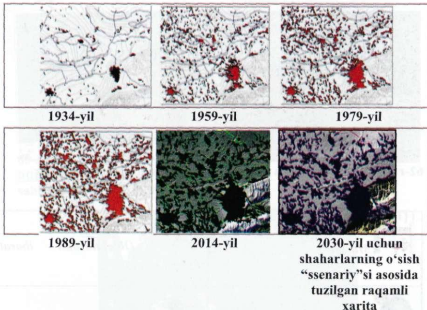
59 -rasm. Andijon viloyatida 1934-2014-yillardagi shaharlarning hududiy o'sishi va 2030-yil uchun "ssenariyi" raqamli xaritalar.
