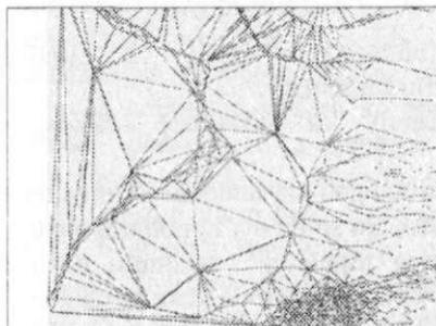
19-rasm. Andijon viloyati uchun tuzilgan balandlik nuqtalarini birlashtiruvchi uchburchaklar
