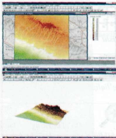
61-rasm. Joyning uch o'lchovli raqamli modeli TIN interpolatsiya usuli orqali tuzilgan
