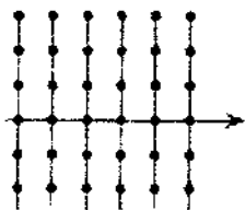
(4) Ko'ndalang kesma
