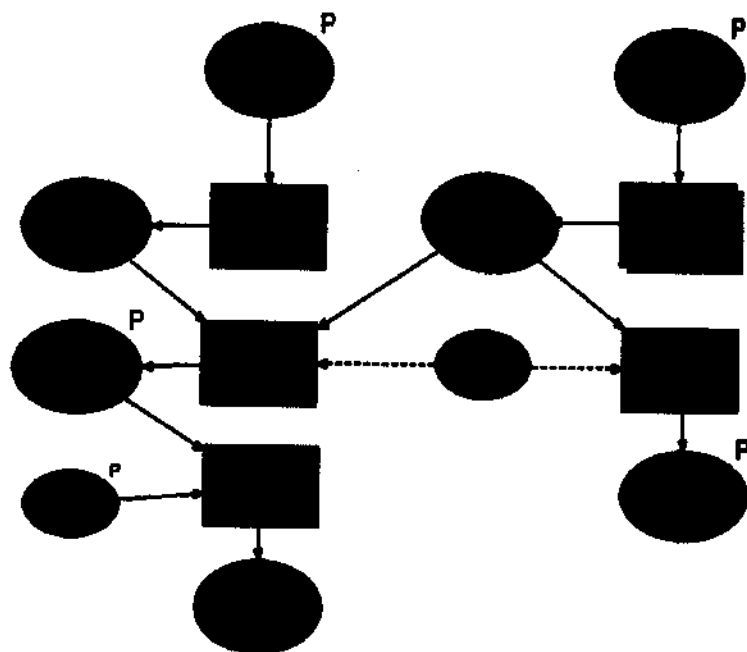
Modellashtirish algoritmi
