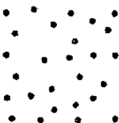
(2) Tasodifiy nuqtalar
