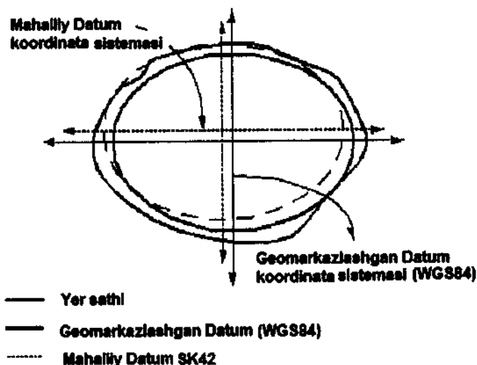
2.3-rasm. Mahalliy va umumjahon datumlari orasidagi farq (manba: Internet)
