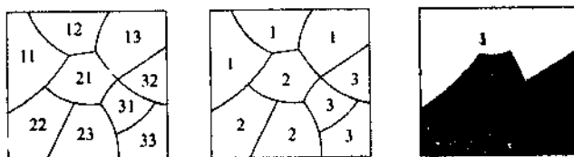
(a) Generalizatsiya
