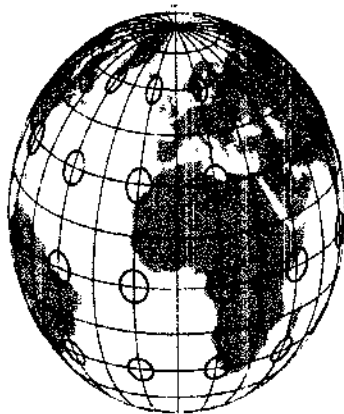
2.5-rasm. Geografik koordinatalarning sferik (chapda) va dekart (o'ngda) ko'rinishi (manba: Internet)
