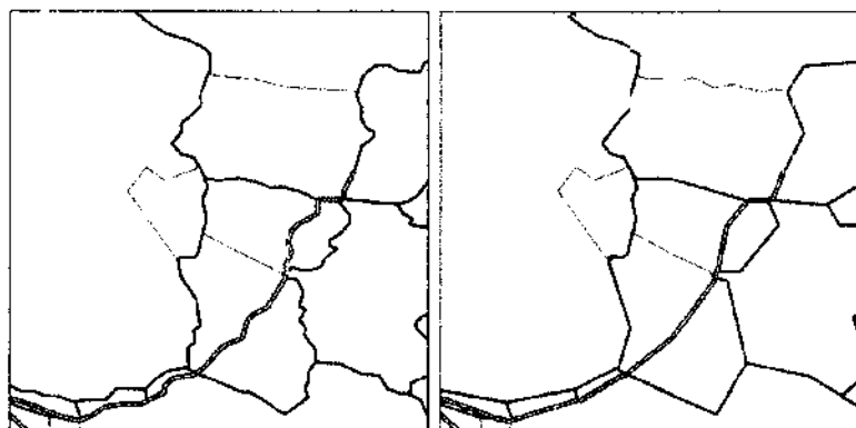
Generalizatsiyadan oldin
