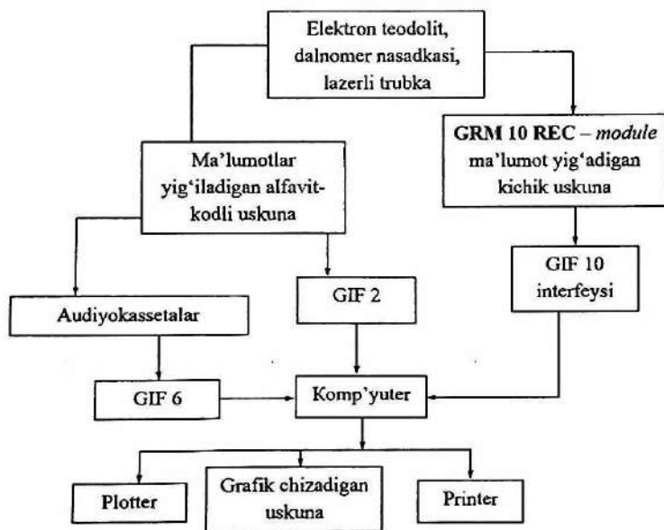
11.11-rasm. Lazerli elektron geodezik asboblarning ishlash tamoyili
