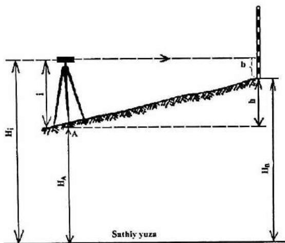
10.1-rasm. Olg'a nivelirlash
