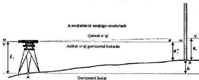
a) A nuqtadan B nuqtachacha nivelirlash.
