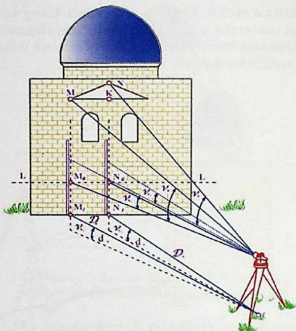
11.30-rasm. Binolarning tik tekislikda joylashgan qiya holatdagi elementlarining o'lchamlarini aniqlash
