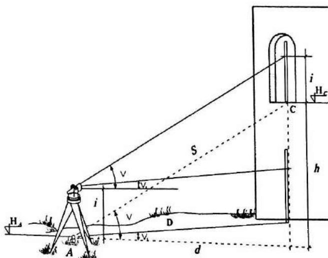
11.27-rasm. Trigonometrik nivelirlash usulida nuqtalarning o'tmetkalarini aniqlash
