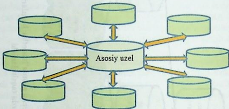
6.2-rasm. Replikalarning asosiy uzal yordamida sinxronlashtirilishi
