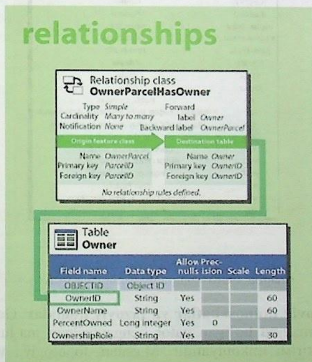
3.3-rasm. Munosabatlar va ularning xususiyatlari (manba: ESRI kompaniyasining Veb-sayti)
