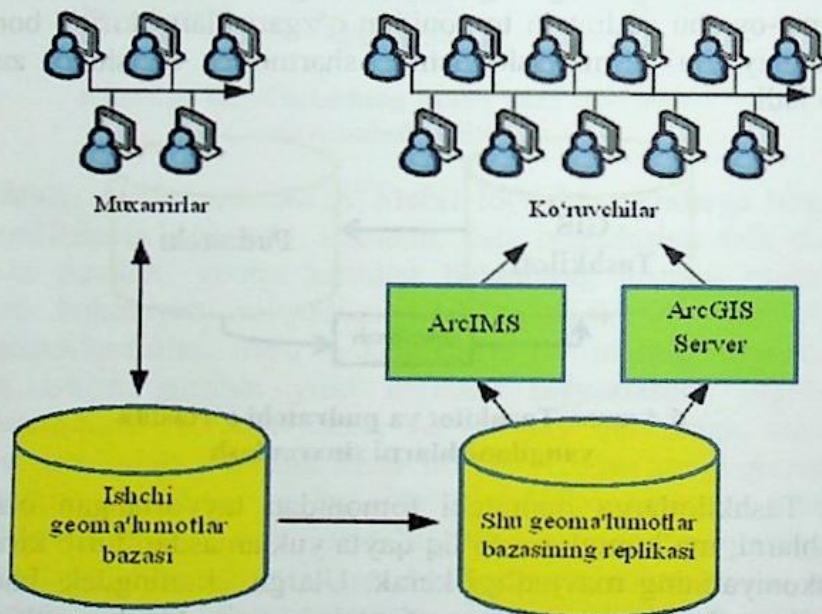
6.5-rasm. Har bir guruhga kirish imkoniyatini ta'minlash uchun tashkilot ArcSDE geoma'lumotlar bazasi
