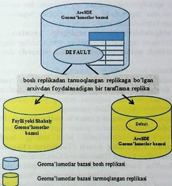
6.13-rasm. ArcSDE geoma'lumotlar bazalari o'rtasida bosh replikadan tarmoqlangan replikaga bo'lgan bir taraflama replika ko'rinishi
