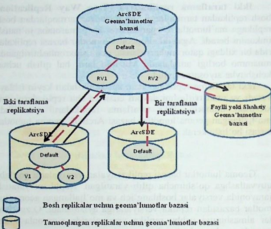
6.1-rasm. Bir taraflama va ikki taraflama replikalar uchun versiyalar
