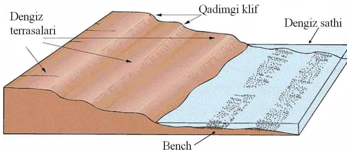
67-rasm. Dengiz terrasasi
