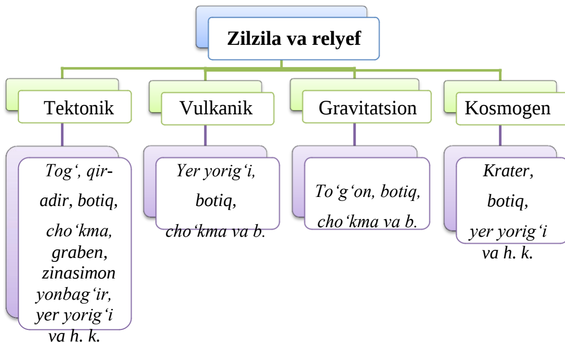
9-chizma. Tabiiy zilzila natijasida kelib chiqqan relyef shakllari
