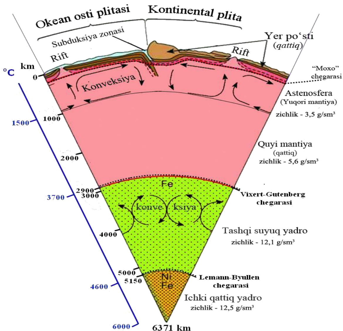
2-rasm. Yerning ichki tuzilishi
