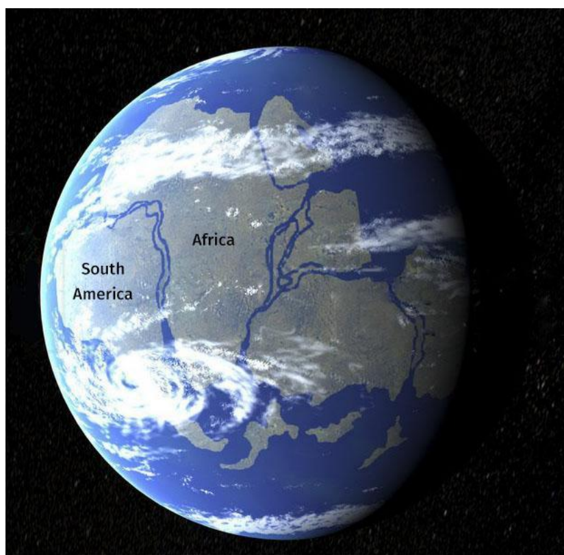
20-rasm. Pannotiya supermaterigi
