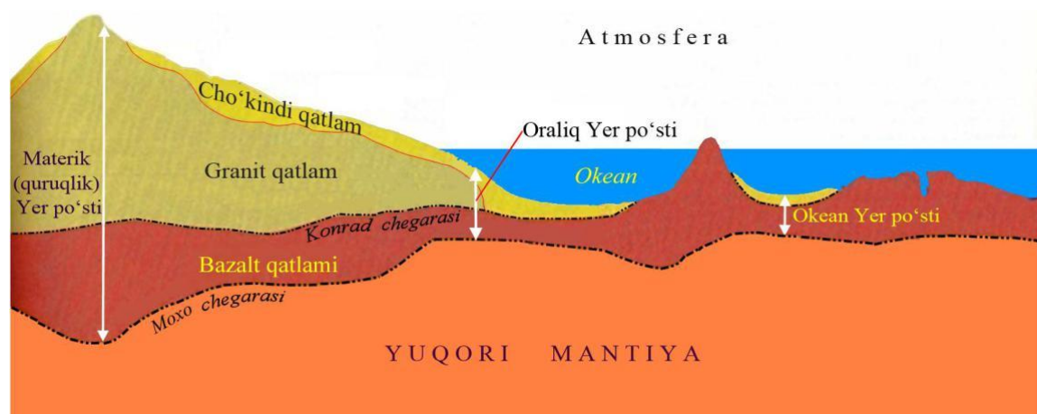
3-rasm. Yer po'sti turlari va qatlamlari
