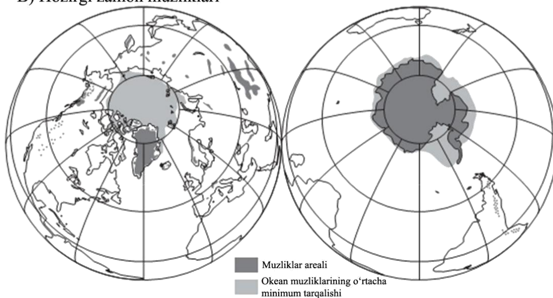
59-rasm. Muzliklarning tarqalishi
