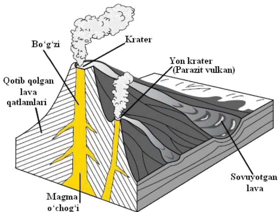
35-rasm. Markaziy turkumidagi vulkan va uning tuzilishi
