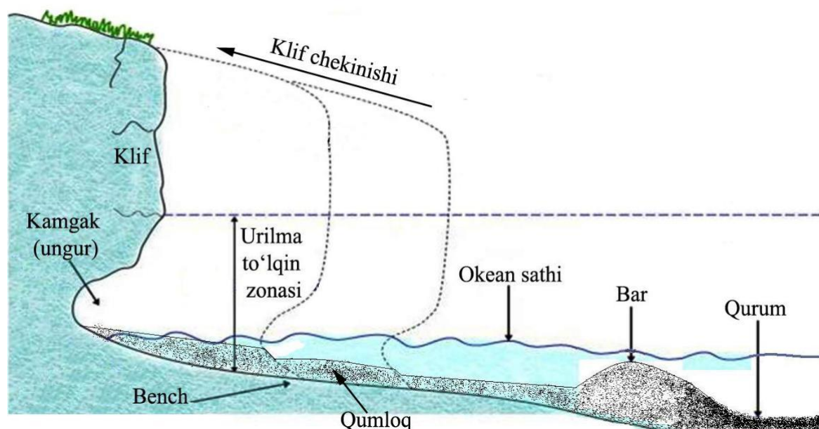
64-rasm. Qirg'oqning morfologik elementlari
