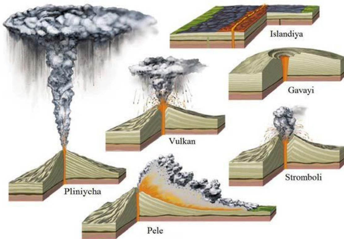
36-rasm. Vulkan turlari
