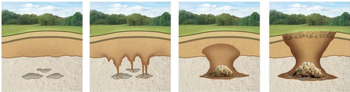
49-rasm. Tabiiy suffoziya jarayoni evolyutsiyasi
