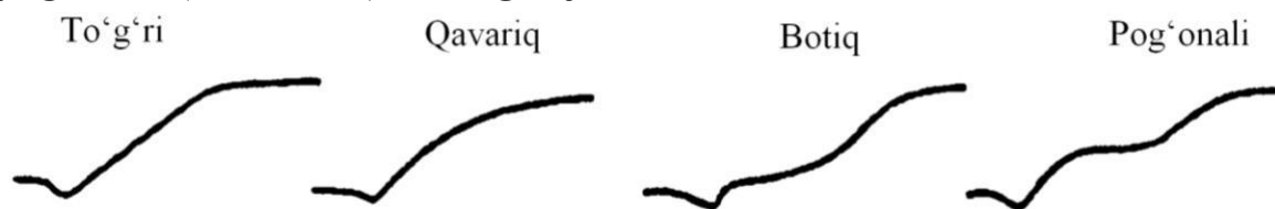
41-rasm. Yonbag'irning shakliga ko'ra turlari
