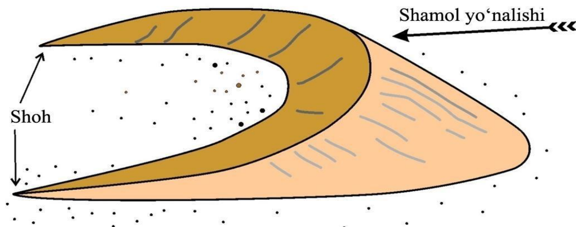
58-rasm. Barxan tuzilishi
