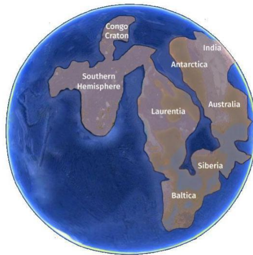
18-rasm. Kolumbiya supermaterigi
