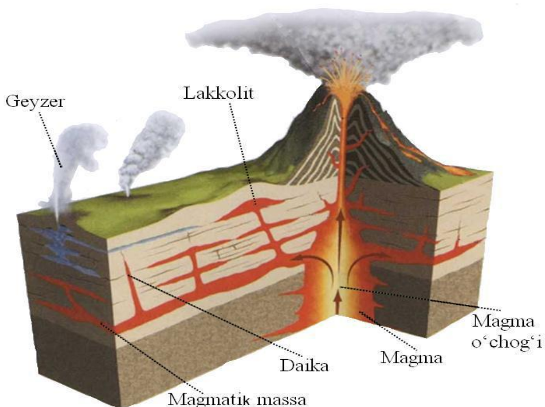
31-rasm. Lakkolitning paydo boʻlishi
