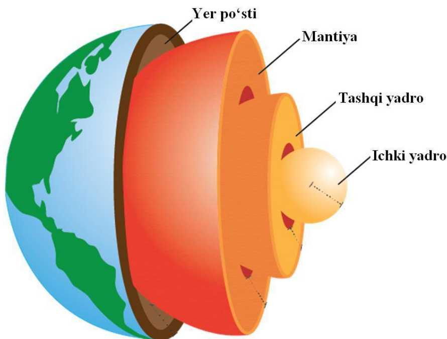
1-rasm. Yerning ichki tuzilishi
