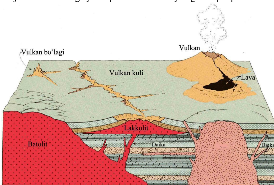
30-rasm. Batolit va lakkolitlarning paydo bo‘lishi
