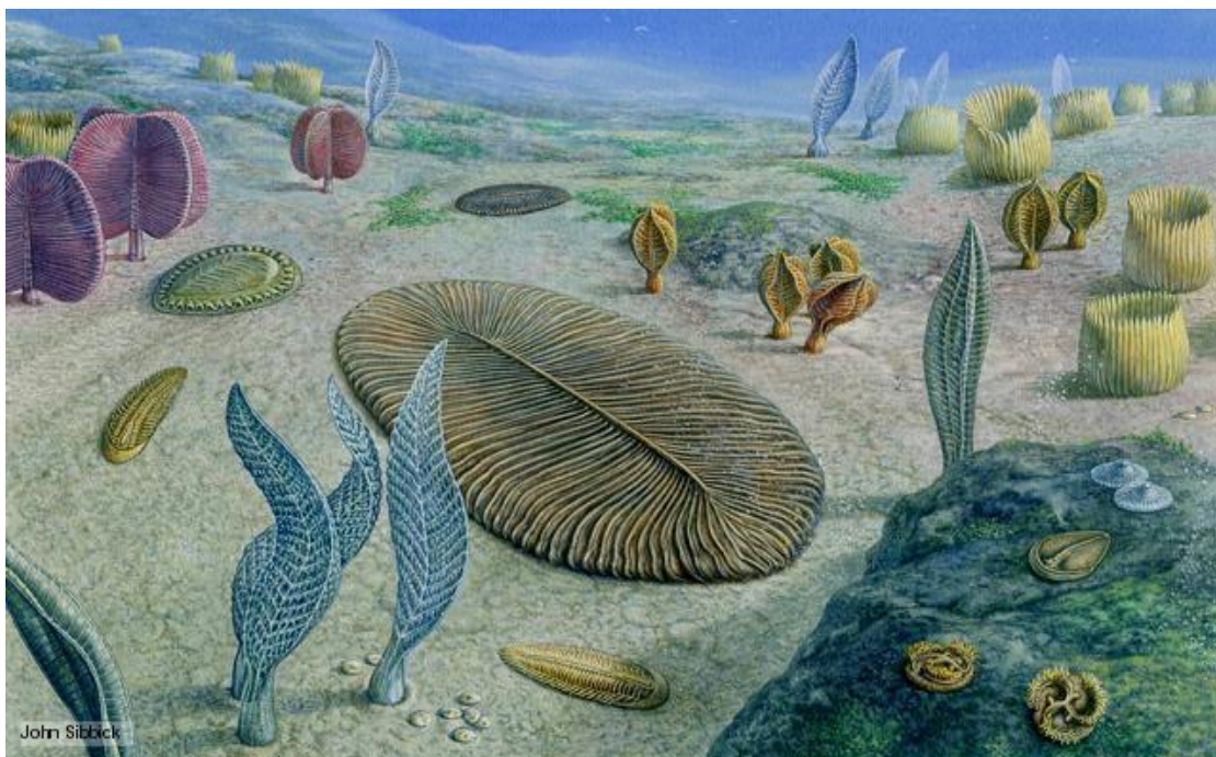
21-rasm. Edikariy davri organizmlari
