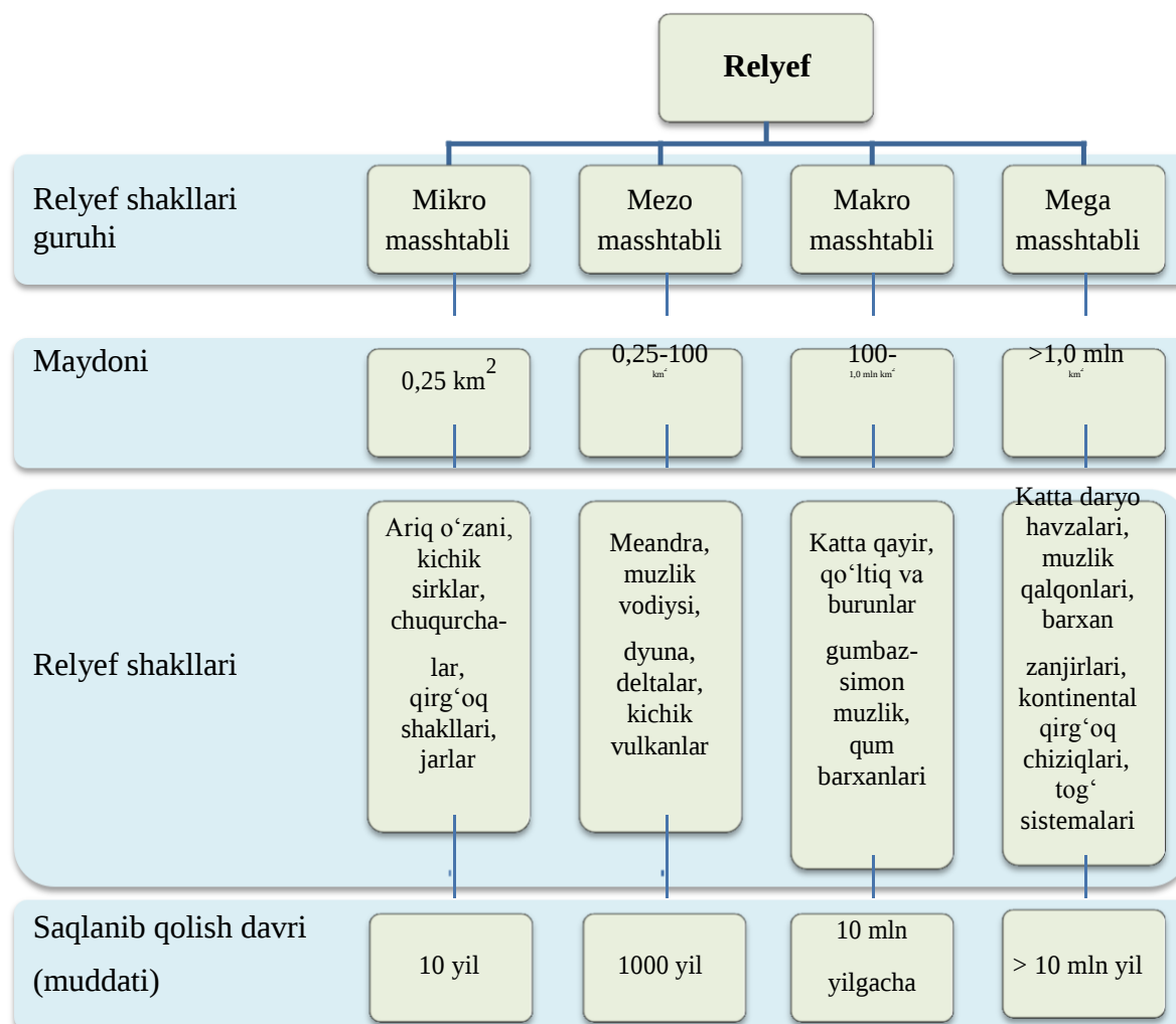
5-chizma. R.J.Xagget bo'yicha relyef shakllarining katta-kichikligi bo'yicha tavsifi
