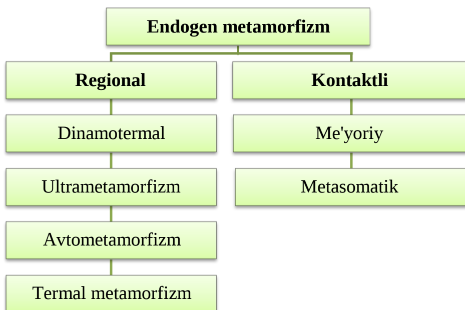
10-chizma. Metamorfizm turlari
