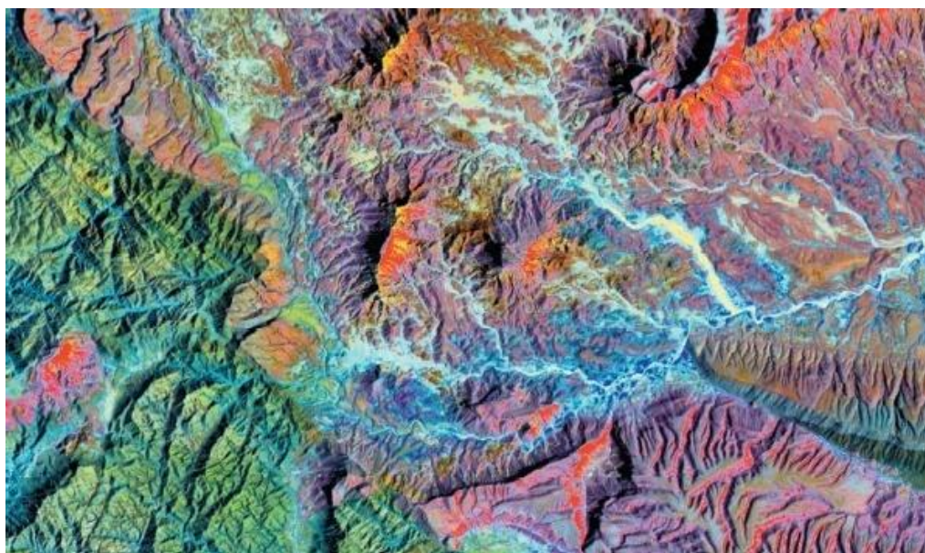
3.4-rasm. Yaman davlatidagi ma’lum bir maydonning Landsat TM murakkab rangli (RGB=457) tasviri.
