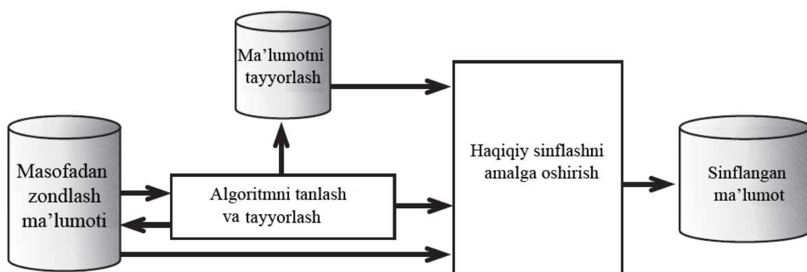
7.6-rasm. Sinflash jarayoni.
