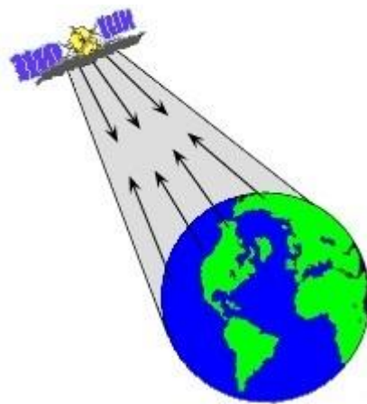
2.7-rasm. Aktiv masofadan zondlash.
