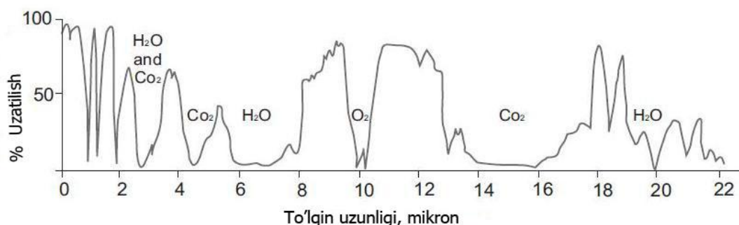
2.12-rasm. Atmosferik uzatilish foizlarda keltirilgan.
