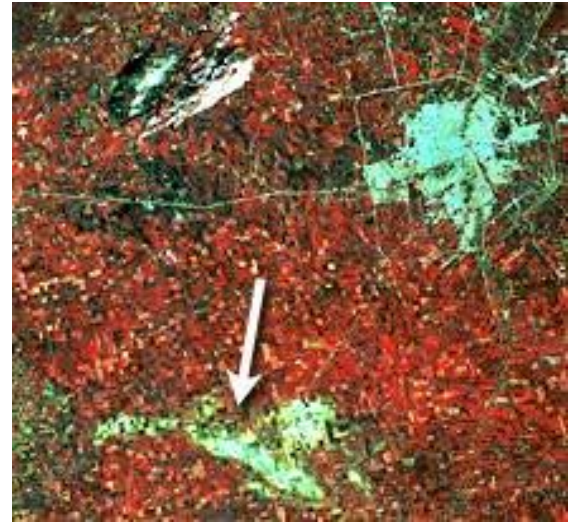
8.3-rasm. (a) Ekin turi va (b) zararlangan ekinlarni aniqlash uchun Landsat-TM va SAR ma'lumotlari birlashtirilgan.
