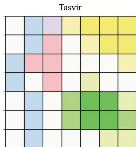
7.15-rasm. Aralash piksellar: turli yer qoplami turlari bitta pikselga tushadi.
