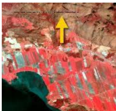
6.4-rasm. Skanerlash chizig‘ining tushirib qoldirilishi.
