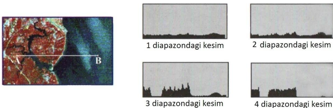
6.12-rasm. Ko'p spektrli tasvirning kesimi.
