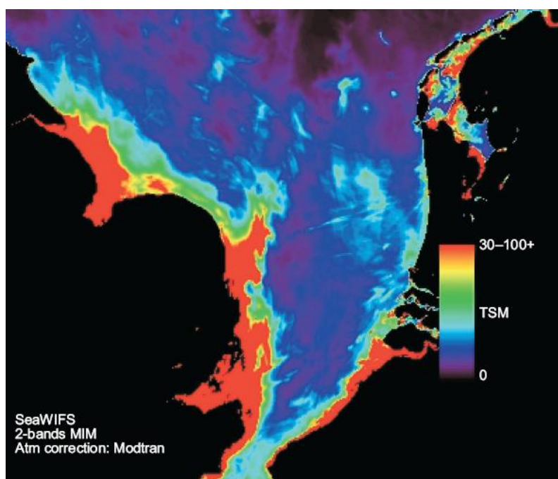
3.5-rasm. Shimoliy dengizda to'plangan fizik moddaning umumiy konsentratsiyasi, SeaWiFS (Orb-View2) sun'iy yo'ldosh ma'lumotidan olingan.
