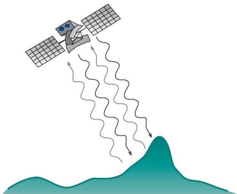
4.1-rasm. Aktiv mikroto‘lqinli masofadan zondlash tamoyillari.
