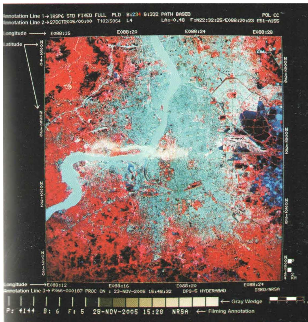
5.6-rasm. NRSA tomonidan berilgan fotografik mahsulot.
