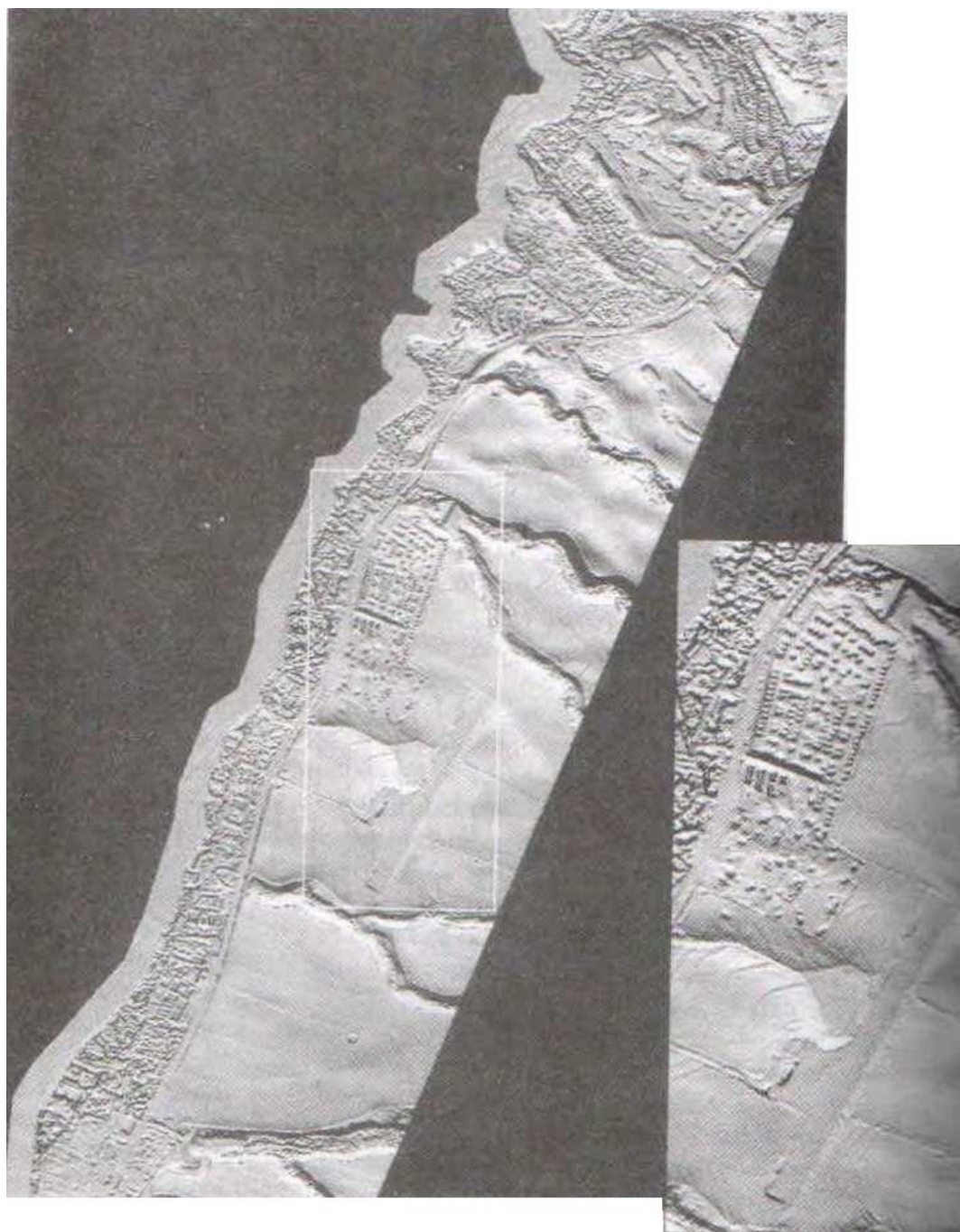
4.10-rasm. Leica Geosystems ALS-40 Havo lazer skanerli ma'lumotdan olingan soyali relyef DEM (Balandlikning raqamli modeli), G'arbiy Maui, Gavay. 1:40000 masshtab (asosiy tasvir), 1:24000 masshtab (alohida qismi).
