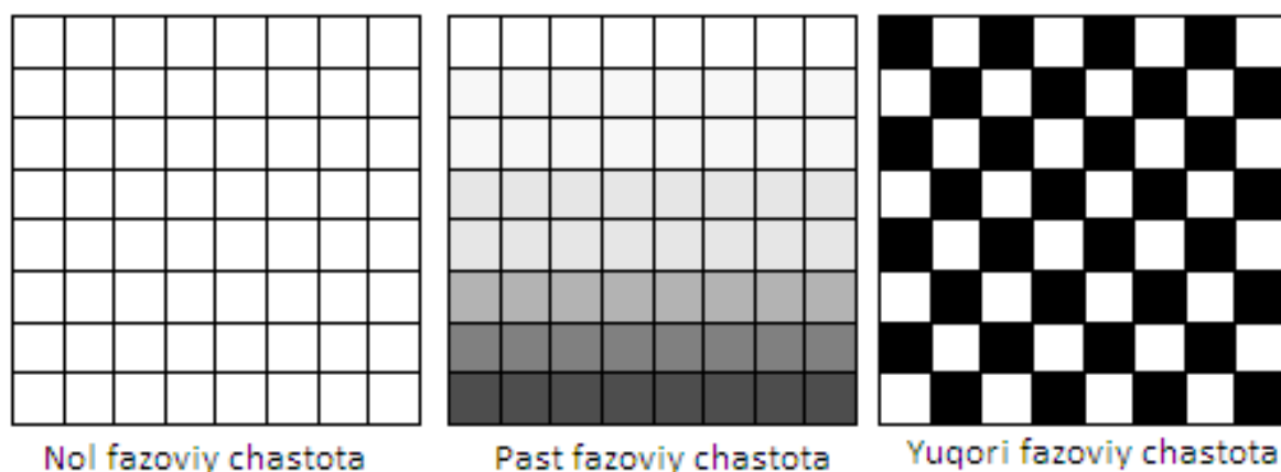
6.15-rasm. Nol fazoviy chastota, past fazoviy chastota va yuqori fazoviy chastotaga namunalar.
