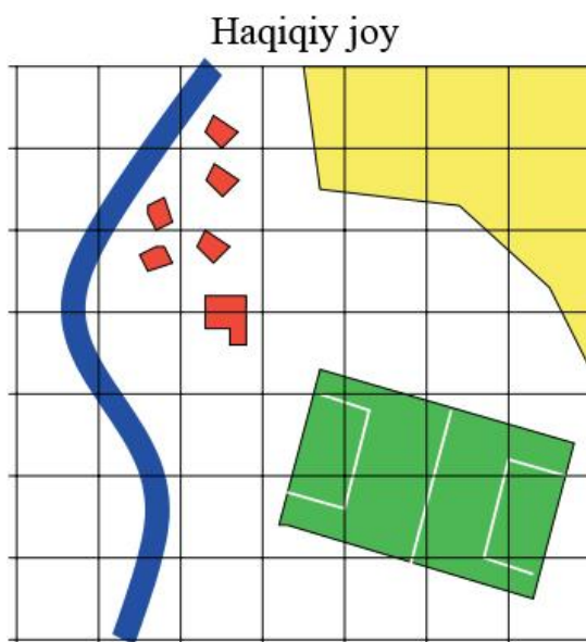
7.15-rasm. Aralash piksellar: turli yer qoplami turlari bitta pikselga tushadi.
