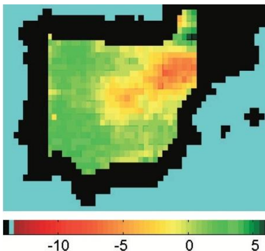
3.7-rasm. Iberey yarim orolining 10 yil mobaynida tuproq namligining o‘zgarish kartasi.
