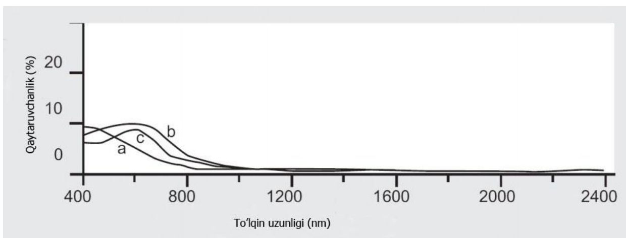
2.17-rasm. Xlorofill va loyqaning suvni qaytaruvchanligiga ta'siri: a) okean suvi; b) loyqa suv; c) xlorofilli suv.
