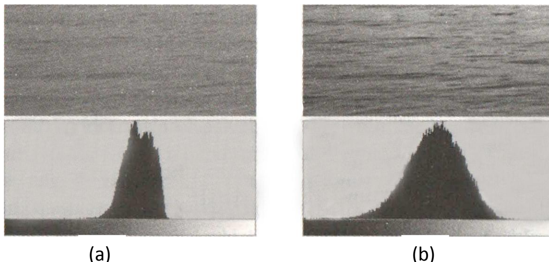
6.14-rasm. Qisqa grafik past kontrastni (a) va keng grafik esa yuqori kontrastni (b) anglatadi.
