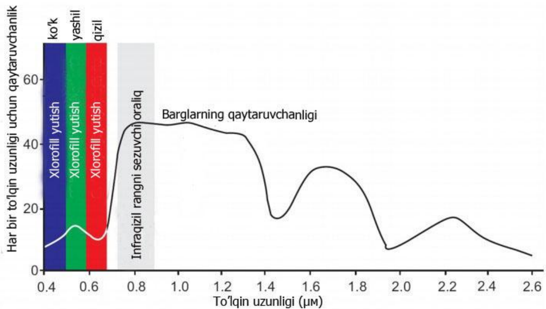
2.15-rasm. Sog‘lom o‘simlikning qaytarish egri chizig‘i.
