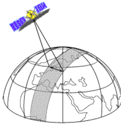
3.14-rasm. Sensorning Yerni egallash kengligi.
