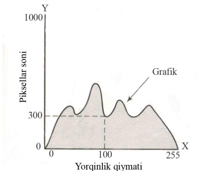
6.13-rasm. Tasvirning grafigi.
