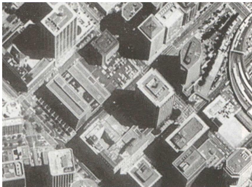
6.13-rasm. Tasvirda qo‘shni binolarning nisbiy balandligi keltirilgan.
