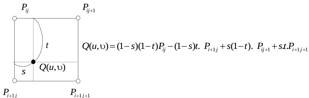
6.10-rasm. Ikki chiziqli interpolyatsiya.
