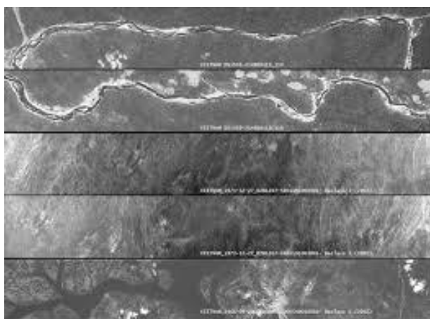
6.3-rasm. Tasvirda yo‘laklarning hosil bo‘lishi.
