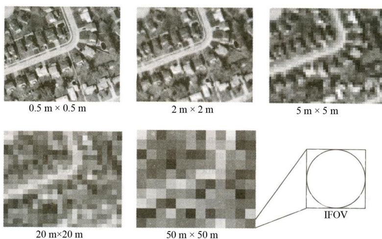
3.17-rasm. Fazoviy imkoniyat kamaysa ma’lumotlar batafsilligi kamayadi.
