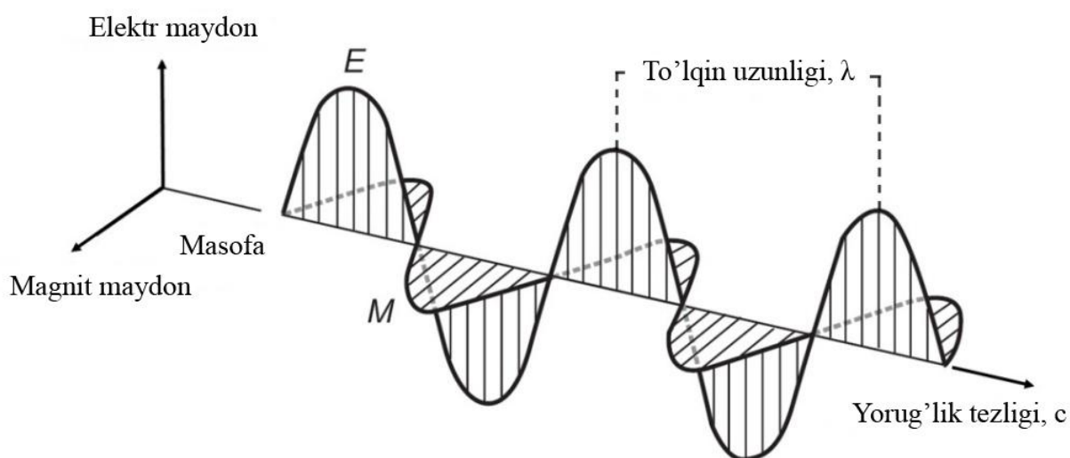
2.2-rasm. Elektromagnit to‘lqinning elektr ( E ) va magnit ( M ) maydoni.
