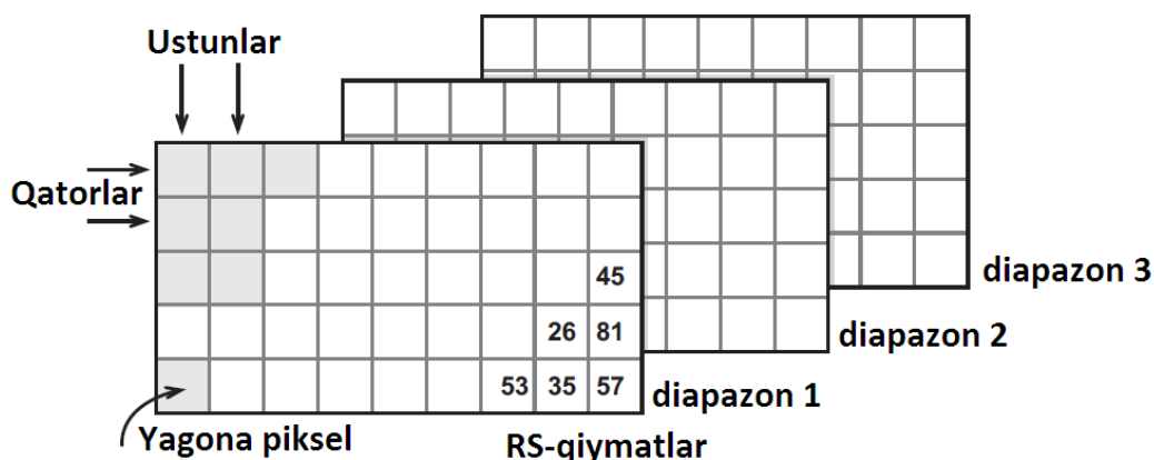
7.1.-rasm. Ko‘p diapazonli tasvirning tuzilmasi.
