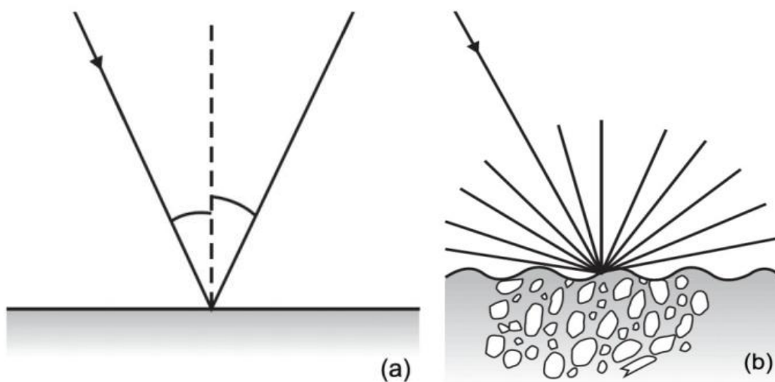
2.14-rasm. (a) ko'zguli va (b) tarqoq qaytishning sxematik diagrammasi.
