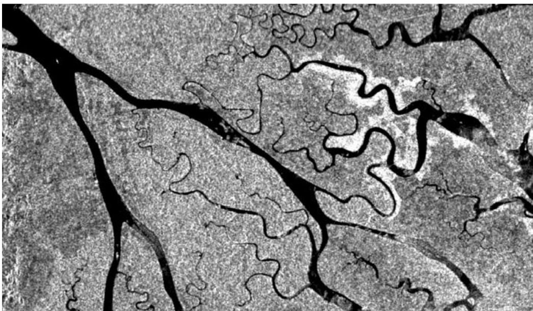
3.10-rasm. Indoneziyaning Kalimantan viloyatidagi daryoning ERS SAR tasviri. Tasvir uch xil o‘rmon turlarini farqlash imkoniyatini beradi.
