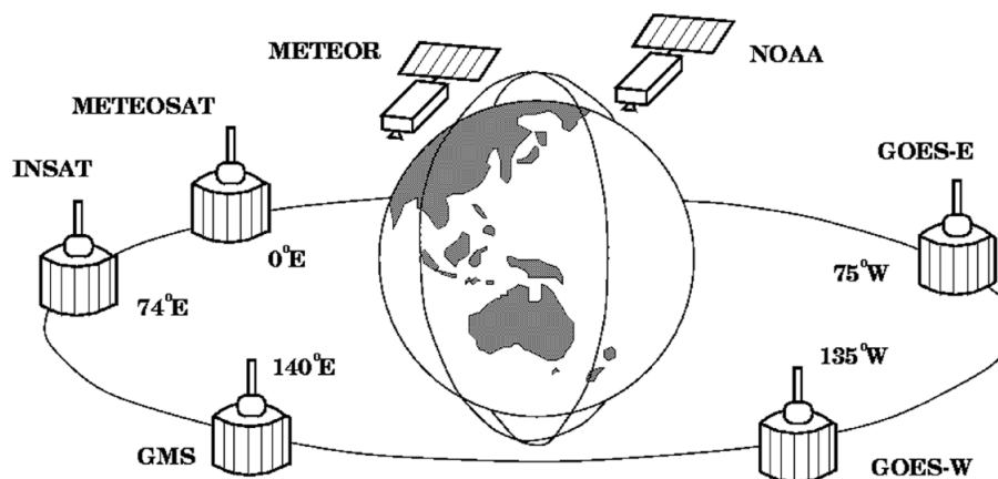
3.13-rasm. Geostatsionar va qutbiy sunʼiy yoʻldoshlardan tashkil topgan meteorologik kuzatish tizimi.
