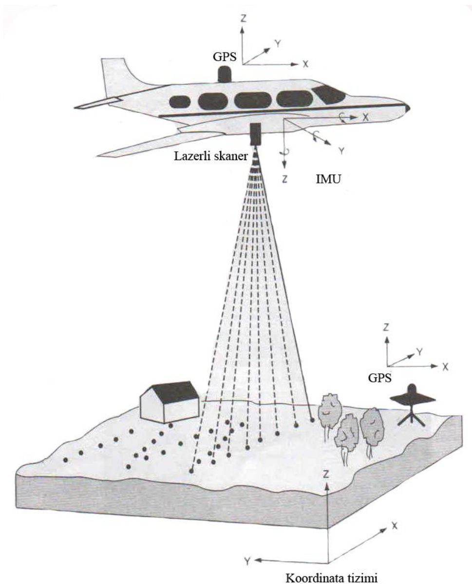
4.9-rasm. Havodan lidar skanerlash tizimining tarkibiy qismlari.
