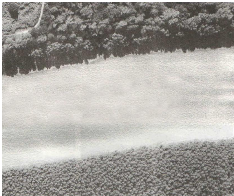
5.12-rasm. Yuqoridagi dag‘al tekstura baland daraxtlarni, pastdagi o‘rtacha tekstura kichik va yosh daraxtlarni, o‘rtadagi tekis tekstura esa qurigan daryoni tasvirlaydi.
