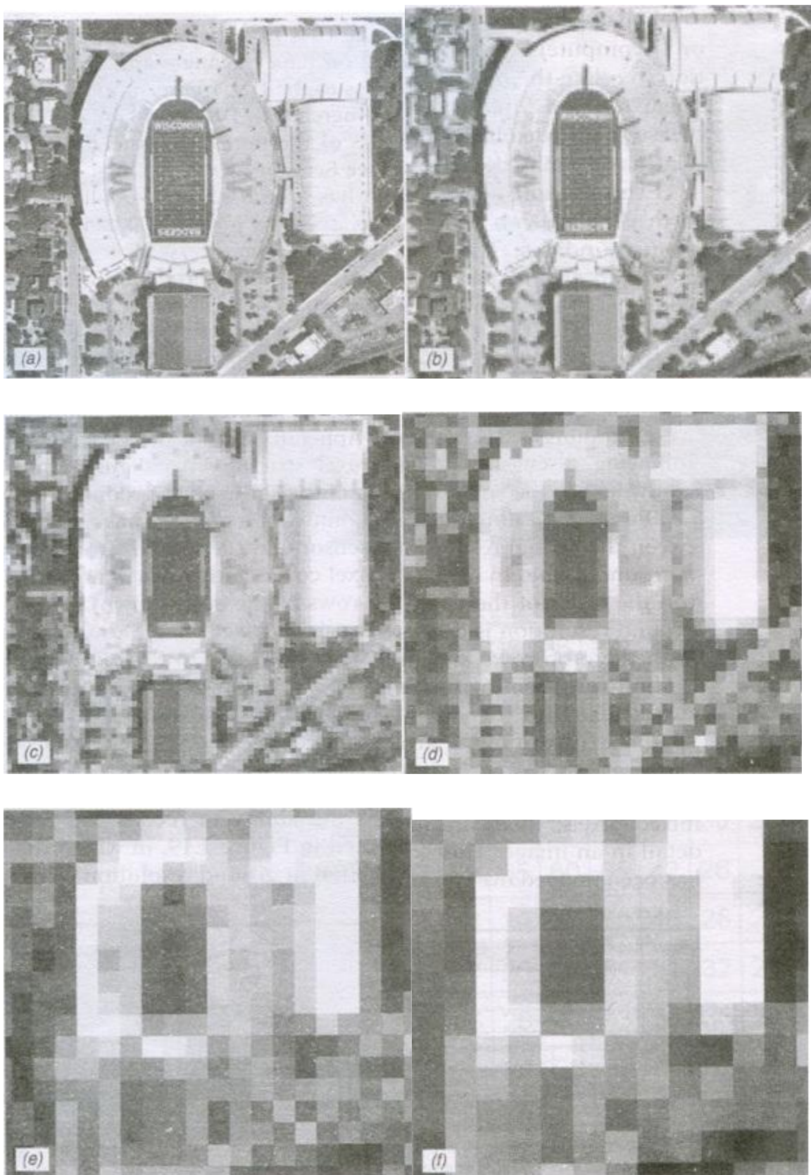
2.2-rasm. Joy imkoniyati katakchalari o'lchamining raqamli tasvirdagi tafsilotlarni ajratib olishga ta'siri. Viskonsin–Madison universiteti kampusining bir
