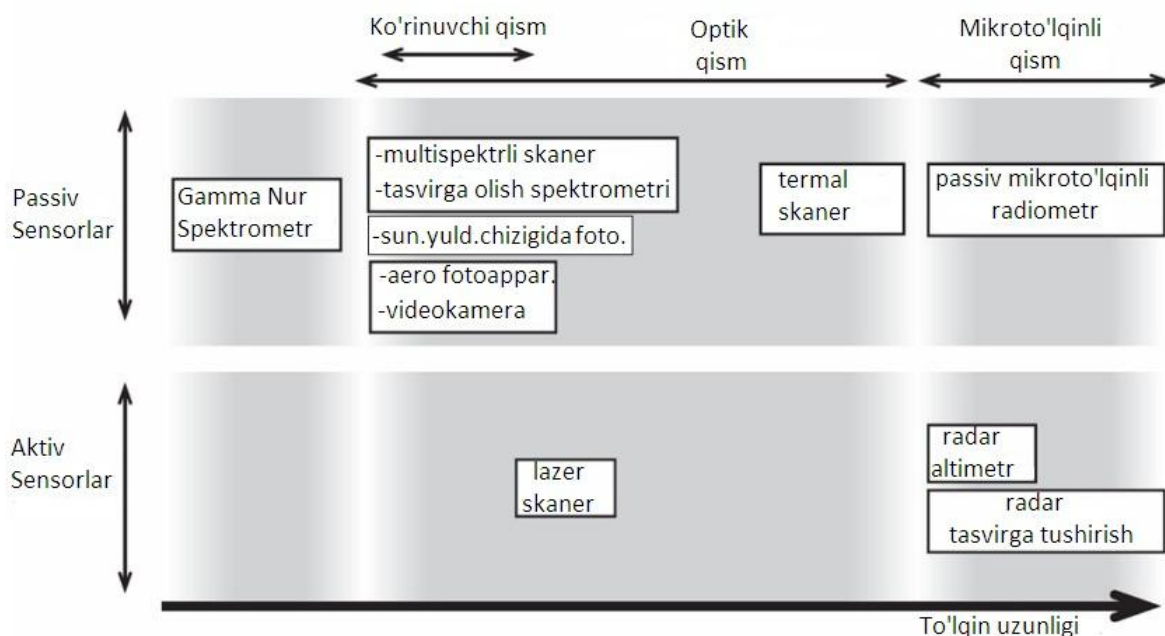
3.1-rasm. Sensorlarning turlari.
