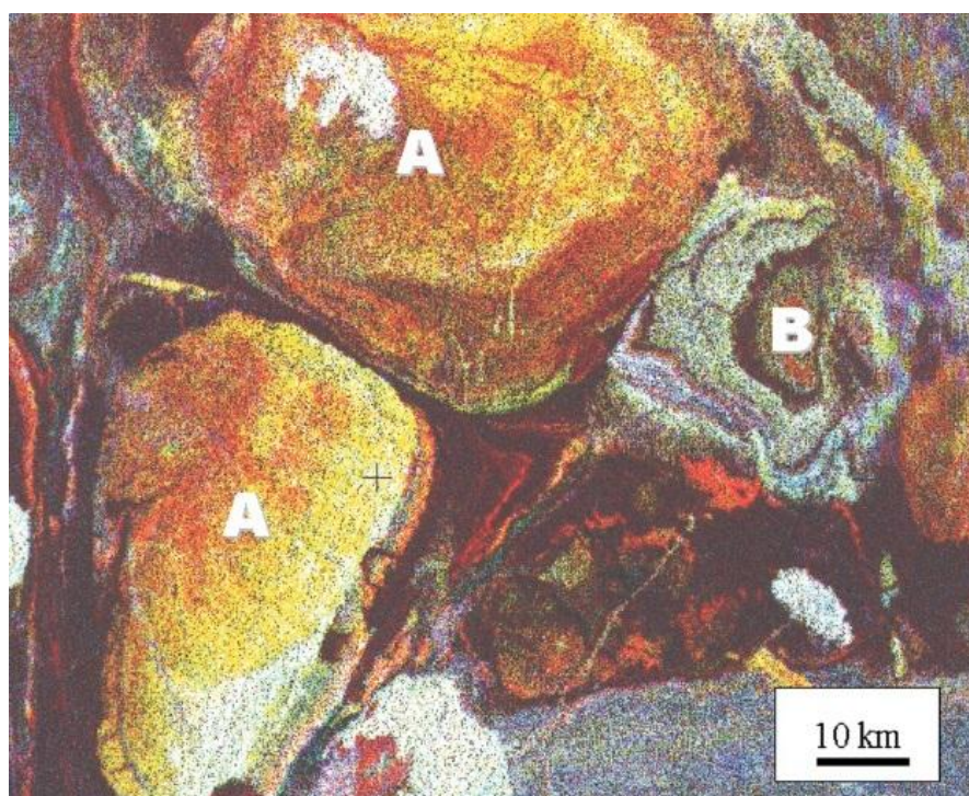
3.2-rasm. Gamma-nur spektrometri orqali olingan tasvir.
