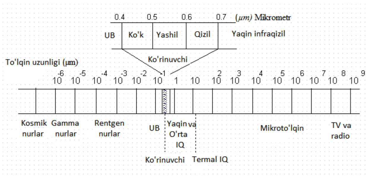
2.5-rasm. Elektromagnit spektr.
