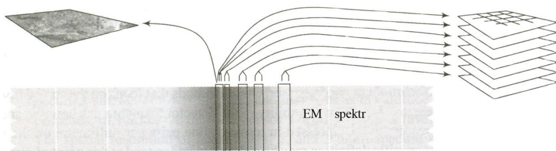
3.18-rasm. Panxromatik va ko'p spektrli tasvirning spektrli imkoniyati.
