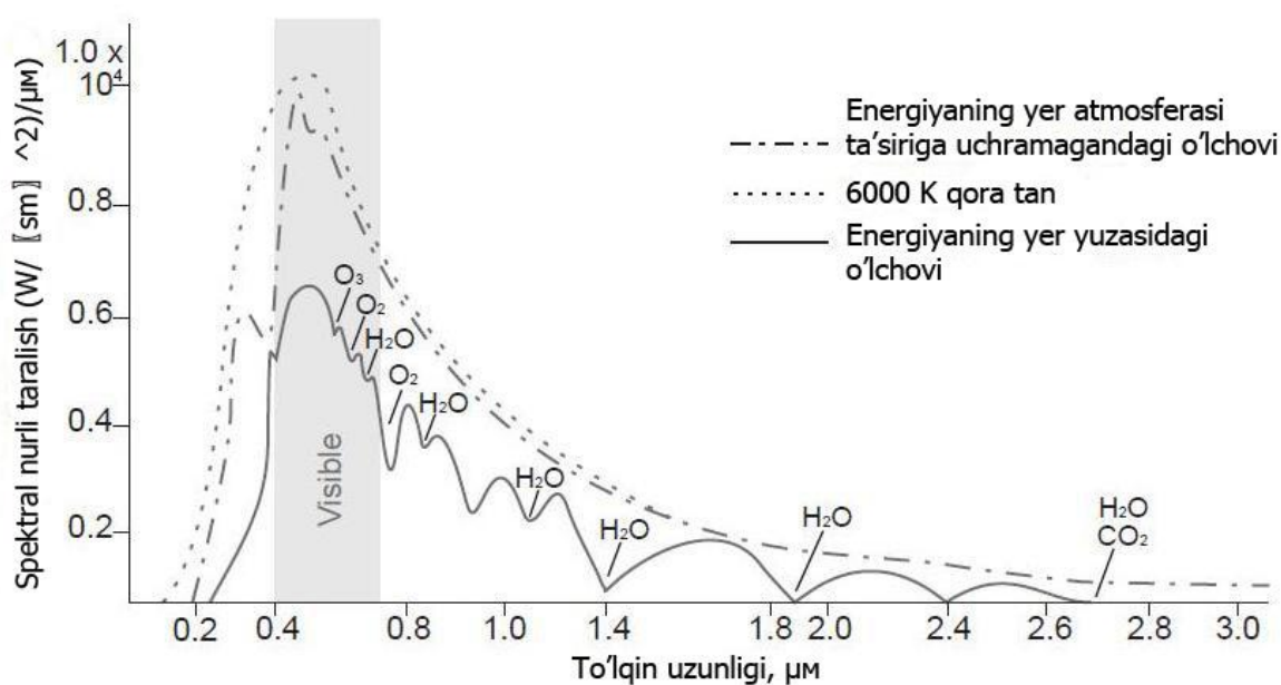
2.13-rasm. Quyoshning elektromagnit spektrni Yer atmosferasi ta'siri bo'lgan va bo'lmagan holatlaridagi kuzatishlar.
