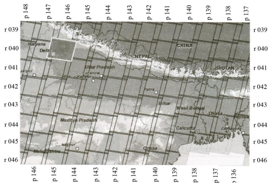
3.22-rasm. Landsat-TM sunʼiy yoʻldoshining yoʻlak-qator bogʻlash tizimi.
