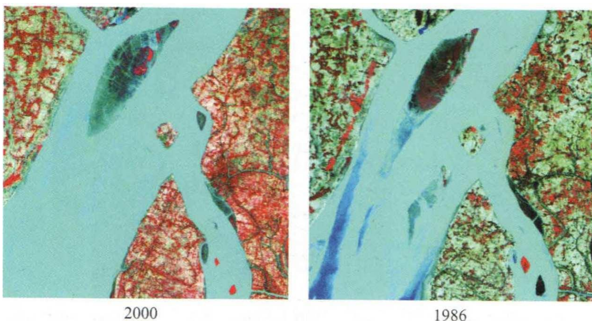
8.2-rasm. Ganga daryosi qirg'og'idagi yer qoplaminig o'zgarishi.
