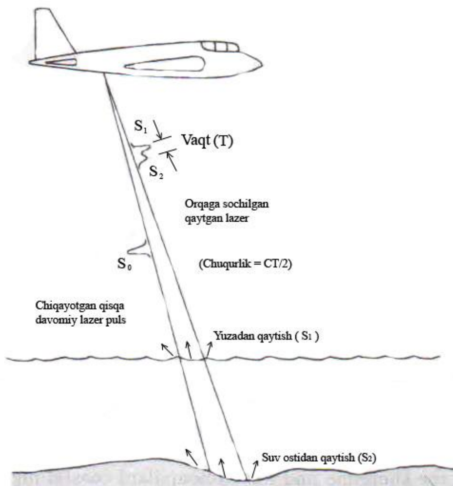
4.8-rasm. Lidar batimetriya (chuqurlikni o'lchash) tamoyillari
