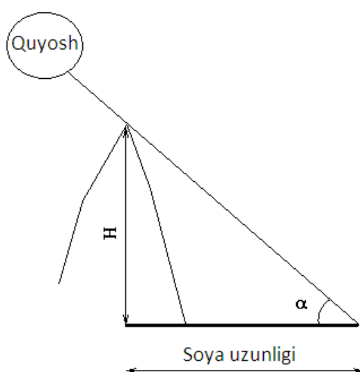
5.10-rasm. Soya uzunligiga asosan balandlikni hisoblash.
