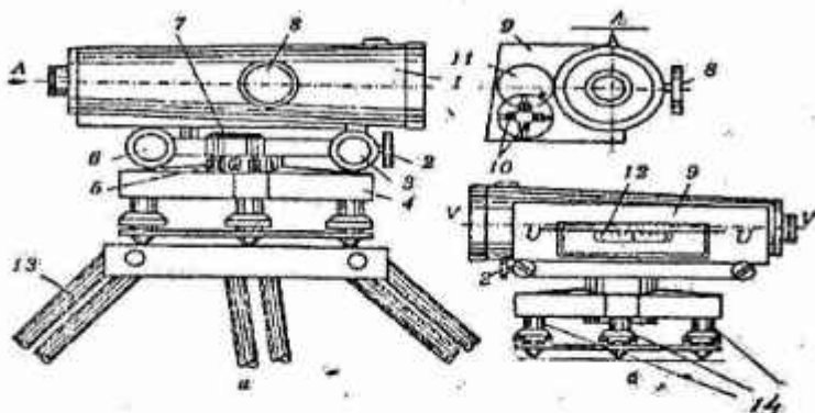
6.6-rasm. H3 niveliri tuzilishi
