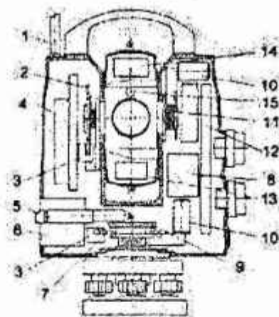
6.12-rasm. Elektron taxometr tuzilishi sxemasi
