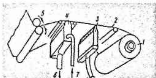
22.12-rasm. Elektrostatik bosma uskunaning ishlash chizmasi. 1-qog'oz ruloni, 2-qog'oz tasma, 3-elektrodlar, 4-bo'yovchi eritma, 5-qog'oz uzatish moslamasi, 6-ortiqcha bo'yoqning oqovasi, 7-bo'yoq berish moslamasi
