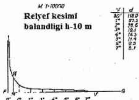
3.3-rasm. Quyilish mashtabi grafigi
