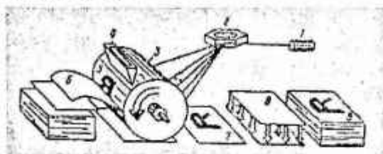
22.13-rasm. Elektronografik (lazer) printyerlarning ishlash chizmasi.
