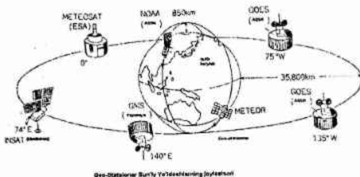
20.3-rasm. Yer shari atrofida harakatlanayotgan sun'iy yo'ldoshlar
