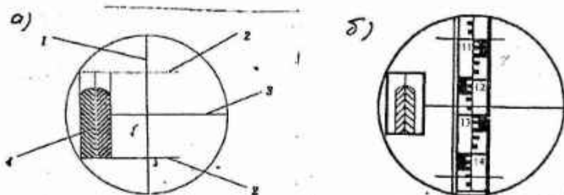
6.7-rasm. 1-verikal ip; 2-dalnomer iplari; 3- o'rta ip; 4- silindrik adilak pufakchasinig uchlari ,bir-biriga to'g'ri keltirilgan (kontakt) holati; 6) qarash trubasida reyka tasviri
