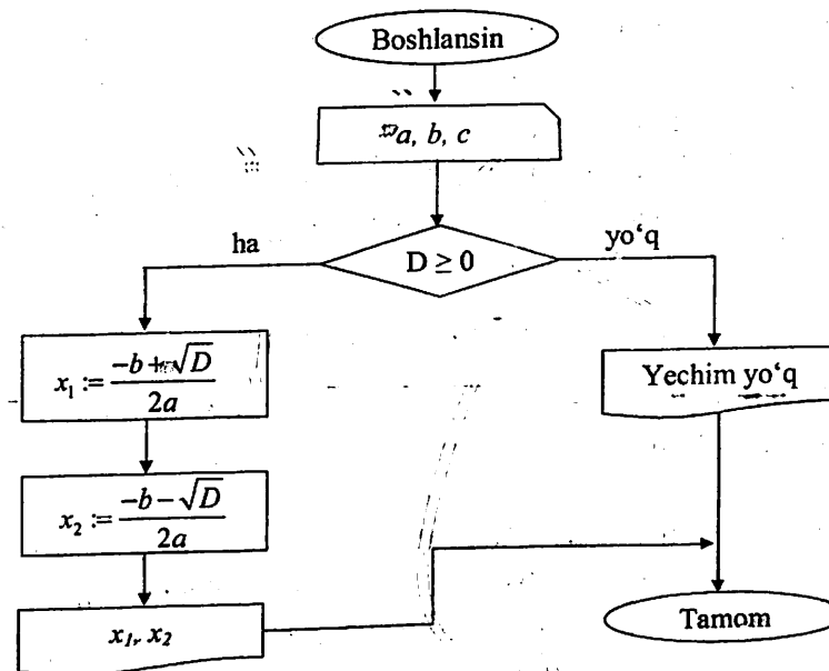
1-rasm. Kvadrat tenglama uchun blok-sxema.
