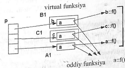
22-rasm Virtual funksiya.
