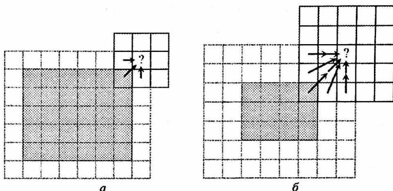
5.30-расм. Рақамли филтрациялашда четки узеллар муаммоси
