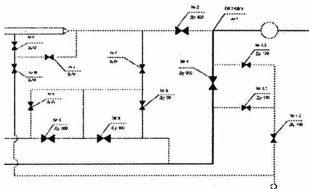
8.1-расм. Газ қувири участкаси технологик схемасининг наъмунаси
