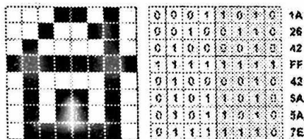
3.9-расм. Энг содда растрли тасвир
