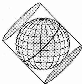
2.14-расм. Қиялама проекцияга мисол
