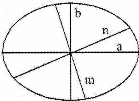
2.9-расм. Эллипснинг бузилиши
