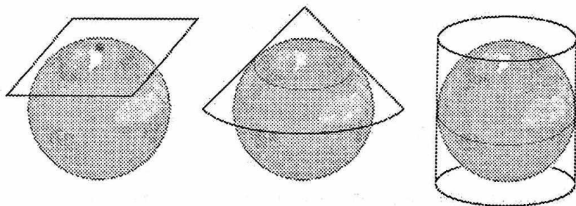
2.13-расм. Кўндаланг проекцияларга мисоллар:
