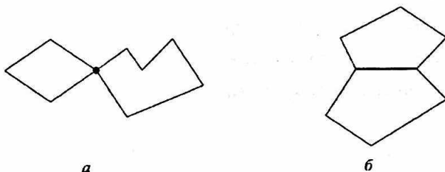
3.15-расм. Объектлар ўртасидаги топологик боғланишларга мисоллар
