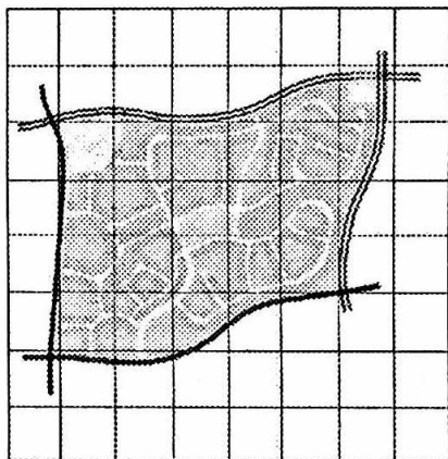
3.7-расм. Шаҳар ҳудуди фрагментини тўғрибурчаклар тўрига бўлиб чиқиш
