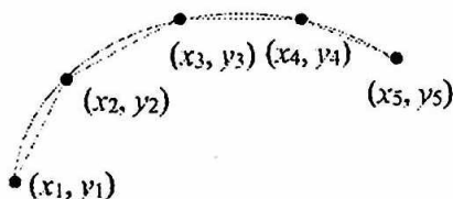
3.13-рasm. Объектни чизиқли кесимлар билан аппроксимациялаш
