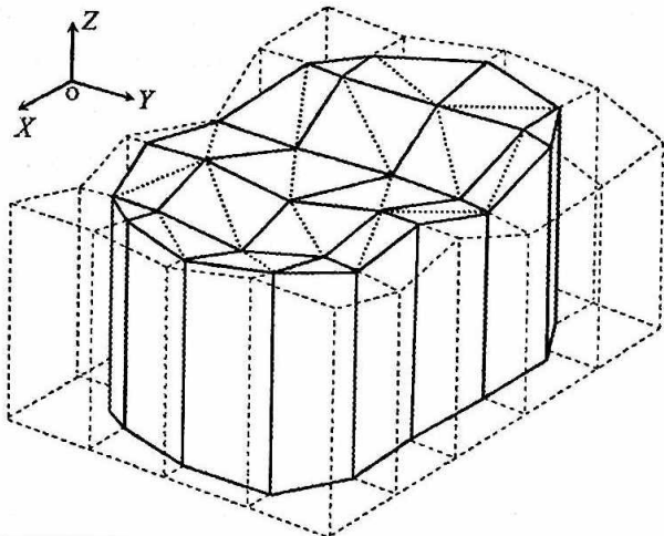
5.27-расм. Жисми кўпбурчаклар билан аппроксимациялаш
