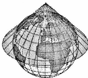
2.12-расм. Коник проекция. Уринма конус ҳолати
