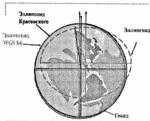
2.4-расм. Тик чизиқлар ва нормалларнинг референц-эллипсоид ва геоидга жойлашиши схемаси
