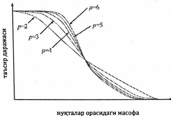
5.33-расм. Турли "р" лар учун таъсир кўрсатиш даражасининг бошланғич ва ҳисобланадиган нуқталар орасида масофага боғлиқлиги
