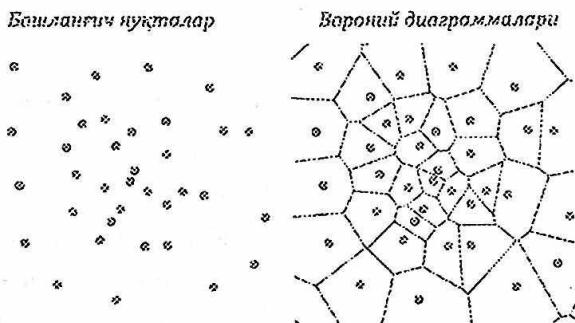
5.16-расм. Яқинлик зоналари
