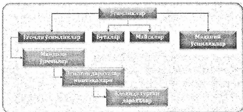
3.3-расм. Ўсимликларни таърифлаш учун маълумотларнинг объектга ориентирланган моделининг схемаси
