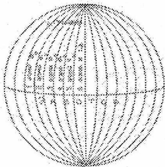
2.20-расм. Ер эллипсоиднинг қўп полосали тасвири схемаси
