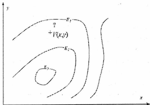
5.34-расм. Геомайдонни изолиниялар бўйича тиклаш
