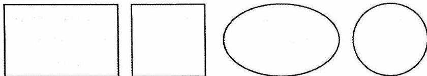
3.14-расм. Бир хил топологик хусусиятларга эга бўлган фигураларга мисоллар
