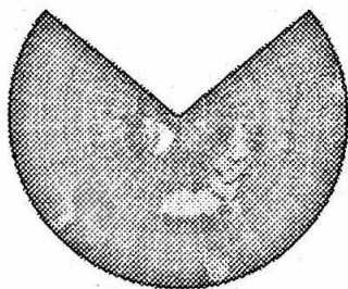
2.16-расм. Конус проекция
