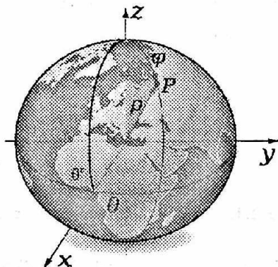
2.1.-расм. Красовский референц-эллипсоиди 1
