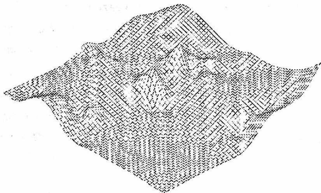
3.20-расм. Мунтазам тармоққа мисол
