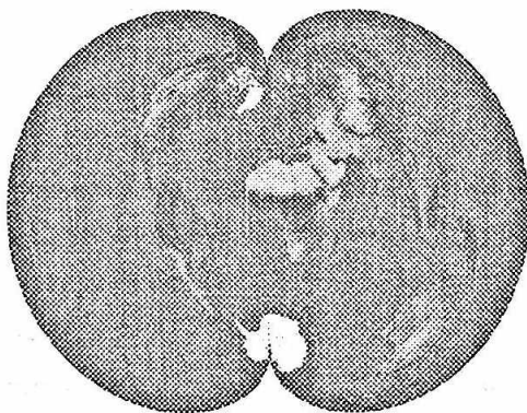
2.19-расм. Поликоник проекция
