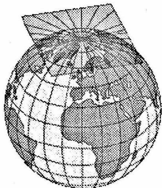
2.10-расм. Азимутал проекция Уринма текислик ҳолати
