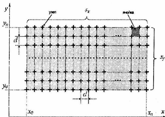
3.21-расм. Мунтазам тармоқ геометрияси
