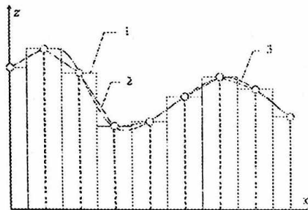
3.23-расм. Юза аппроксимацияси усулларини аниқлик бўйича таққослаш
