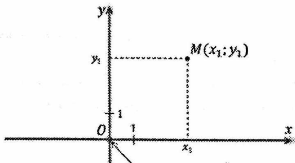
2.5-расм. M ва M' нуқталарнинг тўғри бурчакли координаталар тизимидаги ҳолати
