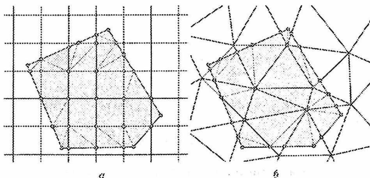
5.25-расм. Фигуранинг майдонини рельеф модели асосида аниқлаш а – мунтазам тармоқни қўллаб, б – триангуляция тармоғини қўллаб
