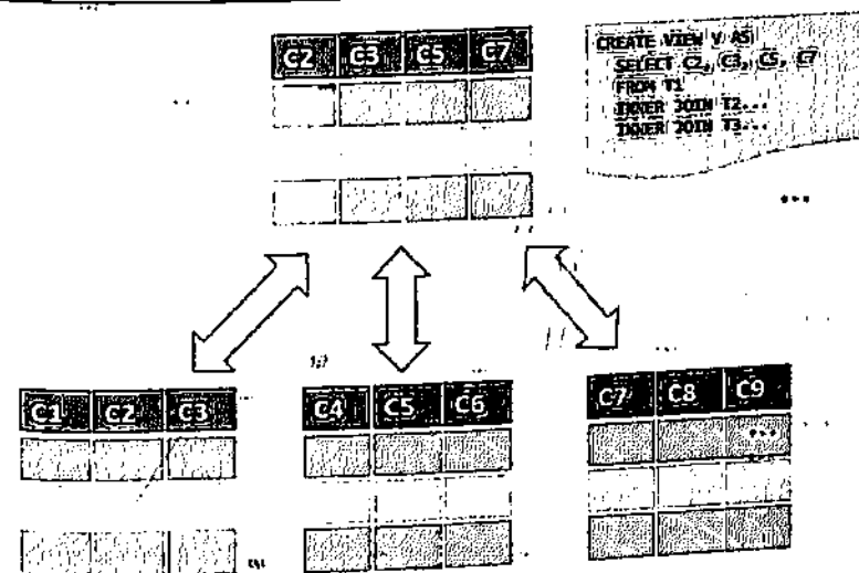
5.2.2-rasm. Tasavvurlarning tuzilmasiga namuna
