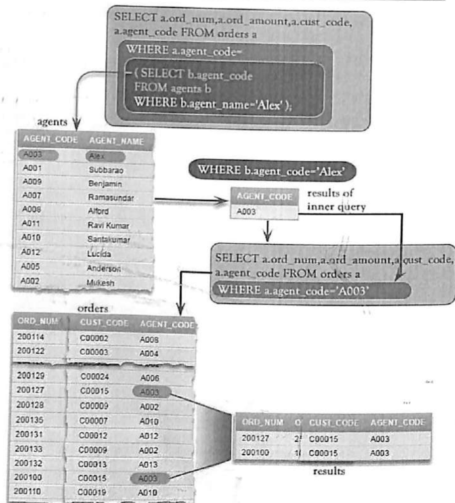
5.1.8-rasm. So'rov sxemasi
