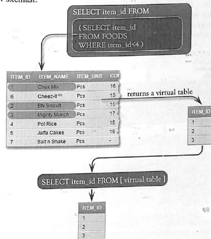
5.1.4-rasm. So'rov sxemasi
