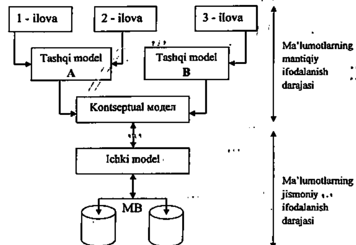
1.3.2- rasm. Ma'lumotlarning MB da ko'ppog'onali ifodalanishi
