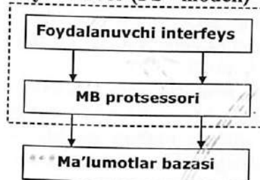
1.3.4 - rasm. «Fayl-server» va «klient-server» texnologiyalari
