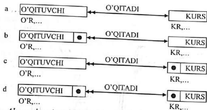
2.2.10-rasm. Aloqa darajasi N:1 bo'lgan holatlarga ER-tur diagrammalar
