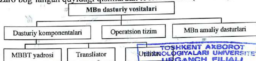
1.9-rasm. Ma'lumotlar bankining dasturiy ta'minoti
