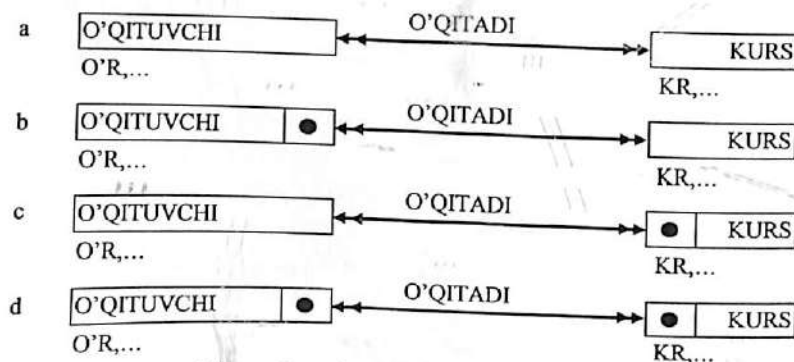
2.2.11-rasm. Aloqa darajasi N:M bo'lgan holatlarga ER-tur diagrammalar
