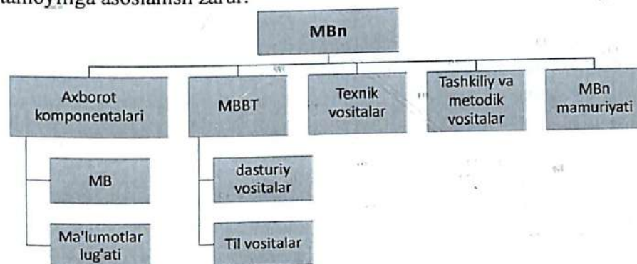
1.8-rasm. Ma'lumotlar banki komponentalari
