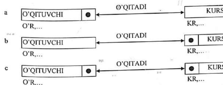
2.2.8-rasm. 1:1 aloqa darajasi va turli mansublik sinflari uchun diagrammalar
