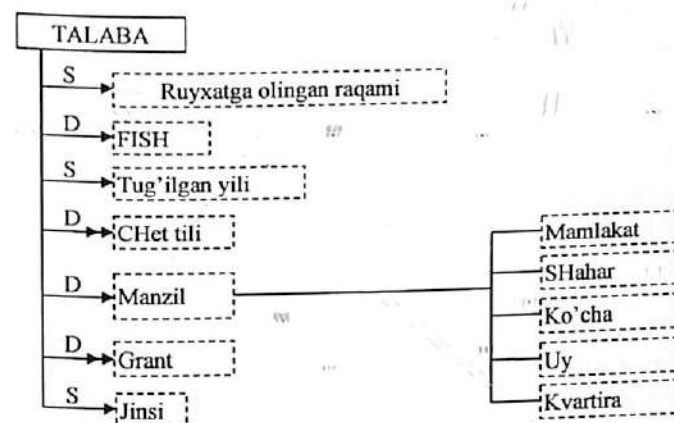
2.2.3-rasm. «ob'ekt — xususiyat» aloqasi
