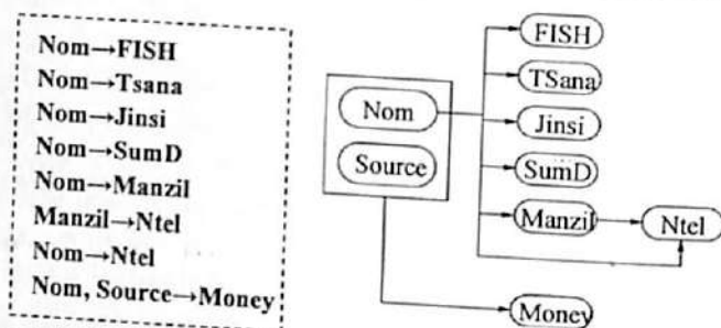
2.1.4-rasm. T-TN-T munosabatlarining atributlari o'rtasida mavjud funksional bog'liqlikni taqdim etishning turli usullari
