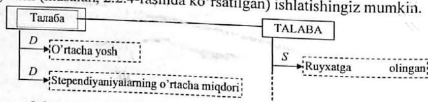
2.2.4-rasm. Ob'ektlar sinfi va integral xususiyatlar tasviri
