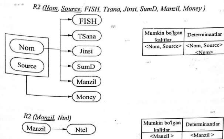
2.1.5-rasm. T-TN-T munosabati proektsiyalarining natijalari bo'lgan R1 va R2 munosabatlari
