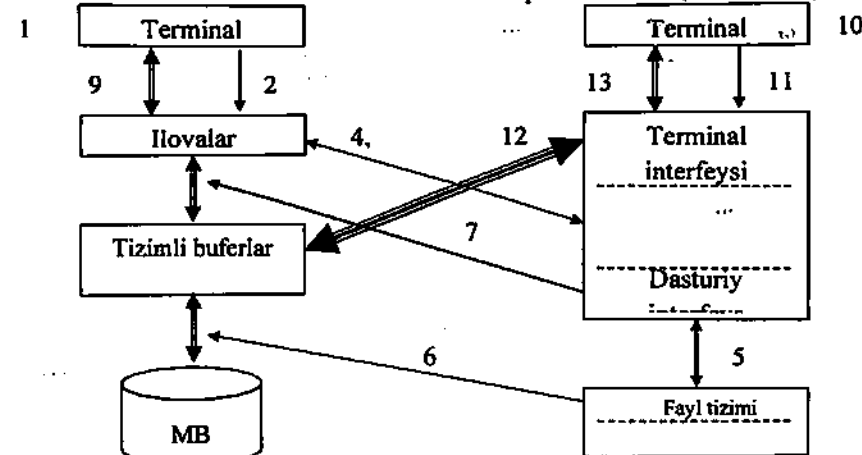
1.13-rasm. MB bilan ishlashda ma'lumotlarning almashinish sxemasi
