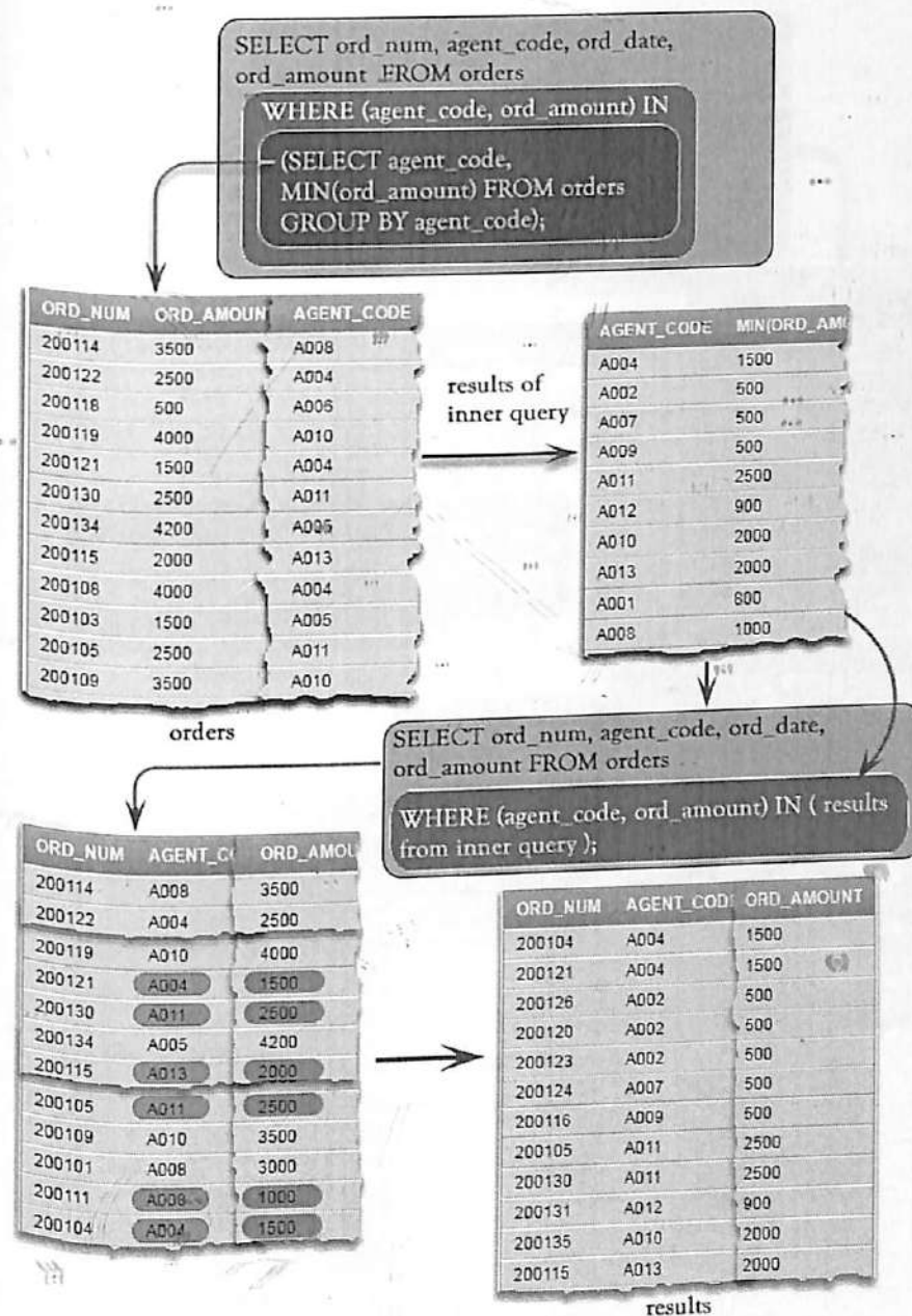
5.1.7-rasm. So'rov sxemasi
