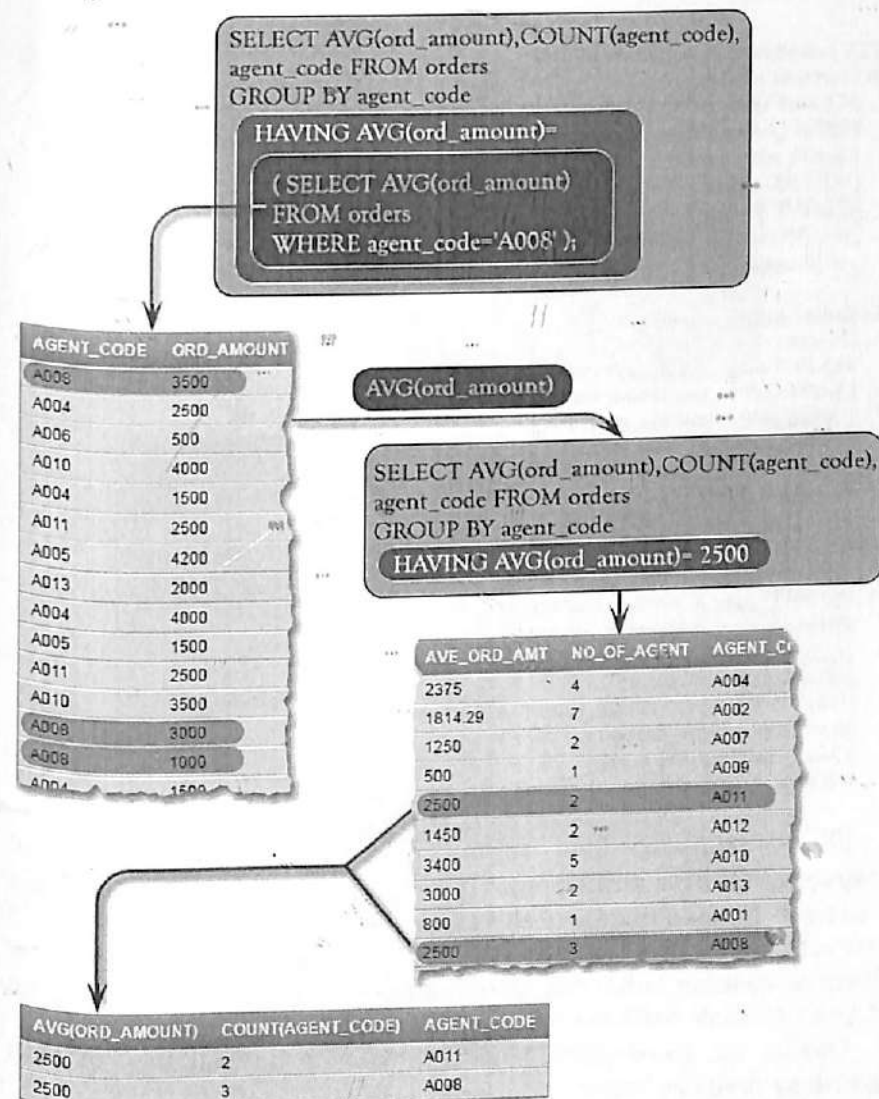
5.1.3-rasm. So'rov sxemasi
