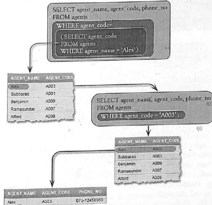
5.1.2-rasm. So'rov sxemasi
