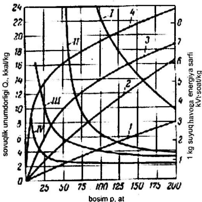
10.17-rasm. Suyuq havo olishda ishlatiladigan asosiy sovitish sikllarining solishtirma xarakteristikalar:
