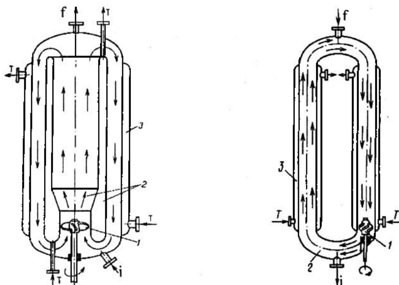
3.52-rasm. Diffuzorli va vintsimon aralashtirgichli qurilma. 1 - vintsimon aralashtirgich; 2 - issiqlik almashinish kamerali diffuzor; 3 - g'ilof; \tau - issiqlik eltich; j - aralashtirilayotgan suyuqlik.
