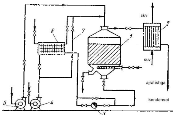
5.106-rasın. Bug'-havo aralashmasini tozalash uchun adsorbsion qurilma sxemasi.
