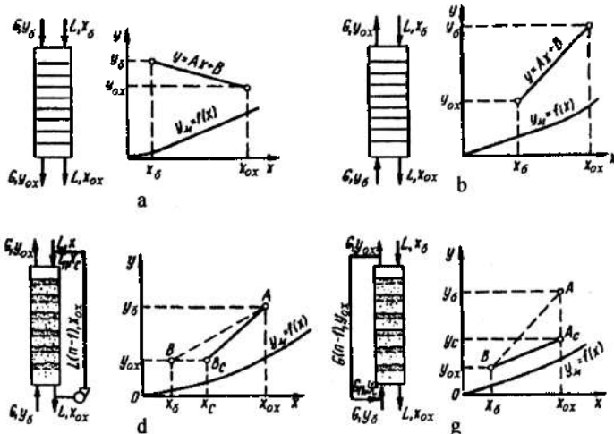
5.15-rasm. Absorbsiya sxemalari va jarayonni
