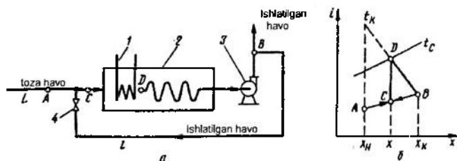
5.127-rasm. Ishlatilgan havoni qisman resirkulatsiya qiladigan quritkich sxemasi (a) va jarayonni i-x diagrammada tasvirlash (b). 1 - kalorifer; 2 - quritish kamerasi; 3 - ventilator; 4 - kran.
