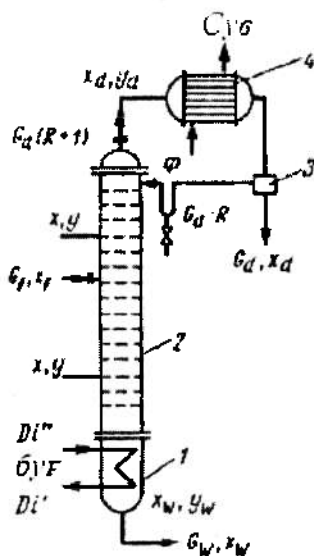
5.56-rasm. Rektifikatsiya jarayonining moddiy va issiqlik balanslarini tuzishga oid.
