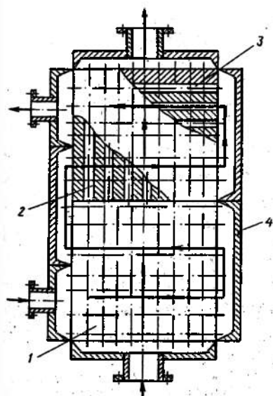
4.41-rasm. Blok-grafitli issiqlik almashinish qurilmasi.
