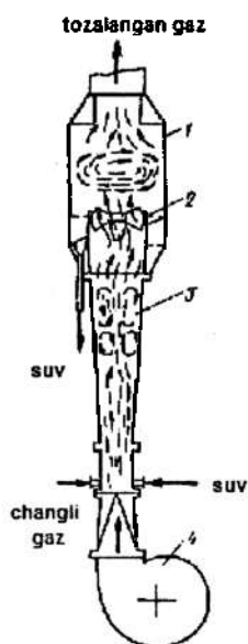
3.34b-rasm. Venturi skrubberi.
