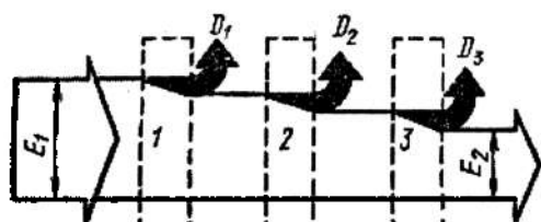
11.4-rasm. Eksergiya yo'qotilishining EKTS dagi o'ziga xos tomoni.
