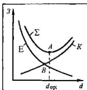
2.20-rasm. Truba quvurining eng samarador diametrini aniqlashga oid.
