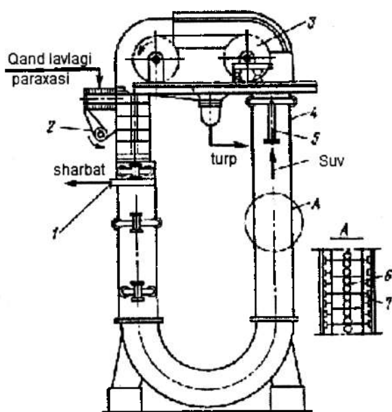
5.87-rasm. Ikki kolonnali diffuzion qurilma.
