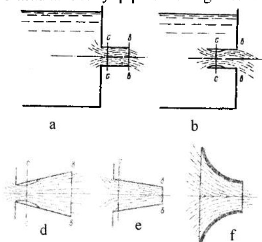
2.21-rasm. Nasadka turlari.
