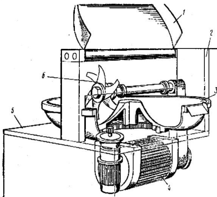
7.14 - rasm. Go'sht maydalagich (kutter)
