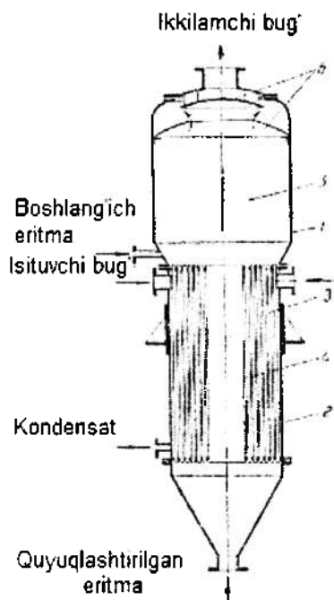
4.61-rasm. Ichki isituvchi kamera va markaziy sirkulatsion trubali bug'latish qurilmasi.
