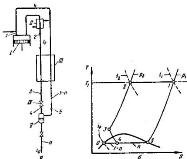
10.11-rasm. Bir karra drossellanishli, yuqori bosimli regenerativ sikl.
