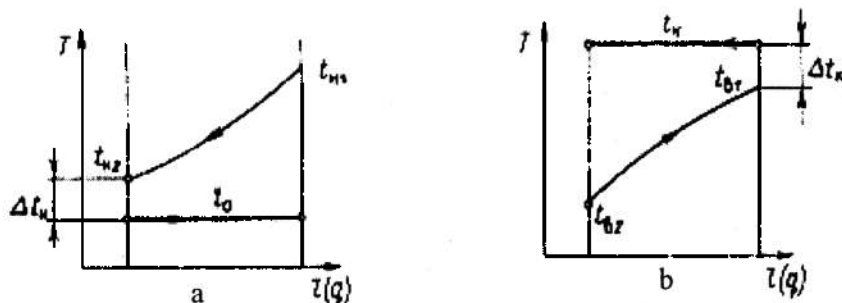
10.21-rasm. Oqimlar temperaturasi o'zgarish grafiklari a) bug'latkichdagi; b) kondensatordagi.
