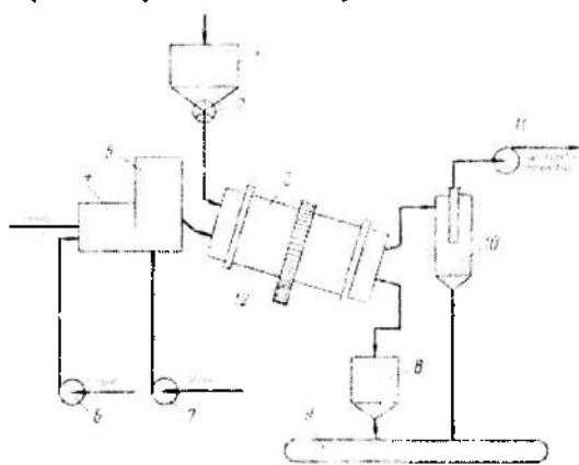
5.146-rasm. Barabanli quritkichning prinsiplial sxemasi.
