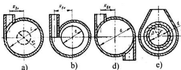
4.51-rasm. Issiqlik eltkichni tangensial yo'nalishda uzatish moslamalari. a - bitta teshikli tangensial uyurmaltirgich; b - chig'anoq shaklli uyurmaltirgich; d - ikkita teshikli uyurmaltirgich; e - tangensial kurakchali uyurmaltirgich.
