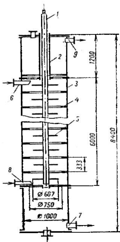
5.82-rasm. Rotor-diskli ekstraktor.
