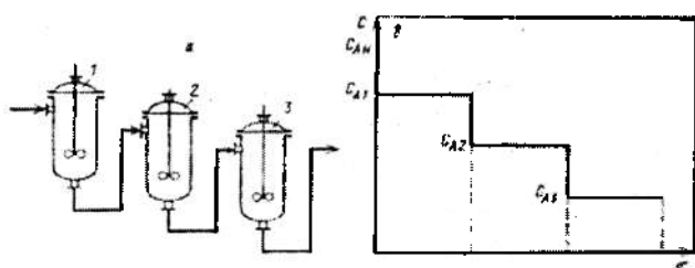
9.19-rasm. Ideal aralashish qurilmalar kaskadi (a) va unda konsentratsiya s ning vaqt \tau ga bog'liqligi (b).
