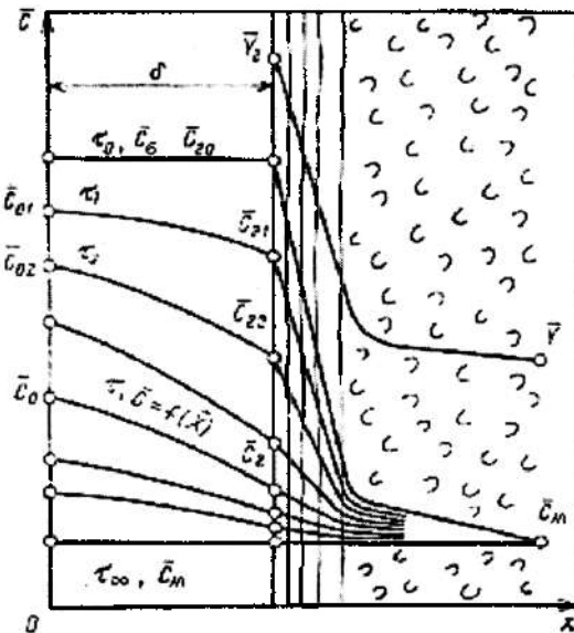
5.6-rasm. Kapillar - g'ovakli jismda massa almashinish modeli.
