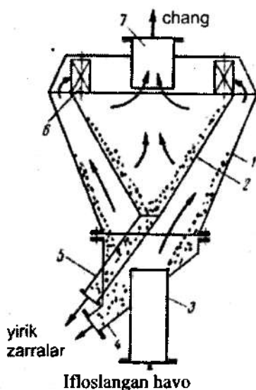
7.19-rasm. Markazdan qochma separator sxemasi.
