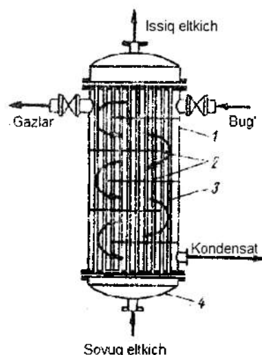
4.27-rasm. Ko'p yo'li issiqlik almashinish qurilmasi (trubalararo bo'shliq bo'yicha). 1 - qobiq; 2 - to'siq; 3 - isituvchi 2 - truba; 4 - qopqoq.
