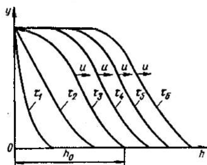
5.95-rasm. Adsorbsiya ko'lamining o'zgarish sxemasi.
