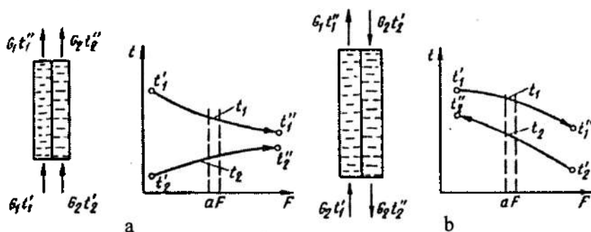
4.15-rasm. Issiqlik eltichlar temperaturalarining o'zgarish sxemasi: a - parallel yo'nalish; d - qarama - qarshi yo'nalish.
