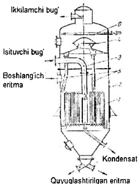
4.62-rasm. Osma isituvchi kamerali bug'latish qurilmasi.
