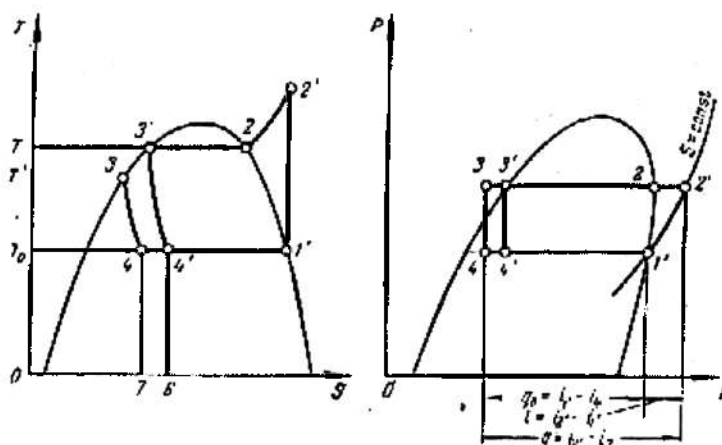
10.6-rasm. Haqiqiy kompressor sovitish mashinasi siklining T-S va p-i diagrammalardagi ko'rinishi.
