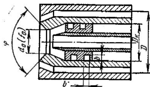
8.20-rasm. Purkagich maydalash kallagining konstruksiyasi.
