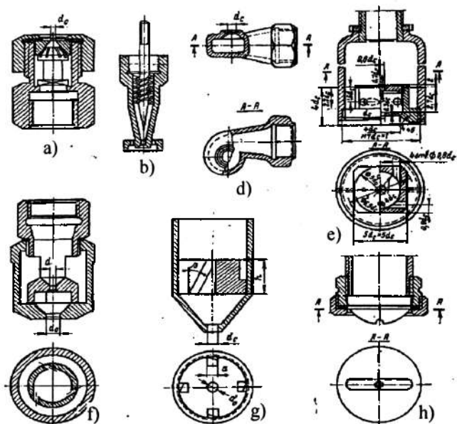
3.35d-rasm. Mexanik purkagichlar. a-d-markazdan qochma purkagichlar; e-evolvent purkagich; f-g-oqimchali-markazdan qochma; (g-VTI; d-vkladish silindrik vkladish va gorizontall kanalli; g-silindrik yassi vkladishli va chetida vintsimon kanalli); h - yassi favvorali, oqimchali purkagich.
