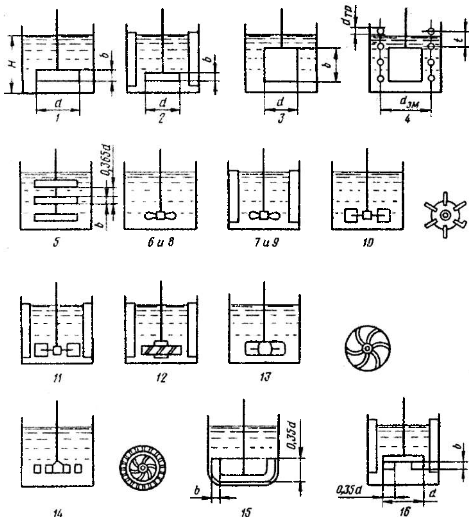
3.62-rasm. Aralashtirgichlar konstruksiyalari.
