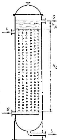
5.76-rasm. Ichi bo'sh (purkovchi) ekstraktor.
