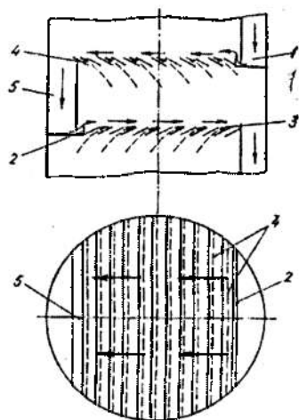
5.28-rasm. Oqimchali tarelka.
