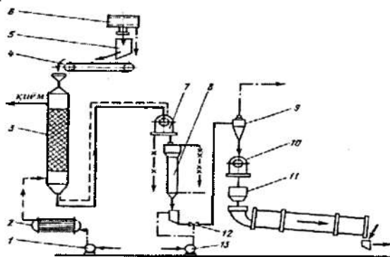
5.105-rasm. Qiyomni uzluksiz tozalash qurilmasi.
