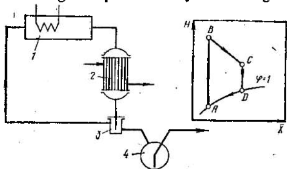
5.128-rasm. Ishlatilgan gazdan ko'p marta foydalanish usulida quritish sxemasi.
