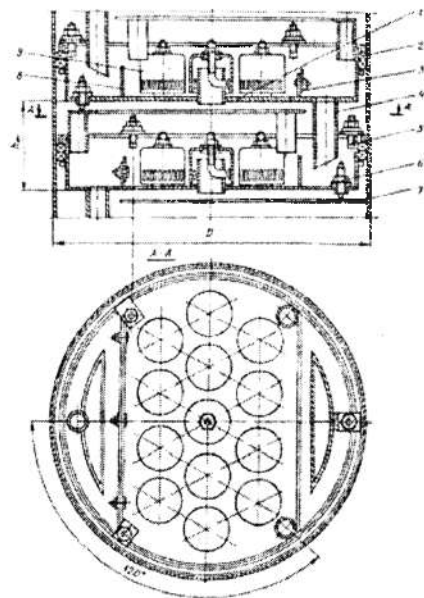
5.24-rasm. Qalpoqchali tarelka.
