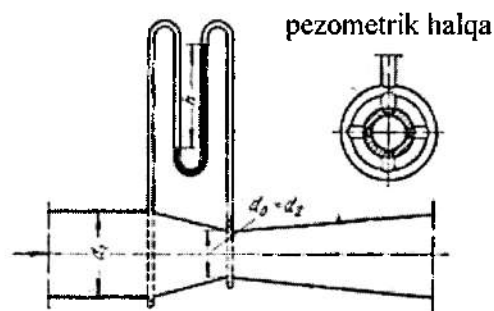
2.11-rasm. Venturi trubasi.
