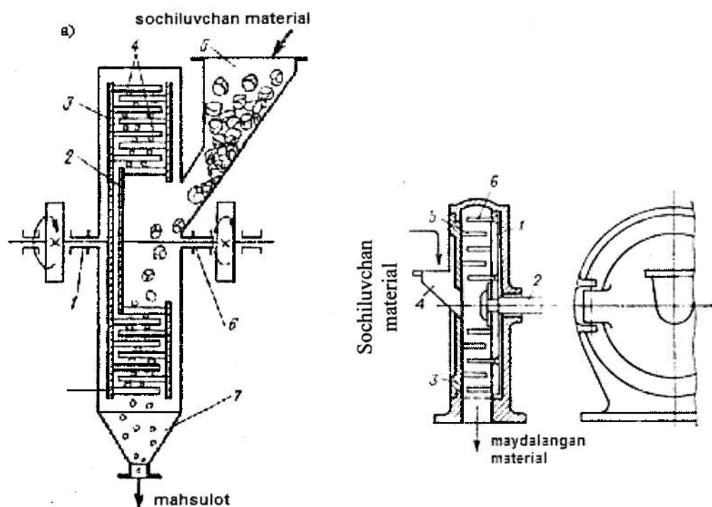
7.7-rasm. Dezintegrator (a) va dismembrator (b).
