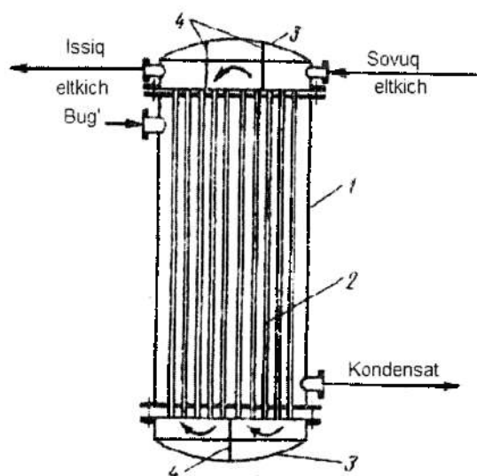
4.26-rasm. Ko'p yo'li issiqlik almashinish qurilmasi (truba bo'shlig'i bo'yicha). 1 - qobiq; 2 - isituvchi truba; 3 - qopqoq 4 - to'siq.
