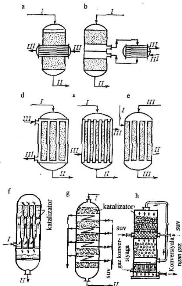
9.15-rasm. Siqib chiqarish reaktorining issiqlik almashinish moslamalari.
