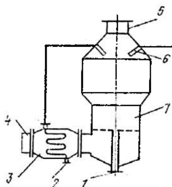
8.9-rasm. Markaziy to'kish va isitilgan eritmani qatlamlariga uzatuvchi silindrik qurilma.
