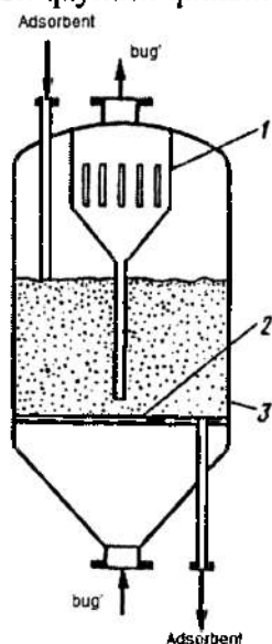
5.102-rasm. Uzlüksiz ishlaydigan, bir pog'onali mavhum qaynash qatlamli adsorber. 1 - qobiq; 2 - gaz taqsimlagich; 3 - chang yig'gich.
