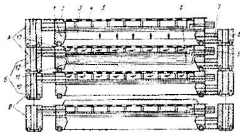
3.21-rasm. Gorizontall kamerali filtr - press (FPKAM).
