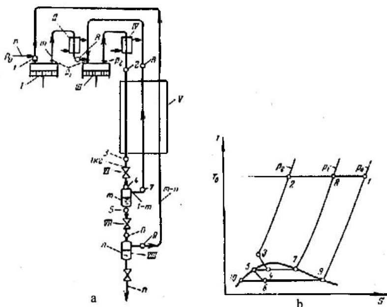
10.13-rasm. Ikki karra drossellanishli va gazning bosim ostidagi aylanishli sikl.
