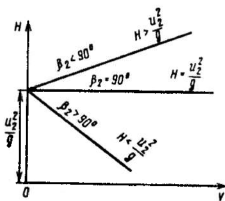
2.32-rasm. Markazdan qochma nasos naporiga \beta_2 burchakning ta'siri.
