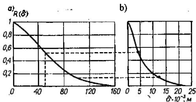
7.22-rasm. Bolg'ali mashinada maydalangan mahsulot R(\delta) funksiyasini aniqlashga oid.
