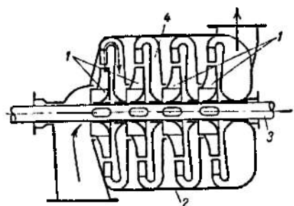
2.30-rasm. Ko'p bosqichli, markazdan qochma nasos sxemasi: 1-ishchi g'ildirak; 2-qobiq; 3 - o'q; 4- aylanma kanal.
