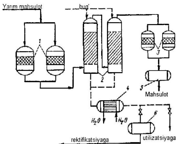
5.104-rasm. Qo'zg'almas faollangan ko'mir qatlamida suv-spirt aralashmasini tozalash qurilmasining sxemasi. 1,3-filtrlar; 2-adsorberlar; 4,6-yig'gichlar; 5-kondensator-sovutkich.
