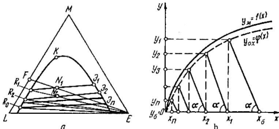
5.73-rasm. O'zaro kesishgan yo'nalishli ko'p pog'onali ekstraksiya jarayonini uchburchakli diagramma (a) va u-x koordinatlarda (b) tasvirlash.
