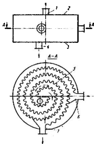
4.69-rasm. Plastinali spiralsimon issiqlik almashinish qurilmasi. 1,4,6,7 – shtuserlar; 2,3 – tekis qopqoqlar; 5 – gofrirlangan list.
