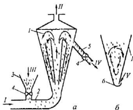
5.138. Aerofontan quritkich.
