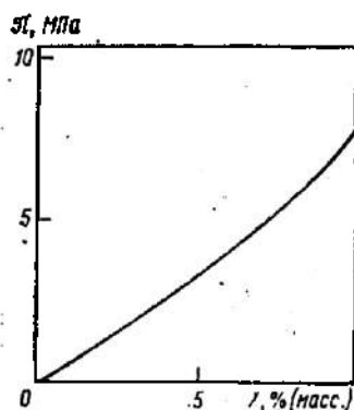
3.75-rasm. Temperatura 25°C dagi \text{CaCl}_2 ning suvli eritmasi osmotik bosimining konsentratsiyaga bog'liqligi.
