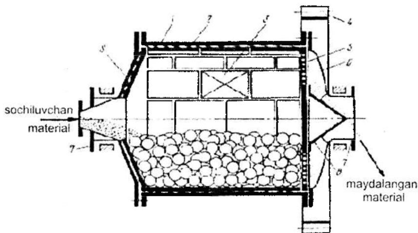
7.11-rasm. Sharli tegirmon.
