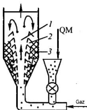
3.42-rasm. Favvorasimon qatlam.
