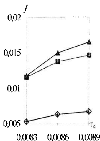
10.19-rasm. Nisbiy yuzaning eksergetik harorat funksiyasiga bog'liqligi.
