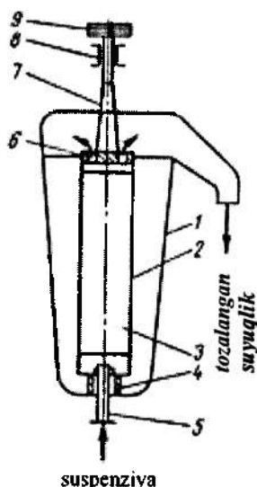
3.13-rasm. O'ta samarali sentrifuga.
