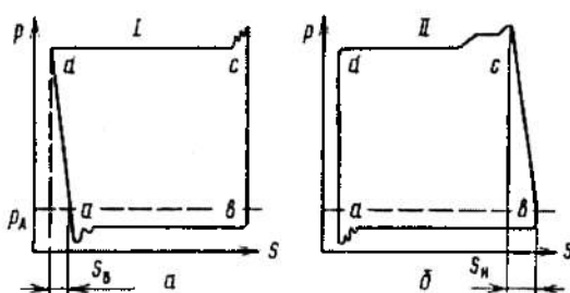
2.46-rasm. Nasos ishidagi ba'zi nosozliklar: a - klapaning yopishib qolishi; b - so'rish klapani yopilishining kechikishi.
