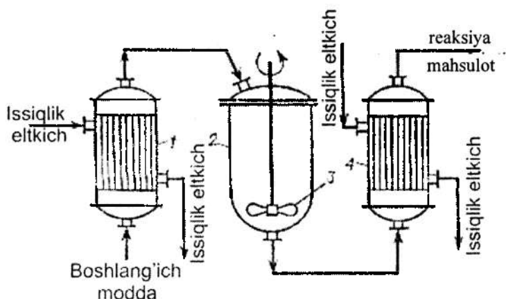
9.9-rasm. Uzlüksiz ishlaydigan reaktör 1,4-issitkichlar; 2-reaktor; 3-aralashtirgich.
