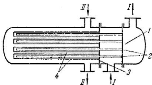
4.30-rasm. Qo'shaloq trubali qobiq - trubali issiqlik almashinish qurilmasi. 1, 3 - teshikli panjara; 2 - ichki truba; 4-tashqi truba.
