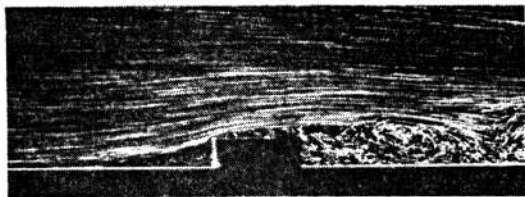
4.48-rasm. Silliq (a) va to'g'ri to'rtburchak (b) shaklidagi bo'rtiq to'siqlarda oqim turbulentsligining tuzilishi.
