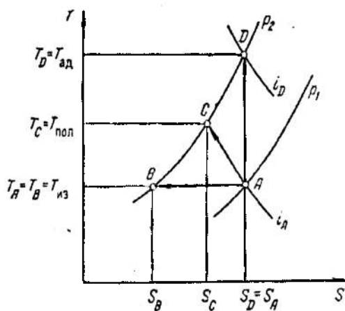
2.61-rasm. T - S diagrammada gazni siqish jarayonini tasvirlash.
