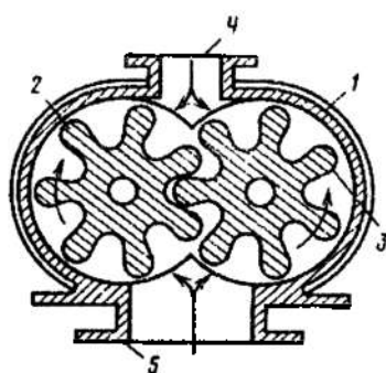
2.51-rasm. Shesternyali nasos sxemasi:
