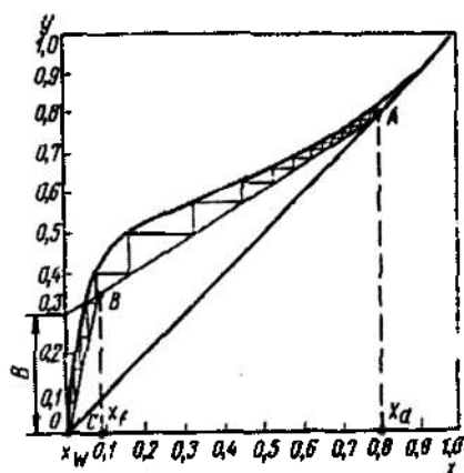
5.63-rasm. Rektifikatsion kolonna tarelkalarining sonini grafik usulda aniqlash.
