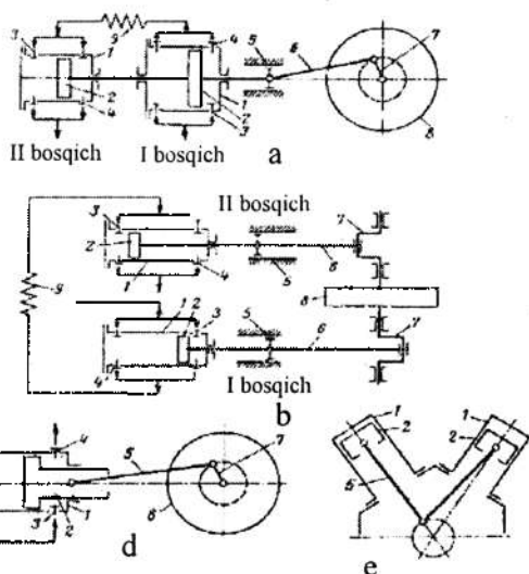
2.63-rasm. Ikki bosqichli porshenli kompressor:
