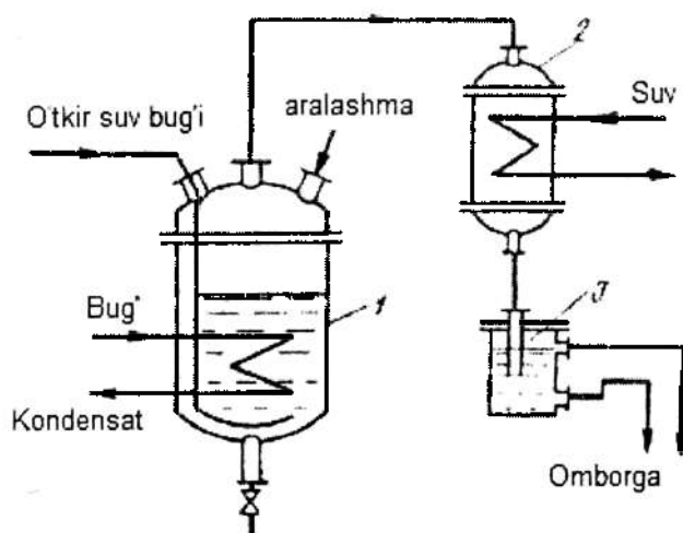
5.53-rasm. Suv bug'i bilan oddiy haydash qurilmasi
