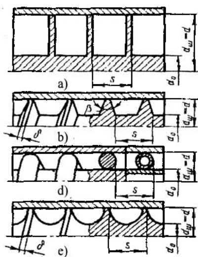
4.50-rasm. Shneksimon uyurmaltirgichlar konstruksiyalari.
