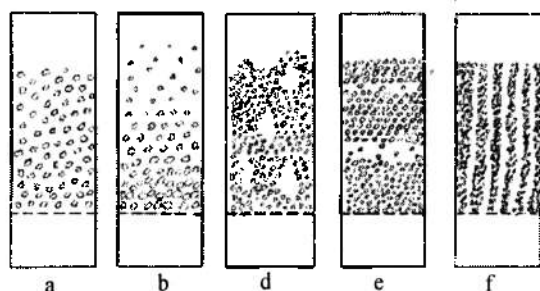
3.41-rasm. Mavhum qaynash qatlamining turlari. a - bir jinsli; b - turli jinsli; d - barbotajli; e - porshenli; f - kanalli.
