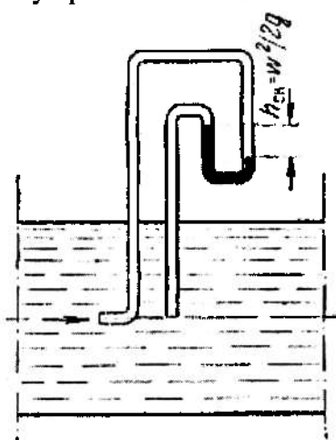
2.8-rasm. Pito-Prandtl pnevmometrik trubka yordamida suyuqlik tezligini o‘lchash.
