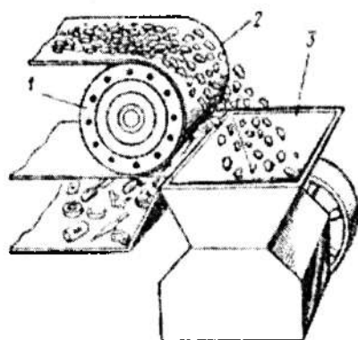
7.18-rasm. Elektromagnit barabanli g'alvir 1-ajratkich; 2-konveyer; 3-bunker.
