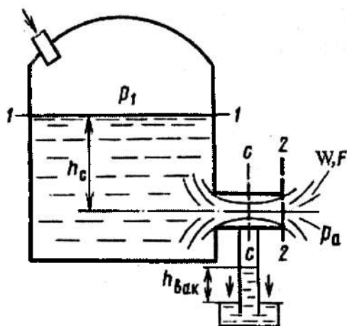
2.24-rasm. Idishdagi suyuqlik o'zgar-mas bo'lganda silindrik nasadkadan suyuqlik oqib chiqishi.
