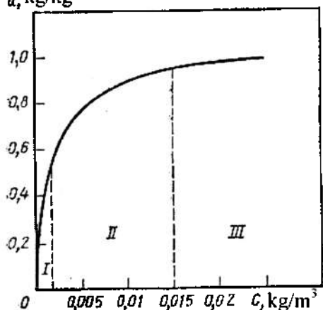
5.109-rasm. ЭДЭ – 10Π anionitda limon kislotasining muvozanat izotermalari.
