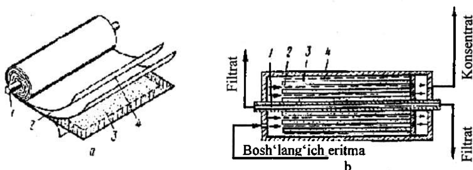
3.70-rasm. O'ramli filtr element (a) va shunday elementli qurilma (b)
