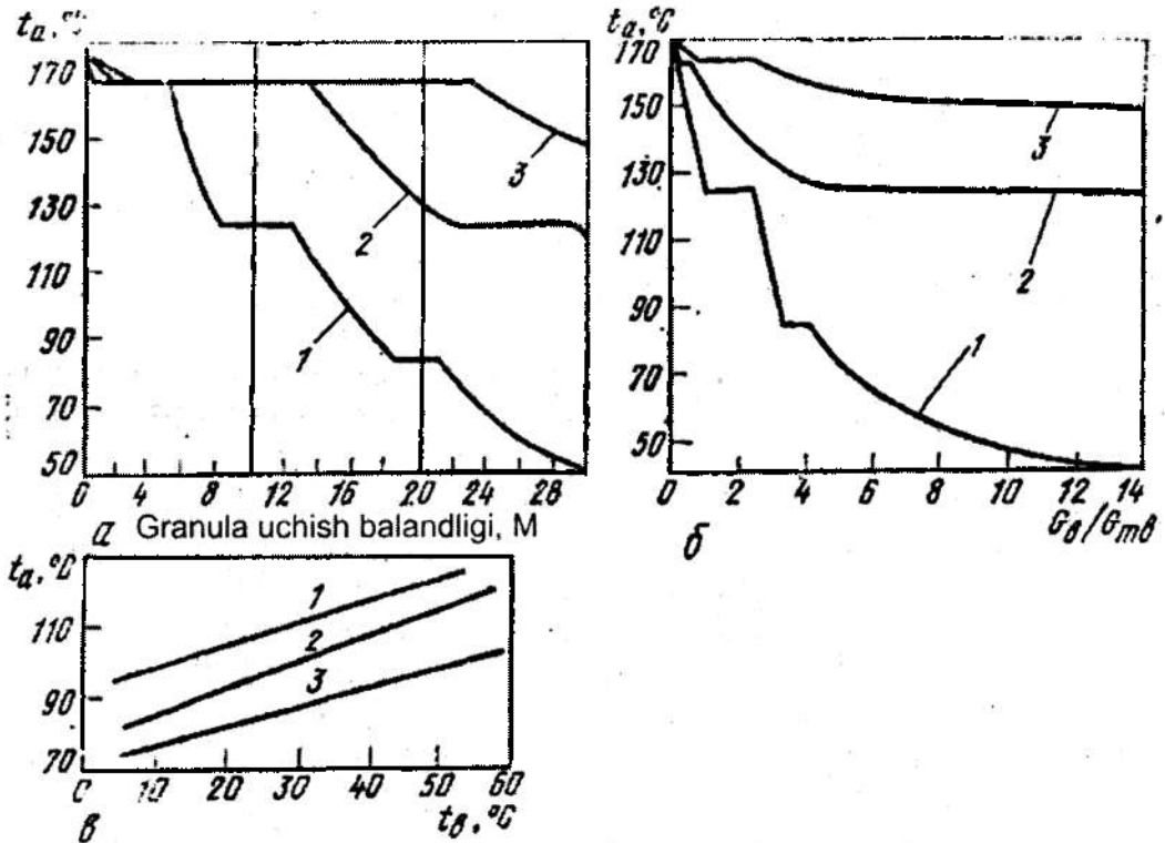
8.18-rasm. Granula adiabatik temperaturasi t_a ning jarayonning turli parametrlariga bog'liqligi.
