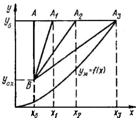
5.13-rasm. Absorbentning solishtirma sarfini aniqlashga oid.
