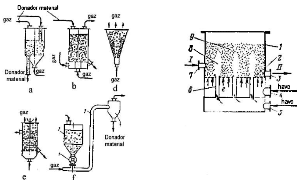
3.49-rasm. Mavhum qaynash qatlamli qurilmalar sxemalari.
