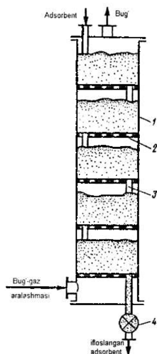
5.103-rasm. Ko'p pog'onali, mavhum qaynash qatlamli adsorber. 1 - qobiq; 2 - gaz taqsimlovchi teshikli panjara; 3 - quyilish patrubkasi; 4 - shlyuzli tamba.
