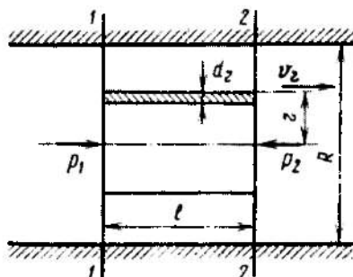
2.14-rasm. Tezliklarni taqsimlanish qonuniga oid keltirib chiqarish.
