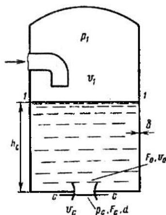
2.22-rasm. Idishda suyuqlik balandligi o'zgarmas bo'lganda, uning tubidagi dumaloq teshikdan oqib chiqishi.
