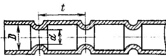
4.49-rasm. Tashqi tomonida ko'ndalang botiq ariqcha va ichki tomoni silliq bo'rtiq to'siqli samarador issiqlik almashinish yuzasi.
