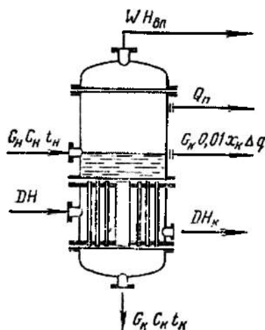
4.56-rasm. Oddiy bug'latish jarayonidagi issiqlik oqimlar sxemasi.
