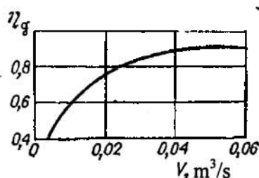
7.24-rasm. Konuvli va jag'li mashinalar f.i.k ning hajmiy sarf V bog'liqligi.
