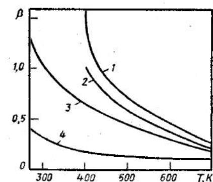
9.6-rasm. Reaksiya tezligi temperaturaviy koeffitsiyenti \beta ning temperatura T va faollashish energiyasi YE ga ta'siri.
