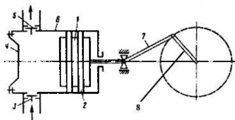
2.38-rasm. Bir tomonlama harakatlanuvchi, gorizontall porshenli nasos sxemasi: 1-porshen; 2-zichlovchi halqalar; 3-so'rish klapani; 4-silindr qopqog'i; 5-haydash (uzatish) klapani; 6-silindr; 7-krivoship; 8-shatun.
