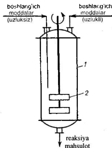
9.10-rasm. Yarim uzluksiz ishlaydigan reaktör. 1-qobiq; 2-aralashtirgich.
