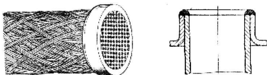
4.73-rasm. Ftoroplast trubali issiqlik almashinish elementi.
