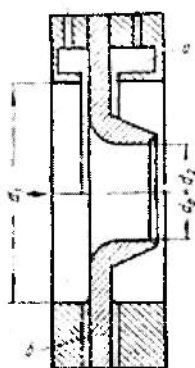
2.10-rasm. O'lchov soplosi.
