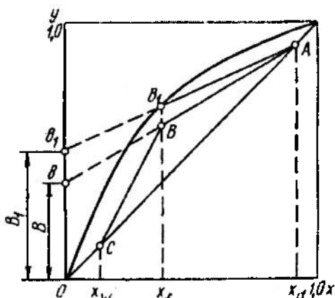
5.57-rasm. Rektifikatsiya jarayoni ishchi chizig'ining tasviri.
