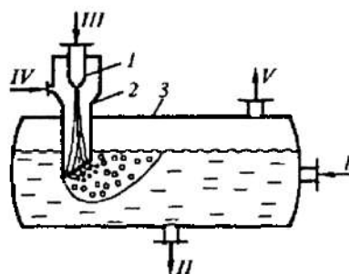
4.68-rasm. Yondirgichi cho'kib turuvchi barbotajli bug'latkich. 1-purkagich; 2-cho'kib turuvchi yondirgich; 3-qobiq. I-dastlabki eritma; II-quyultirilgan eritma; III-yoqilg'i; IV-havo; V-tutun gazlari
