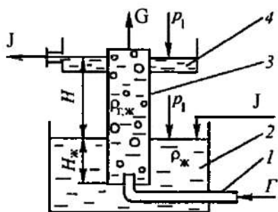
2.58-rasm. Gazlift sxemasi.
