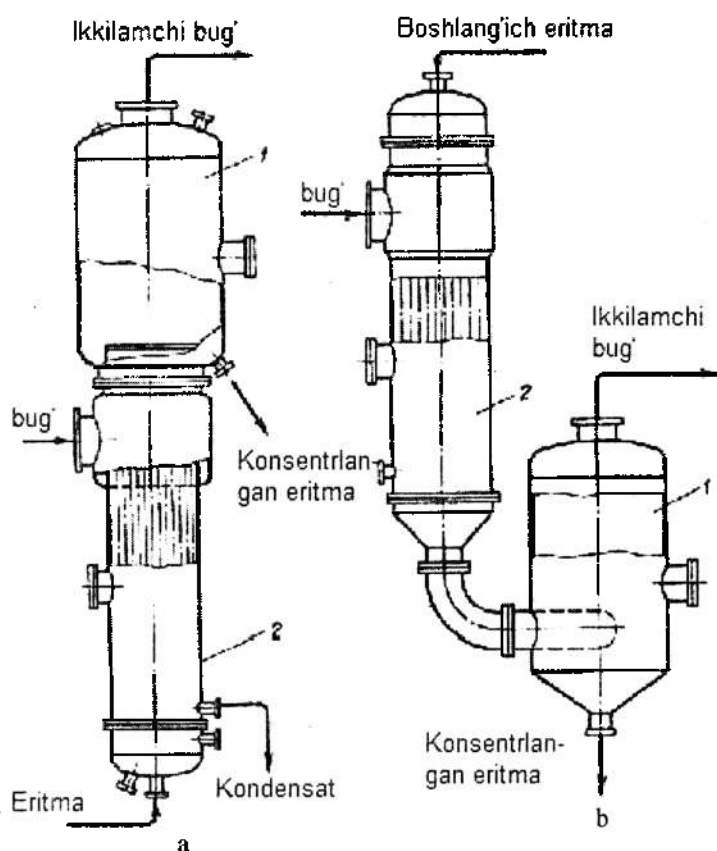
4.65-rasm. Yupqa qatlamli bug'latkichlar. a – ko'tariluvchi qatlamli bug'latkich; b – pastga oqib tushuvchi qatlamli bug'latkich. 1 - separator; 2 - isituvchi kamera.
