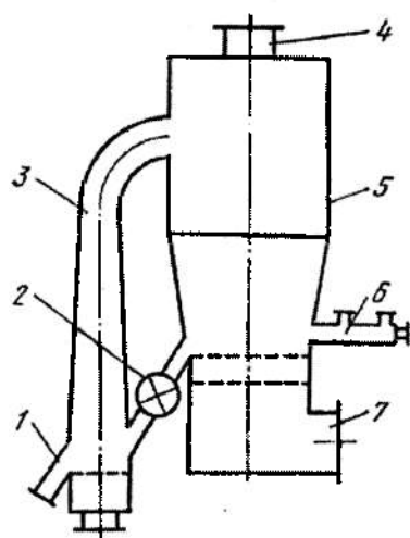
8.13-rasm. Kvadrat shaklidagi mavhum qaynash qatlamli granulator 1-granula to'kish patrubkasi; 2-tamba; 3-havoli konussimon klassifikator; 4-ishlatib bo'lingan issiqlik eltkichni chiqarish patrubkasi; 5-qobiq; 6-suyuqlik va resiklni uzatish bo'lagi; 7-issiqlik eltkich kirish patrubkasi.
