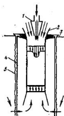
3.32d-rasm. Filtr puflab tozalash ejektor.
