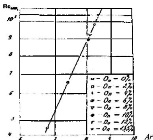
3.44-rasm. Donador-tolali materiallar uchun Re sonining Ar kriteriysiga bog'liqligi.
