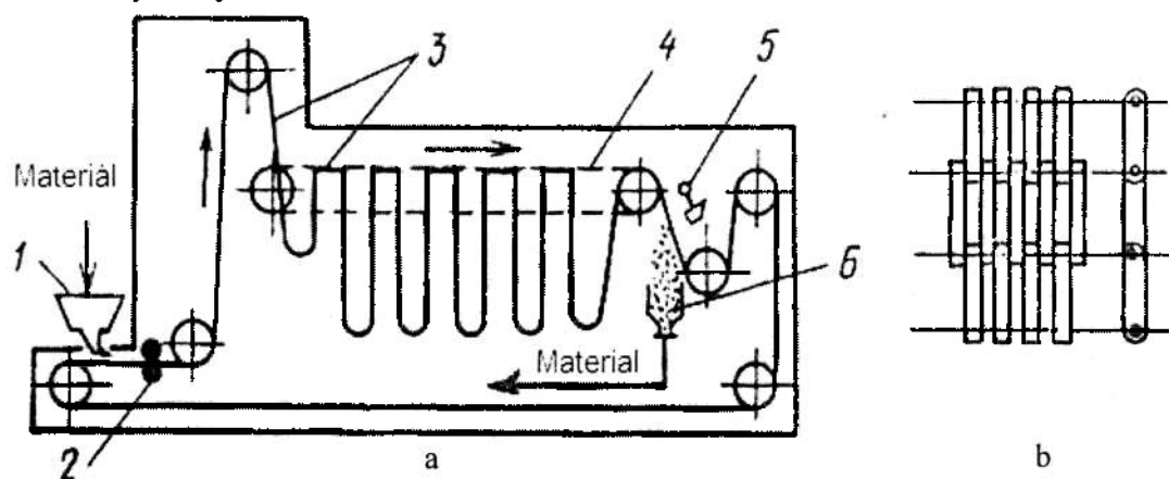
5.133-rasm. Sirtmoqli quritkich (a) va to'rli lenta elementi (b).
