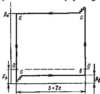
2.45-rasm. Indikator diagrammasi.
