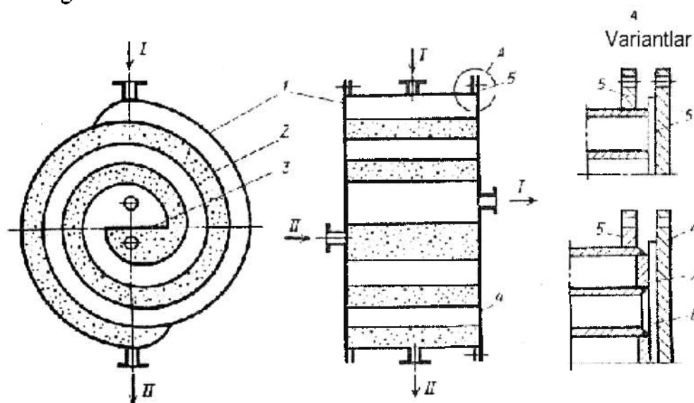
4.36-rasm. Spiralsimon issiqlik almashinish qurilmasi.
