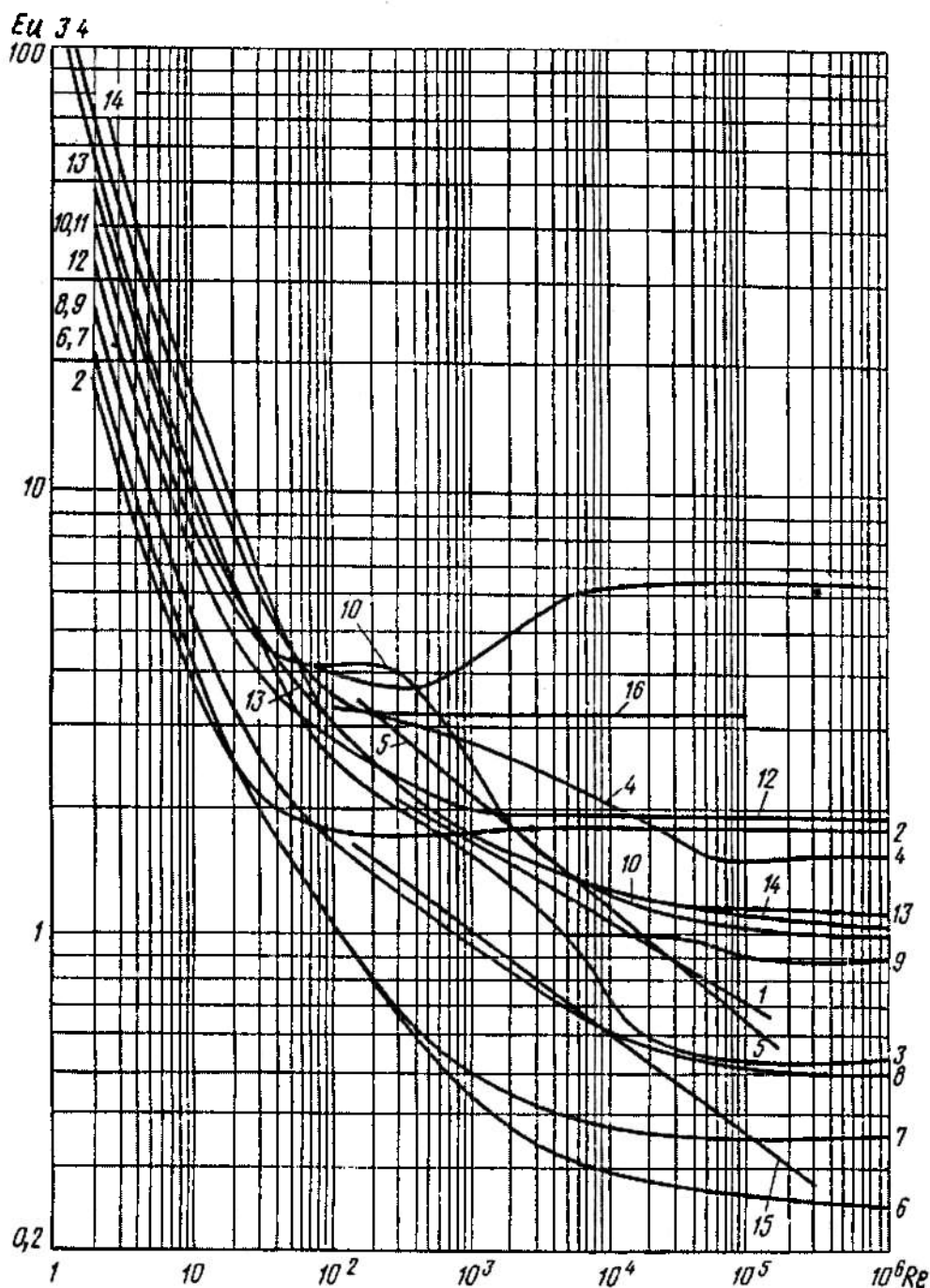
3.63-rasm. Turli turdagi aralashtirgichlar uchun Eu=f(Re) bog'liqligi. Raqamlar 3-4 jadvaldagi va 3.62-rasmlardagi aralashtirgich raqami va turiga mos keladi.
