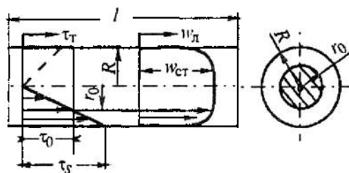
2.18-rasm. Dumaloq trubada bingham suyuqligining plastik oqish qonuniyatlariga oid.
