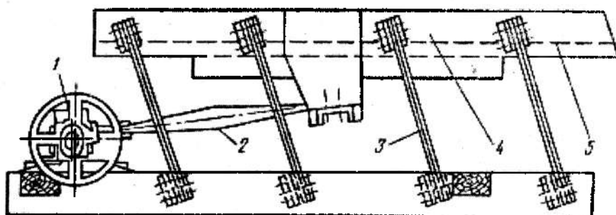
7.16-rasm. Tebranuvchi elak. 1-ekssentrik; 2-shatun; 3- prujina; 4-qobiq; 5-elak.
