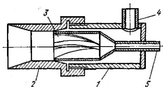
8.14a-rasm. Pnevmatik purkagich. 1-qobiq; 2-soplo; 3-pulpa uyurmalgich; 4-siqilgan havo kirish patrubkasi; 5-pulpa chiqarish patrubkasi.
