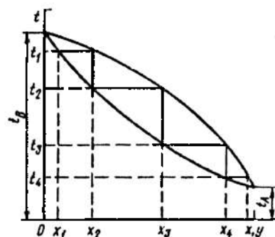
5.55-rasm. t - x, y - diagramma.
