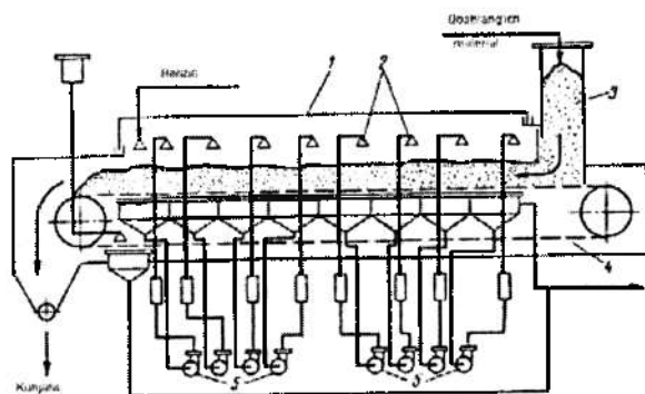
5.88-rasm. Lentali ekstraktor.
