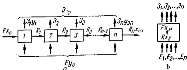
5.72-rasm. Ko'p pog'onali, oqimlar yo'nalishi o'zaro kesishgan ekstraksiyalash sxemasi.
