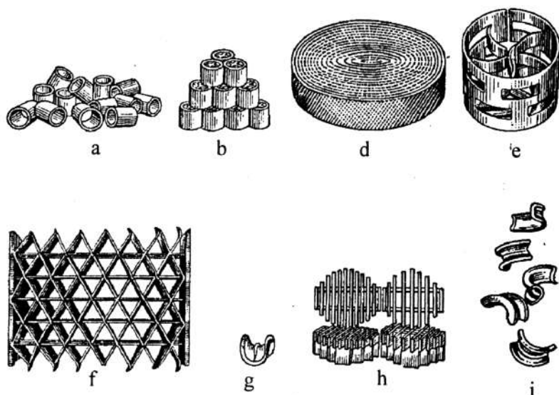
5.19-rasm. Nasadka turlari.
