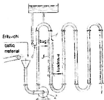
5.89-rasm. Trubali ekstraktor.
