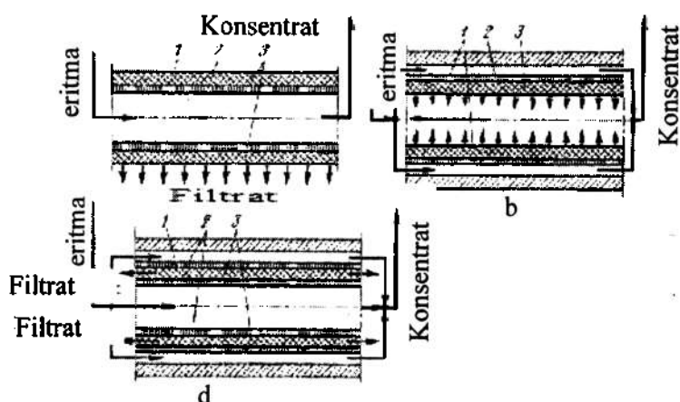
3.69-rasm. Membranasi turlicha joylashtirilgan silindrik filtrlovchi elementlar.
