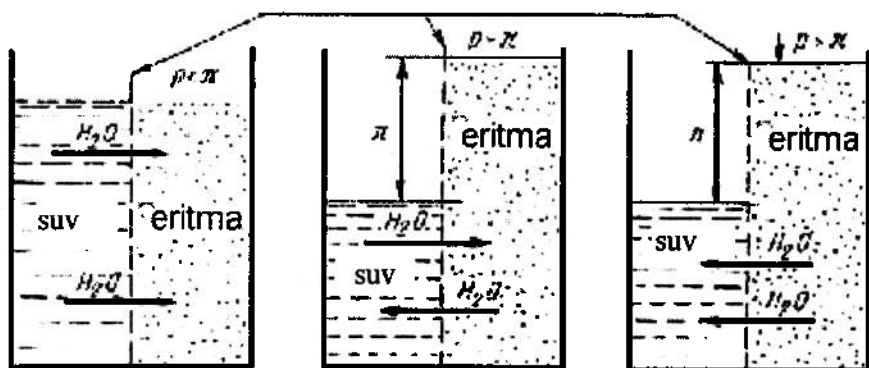
3.66-rasm. Teskari osmos usulida eritmalarni ajratish sxemasi.
