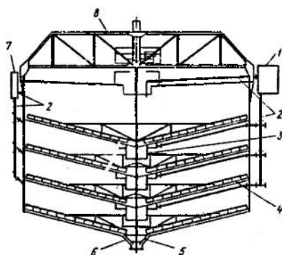
3.6-rasm. Ko'p qavatli tindirgich.
