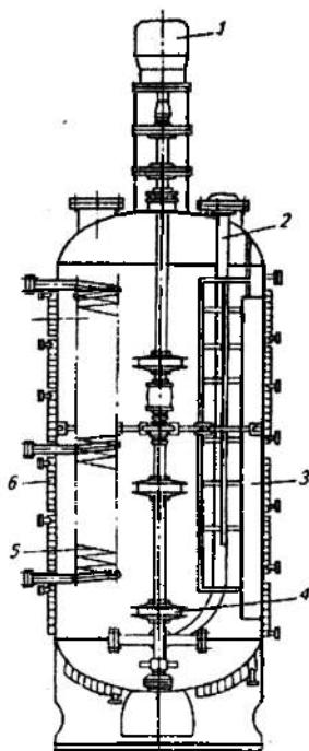
6.4- rasm. Fermentator sxemasi.
