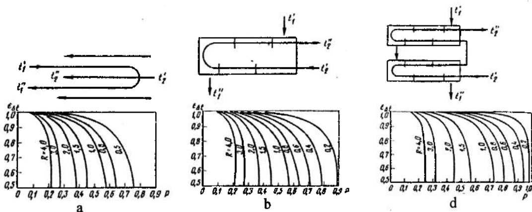
4.16-rasm. Aralash yo'nalishli qobiq - trubali issiqlik almashinish qurilmasida issiqlik eltichlarning harakat sxemasi va \varepsilon koeffitsiyenti:
