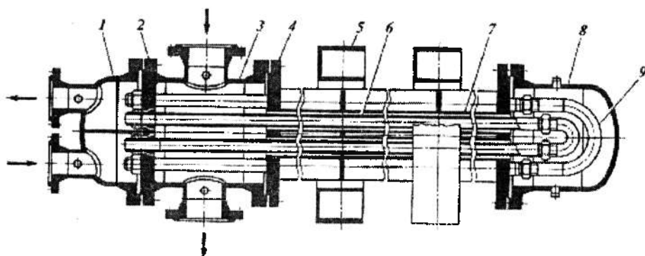
4.33-rasm. «Truba ichida truba» tipidagi ajraluvchan, ko'p oqimli issiqlik almashinish qurilmasi.
