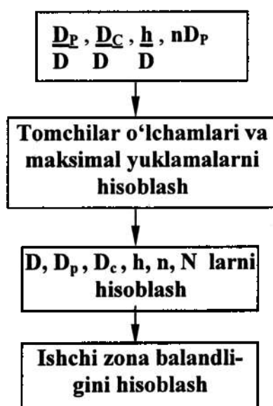
5.81-rasm. Rotor-diskli ekstraktor o'lchamlarini hisoblash sxemasi.
