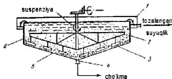
3.5-rasm. Eshkak aralashtirgichli uzluksiz ishlaydigan tindirgich.
