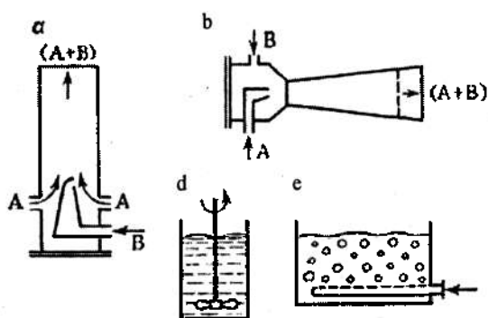
9.17-rasm. Kimyoviy reaktorlar aralashtiruvchi moslamalarining turlari.
