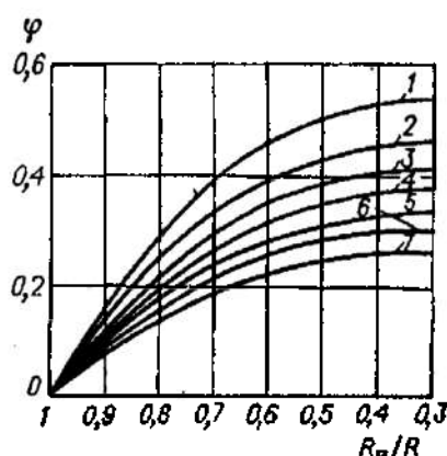
7.28-rasm. To'ldirish ko'effitsiyenti-ning n\sqrt{2R} turli qiymatlarida sharlarning eng kichik radiusiga bog'liqligi. 1-0,62; 2-0,57; 3-0,53; 4-0,5; 5-0,47; 6-0,45; 7-0,42.
