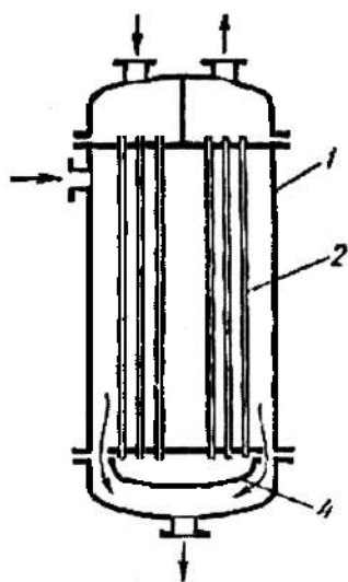
4.29-rasm. Harakatchan qalpoqchali issiqlik almashinish qurilmasi. 1 - qobiq; 2 - isituvchi trubalar; 3 - harakatchan qalpoqcha.
