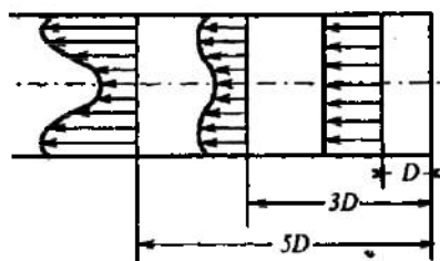
5.18b-rasm. Kolonnali qurilmada baland qatlamli nasadka orqali oqib tushayotgan suyuqlik tezligining epyuralari.
