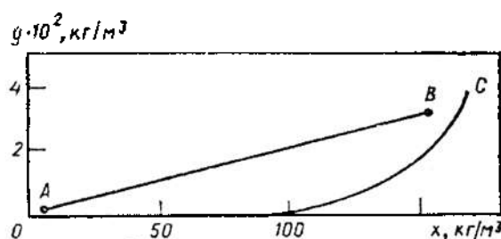
5.107-rasm. AR-A markali faollangan ko'mirda havodan benzolni adsorbsiyalash jarayonining ishchi (IV) va muvozanat (OS) chiziqlari.
