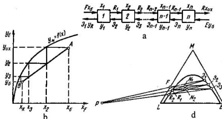
5.71-rasm. Ko'p pog'onali ekstraksiya (a) va jarayonni y - x (b) va uchburchakli (d) diagrammada tasvirlash.
