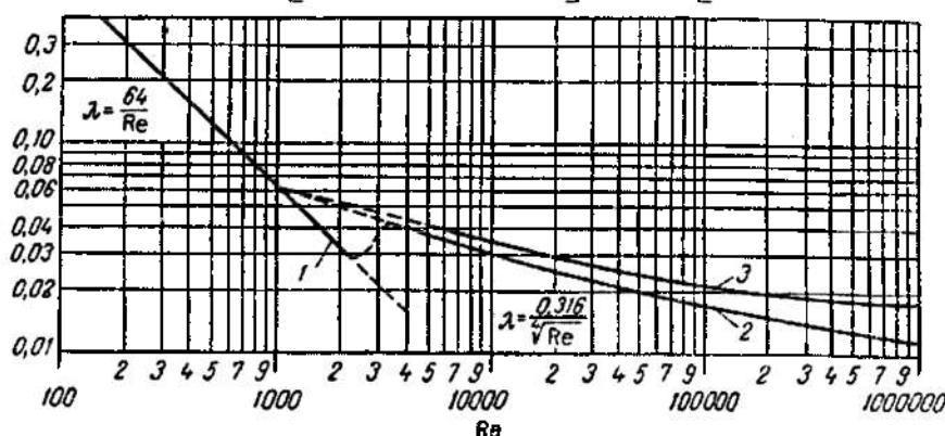
2.16a-rasm. Gidravlik qarshilik ko'effitsiyenti \lambda ning Reynolds kriteriysiga bog'liqligi.
