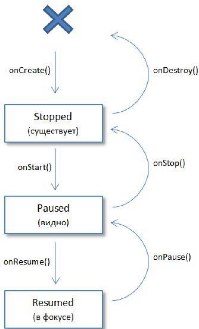
1.30-rasm. Hayot siklining ishlash jarayoni.
