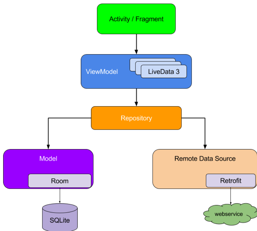
2.8-rasm. Dastur umumiy arxitekturası.
