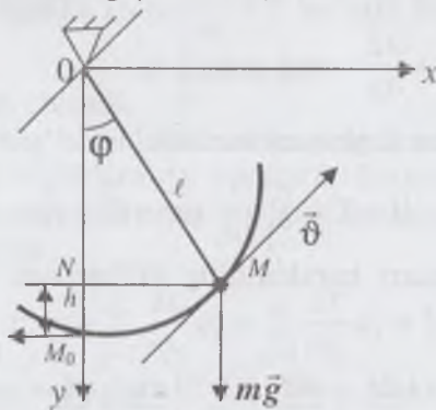
Yechish. Matematik mayatnikning kinetik va potensial energiyalari hisoblaniladi:
