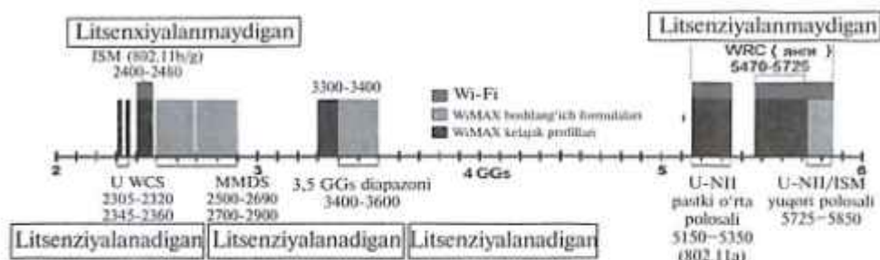
34.1-rasm. 2GGsdan 6 GGsgacha diapazonda KSU tizimlari uchun ruxsat etiladigan chastotalar polosasi.
