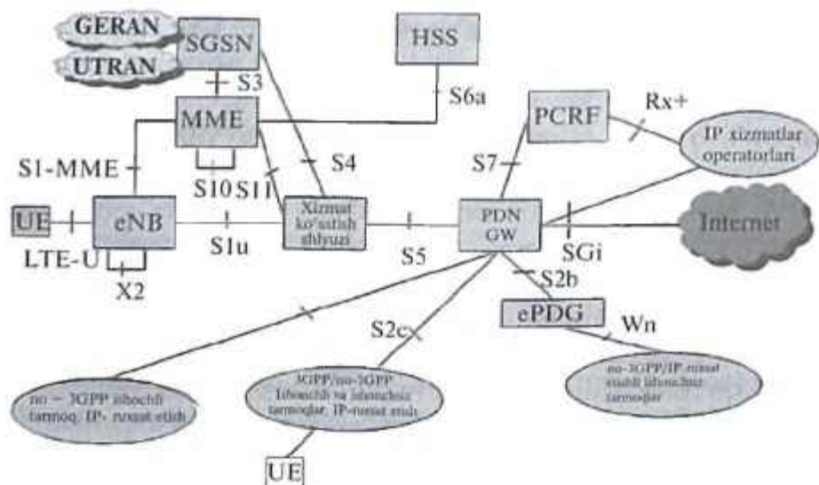
14.3-rasm. LTE/SAE tizimi arxitekturasini.
