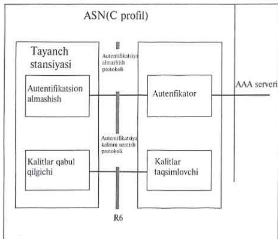
36.7-rasm. S profili uchun ASN tarmog'i xavfsizligi arxitekturası.
