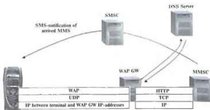
3.8-rasm. MMS bog’lanuvchi qurilma.
