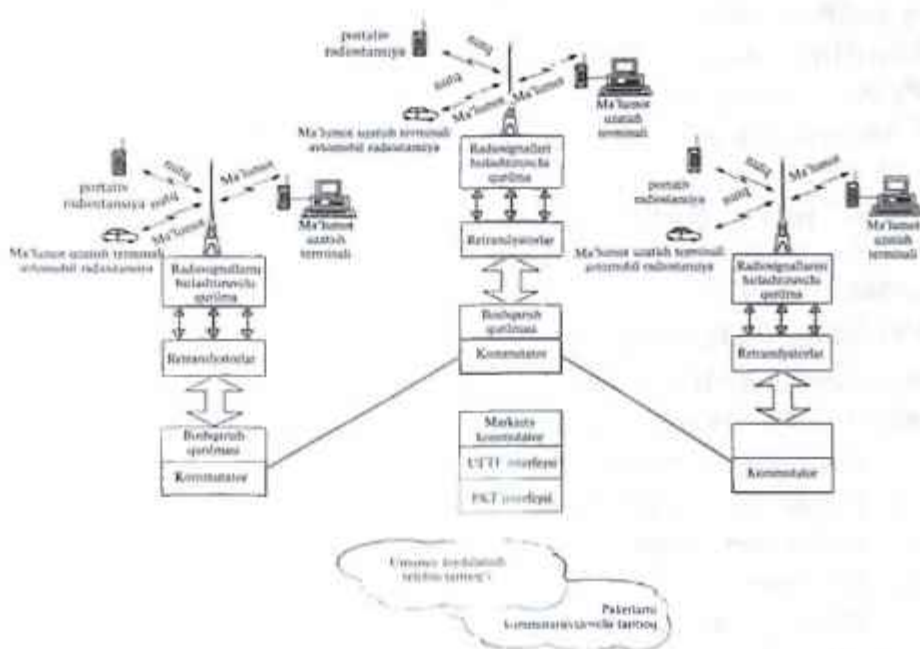
10.3-rasm. Markazlashtirilgan zonalararo kommunikatsiyali trunking tizimning umumlashtirilgan strukturaviy sxemasi.
