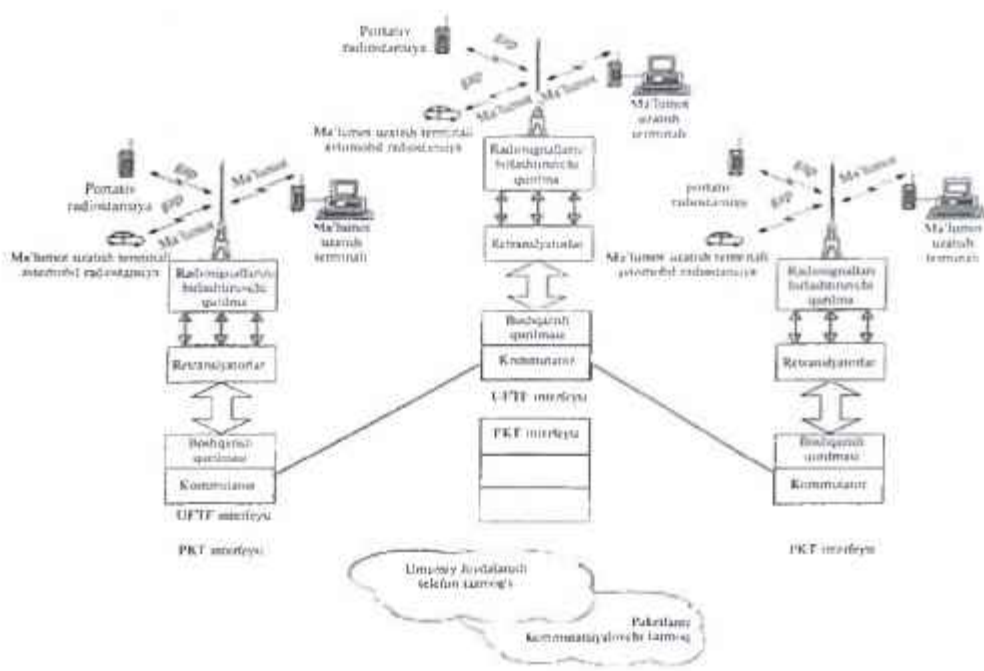
10.2-rasm. Zonalararo taqsimlangan kommutatsiyali tranking tizimning umumlashtirilgan strukturaviy sxemasi.
