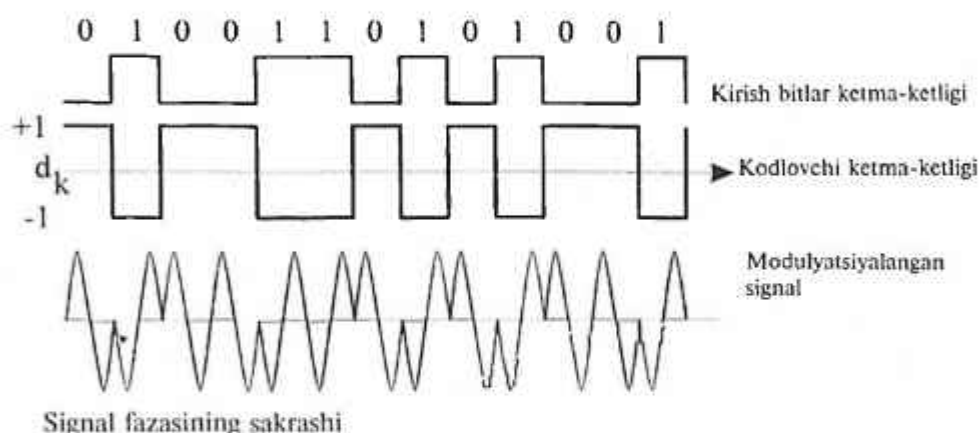
6.1-rasm. BFM (BPSK)ning ikkilik faza modulyatsiyasi.
