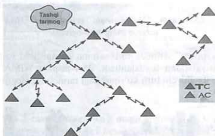
25.5-rasm. “Mesh” rejimida WiMAX tarmog‘i topologiyasi.
