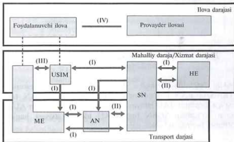
23.2-rasm. LTE/SAE tarmog'ida axborot xavfsizligining tashkil etilishi.
