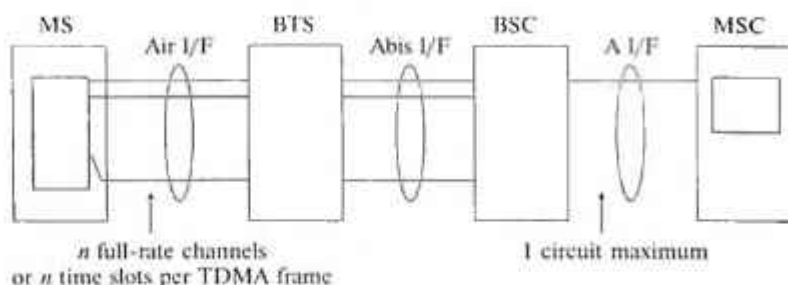
1.5-rasm. HSCSD tizimli arxetekturasi.
