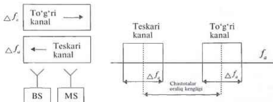
9.4-rasm. Chastotalarni dupleksli tarqoqlash prinsipida tashkillashtirish.
