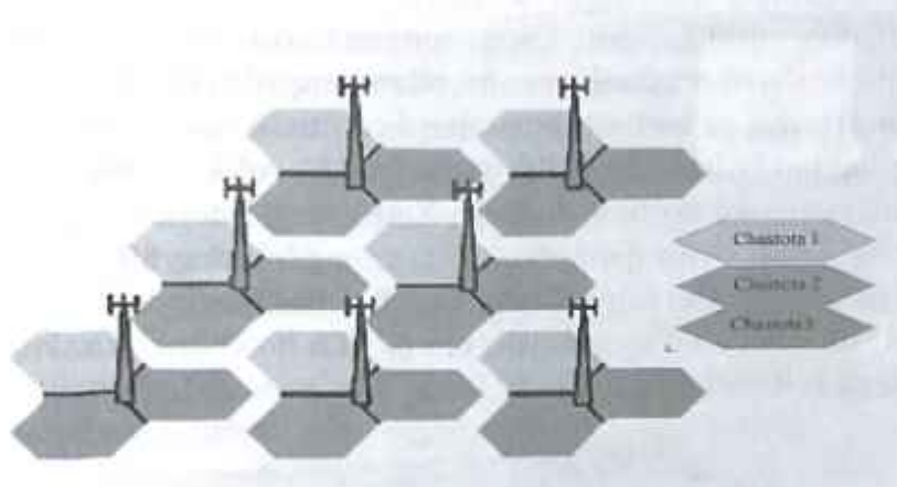
33.2-rasm. WiMAX tarmog'ining sektorli arxitekturası.
