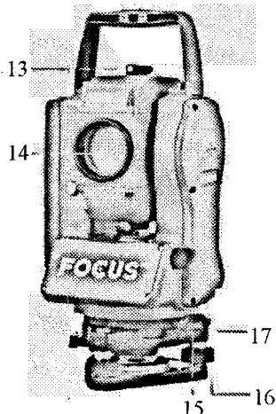
17-rasm. Focus 4 elektron taxeometrining tashqi ko'rinishi va asosiy qismlari:
