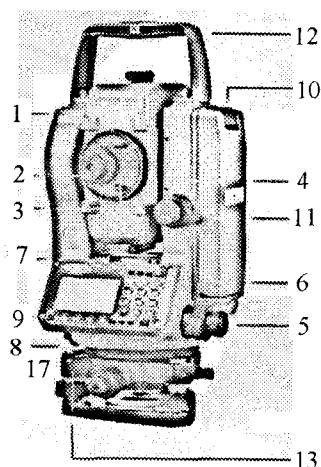
17-rasm. Focus 4 elektron taxeometrining tashqi ko'rinishi va asosiy qismlari:
