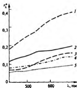
1.5-rasm. Turli xil tuproqlarning nur qayatarish xususiyatlari. 1- serozyom, 2- sod-podzolik, 3- qorong'u kashtan, 4- to'q kulrang o'rmon, 5 chermozem
