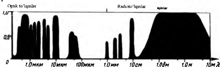
1.7-rasm. Oddiy sharoitlarda 1,5 km balandlikgacha atmosfera qatlamining tiniqligi tufayli turli uzunlikdagi to'qinlarning atmosferadan o'tish qobiliyati
