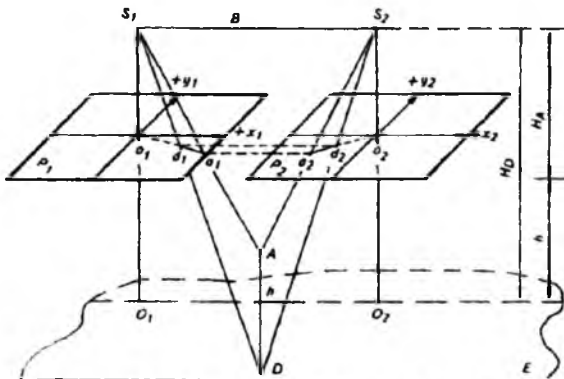
3.5. Nuqta bo'ylama parallaksining o'zgarishi
