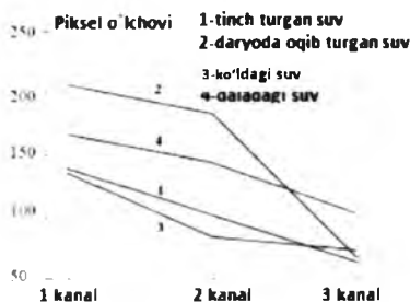
2.14-rasm. Turli holatdagi suvning spektral qiyofasi. 1 kanal – 0,5–0,6 мкм, 2 kanal – 0,6–0,7 мкм и 3 kanal – 0,8–0,9 мкм
