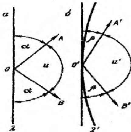
10-rasm. Ikki ta yoʻnalish oʻrtasidagi Burchak: a – yuzada; b – tekislikda
