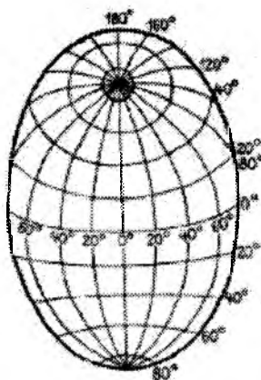
49-rasm. Atlantika okeani kartasi uchun ishlab chiqilgan qiyshiq psevdoozimal proyeksiya
