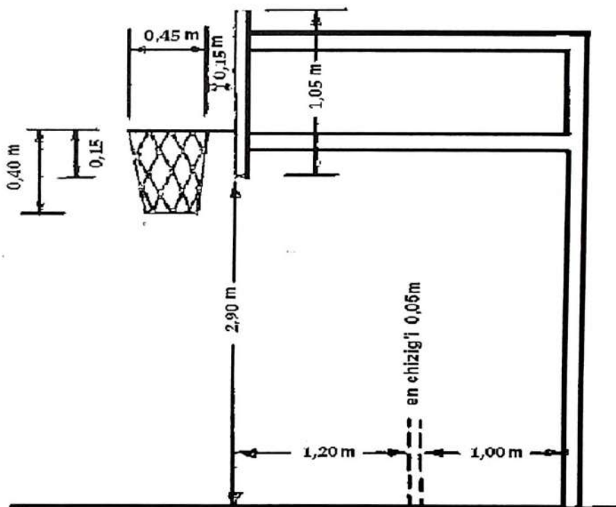
1-rasm. Halqa shi qurilmasi.
