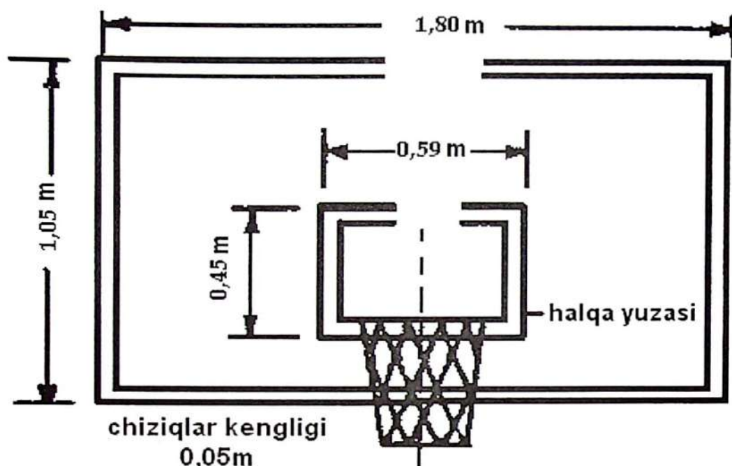
2-rasm. Shit. Uning o'lchovlari.
