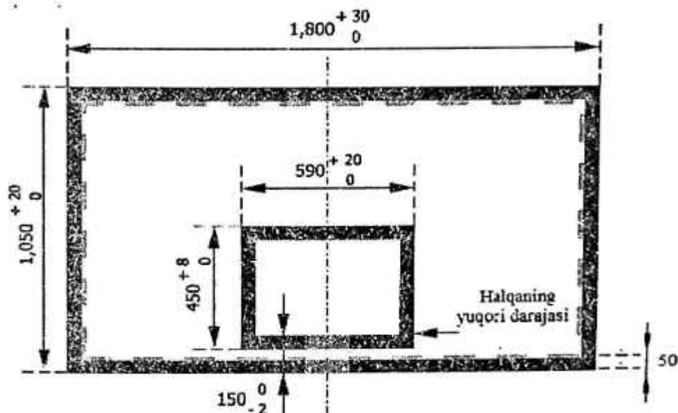
88-rasm. "Shchit" (savat ortidagi to'siq) o'lchamlari
