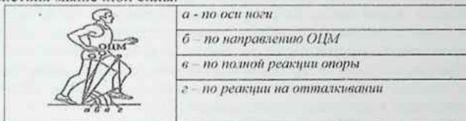
Рис. 5. Углы отталкивания
