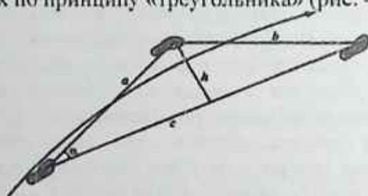
Рис. 40. Треугольник разбега
