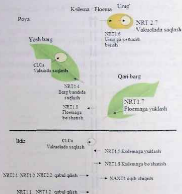
69-rasm. Arabidopsis o'simligida nitrat tashilishining sxematik tasviri. Dechorgnat va boshqalar. (2011) Oksford Universitet matbuotidan.
