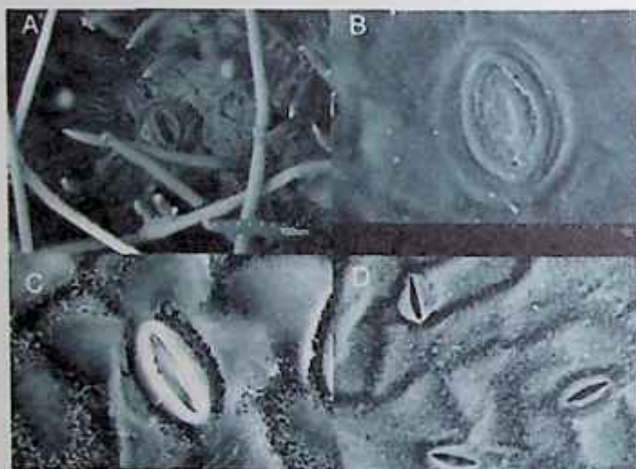
33-rasm. Barg yuzasidagi barg og'izchalarning skanerlash elektron mikrofigi. A) shaftoli mevasi B) olcha mevasi C) atirgul va D) brokkoli karamining ort (abaksiyal) barg yuzasi. Fernandes (2010).
