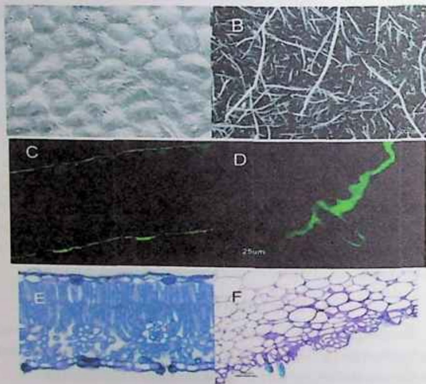
30-rasm. Shaftoli bargi va mevasining mikrografiya. Bargning sirt topografiyasi (A) va meva (B) skanerli elektron mikroskopiya ( \times 400 ). Shaftoli bargi va shaftoli mevasining ko'ndalang kesmasi auramin O bilan bo'yalagan tasviri (ultrabinafsha nurlarini kuzatish: C va D) va toluidin ko'ki bilan bo'yalgan tasviri (yorug'lik o'tkazuvchanligi: E va F). Fernandes, Lopez-Kasado E: E. Dominguez.
