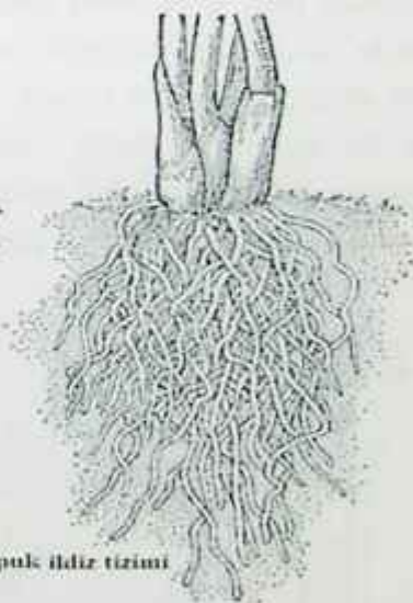
11-rasm. Ildiz tizimi tiplari.
