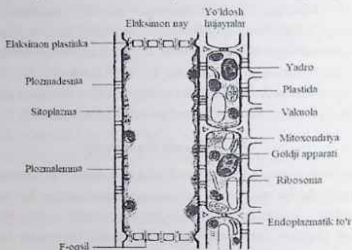
64-rasm. Elaksimon nay va yo'ldosh hujayralarning tuzilishi.
