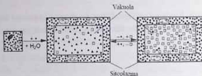
82-rasm K va boshqa eritmalarning hujayra kengayishi va osmoregulyatsiyadagi roli. ●-K; □-qaytaruvchi shakar, saxaroza, Na + ; ▲- organik kislota anionlari. Marschner (2012).
