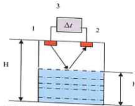
59-rasm. Radioto'liqlik sath balandligini o'lchagich sxemasi.
