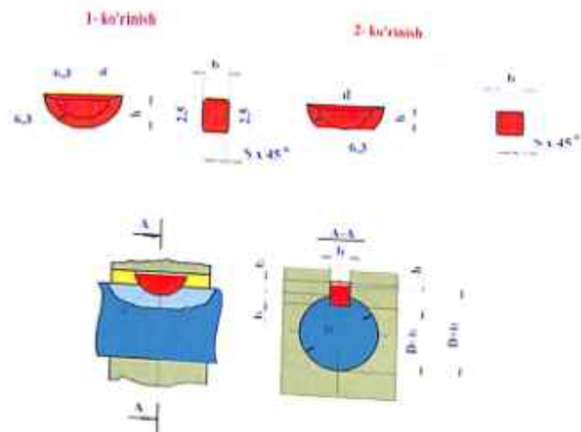
102-rasm. Segment shponkali birikmaning parametrlari.
