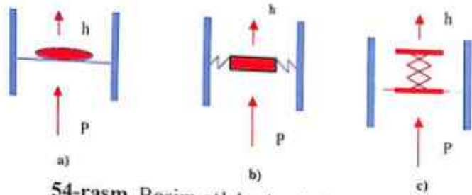
54-rasm. Bosim o'lchash asbobi sxemasi. a) va b) yassi membranali, c) prujinali
