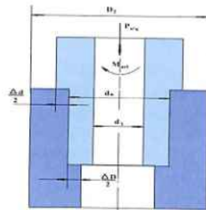
84-rasm. Tarang o'tqazishdagi val va teshik o'lchamlarining munosabati.
