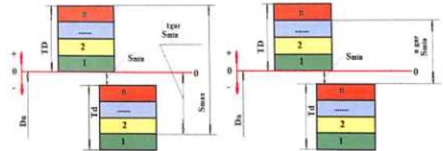
87-rasm. Selectiv yig'ishda tirqishli o'tqazishlar uchun saralash guruhlarini aniqlash sxemasi ( S_{\min}^{gur} berilgan holat uchun).
