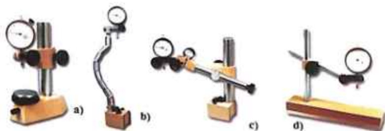
28-rasm. O'lchash kallagi uchun ustunlar va shtativlar:
