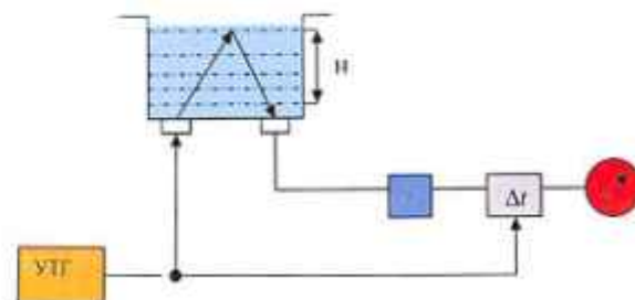
58-rasm. Ultratovushli sath balandligini o'lchagich sxemasi.
