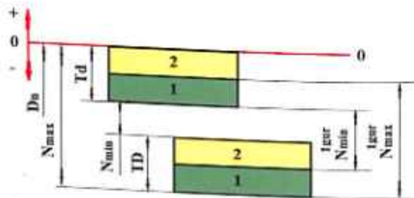
86-rasm. Selectiv yig'ishda tarangli o'tqazish uchun saralash guruhlarini aniqlash sxemasi ( TD = Td ).
