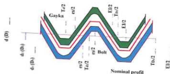
115-rasm. Tirqishli o'tqazishdagi bolt va gayka metrik rezbalari joizlik maydonlarining joylashishi.
