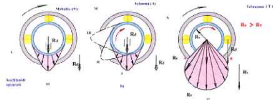
97-rasm. Podshipnik xalqalarining yuklanish turlari. a) tashqi xalqa aylanma, ichki xalqa mahalliy yuklanishda. b) tashqi xalqa mahalliy, ichki xalqa aylanma yuklanishda. v) tebranma yuklanish.
