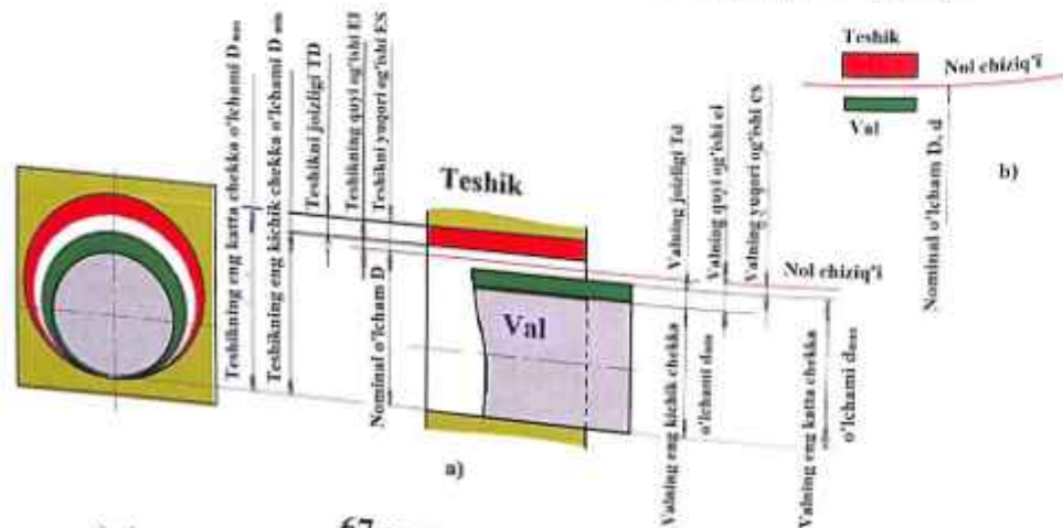
67-rasm. Joizlik maydonlari. a) tirqishli o'tqazma uchun teshik va valning joizlik maydonlarining joylashishi; b) joizlik maydonlarining grafik tasviri.
