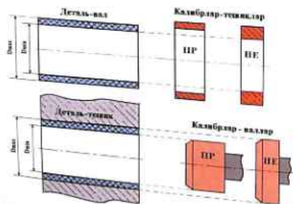
47-rasm. O'tuvchi va o'tmaydigan kalibrlarning prinsipial sxemasi.
