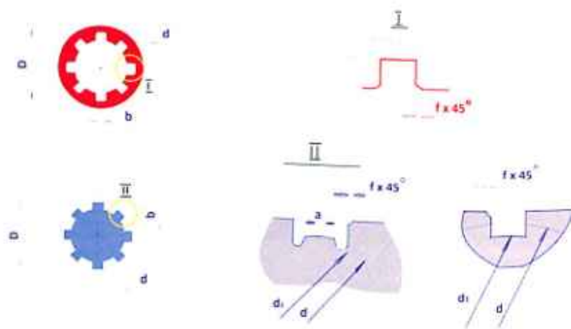
106-rasm. Shlitsali birikmalarning asosiy o'lchamlari.
