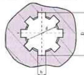
107-rasm. Tashqi diametr "D" bo'yicha markazlashtirish sxemasi.
