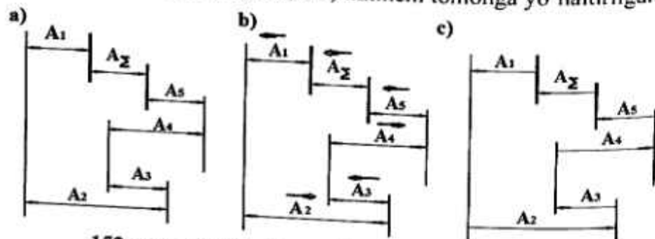
152-rasm. O'lchamlar zanjirlari bo'g'inlarini tartiblash. Harflar ustidagi strelkalar o'miga bo'g'in o'lchamining bir tomoniga strelka qo'yib belgilash o'lchamlar zanjiri sxemasiga ancha aniqlik kiritadi (152-rasm, c).
