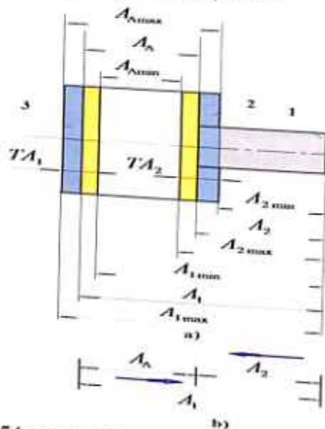
154-rasm. Uch zvenoli o'lchamlar zanjiri.
