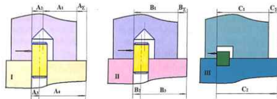
153-rasm. Tirqishli birikmada o'lcham zanjirlari.
