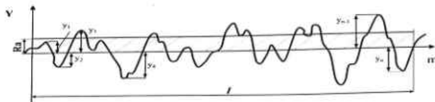
138-rasm. Profilning o'rtacha arifmetik chetga chiqishi (R a ).
