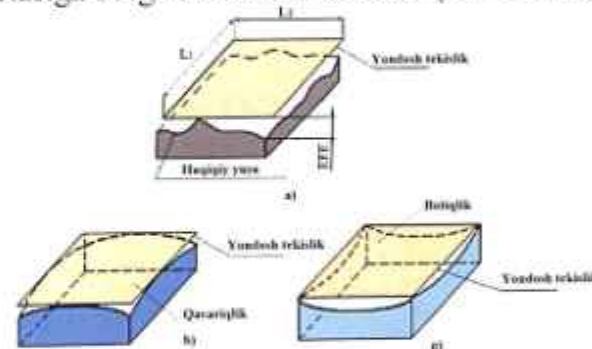
131-rasm. Yassilikdan og'ishi.
