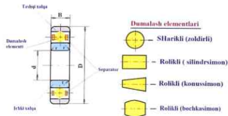
94-rasm. Dumalash podshipnigining tuzilishi, o'lchamlari va elementlari.
