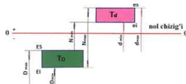
72-rasm. Tarangli birikma va uning joizlik maydoni joylashish sxemasi.
