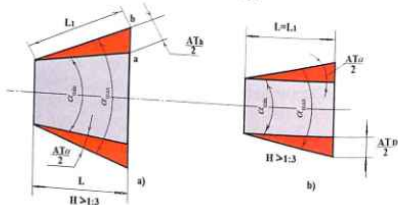
92-rasm. Burchak o'lchamlari joizligi va ularning belgilanishi.
