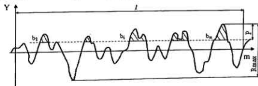
143-rasm. Profilning nisbiy tayanch uzunligi t_p
