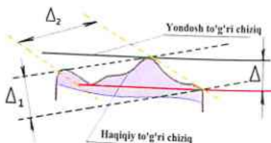
126-rasm. To'g'ri chiziqlik.
