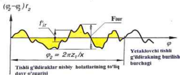
119-rasm. Tishli uzatma kinematik xatoligining egri chizig'i.
