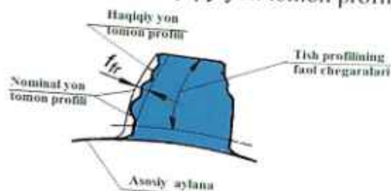
123-rasm. Tish profilning xatoligi.
