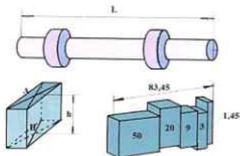
42-rasm. Uzunlikning yassi- parallel uch olchovlari (UYAPUO').
