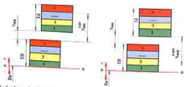
89-rasm. Selektiv yig'ishda tarang o'tqazishlar uchun saralash guruhlarini aniqlash sxemasi ( N_{\min}^{\text{gur}} berilgan holat uchun).
