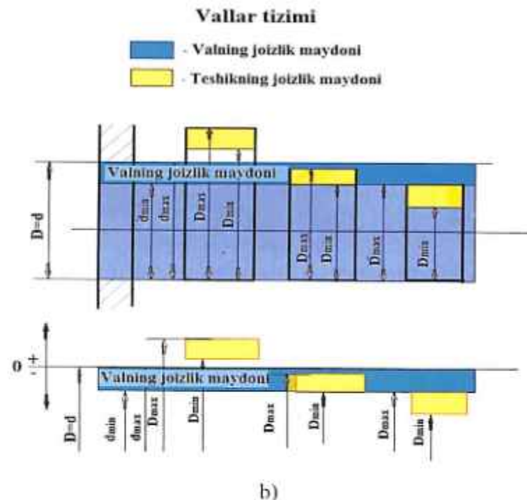
76-rasm. Teshik tizimida (a) va val tizimida (b) o'tqazishlar joizlik maydonlari.
