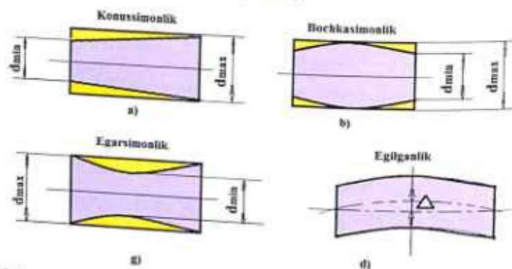
130-rasm. Silindrik detal bo'ylama kesimining og'ishlari. a) konussimonlik; b) bochkasimonlik; g) egarsimonlik; d) egilganlik.
