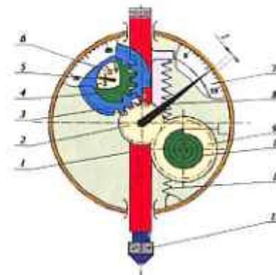
27-rasm. Soat tipidagi indikator(ICH-10)ning tuzilishi.
