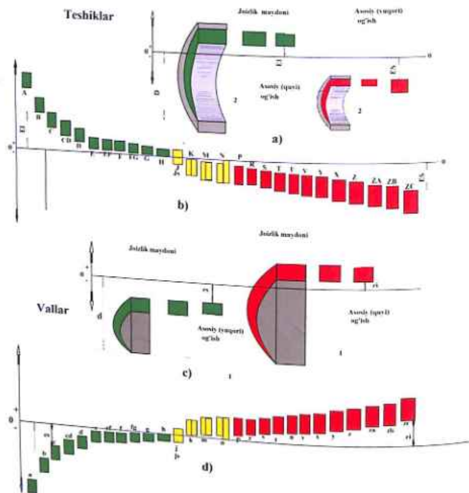
79-rasm. ISO va JO*YaT da qabul qilingan teshik hamda vallarning asosiy og'ishlari. a) va b) teshikning asosiy og'ishlari; s) va d) vallarning asosiy og'ishlari; 1-val; 2- teshik.
