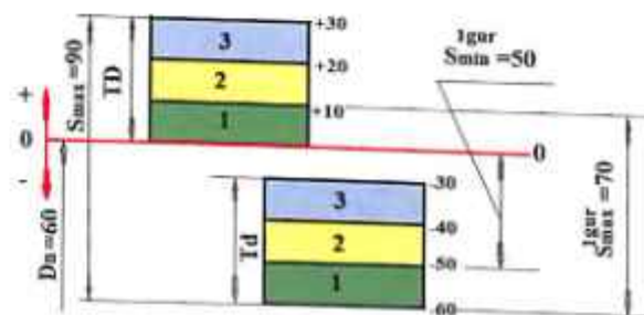
91-rasm. Selektiv tanlash usulida yig'ishga doir misol
