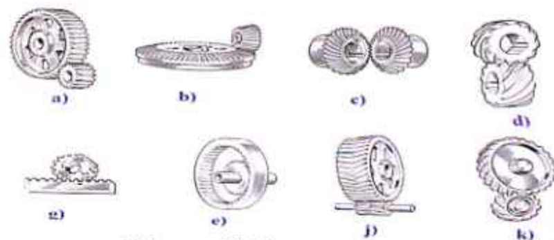
116-rasm. Tishli uzatmalarning turlari.
