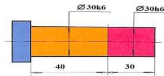
75- rasm. Joizlik maydonlari va o'tqazishlarni chizmalarda belgilash.
