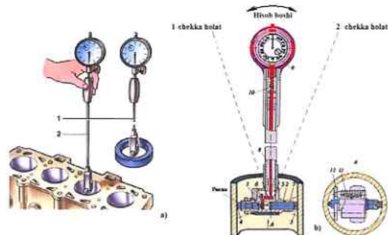
33-rasm. Indikatorli icho'lchagich bilan o'lchash va uning tuzilishi.
