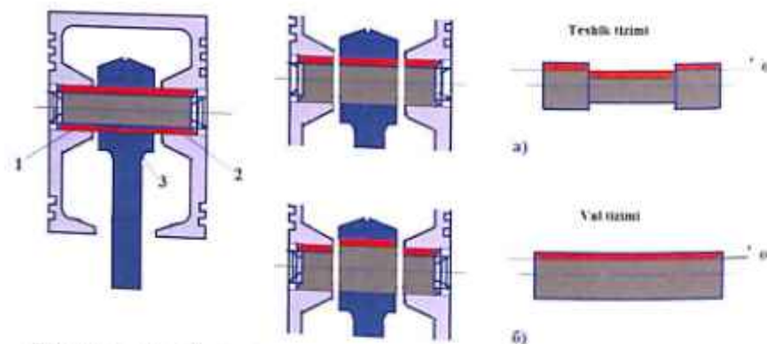
77-rasm. Val tizimining qo'llanilishiga misol (traktor, avtomobi dvigatelidagi – porshen - barmoqcha – shatun birikmasi): a) teshik tizimidagi o'tqazishlar; b) val tizimidagi o'tqazishlar.
