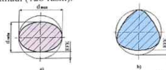
128-rasm. Yuzalarning doiraviylikdan chetga chiqishi a) ovallik; b) qirralilik.
