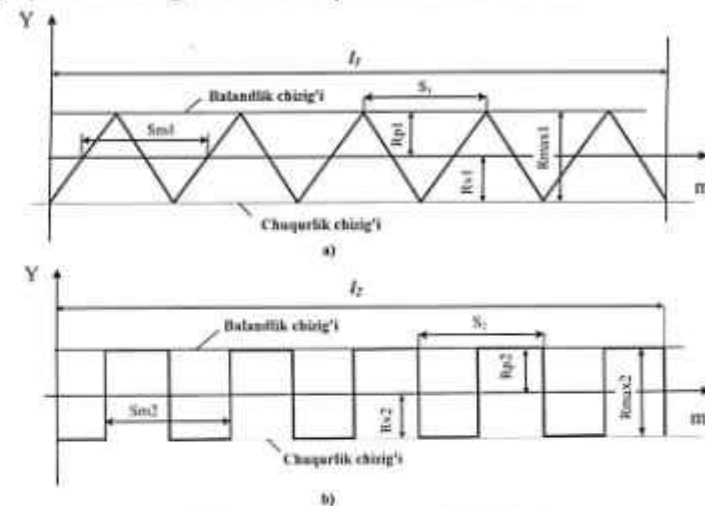
146-rasm. Yuza notekisliklari:
