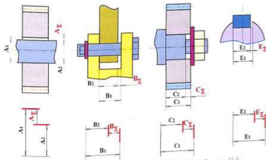
151-rasm. Yig'ma to'g'ri chiziqli o'lchamlar zanjiri.
