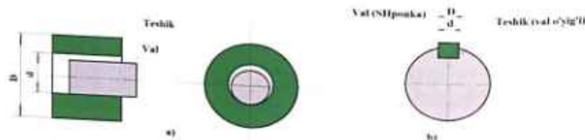
68-rasm. Qamrovchi (teshik) va qamraluvchi (val) sirtlar.
