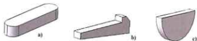
99-rasm. Shponkalar: a) Prizmatik; b) Ponasimon; c) Segment.
