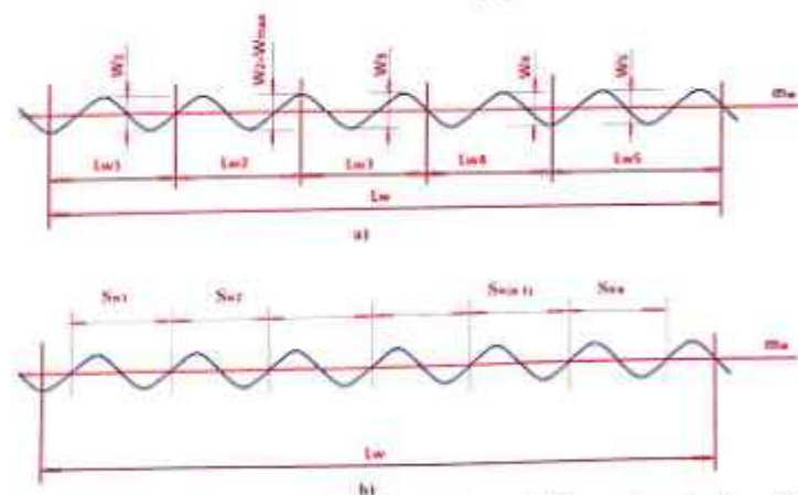
148-rasm. Yuza to'lqinsimonligi a)- to'lqinlikning balandligi, b) qadamini o'lchash
