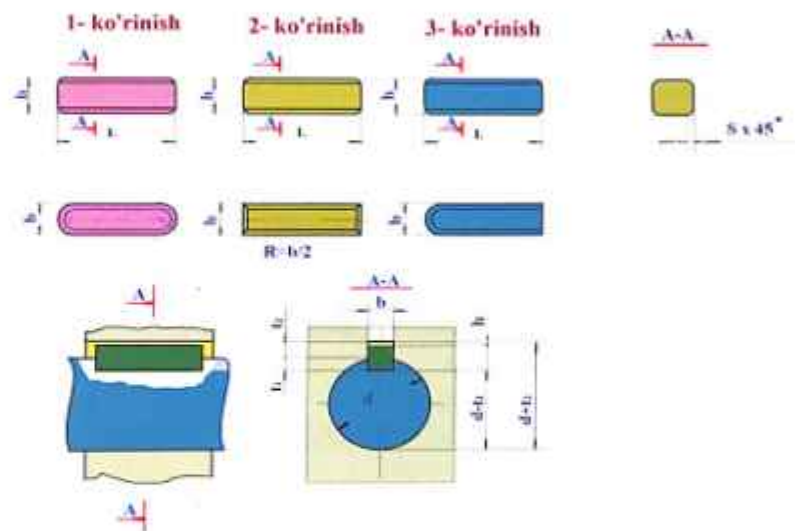
101-rasm. Prizmatik shponkali birikmaning parametrlari.
