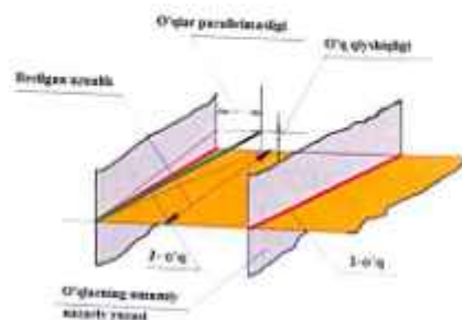
136-rasm. O'qlarning noparalellligi va qiyshayishi.
