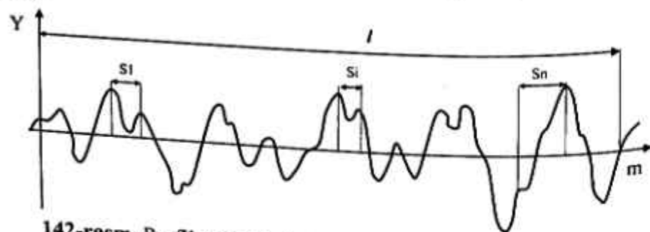
142-rasm. Profil mahalliy balandliklari bo'yicha o'rtacha qadami S
