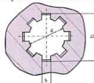
108-rasm. Ichki diametr "d" bo'yicha markazlashtirish sxemasi.
