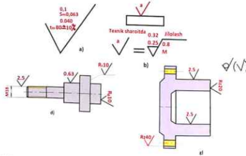
149-rasm. G'adir-budurlikning chizmada belgilanishiga misollar.
