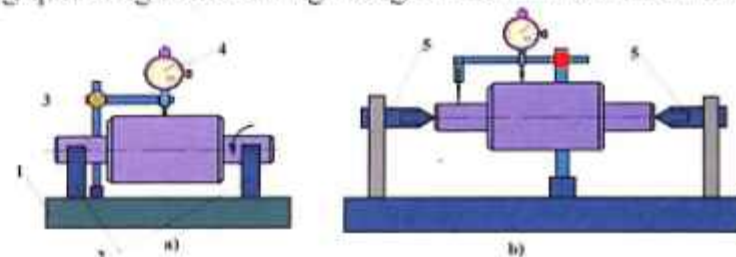
29-rasm. Indikator bilan valni radial tepishini aniqlash: a) umumiy o'qqa nisbatan; b) markaziy o'qqa nisbatan; 1- asos, 2- prizma, 3- tekshirilayotgan val, 4- indikator, 5- markazlar.
