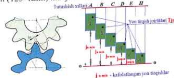
125-rasm. Silindrik tishli uzatmalarga joizlik maydonlari.
