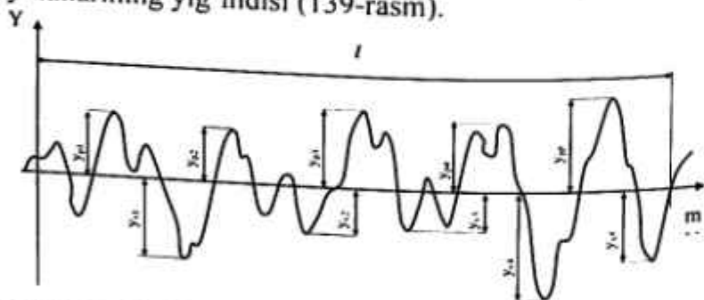
139-rasm. Profil notekisliklarining 10 ta nuqtasi bo'yicha balandligi, R_z
