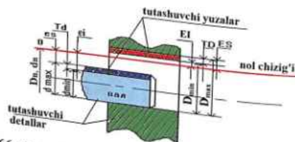
66-rasm. Og'ishlar va joizliklar aniqlash sxemasi.
