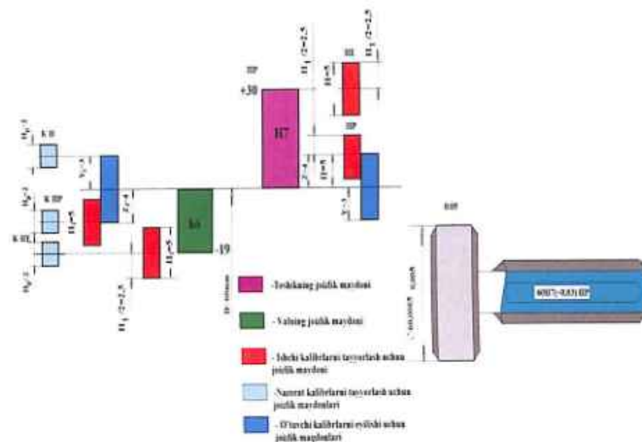
49- rasm. Joizlik maydonlari joylashish sxemasi.
