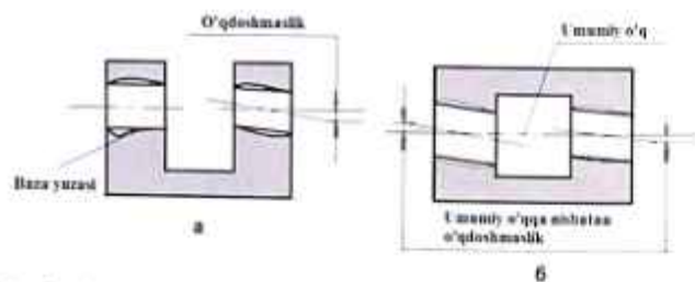
134-rasm. O'qdashmaslik a) baza yuzasiga nisbatan; b) umumiy o'qqa nisbatan.
