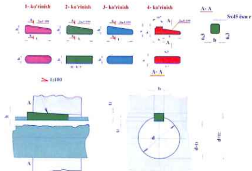
103-rasm. Ponasimon shponkali birikmaning parametrlari.
