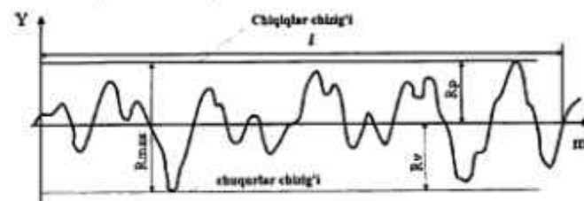
140-rasm. Profil notekisliklarining eng katta balandligi, R_{max}
