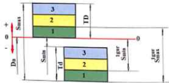
85-rasm. Selectiv yig'ishda tirqishli o'tqazish uchun saralash guruhlarini aniqlash sxemasi ( TD = Td )
